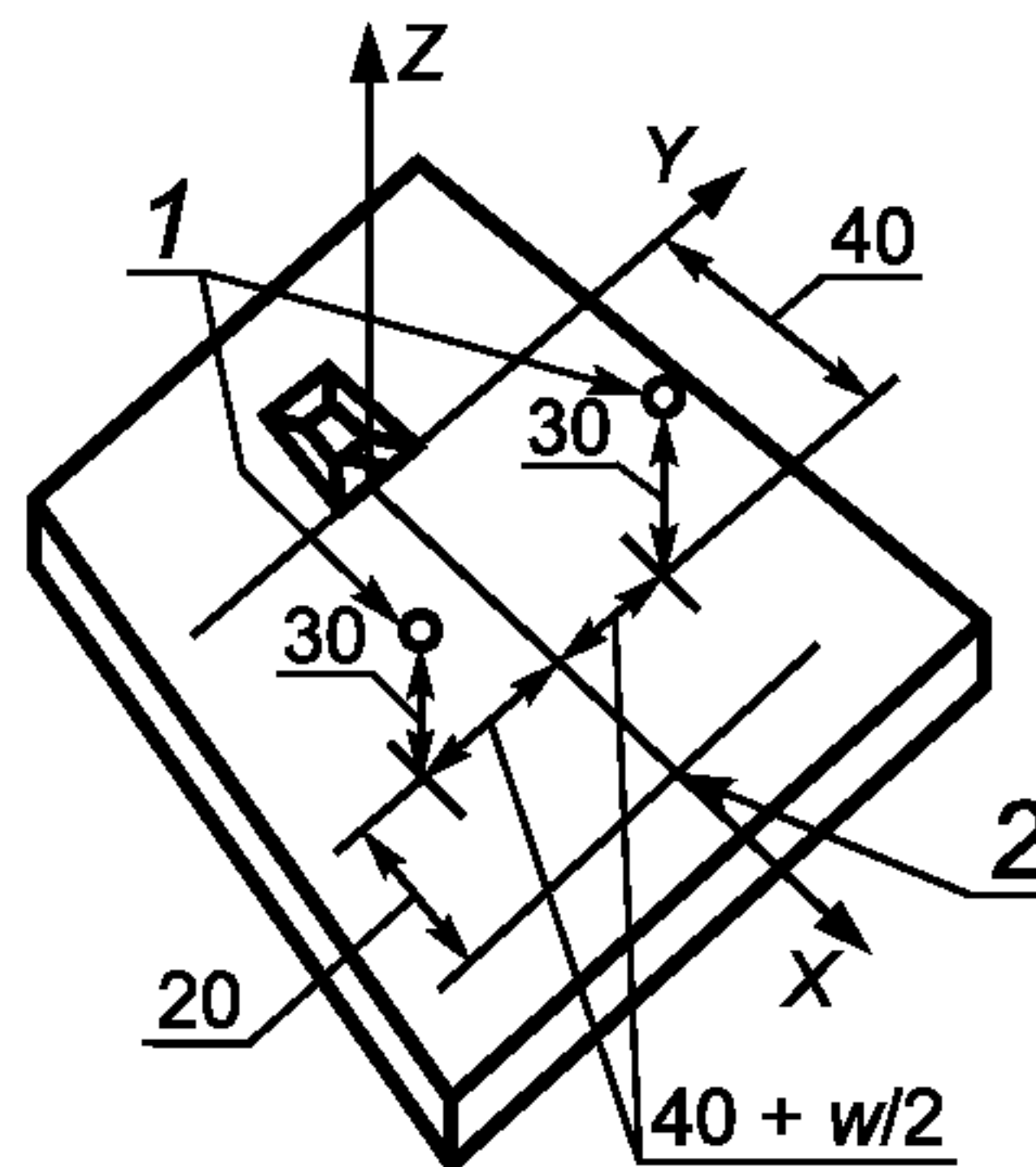
1 — микрофон; 2 — граница зоны измерений; w — ширина игрушки
