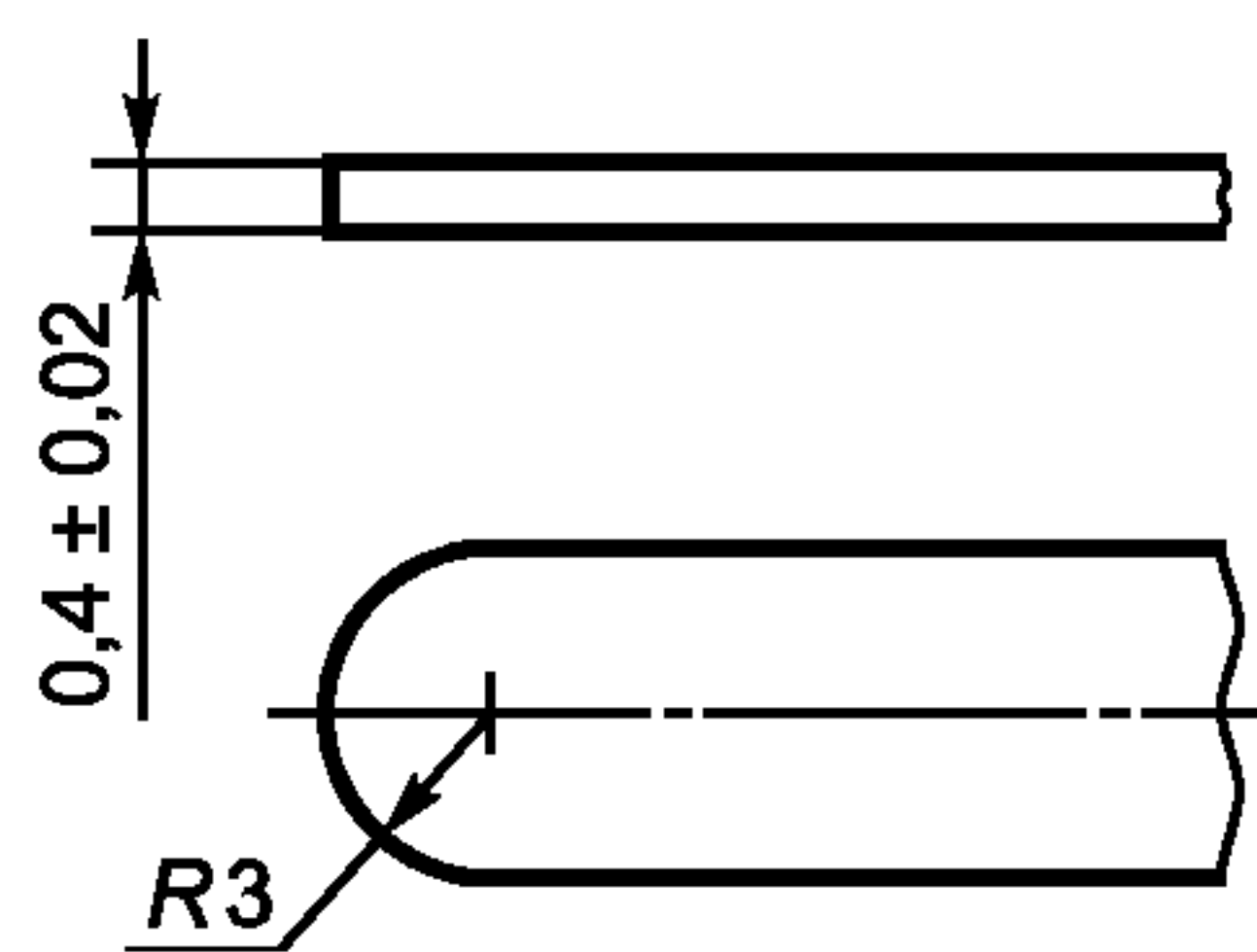
Рисунок 14 — Щуп
