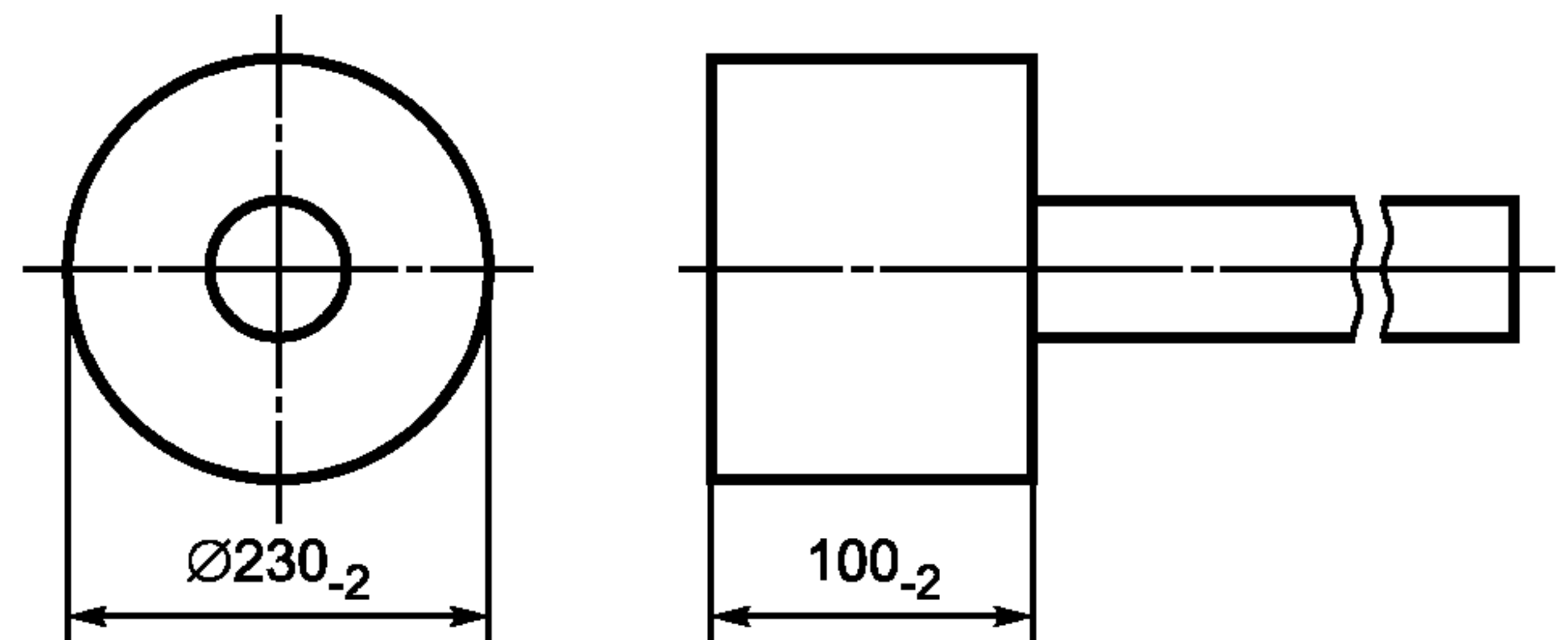
Рисунок 21 — Испытательный зонд D
