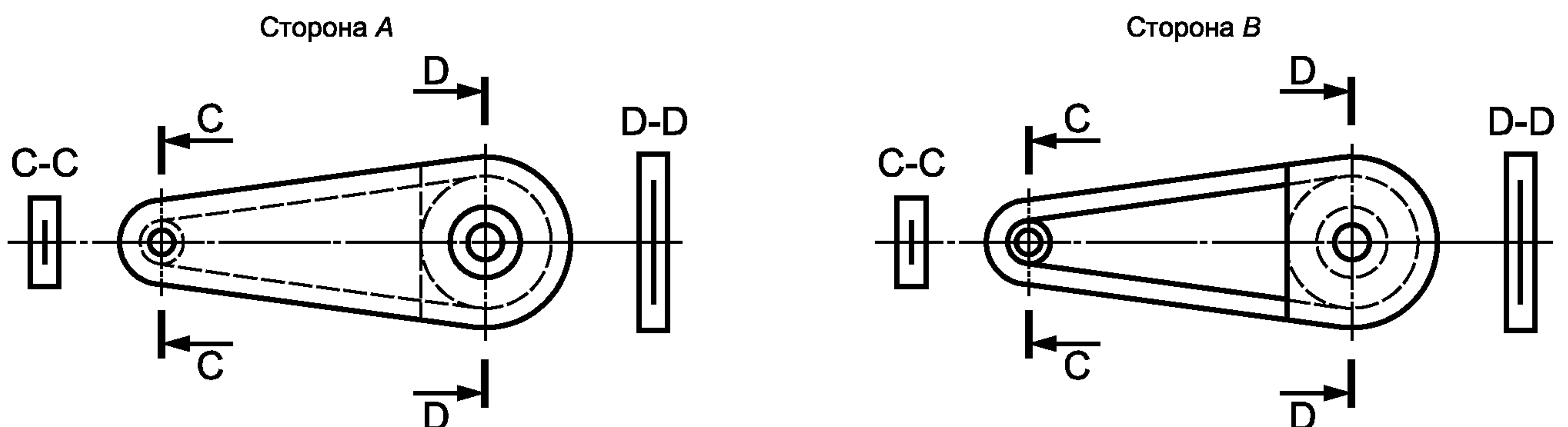
Рисунок 8 — Приводные цепи и защитные устройства цепи
