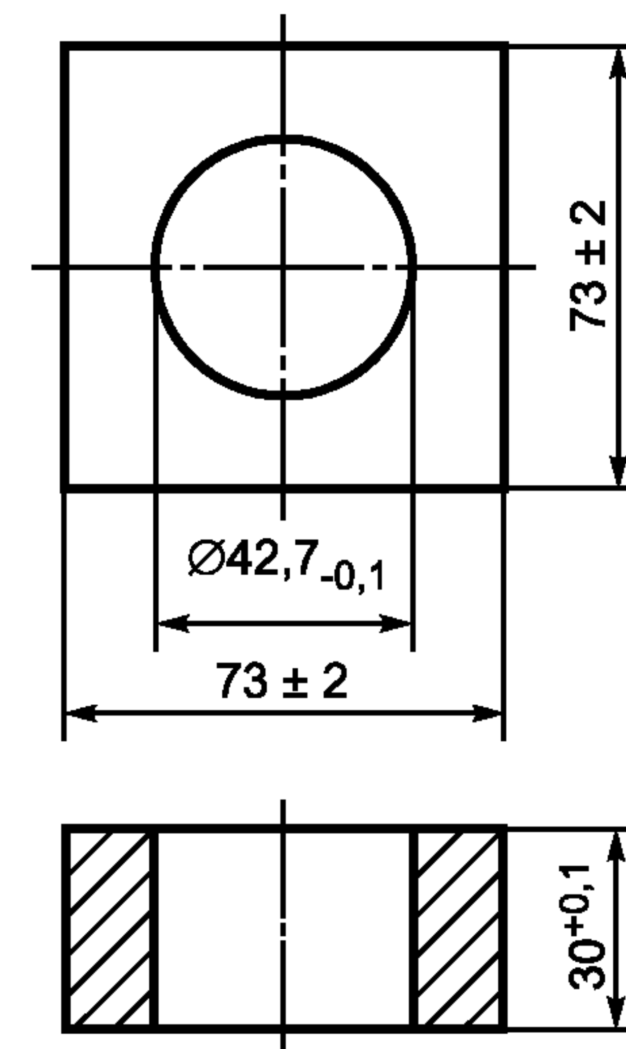
Рисунок 19 — Испытательный шаблон В
