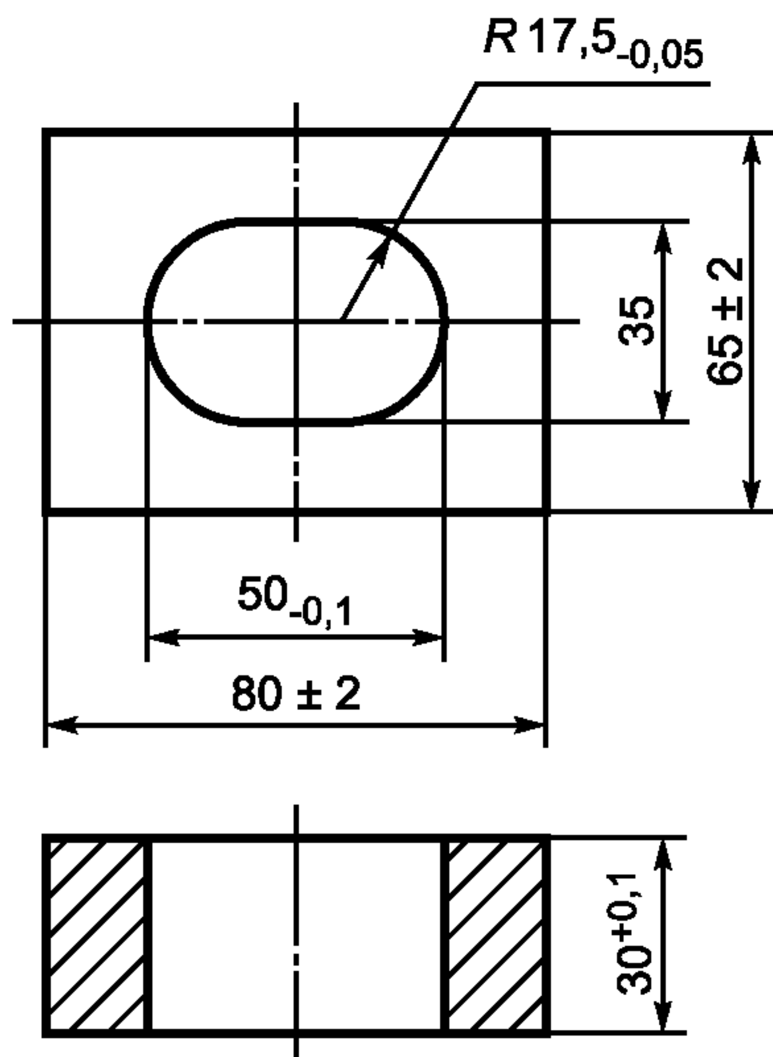
Рисунок 18 — Испытательный шаблон А
