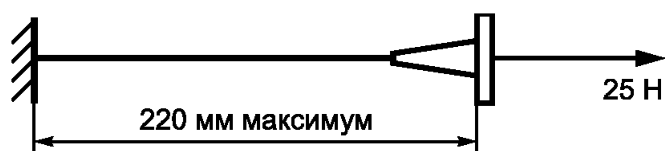
Рисунок 12 — Точки крепления шнура
