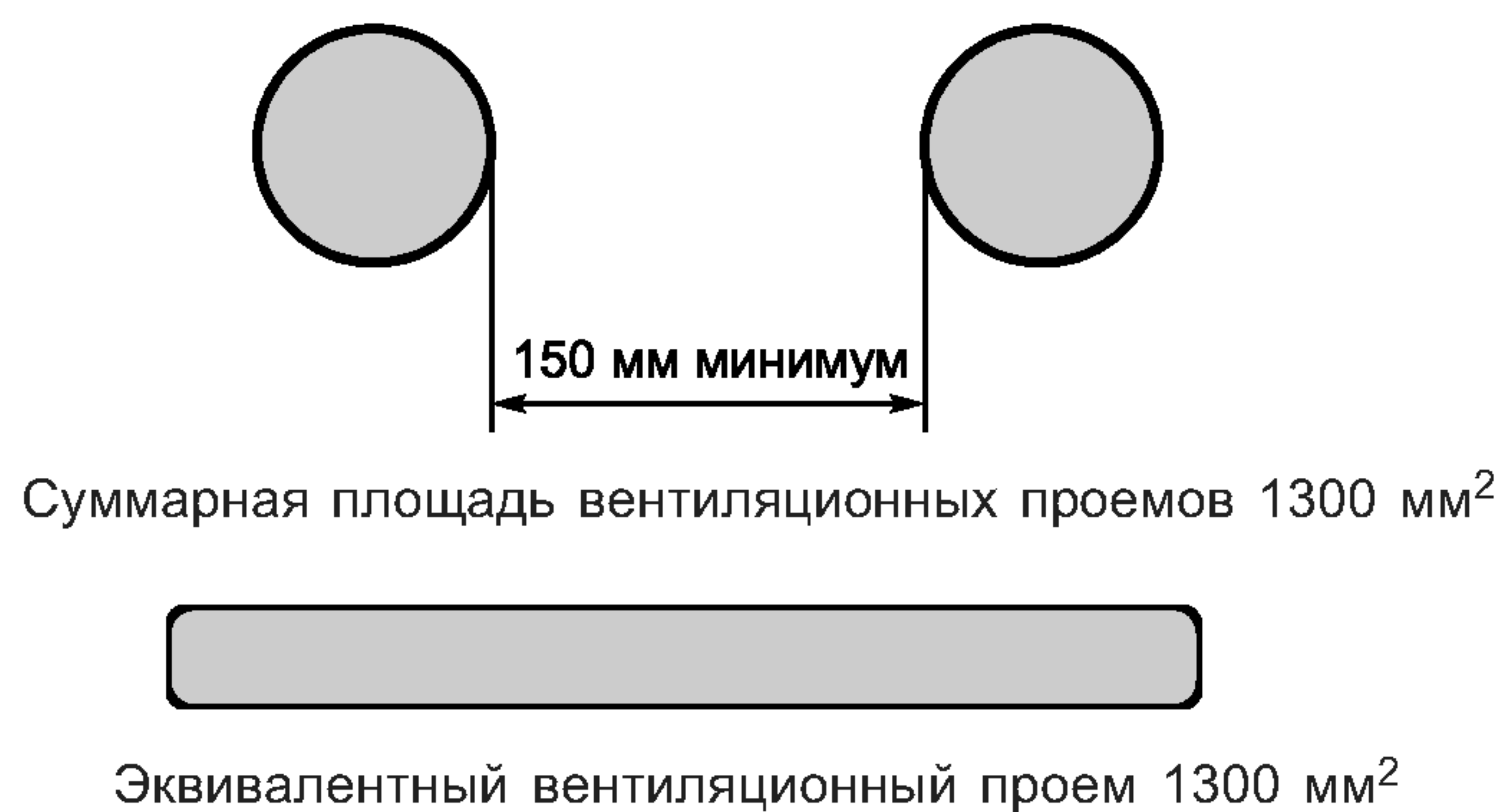
Рисунок 7— Пример разных конструкций вентиляционных отверстий
