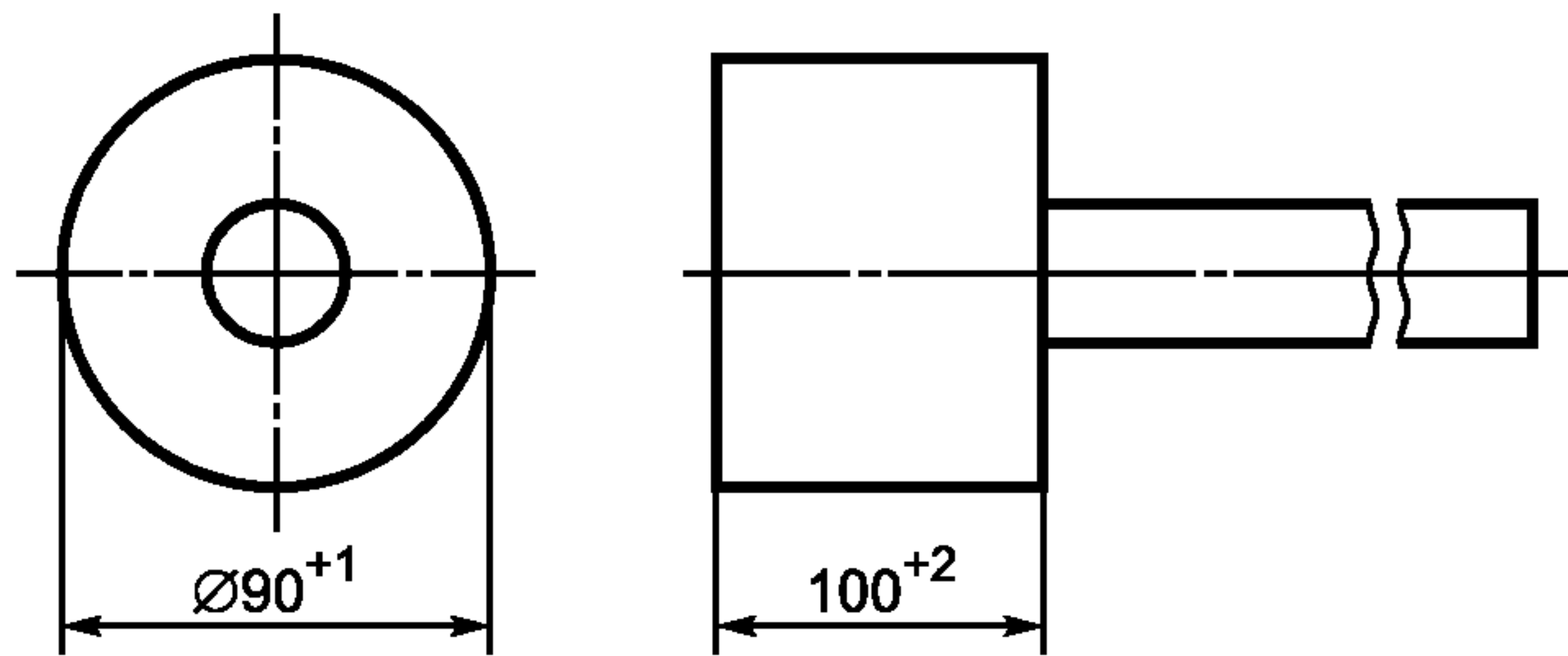
Рисунок 20 — Испытательный зонд C
