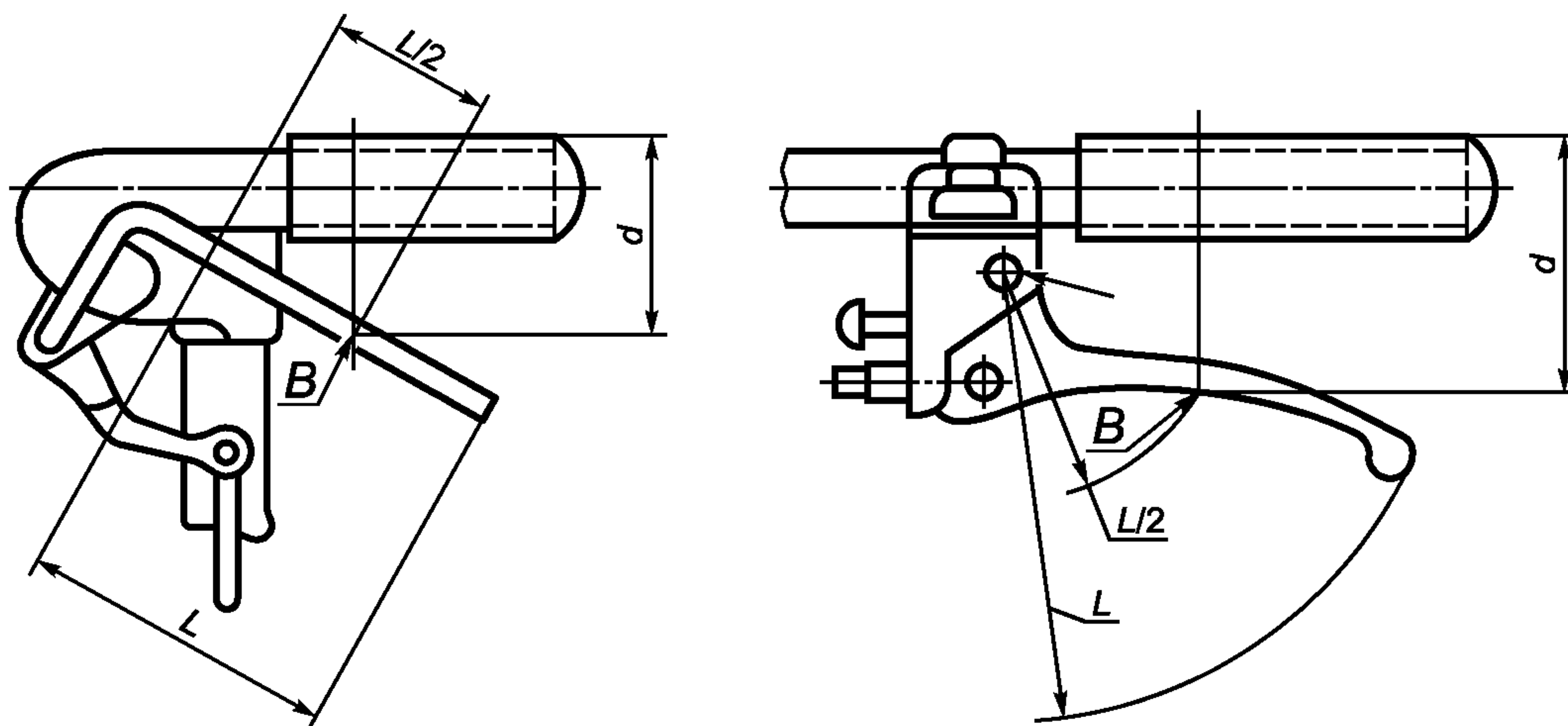
Рисунок 9 — Размеры рычага ручного тормоза
