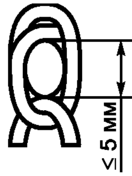
Рисунок 10 — Максимальная величина отверстия цепи качелей
