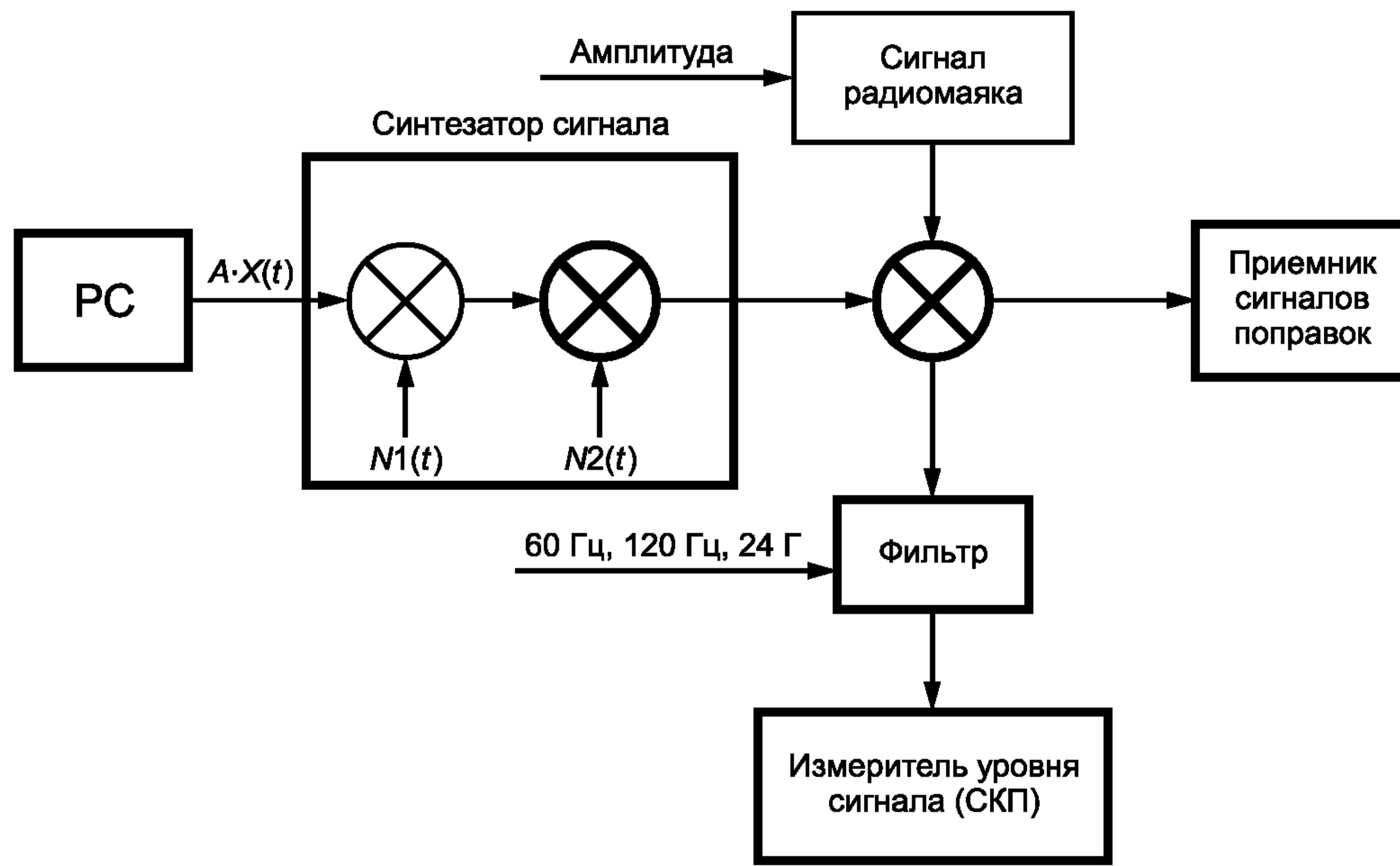
Рисунок А.2 — Схема проведения испытаний
