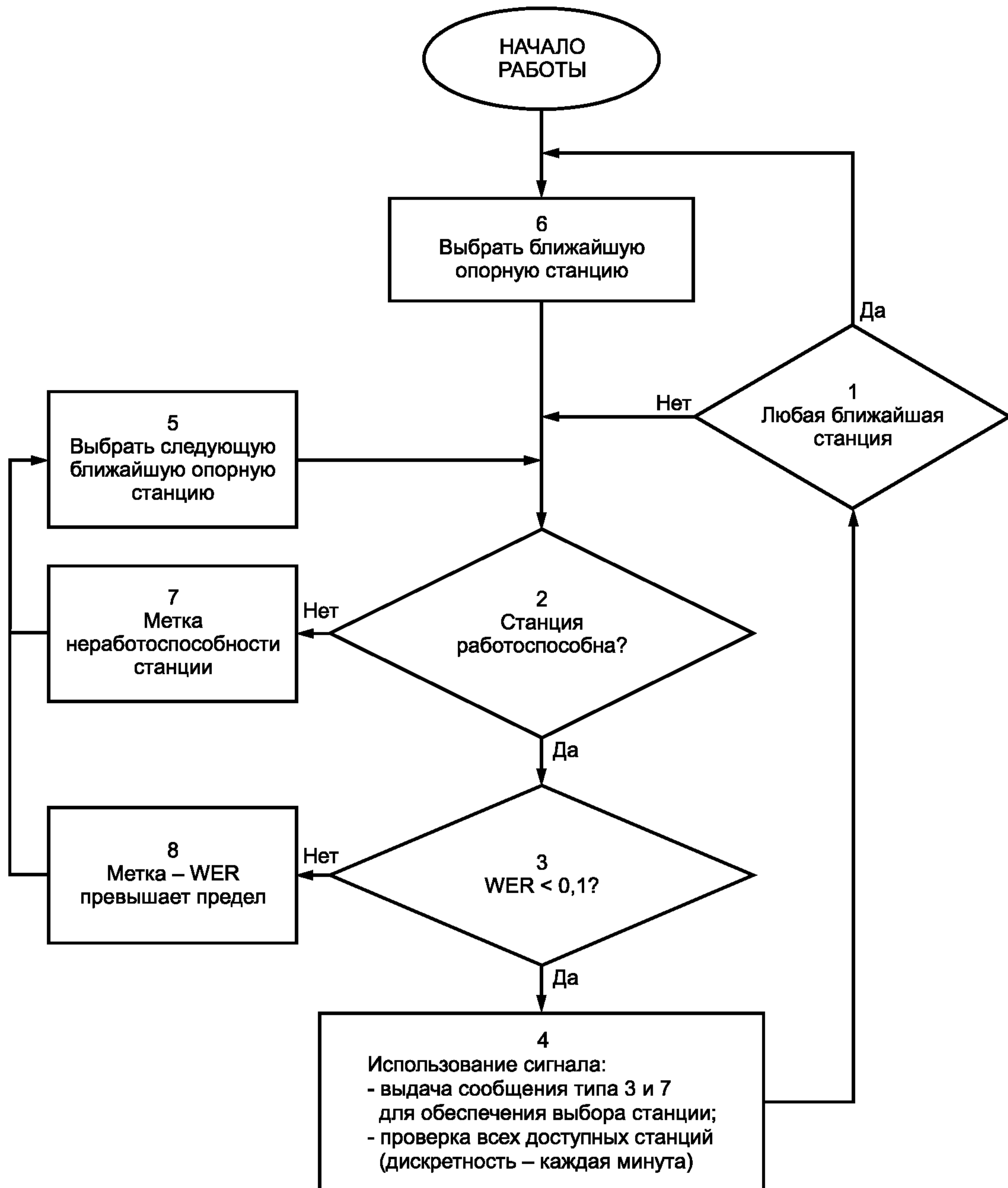
Рисунок Д.2 — Алгоритм обработки навигационных данных
