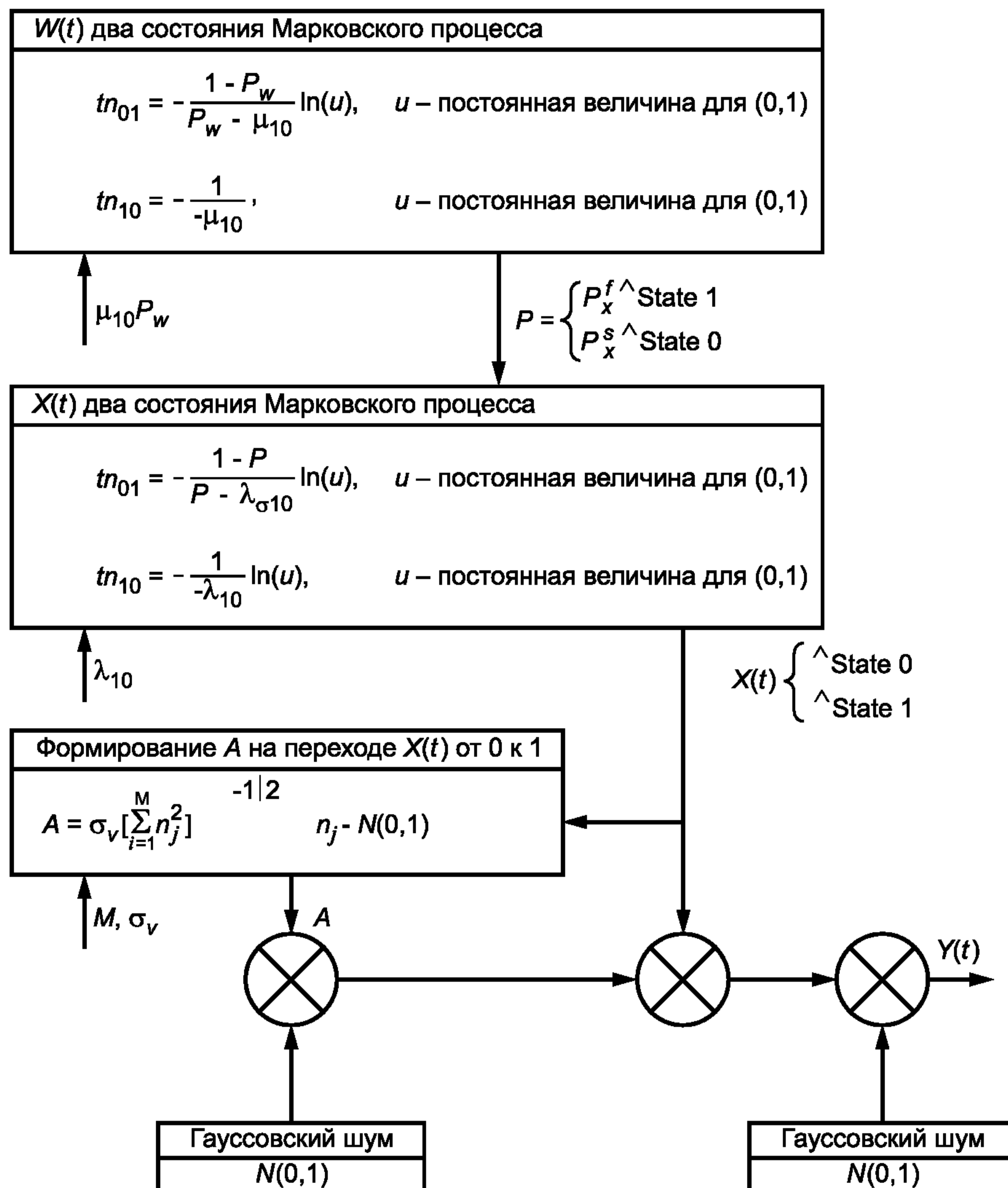
Рисунок А.1 — Модель формирования атмосферных помех
