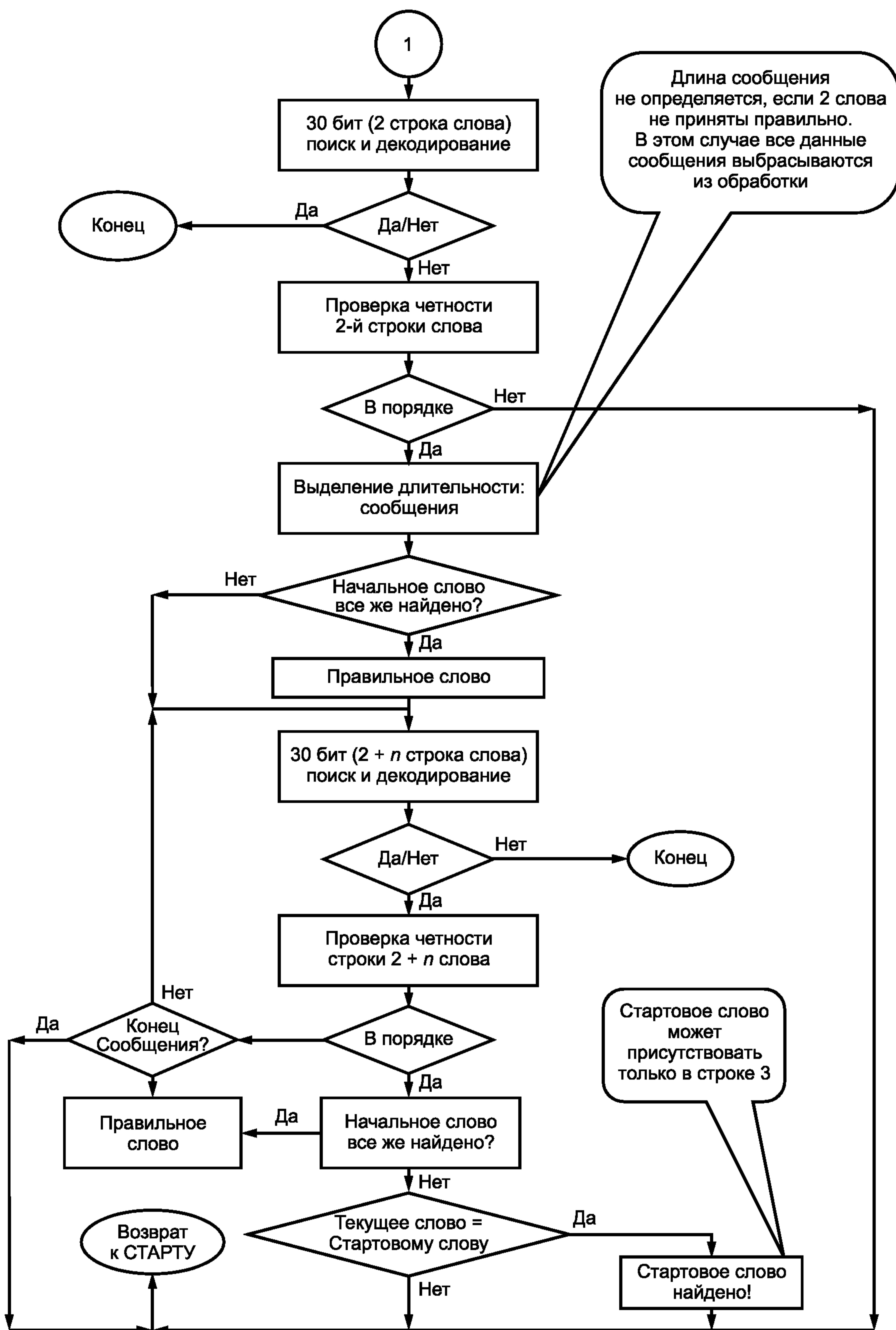
Рисунок Б.1 — Алгоритм оценки ошибки слов
