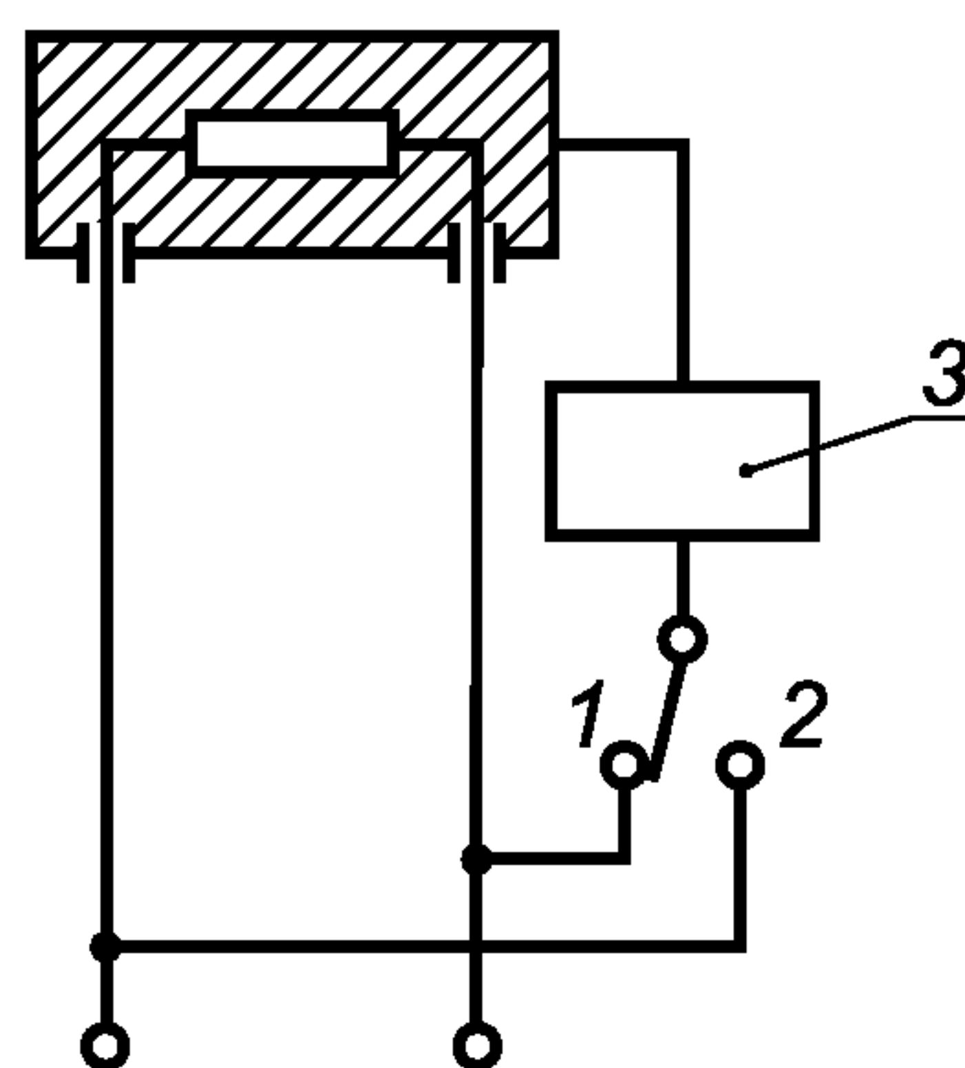
1 и 2 — входные клеммы; 3 — схема по рисунку 1
