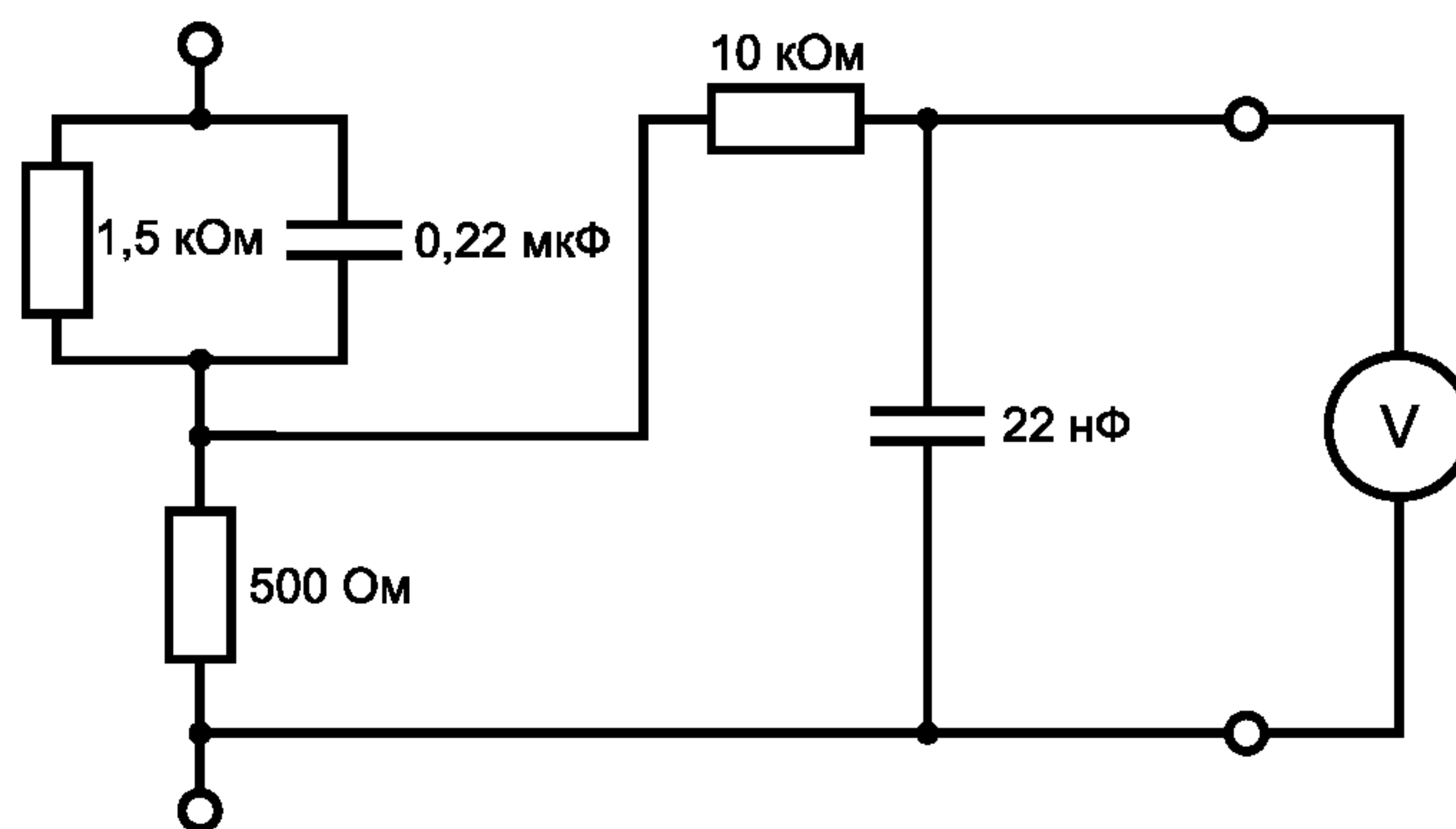
Рисунок 1 — Схема измерения тока прикосновения
