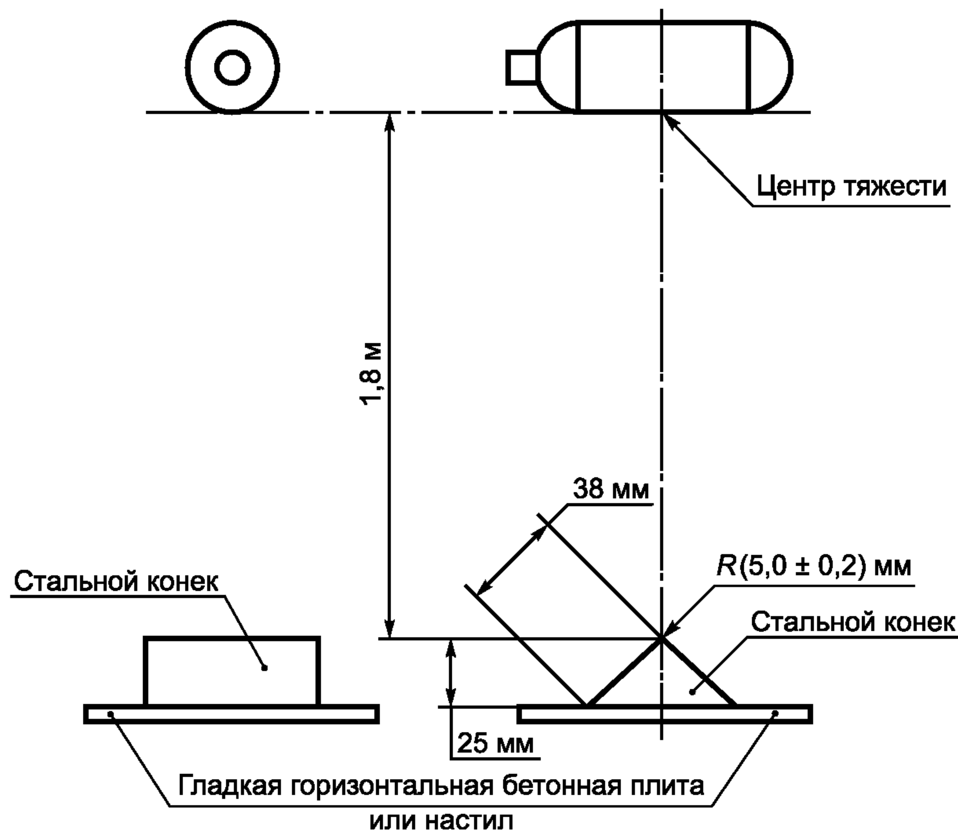
Рисунок 1 — Испытание контейнера падением на конек
