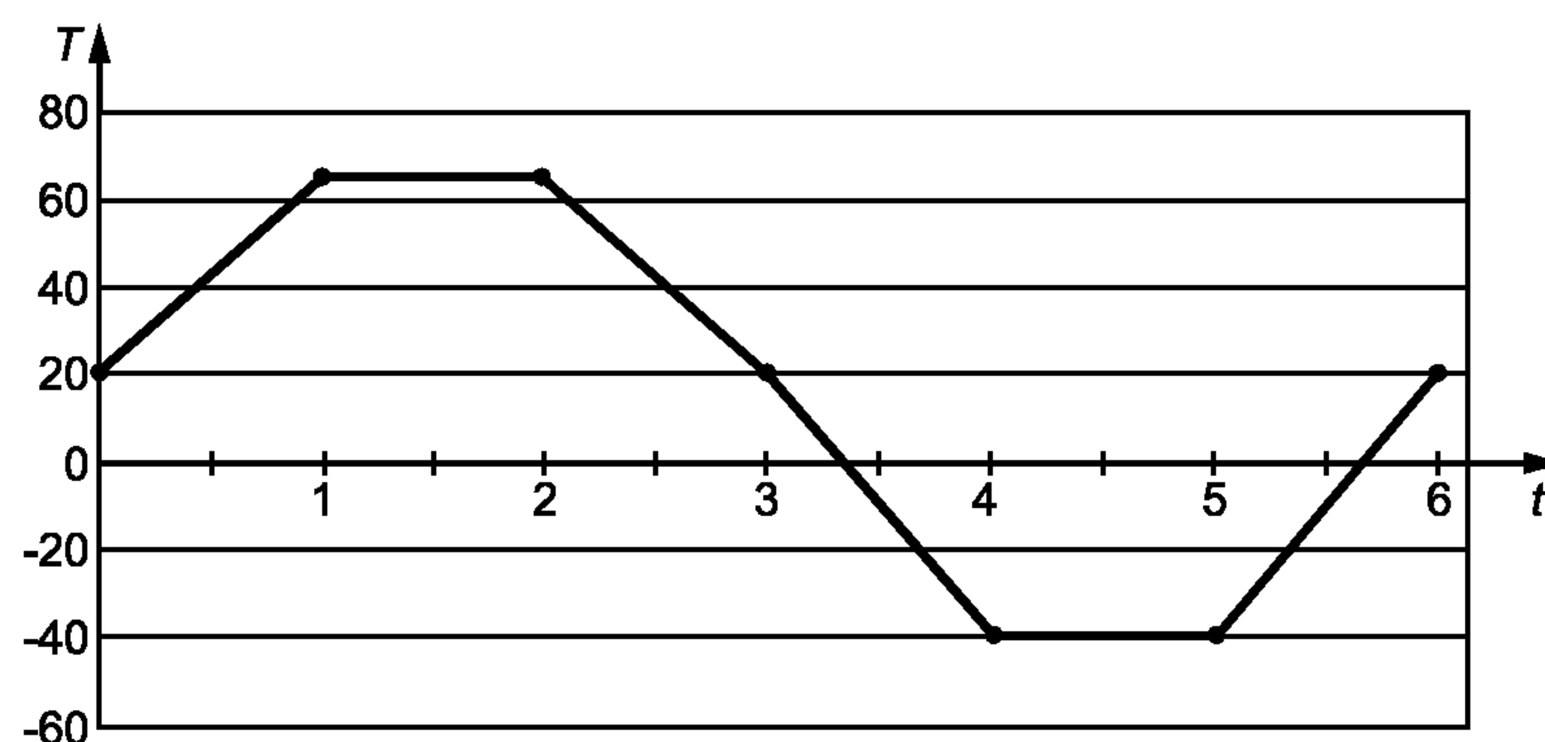
Рисунок 3 — Примерный цикл испытания на термостойкость
