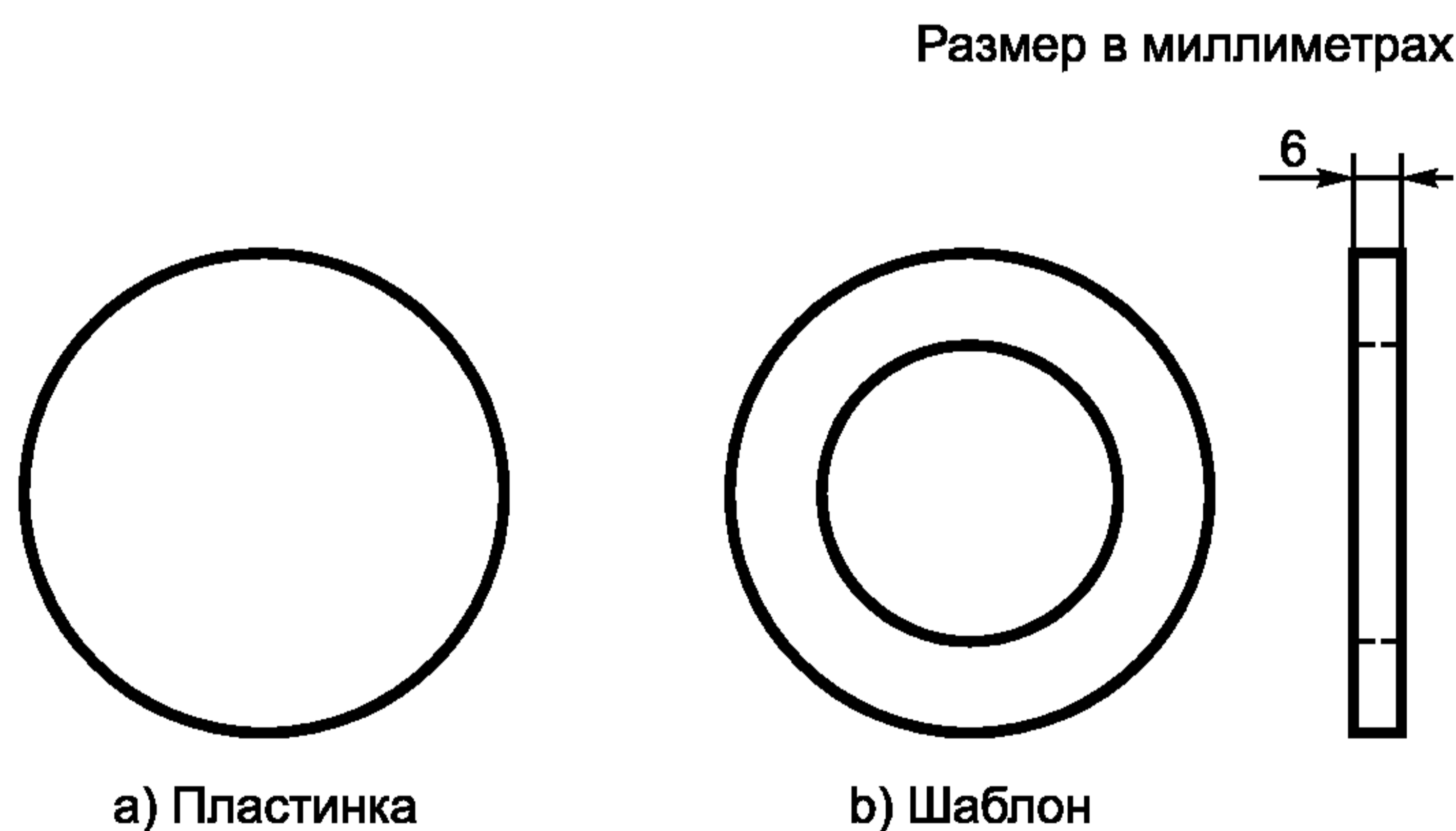
Рисунок 2 — Приспособления для испытаний на проницаемость
