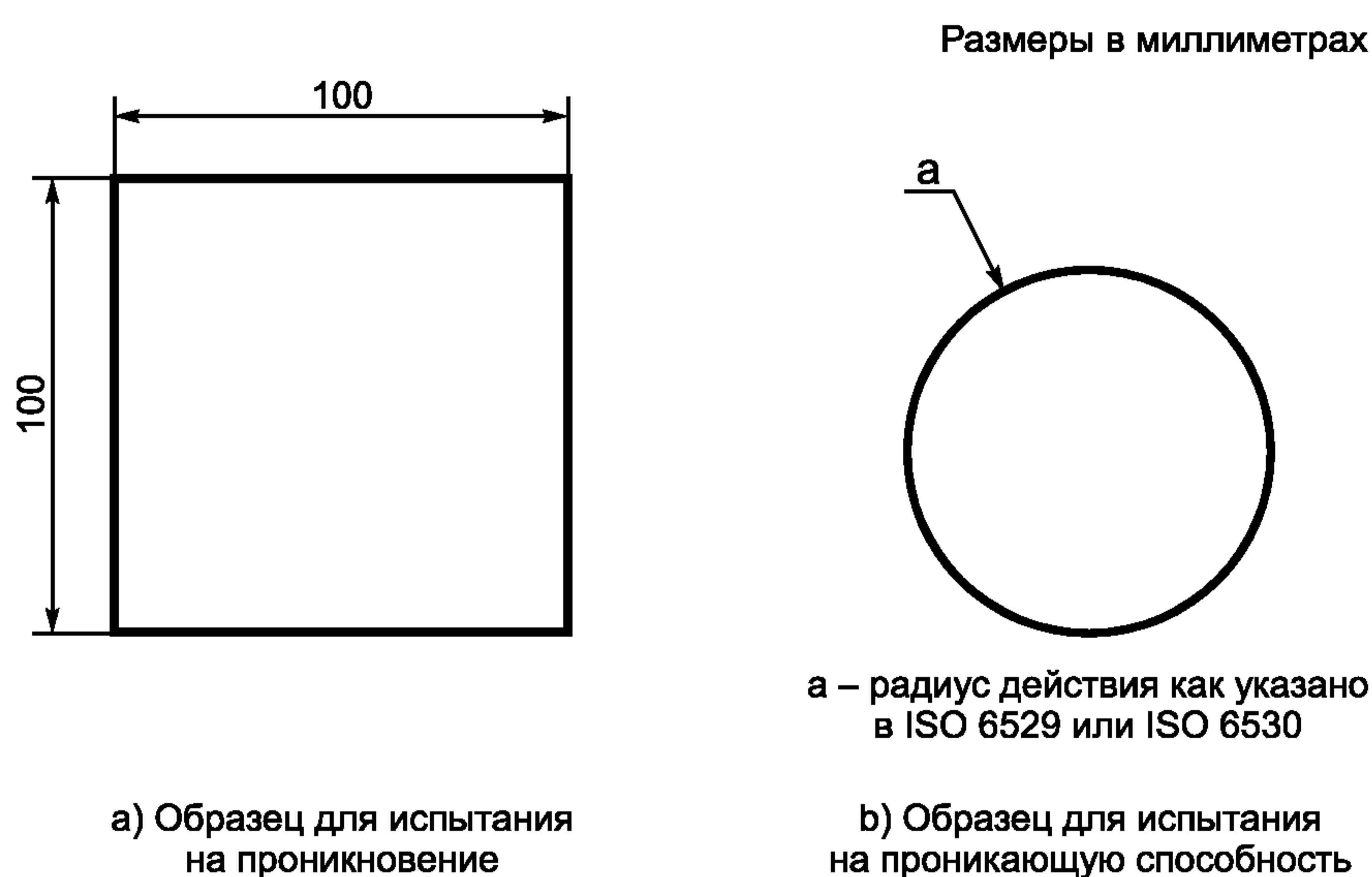
Рисунок 1 — Испытуемые образцы
