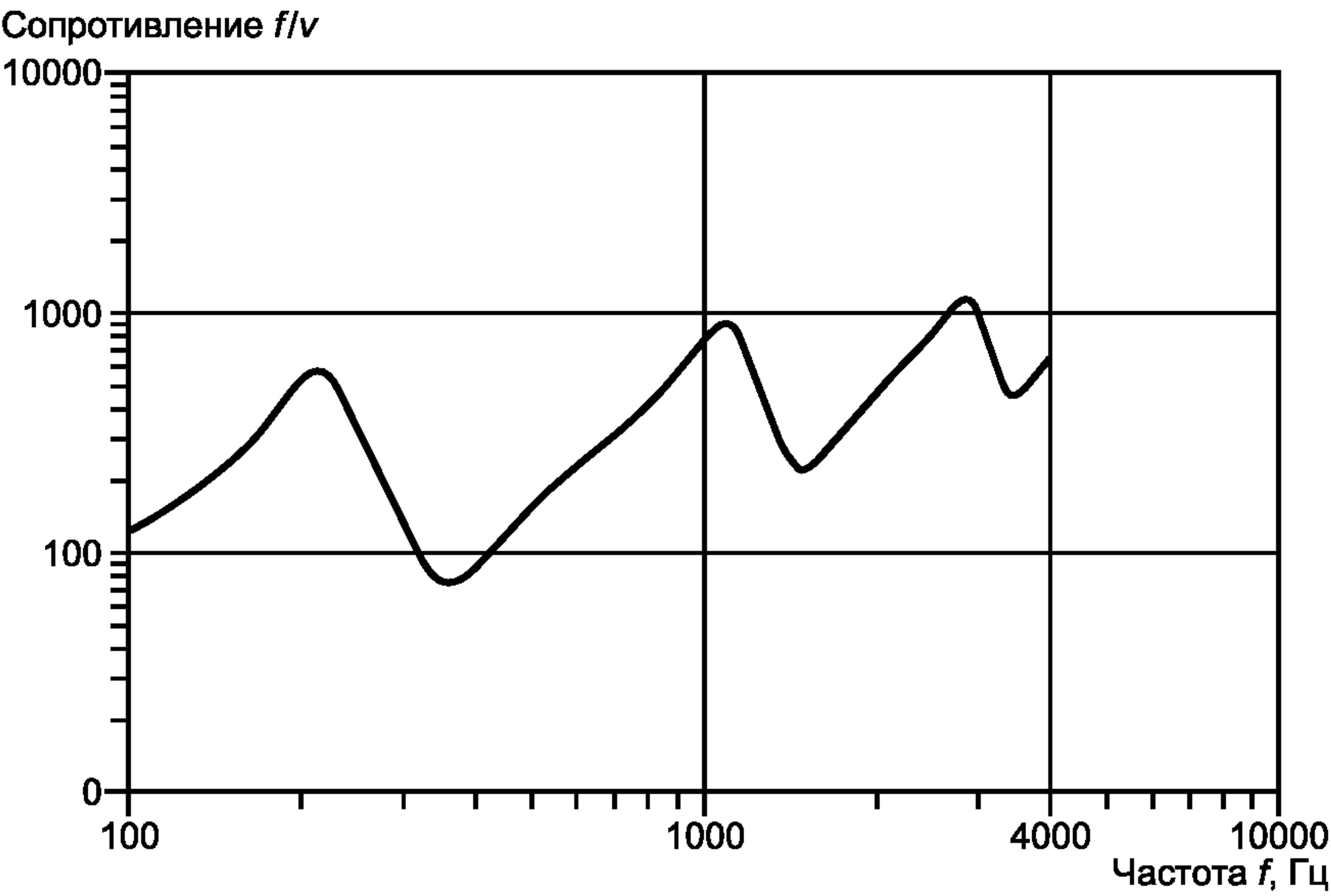
Рисунок D.1 — Типичный пример результата измерения
