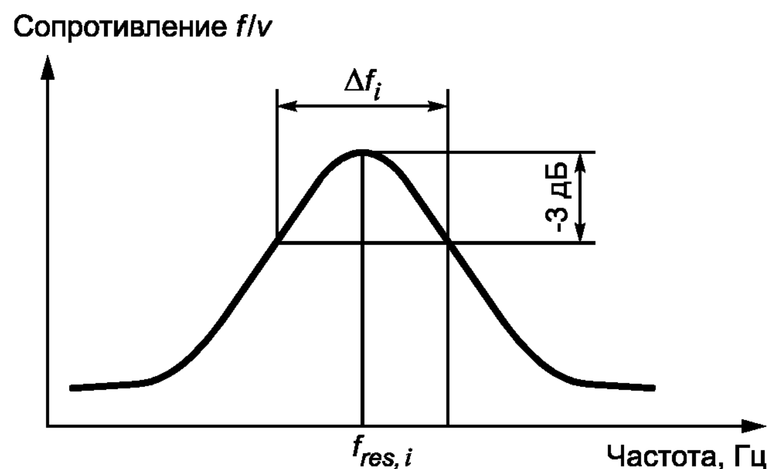
Рисунок 2 — Определение коэффициента затухания звуковых колебаний
