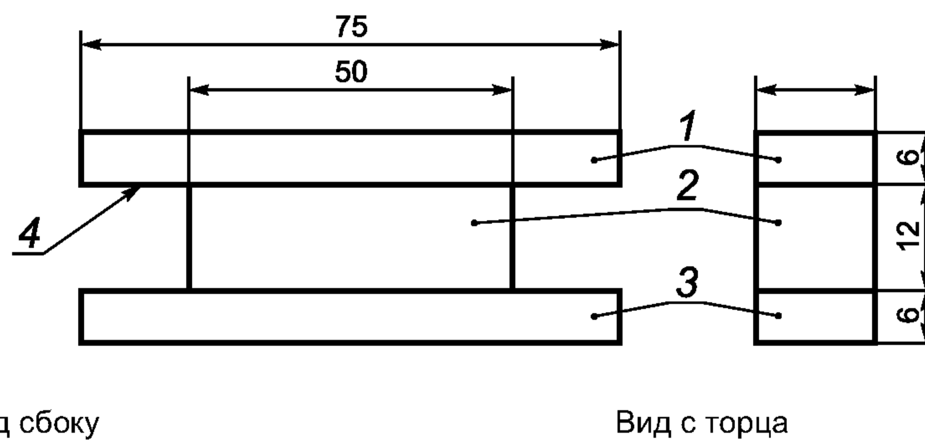
Рисунок А.1 — Испытываемый образец
