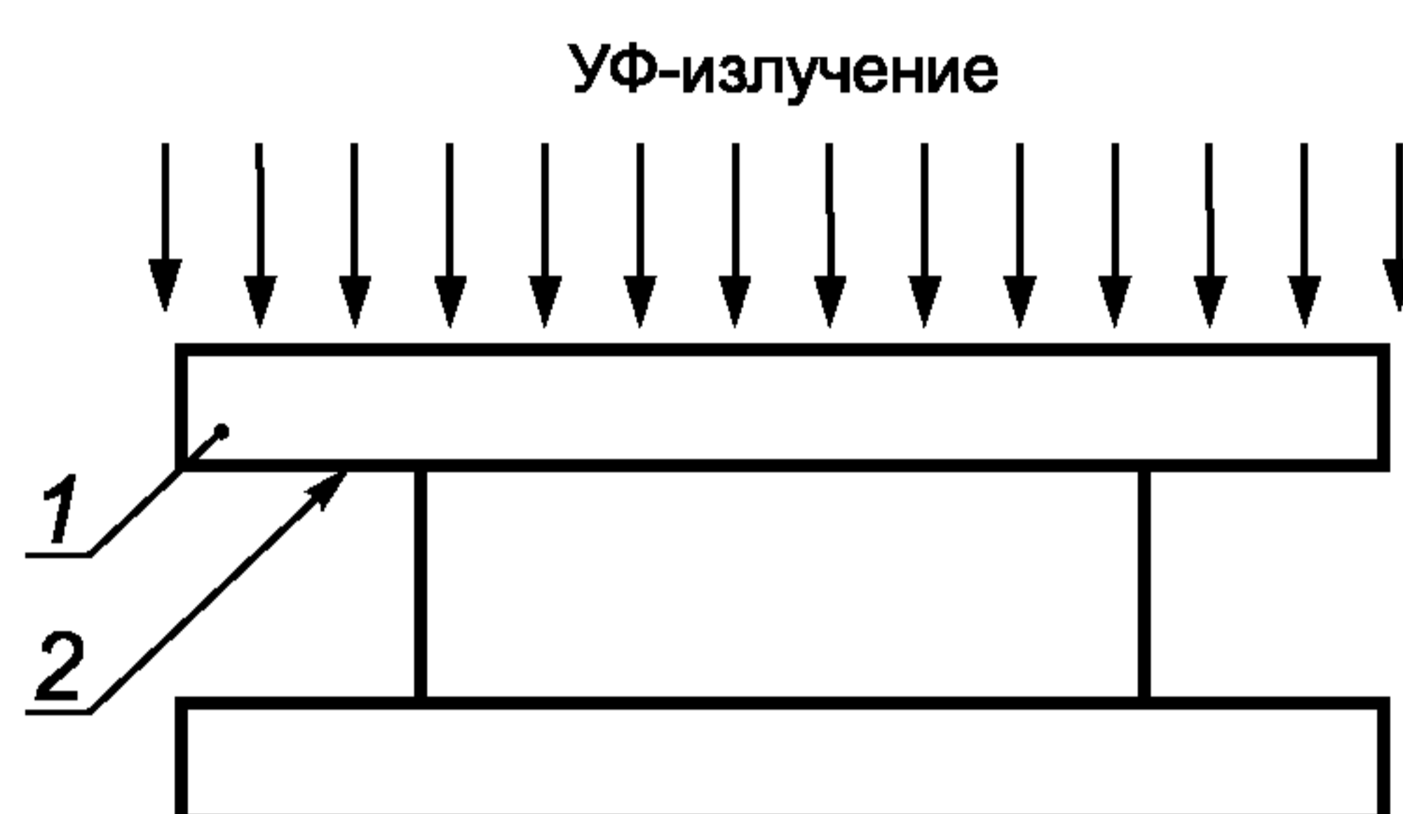
1 — стекло; 2 — испытываемая поверхность (может иметь покрытие)
