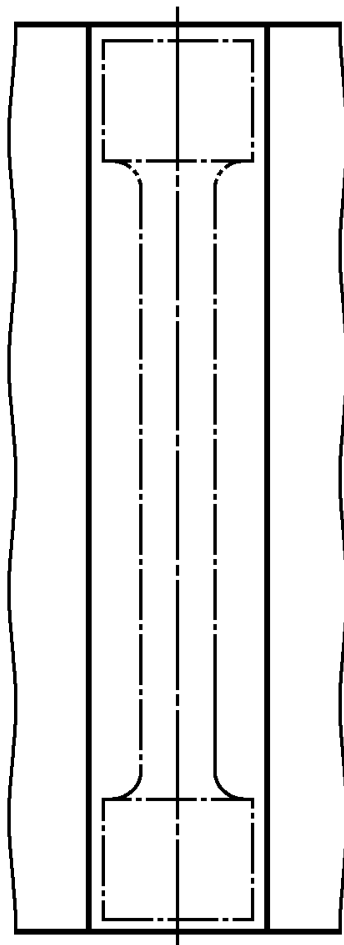
Рисунок 1 — Пример расположения образца для испытаний вдоль шва
