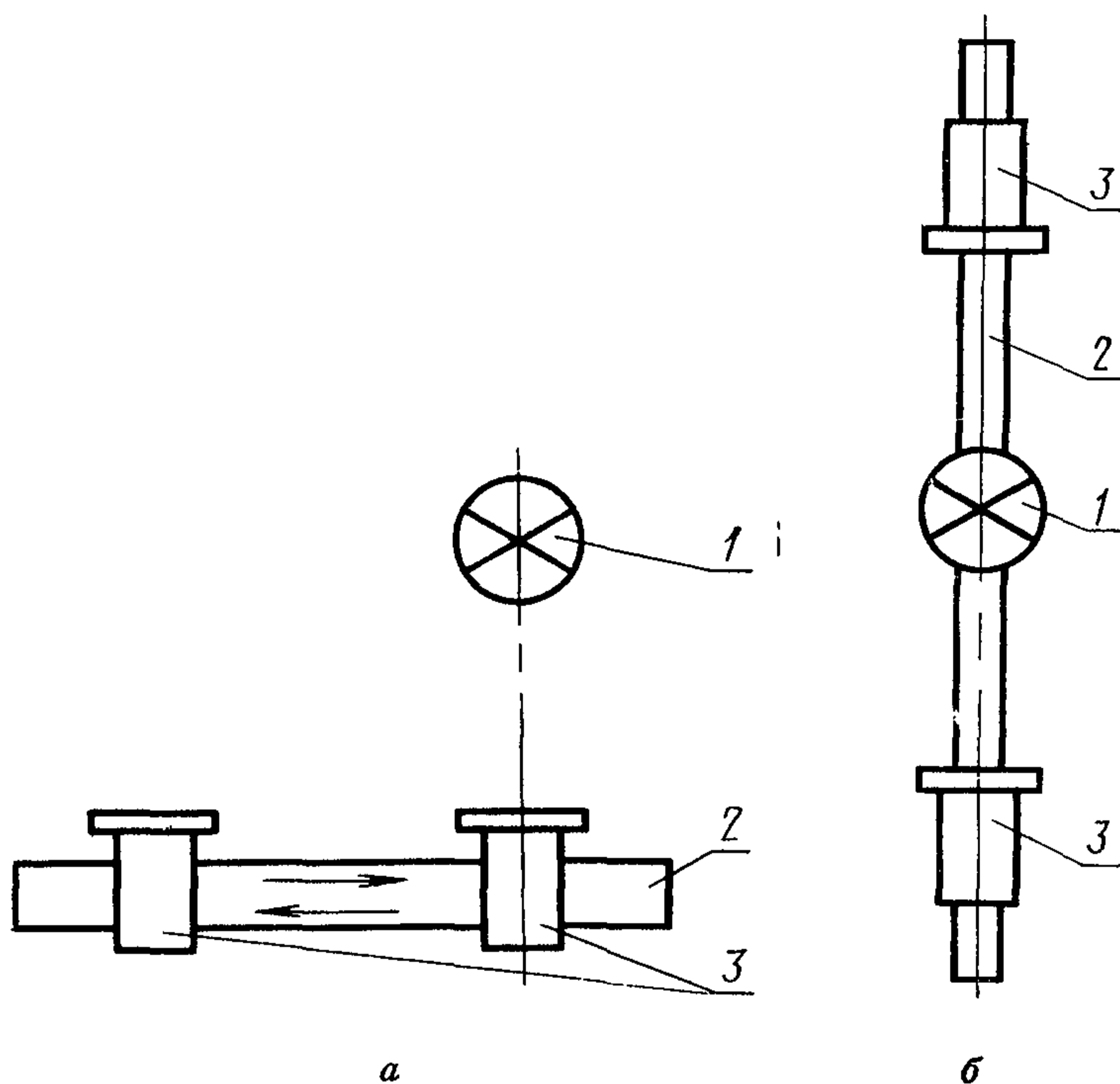
1 — излучатель; 2 — оптическая скамья; 3 — телескоп
