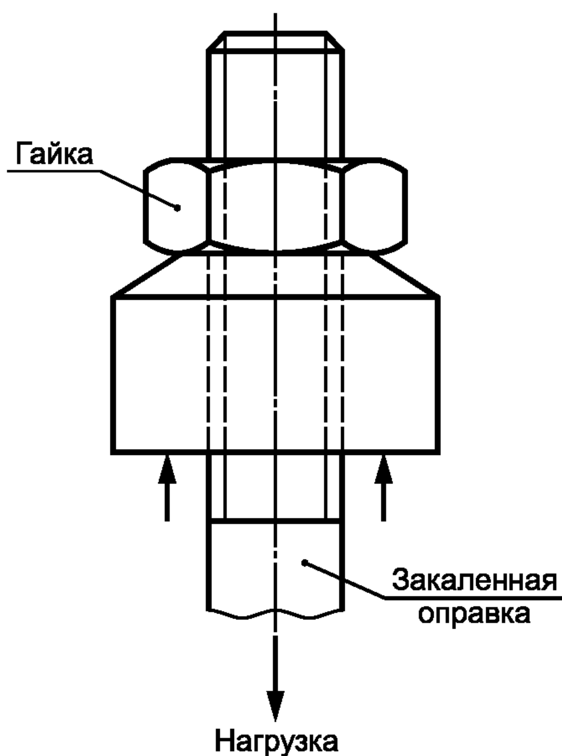
Рисунок 2 — Сборка для испытаний
