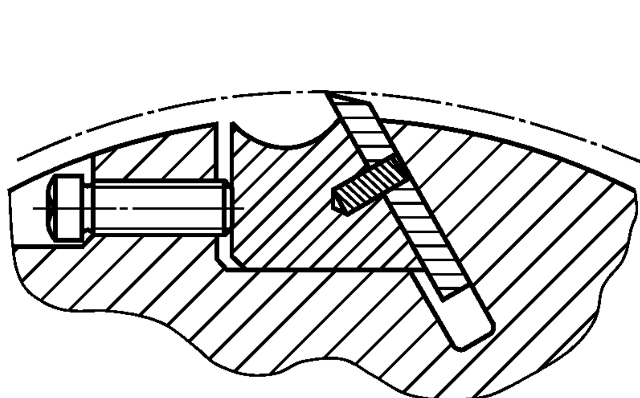
Клиновое крепление с зажимным винтом в корпусе и штифтом в клине
