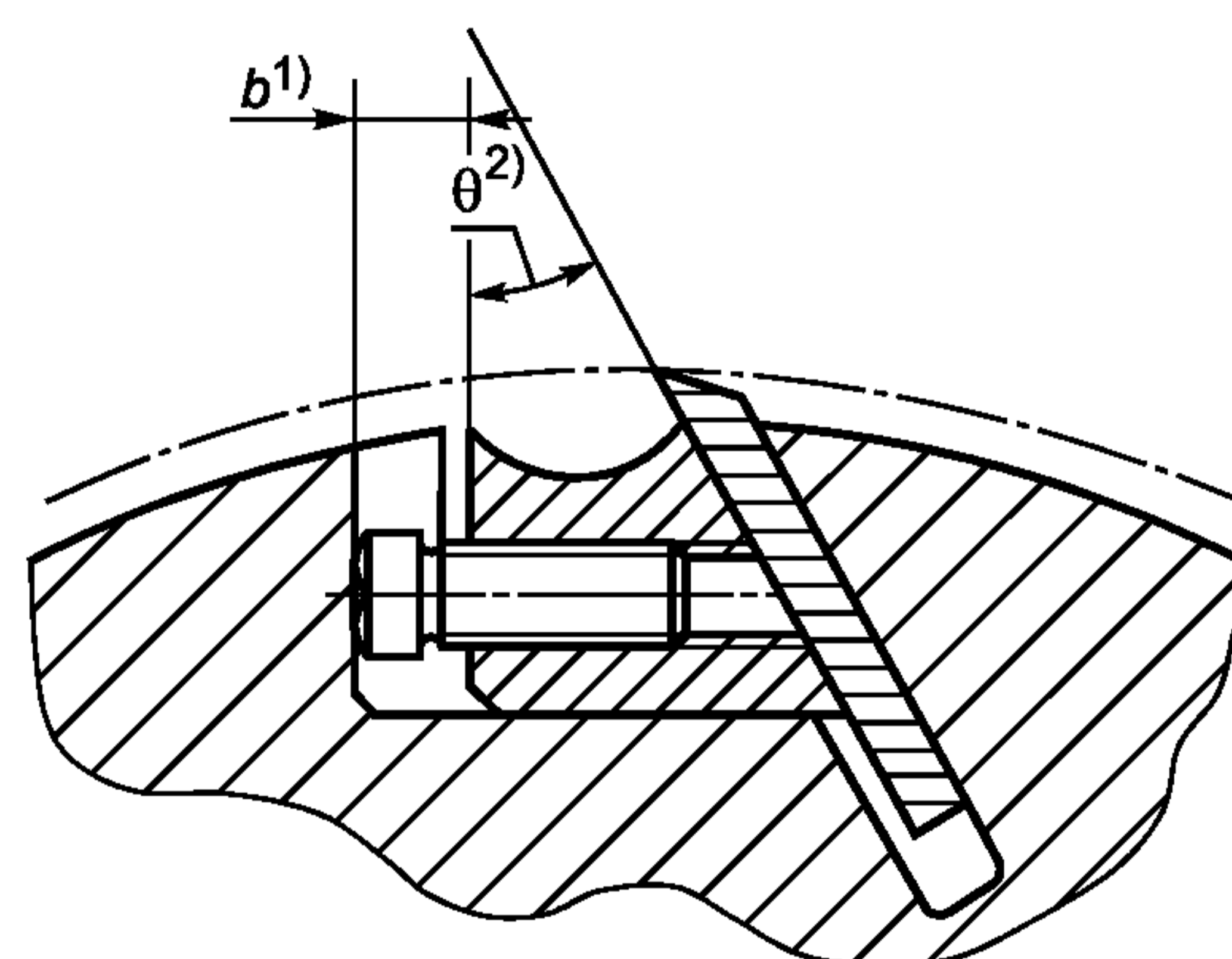
Клиновое крепление с зажимным винтом в клине 3)
