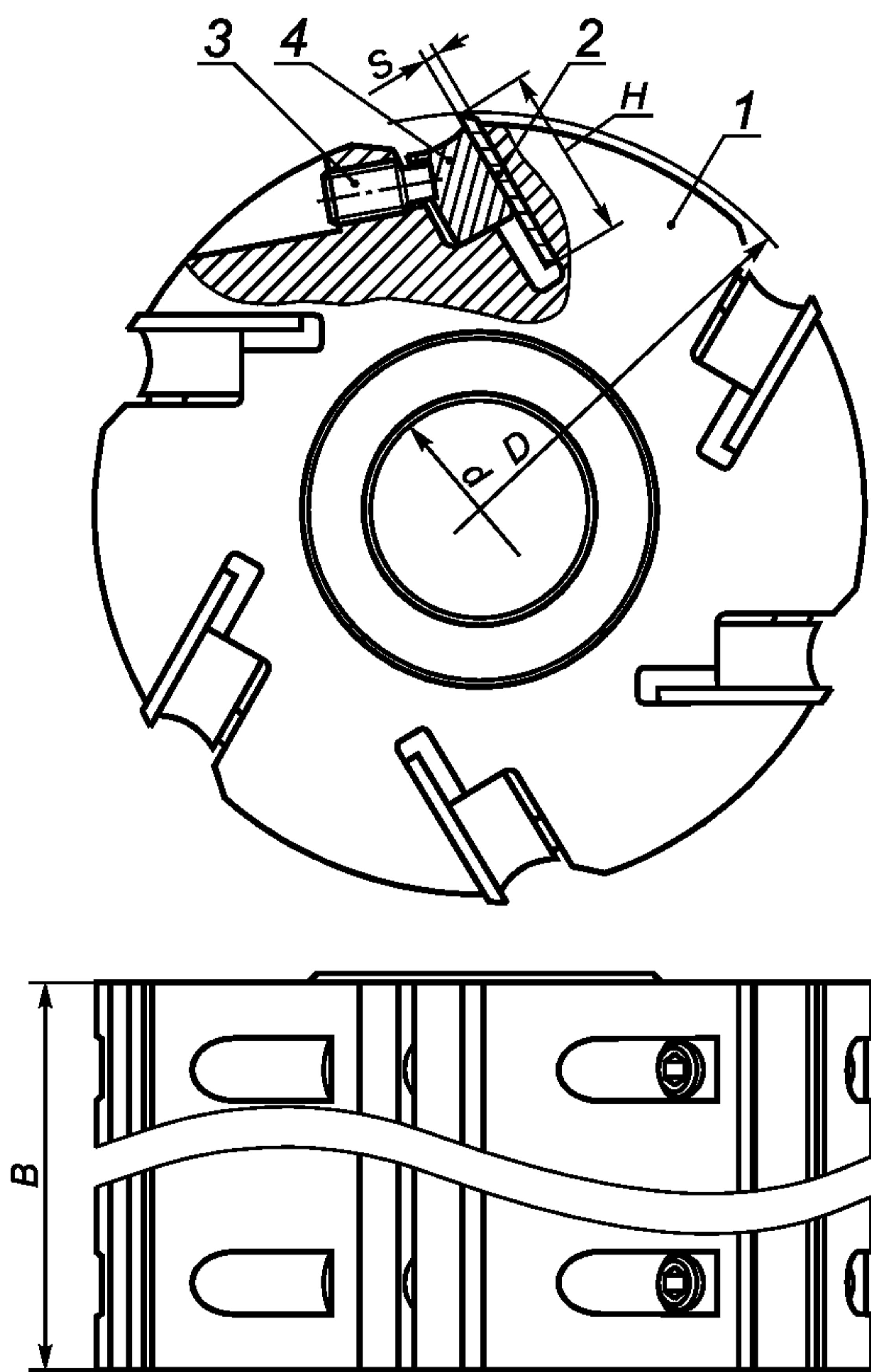
1 — корпус; 2 — нож; 3 — винт; 4 — клин
