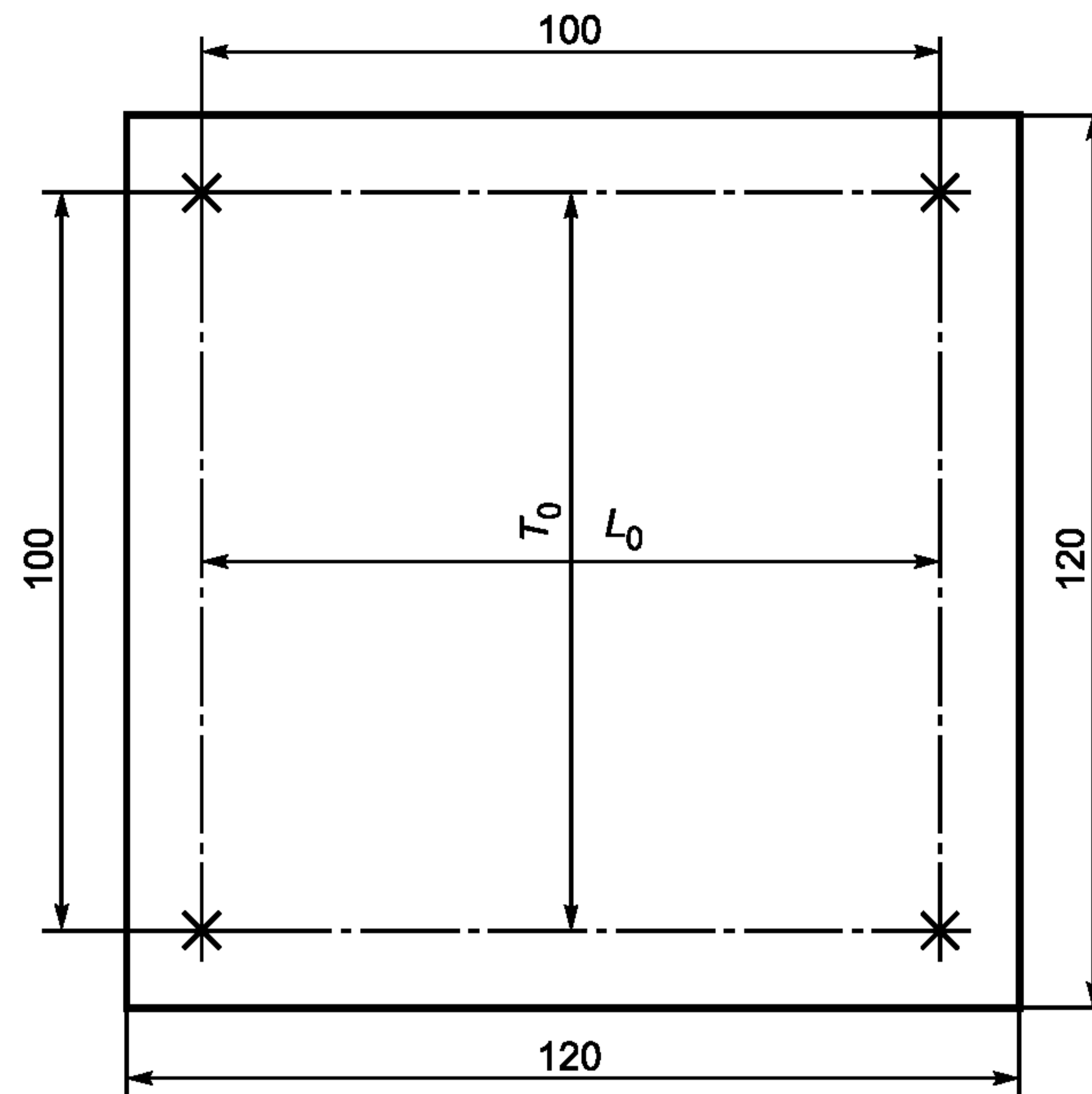
Рисунок 1 — Размеры образца и базовые отрезки
