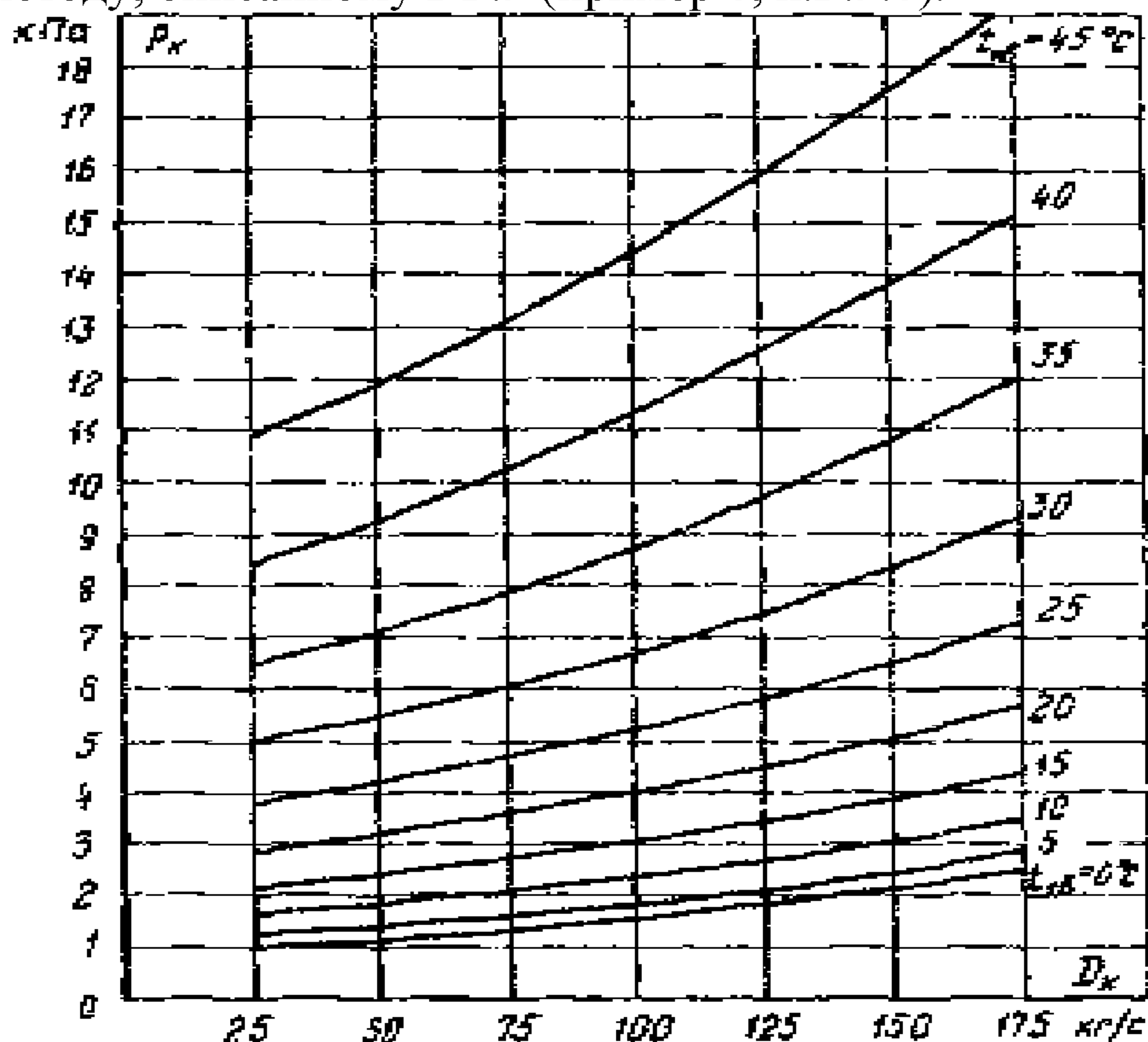
Рисунок Р.5 - Давление в конденсаторе (к примеру 6)
