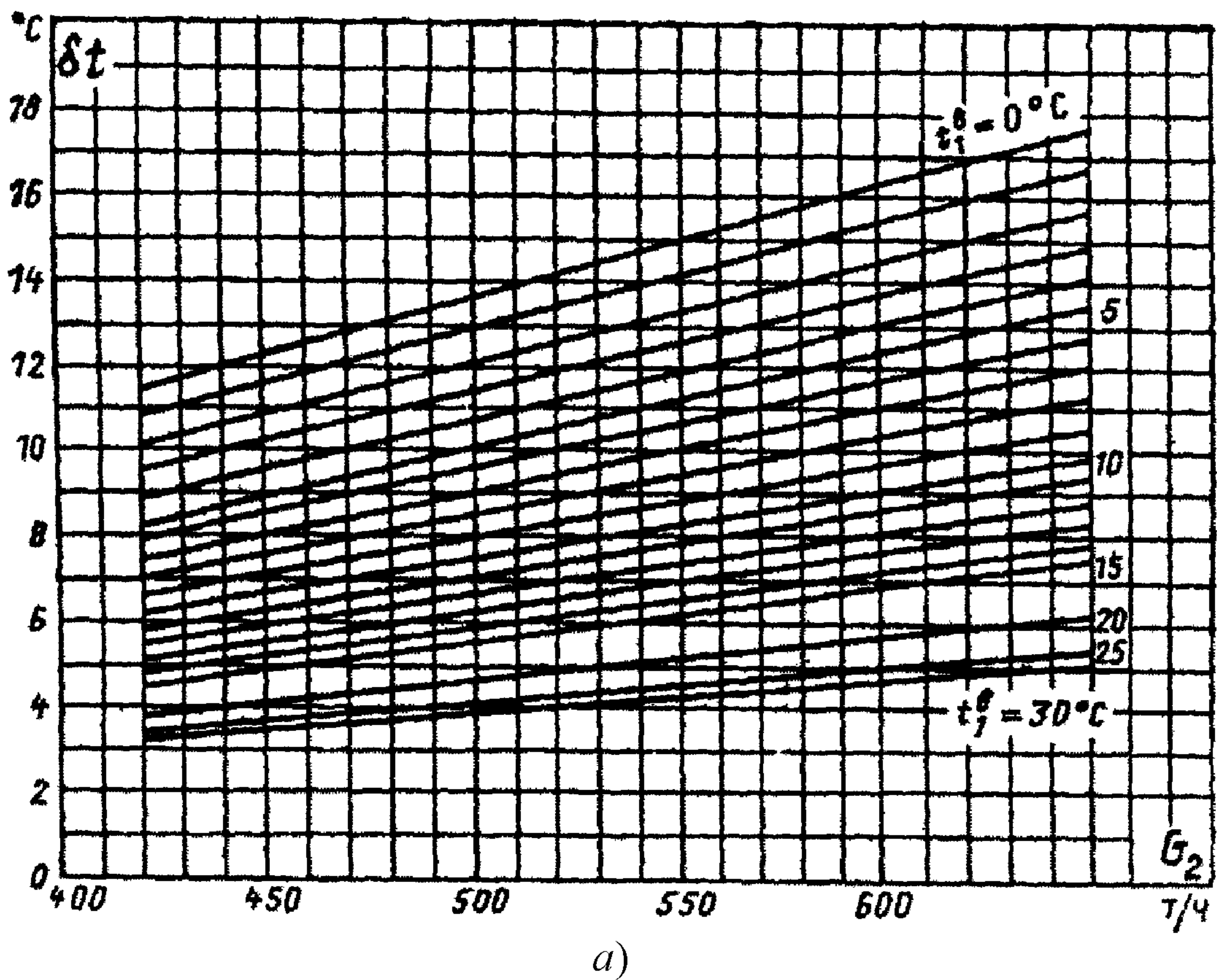
Рисунок Н.3 - Зависимость вакуума в конденсаторе 300-КЦС-1 ( \rho_2 ) от паровой нагрузки ( G_2 ) и температуры охлаждающей воды ( t_1^b )
