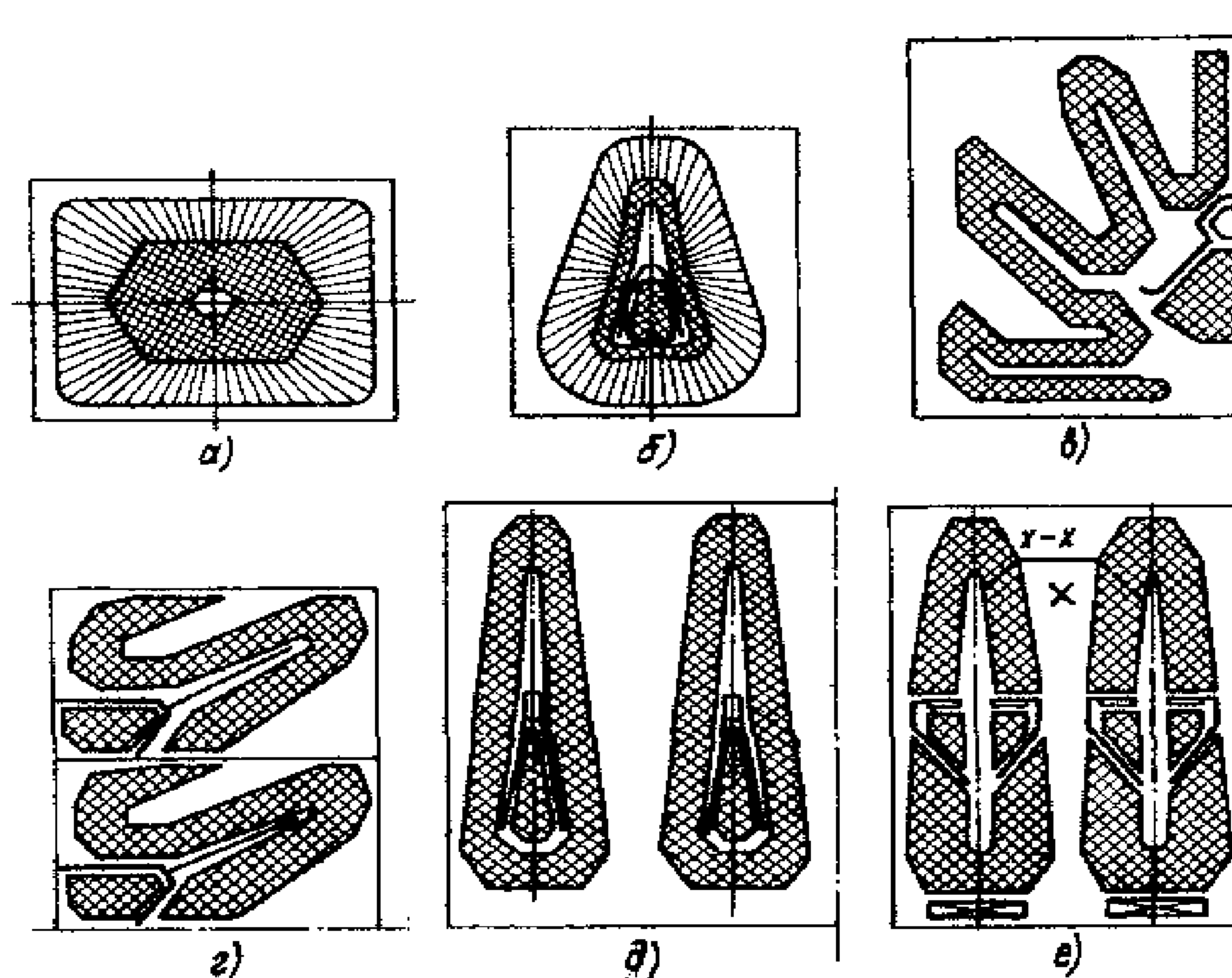
a), б) - радиальная; в), г) - ленточная; д), е) -модульная ленточная; x-x - сечение канала; X для прохода пара
