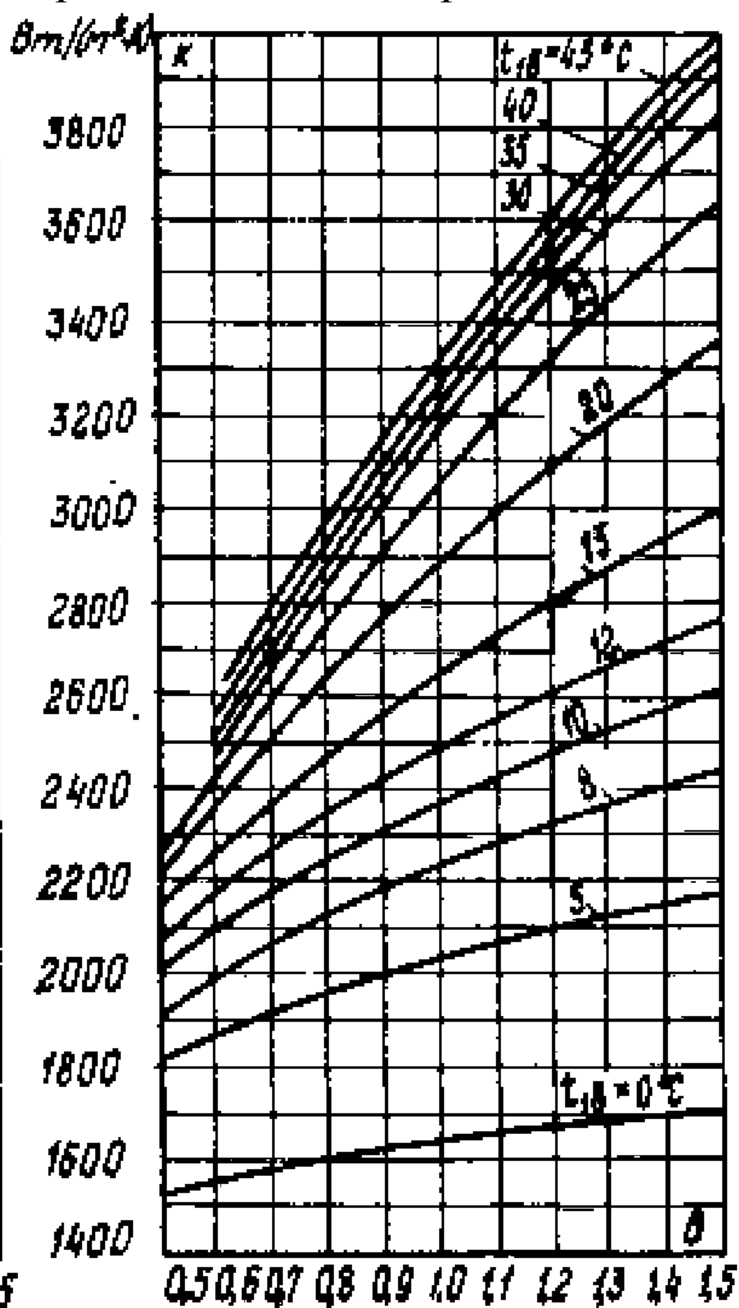
Рис. Р.1.2 - Коэффициент теплопередачи одноходового конденсатора: z = 1; \alpha = 0,8; \delta = 0,42
