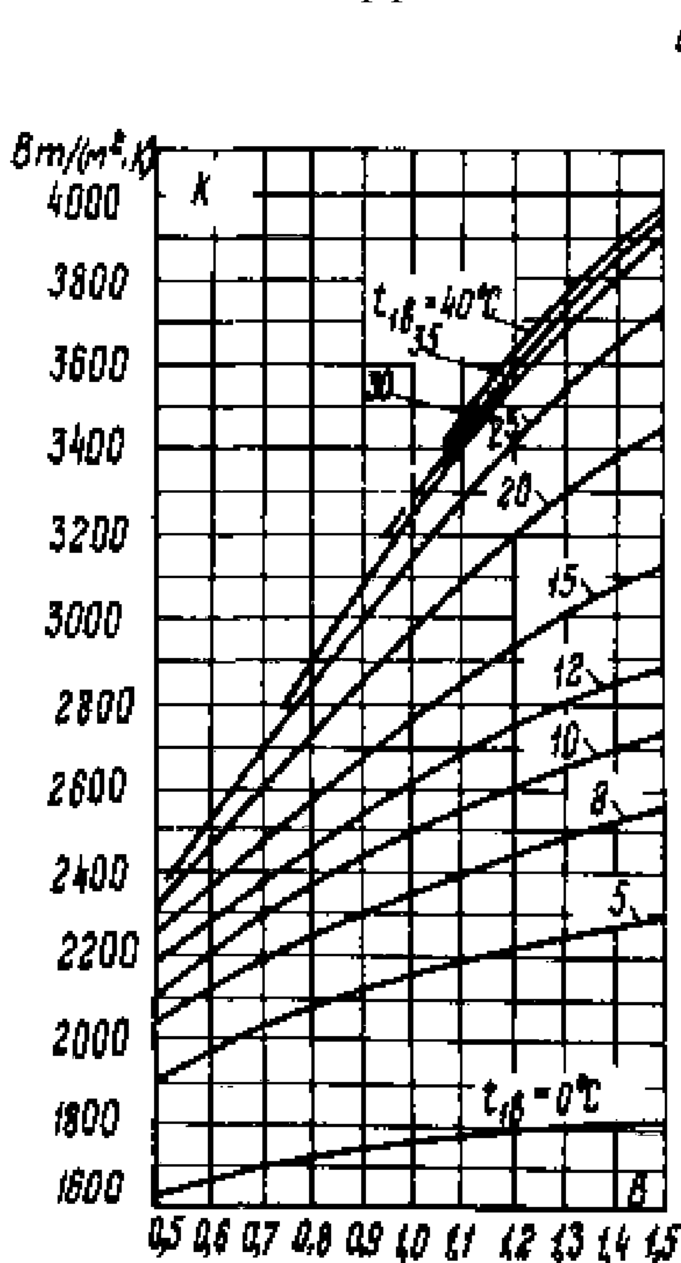
Рис. Р.1.1 - Коэффициент теплопередачи двухходового конденсатора: z = 2; \alpha = 0,8; \delta = 0,42
