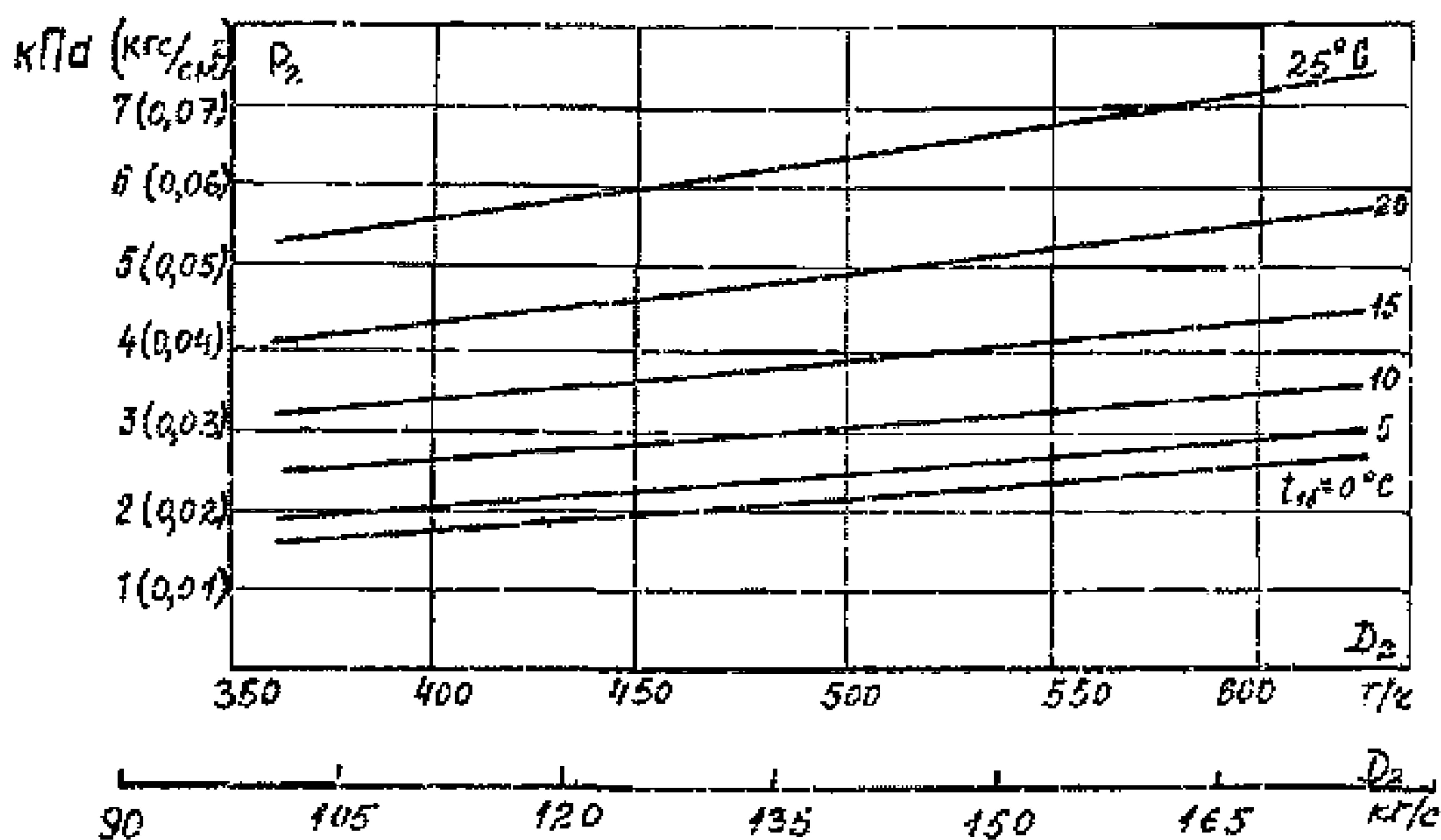
Рисунок П.2 - Давление в конденсаторе Н-15240 ПОАТ ХТЗ в зависимости от расхода пара D_2 и температуры охлаждающей воды t_{1в} (при номинальном расходе охлаждающей воды W = 34800 \text{ м}^3/\text{ч} )
