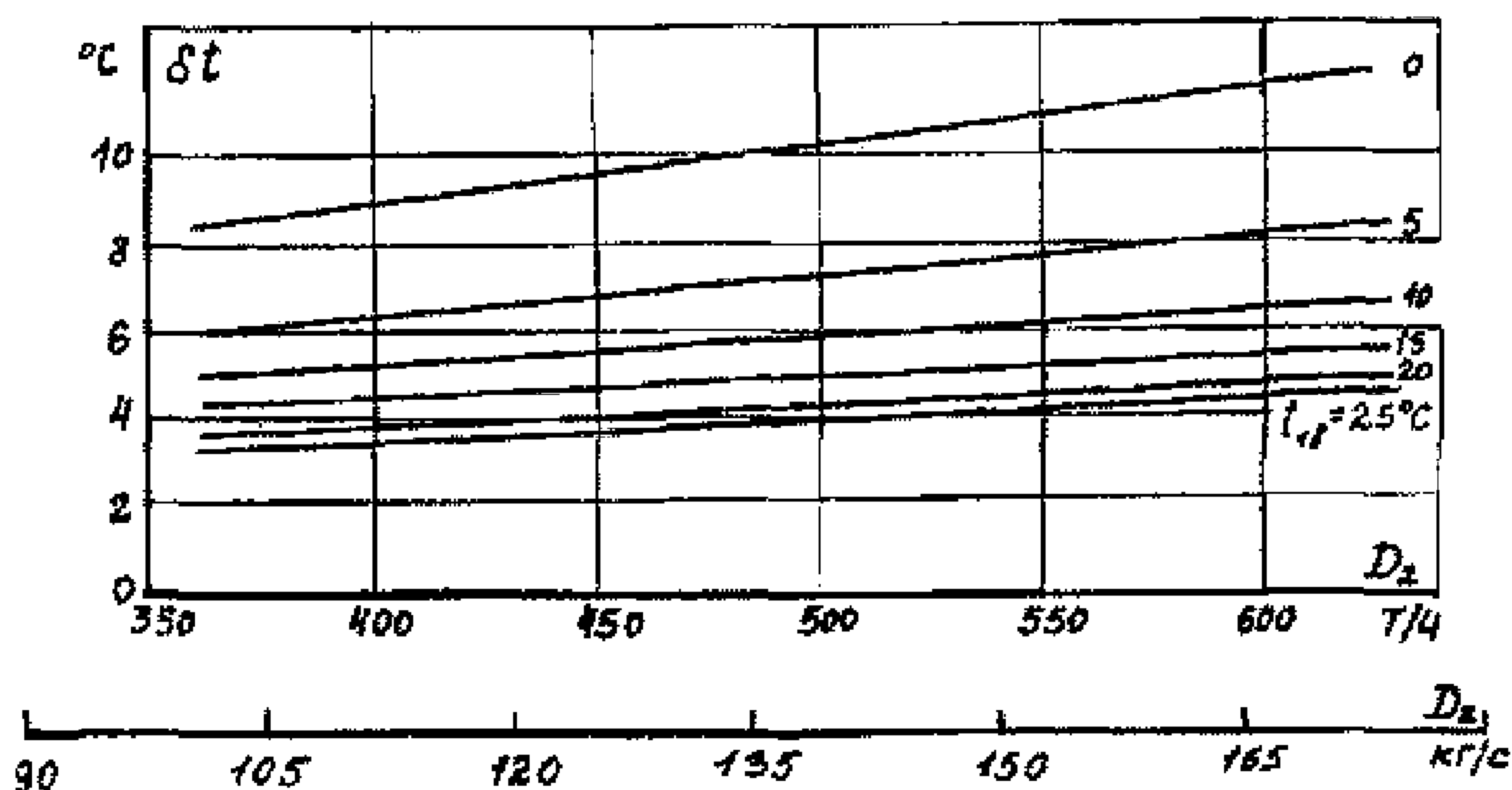
Рисунок П.1 - Температурный напор конденсатора К-15240 ПОАТ ХТЗ в зависимости от расхода пара D_2 и температуры охлаждающей воды t_{1в} (при номинальном расходе охлаждающей воды W = 34800 \text{ м}^3/\text{ч} )
