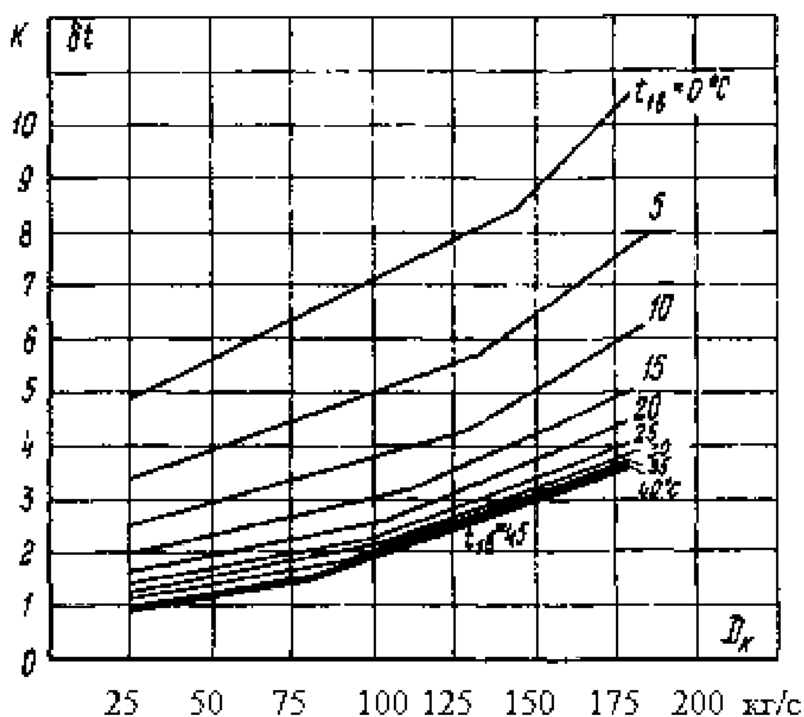
Рисунок Р.4 - Температурный напор в конденсаторе (к примеру б) Найденный таким образом значения P_K для разных значений t_{1в} и D_K и G_0 =
