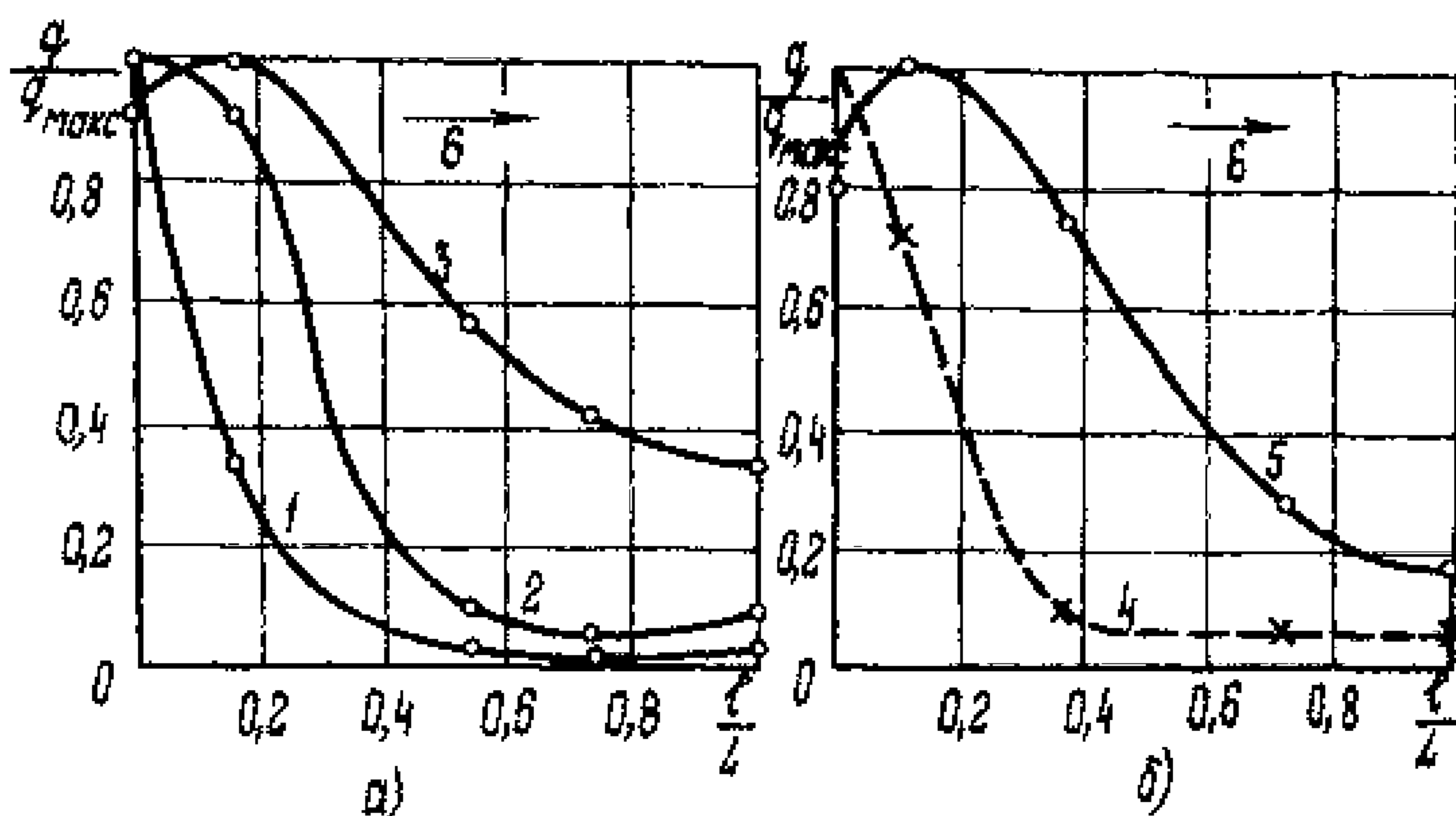
а) - в зависимости от удельной паровой нагрузки d_k и температуры охлаждающей воды t_{16} ; 1 - d_k = 4,17 \text{ г/м}^2\text{с} и t_{16} = 11^\circ\text{C} ; 2 - d_k = 7,2 \text{ г/м}^2\text{с} и t_{16} = 11^\circ\text{C} ; 3 - d_k \geq 9,7 \text{ г/м}^2\text{с} и t_{16} = 24^\circ\text{C} ; б) - в зависимости от количества проникающего в конденсатор воздуха G_e ( d_k = 10 \text{ г/м}^2\text{с} и t_{16} = 17,3^\circ\text{C} ); 4 - G_e = 12 \text{ г/с} ; 5 - G_e = 4,42 \text{ г/с} ; 6 - движение пара; l, L - текущая и полная длина пути пара в трубном пучке; q - удельная тепловая нагрузка
