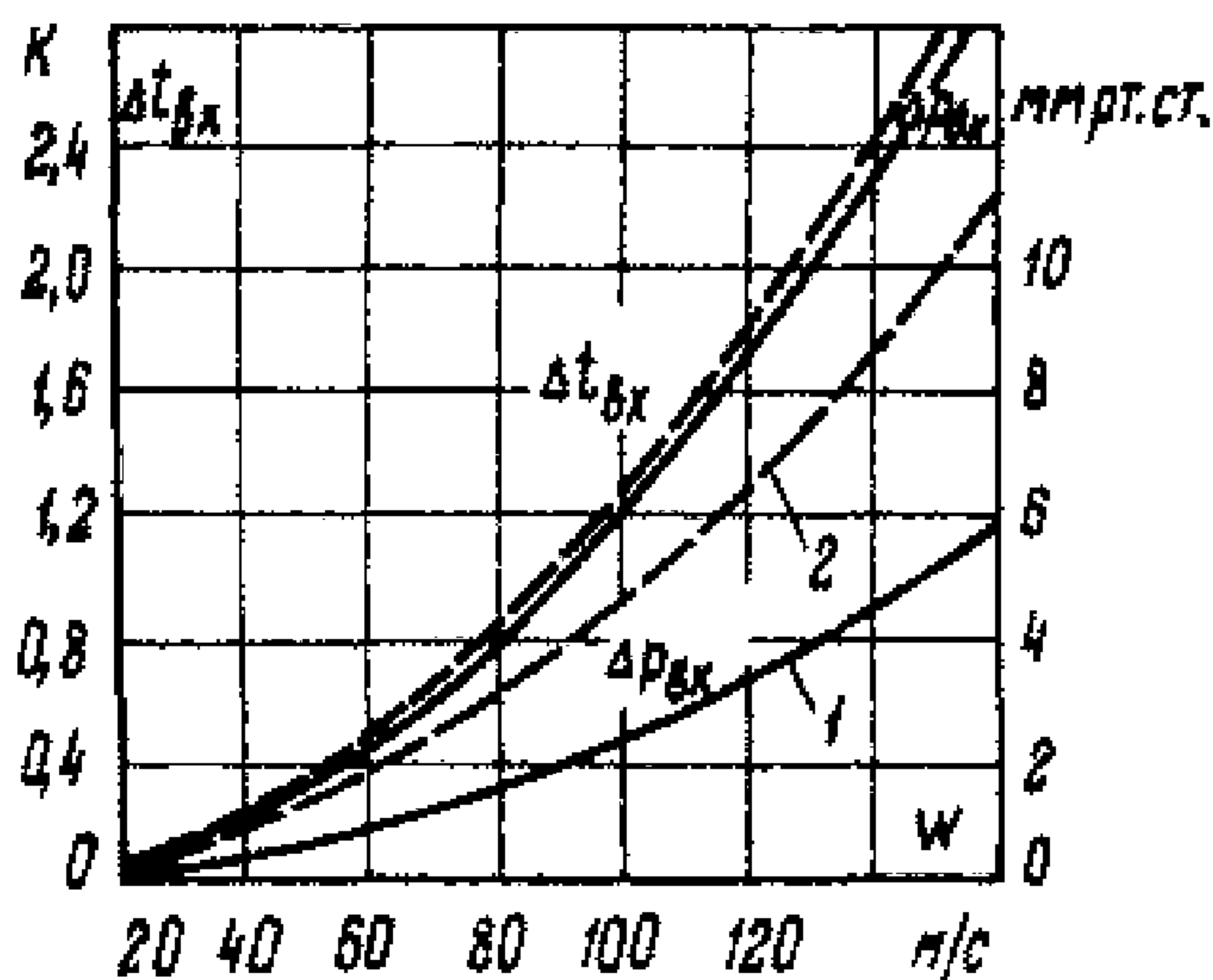
Рисунок Р.13 - Зависимость падения давления \Delta P_{вх} и снижения температуры \Delta t_{вх} пара при входе в трубный пучок от скорости W в узком сечении первого ряда трубок
