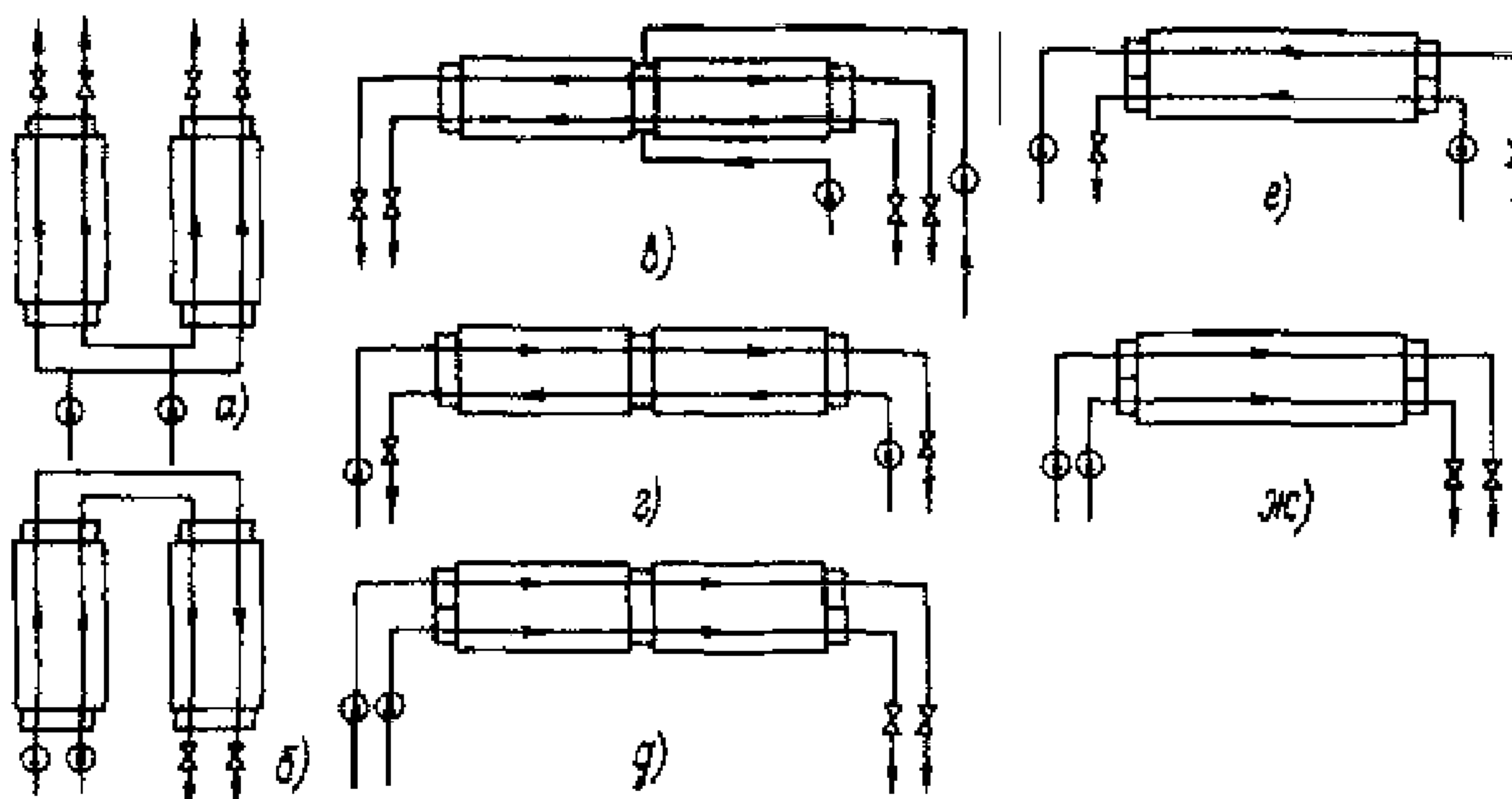
Рисунок Р.8. - Расположение конденсатора относительно оси турбины:
