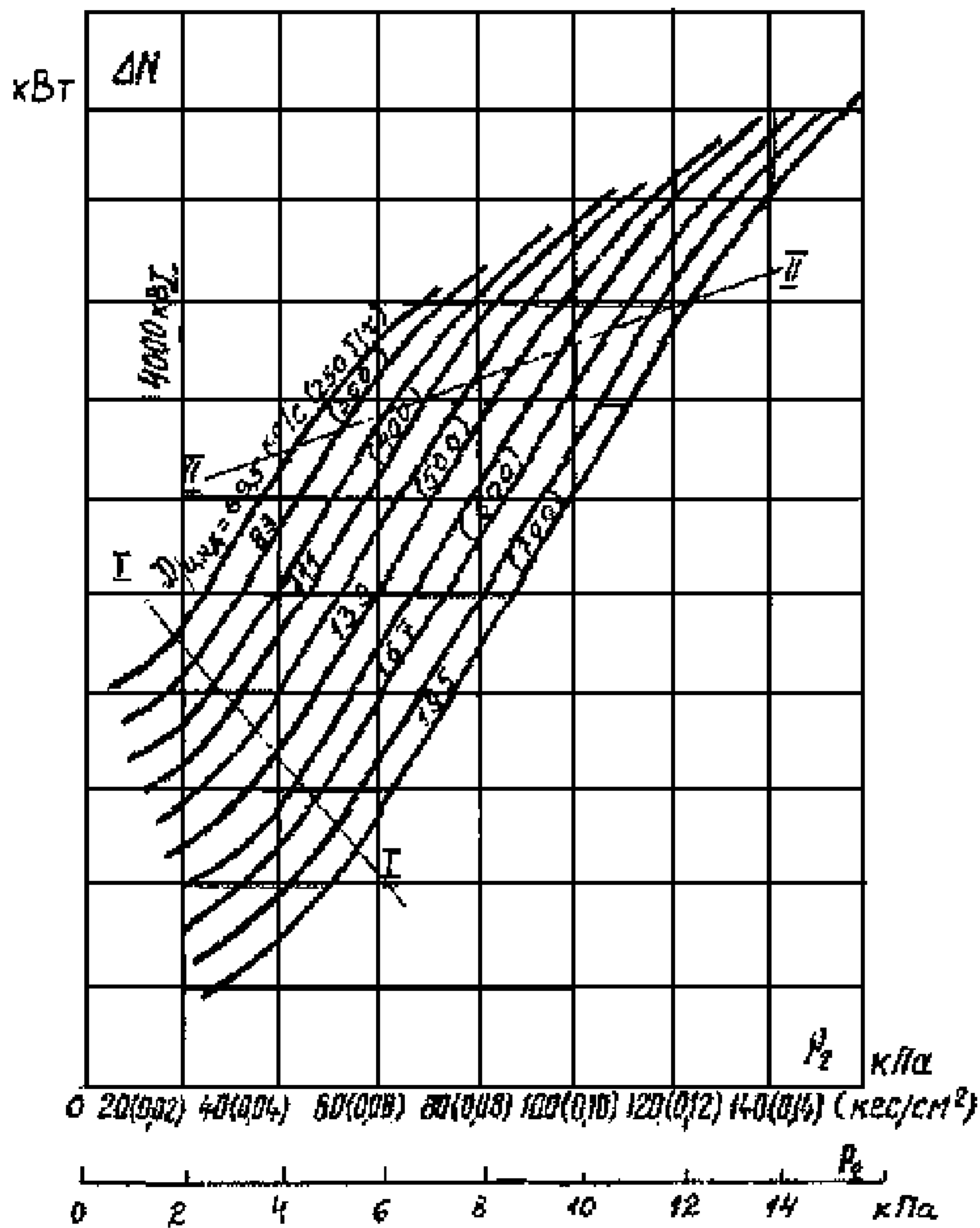
Рисунок П.3 - Поправки к мощности зтурбины К-300-240 ПОАТ ХТЗ на изменение давления в конденсаторе
