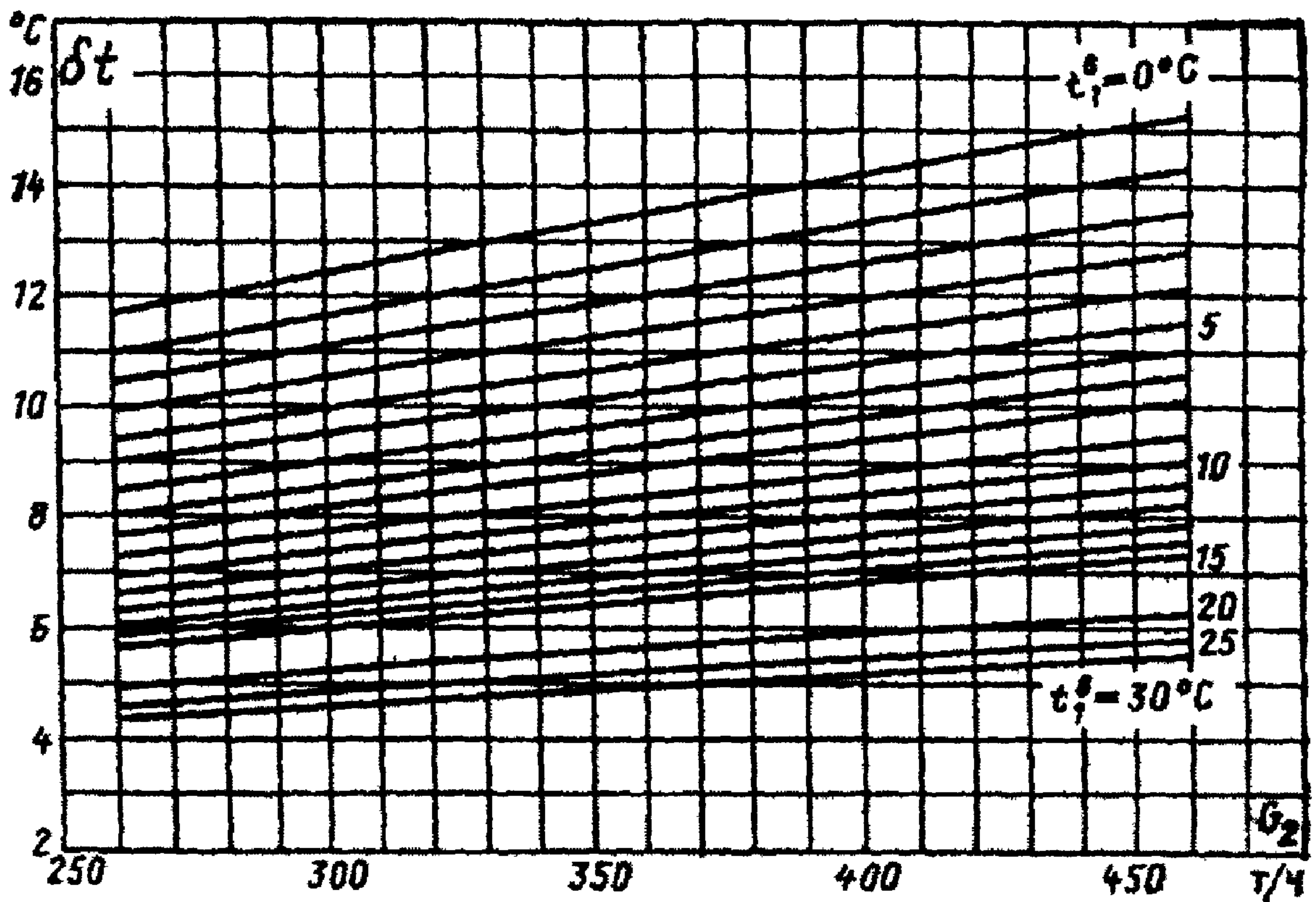
Рисунок Н.4 - Зависимость температурного напора в конденсаторе 300-КЦС-1 ( \delta t ) от паровой нагрузки ( G_2 ) и температуры охлаждающей воды ( t_1^B )
