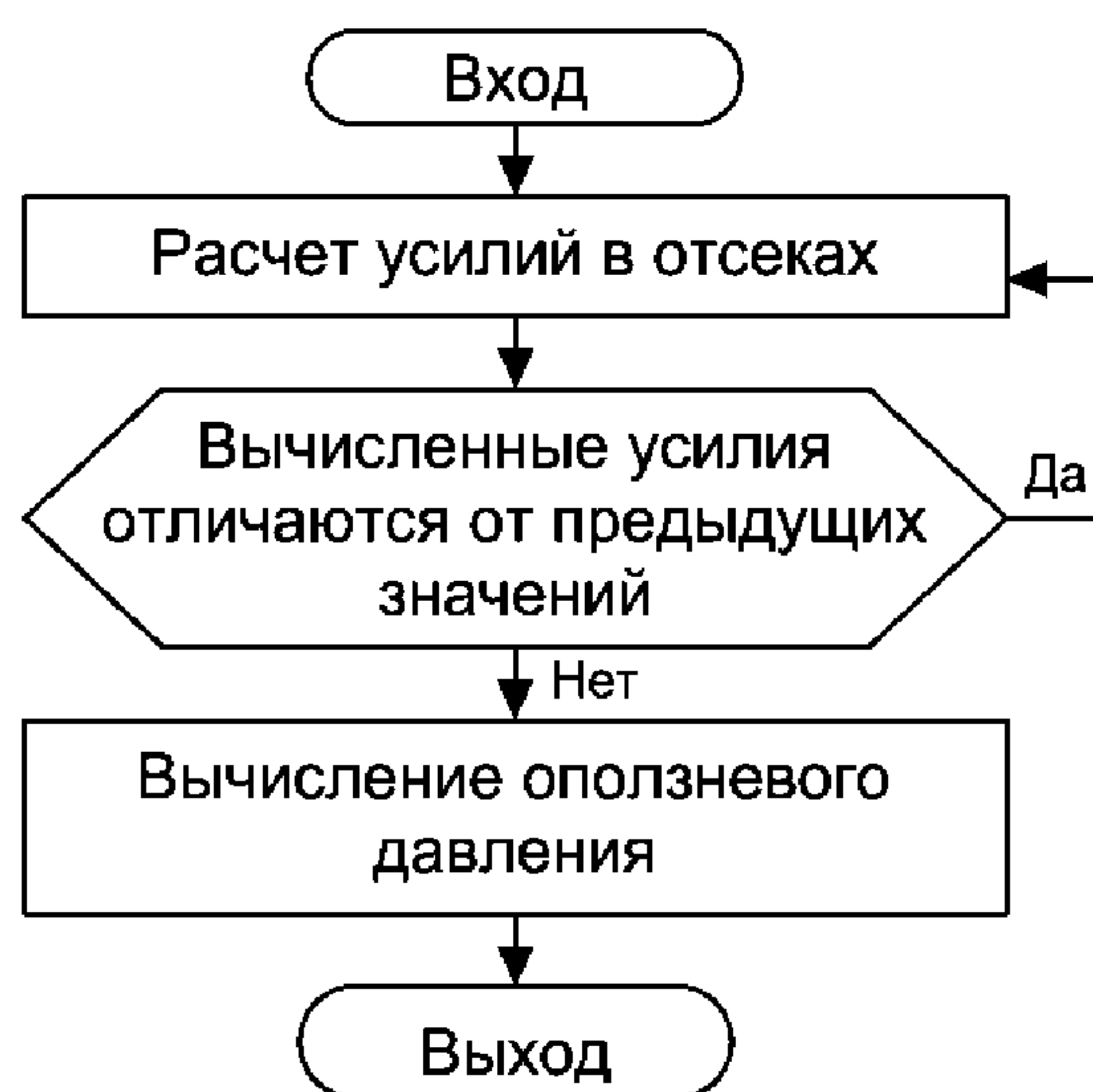
Рисунок 9 – Блок-схема расчета составляющих оползневого давления из условия равновесия сил (моментов)
