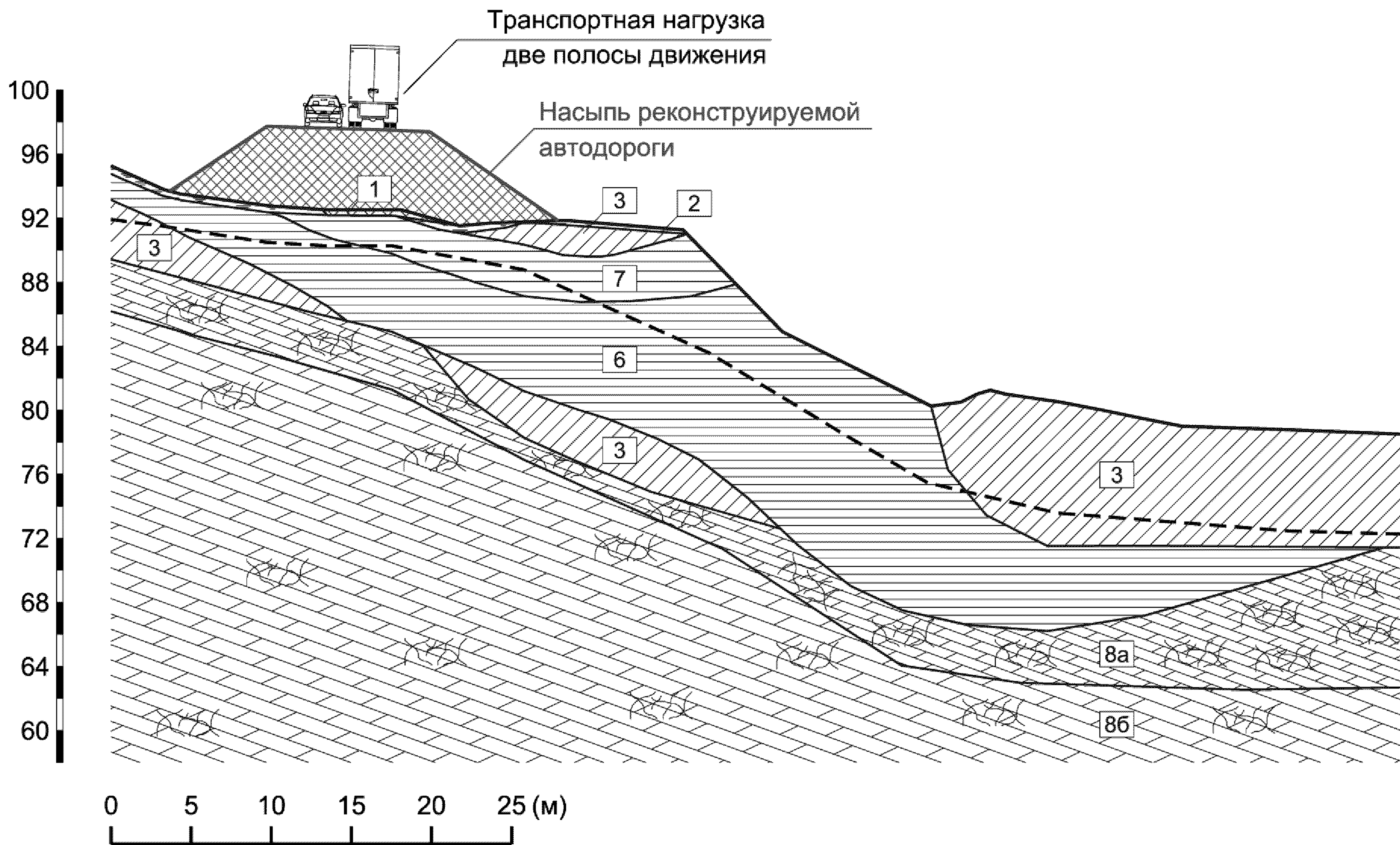
Рисунок А.5 – Инженерно-геологический разрез линии 2-2
