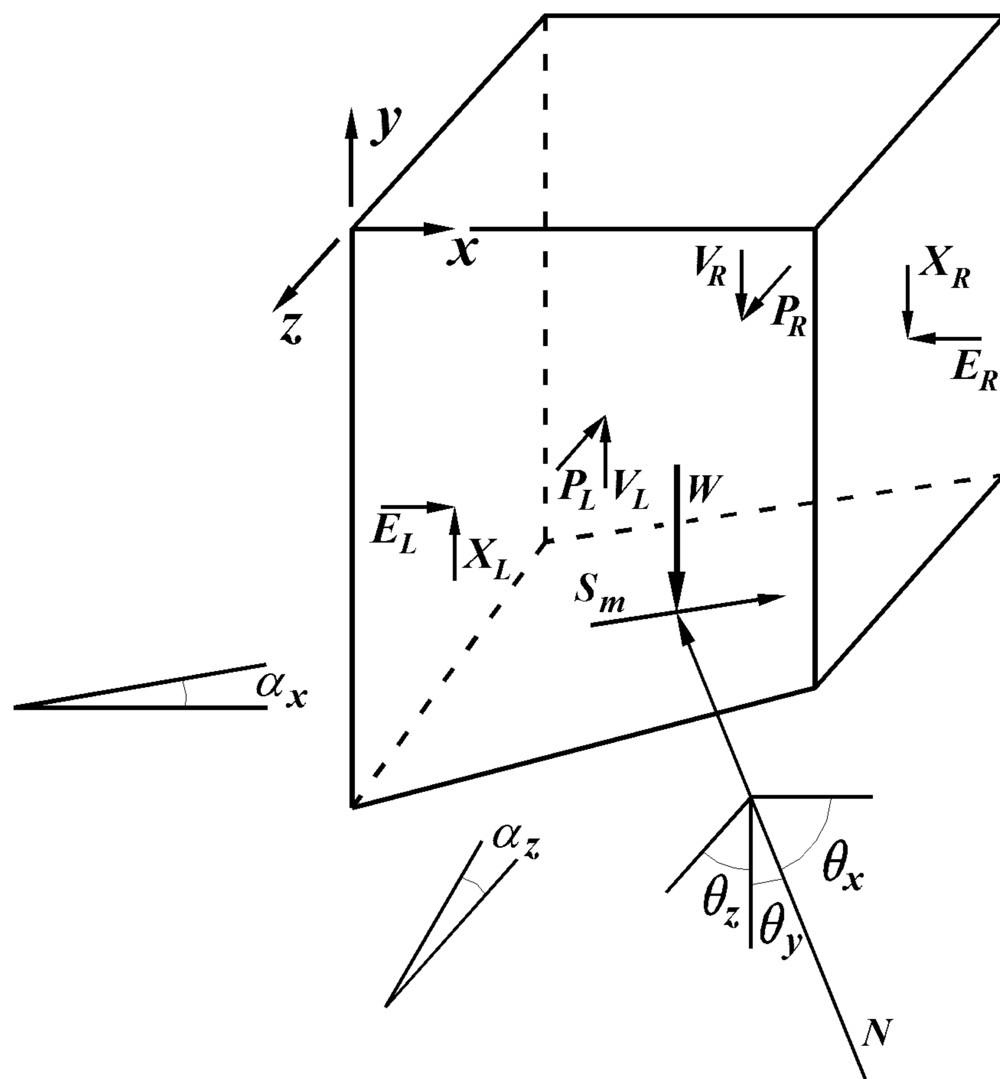
Рисунок 5 – Расчетная схема колонки грунта с приложенными усилиями
