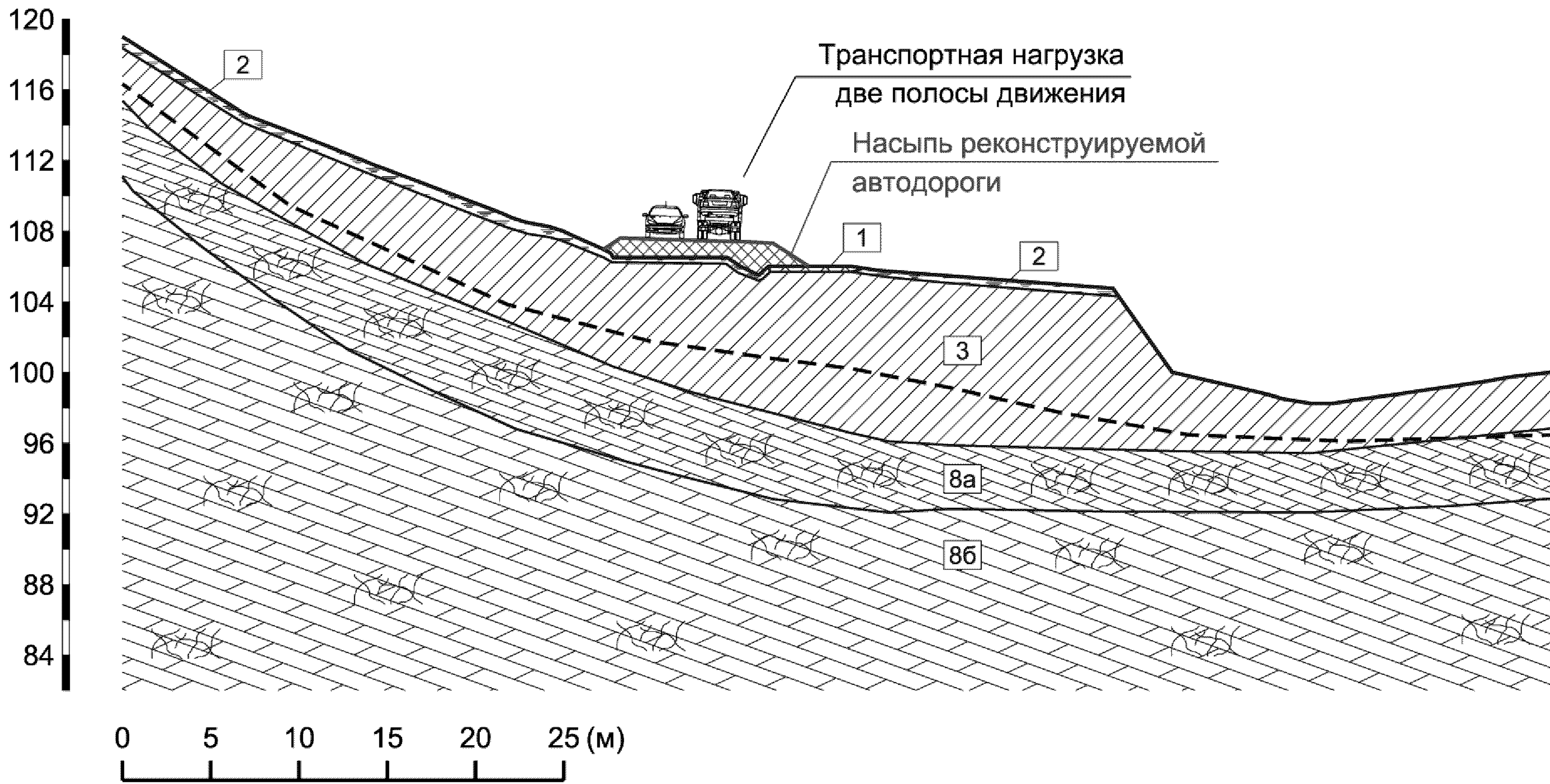
Рисунок А.8 – Инженерно-геологический разрез линии 5-5
