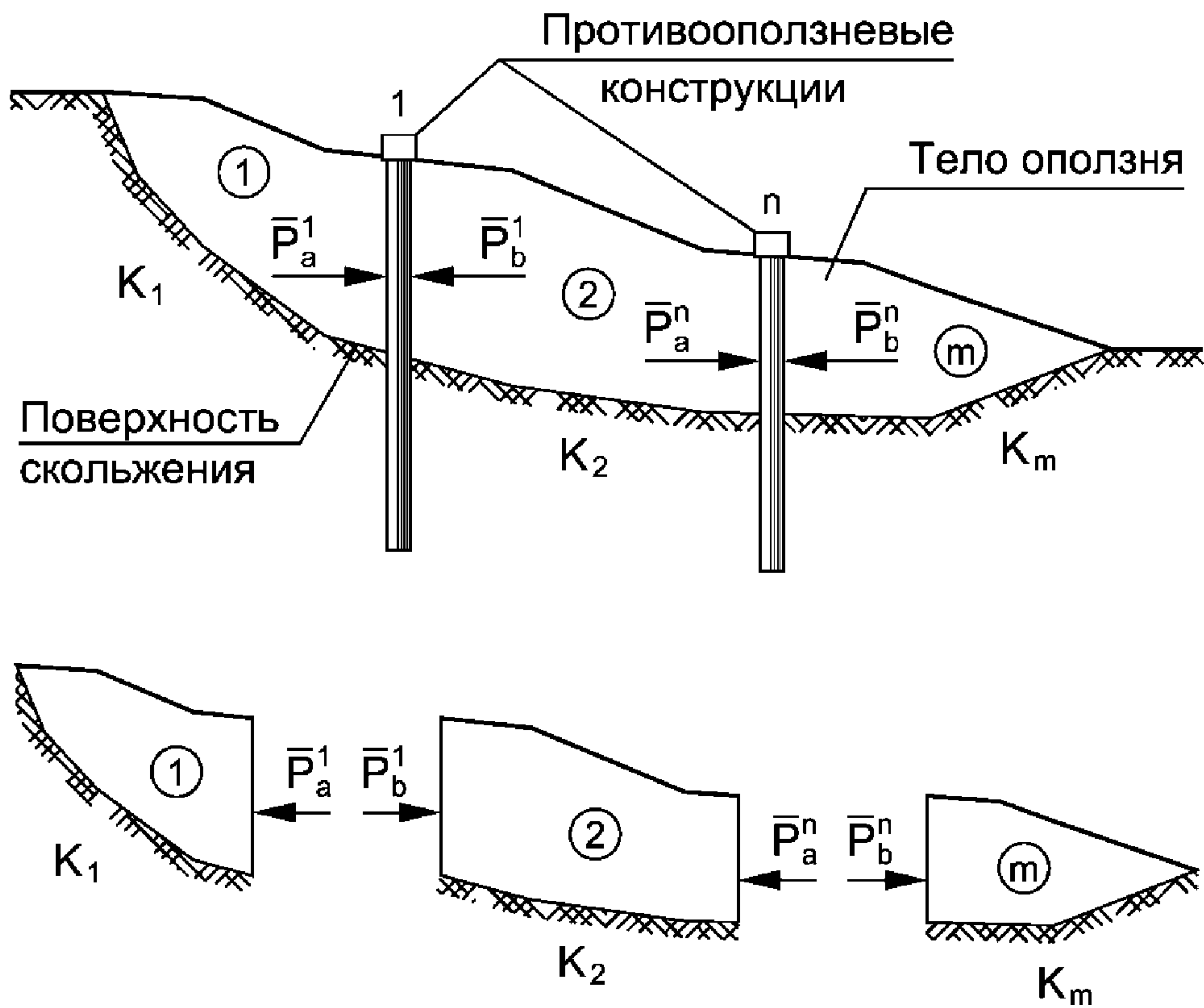
Рисунок 10 – Принципиальная схема расчета оползневых давлений на ярусы свайных сооружений с учетом отпора грунта
