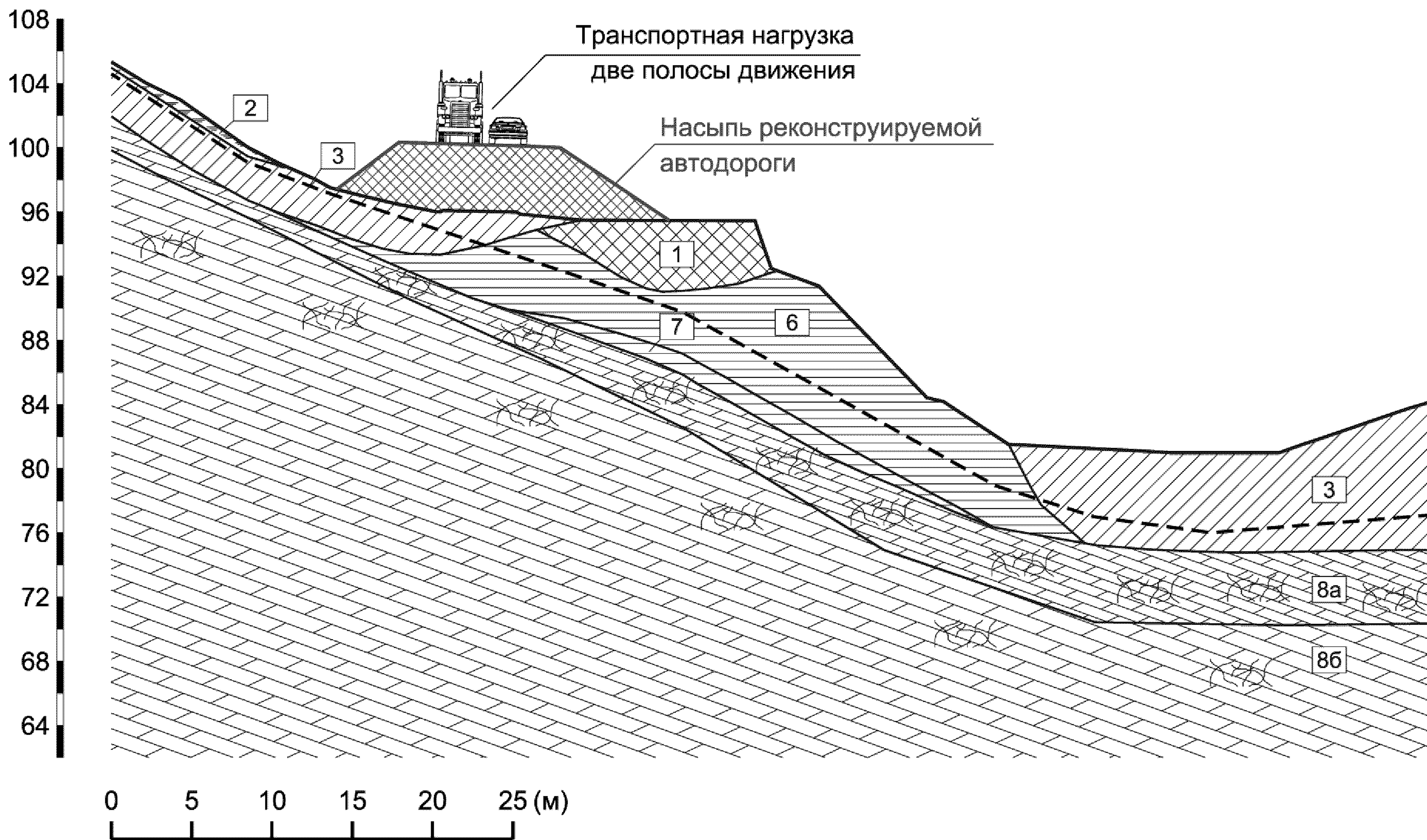
Рисунок А.6 – Инженерно-геологический разрез линии 3-3
