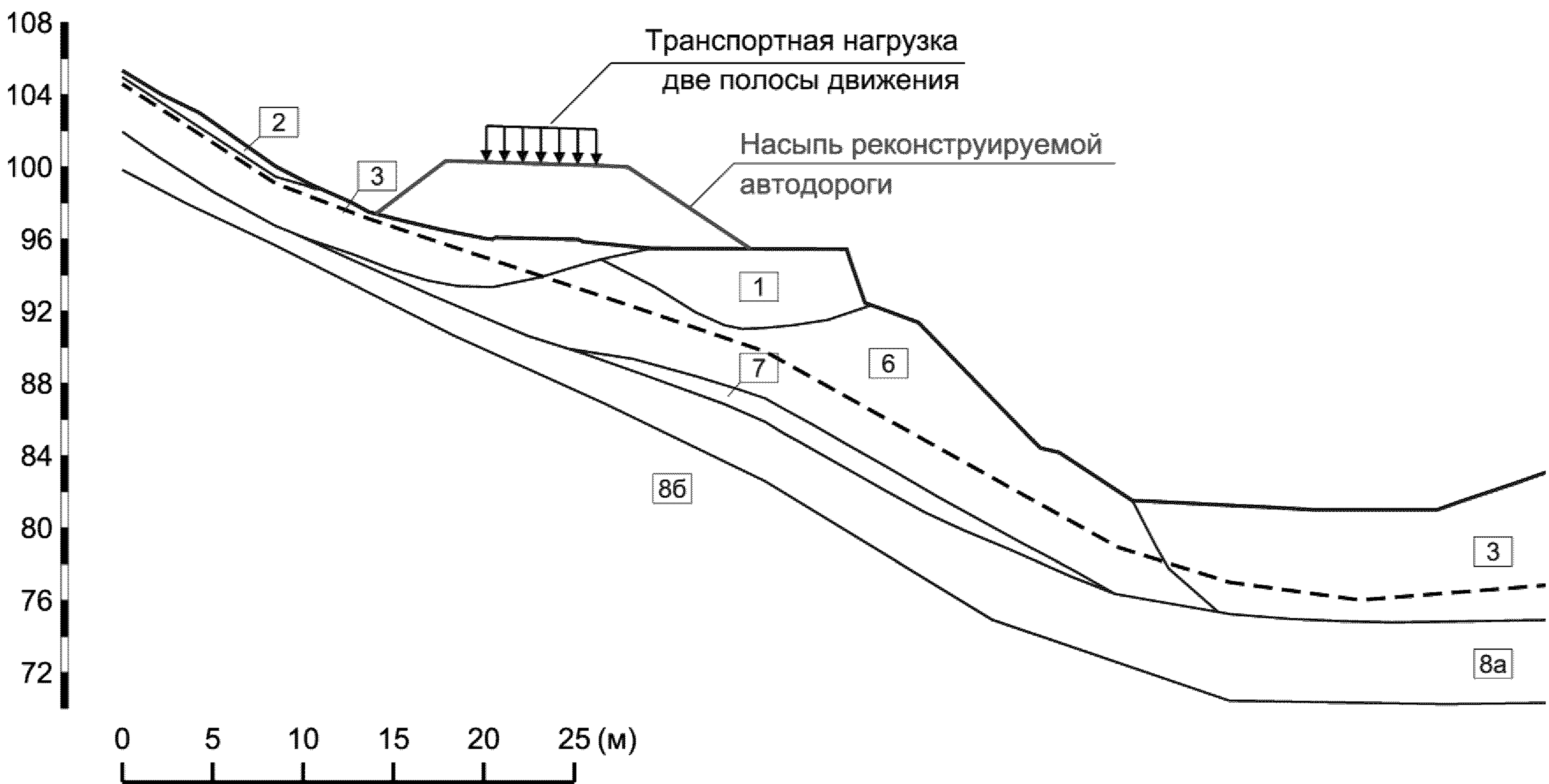
Рисунок Б.1 – Расчетная схема по линии разреза 3-3
