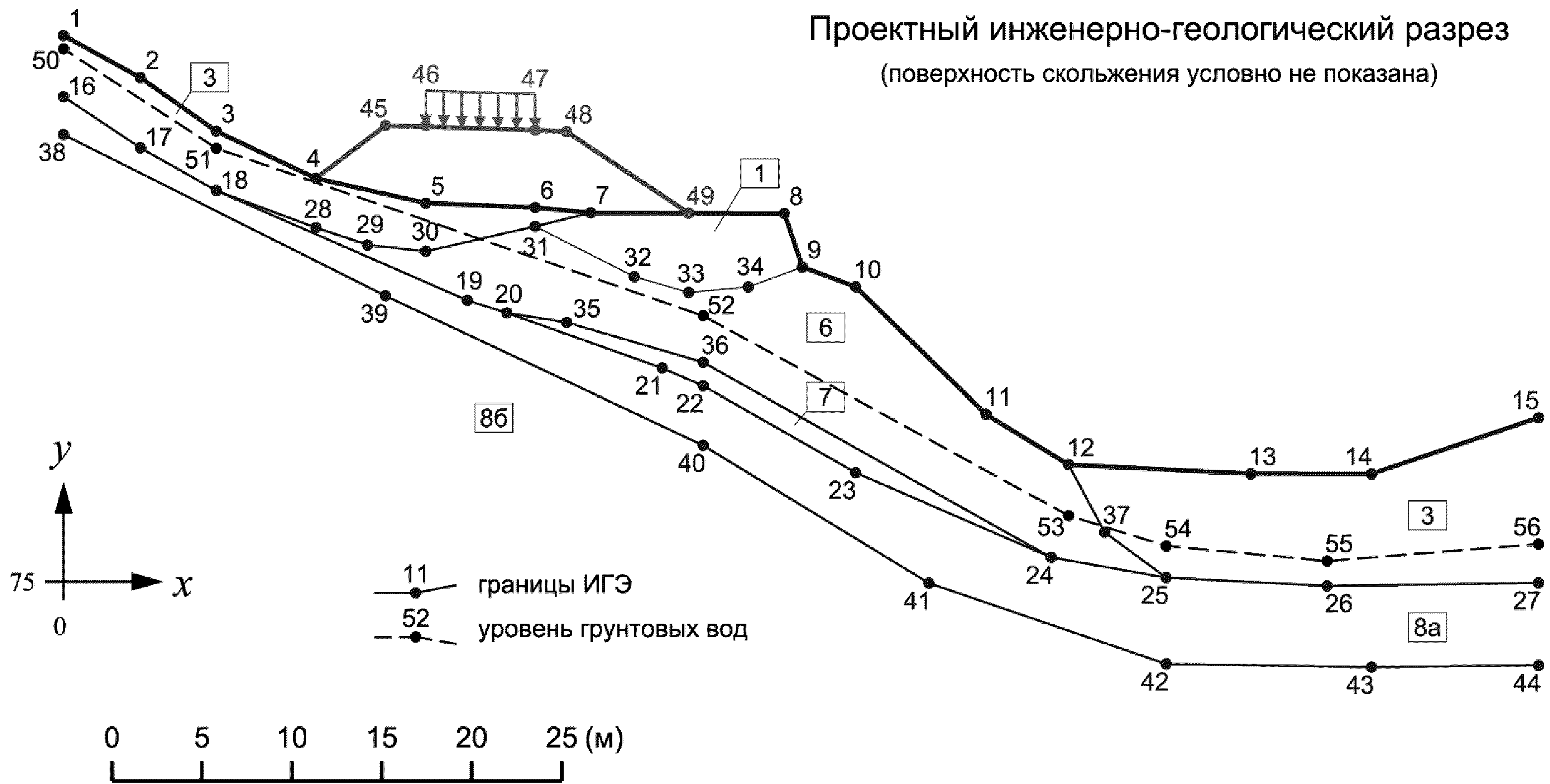
Рисунок Б.2 – Результаты генерализации расчетной схемы
