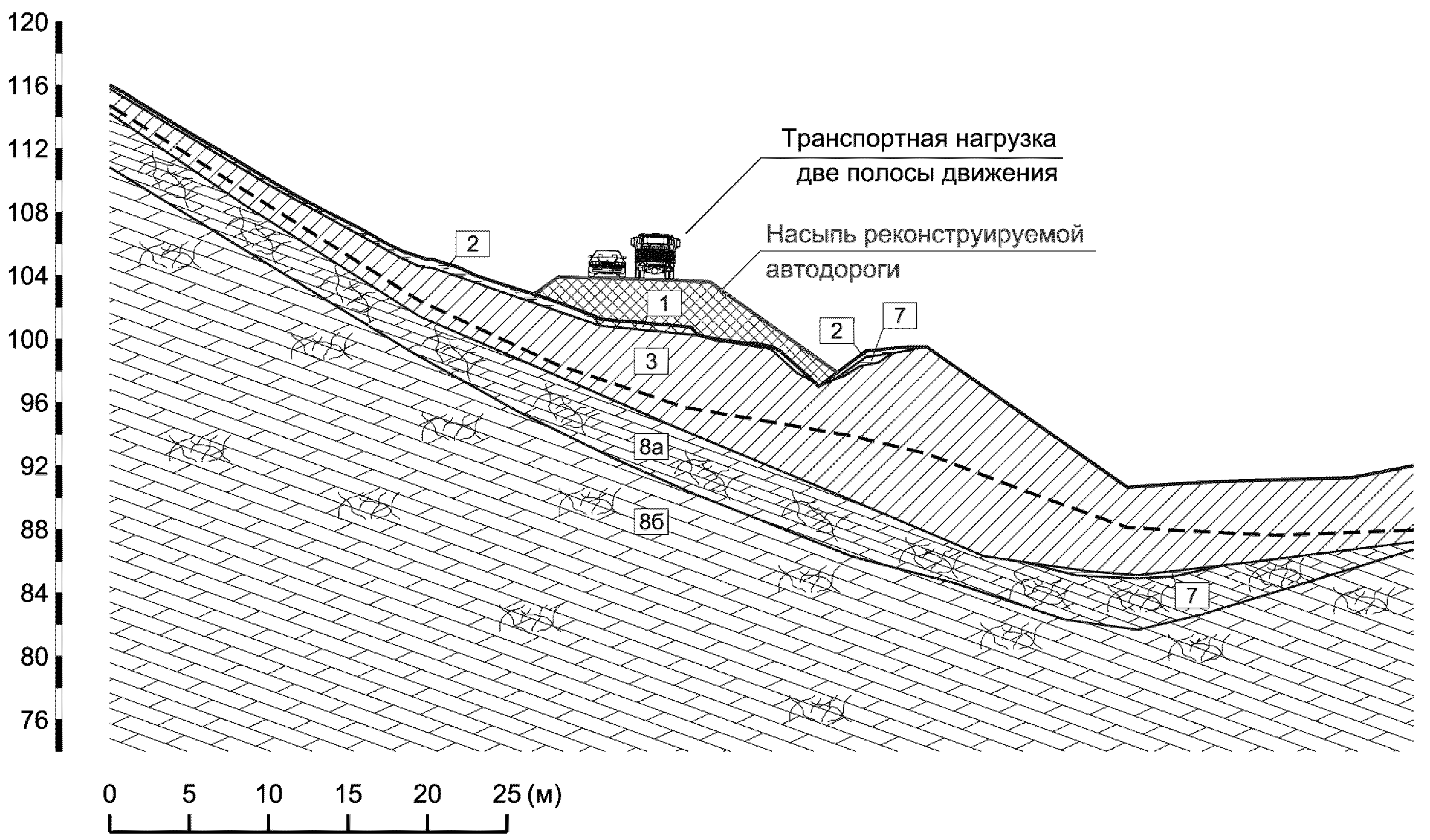
Рисунок А.7 – Инженерно-геологический разрез линии 4-4
