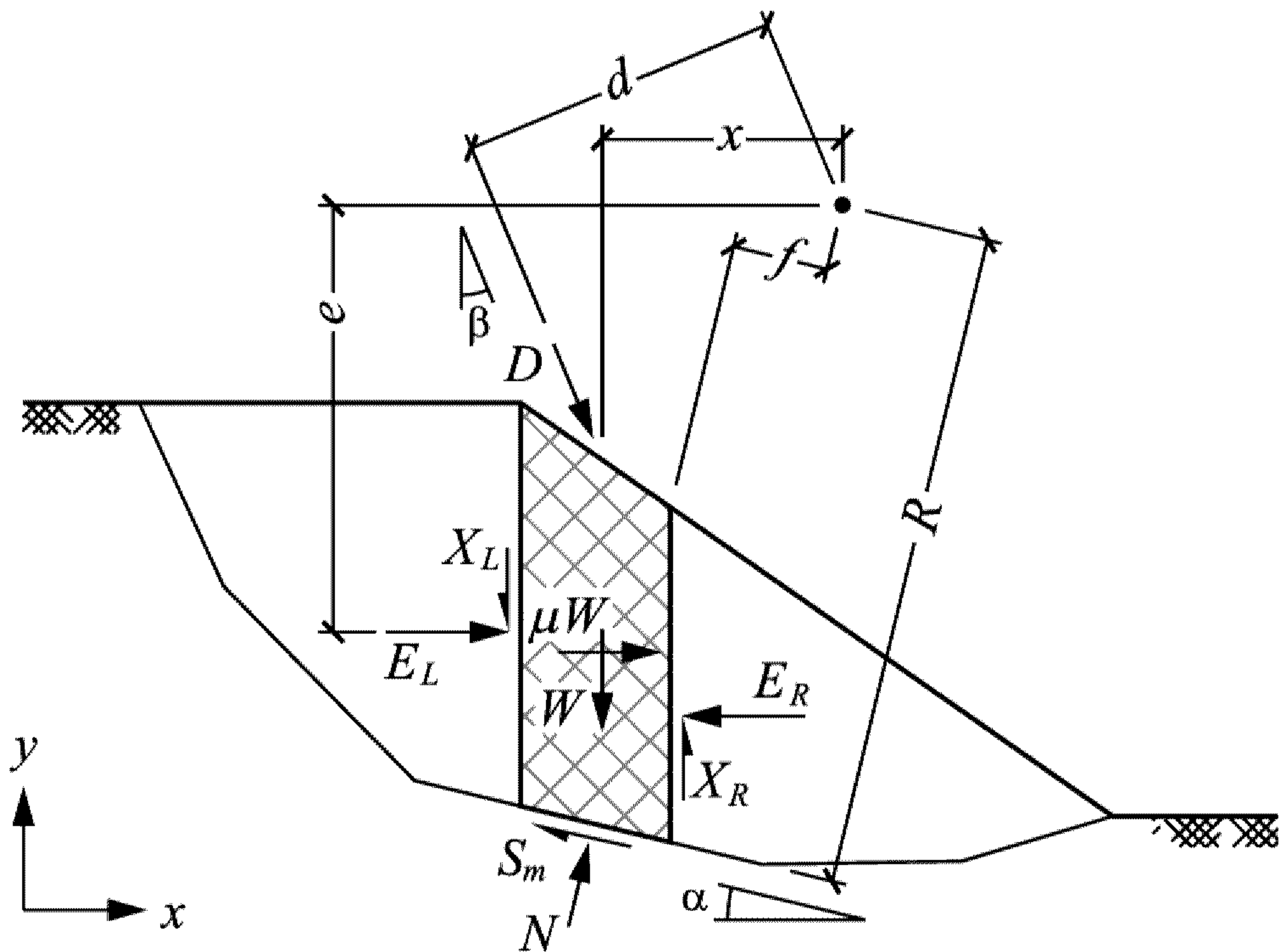
Рисунок 1 – Расчетная схема метода общего предельного равновесия
