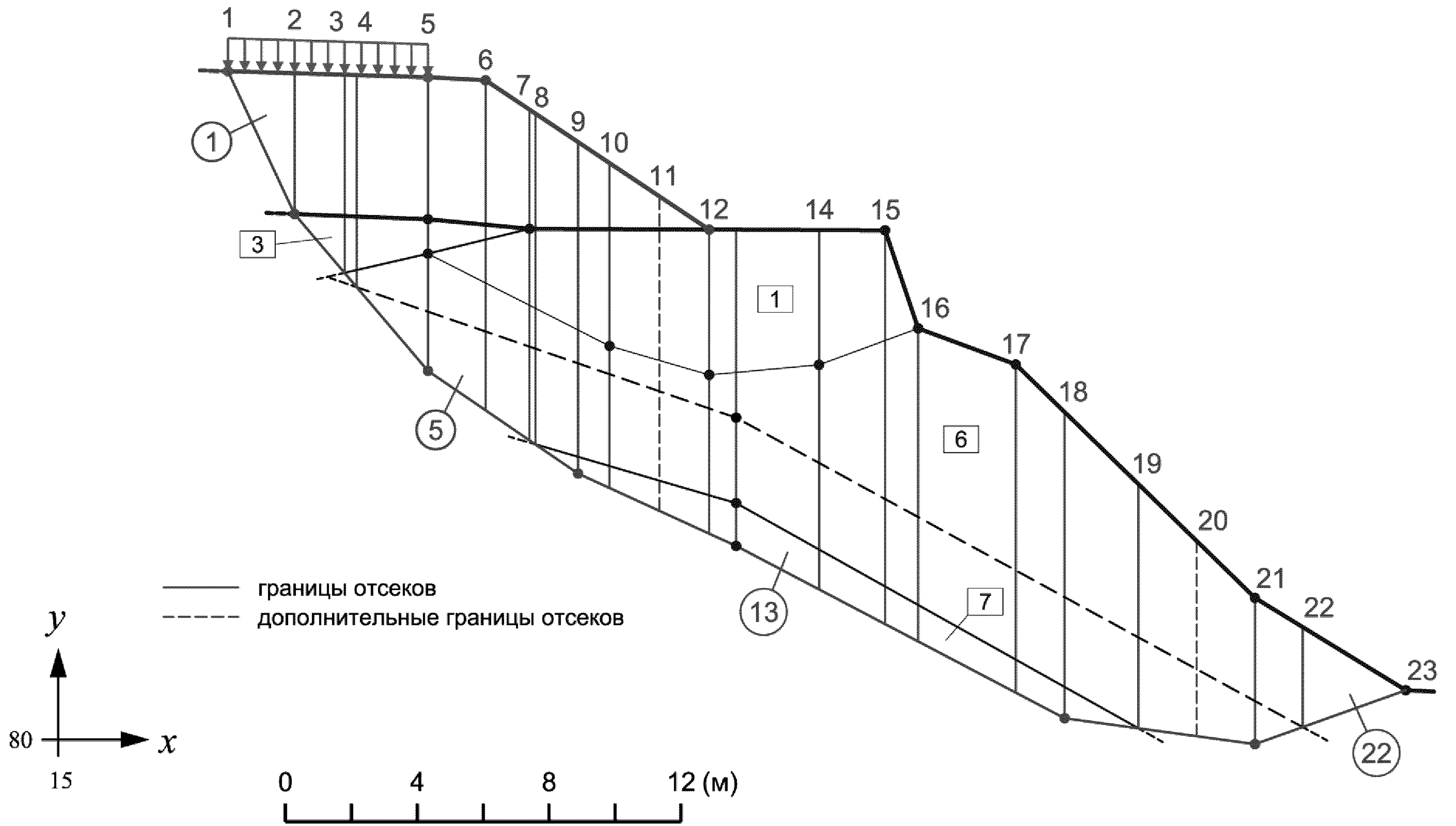
Рисунок Б.4 – Отсековая модель оползня
