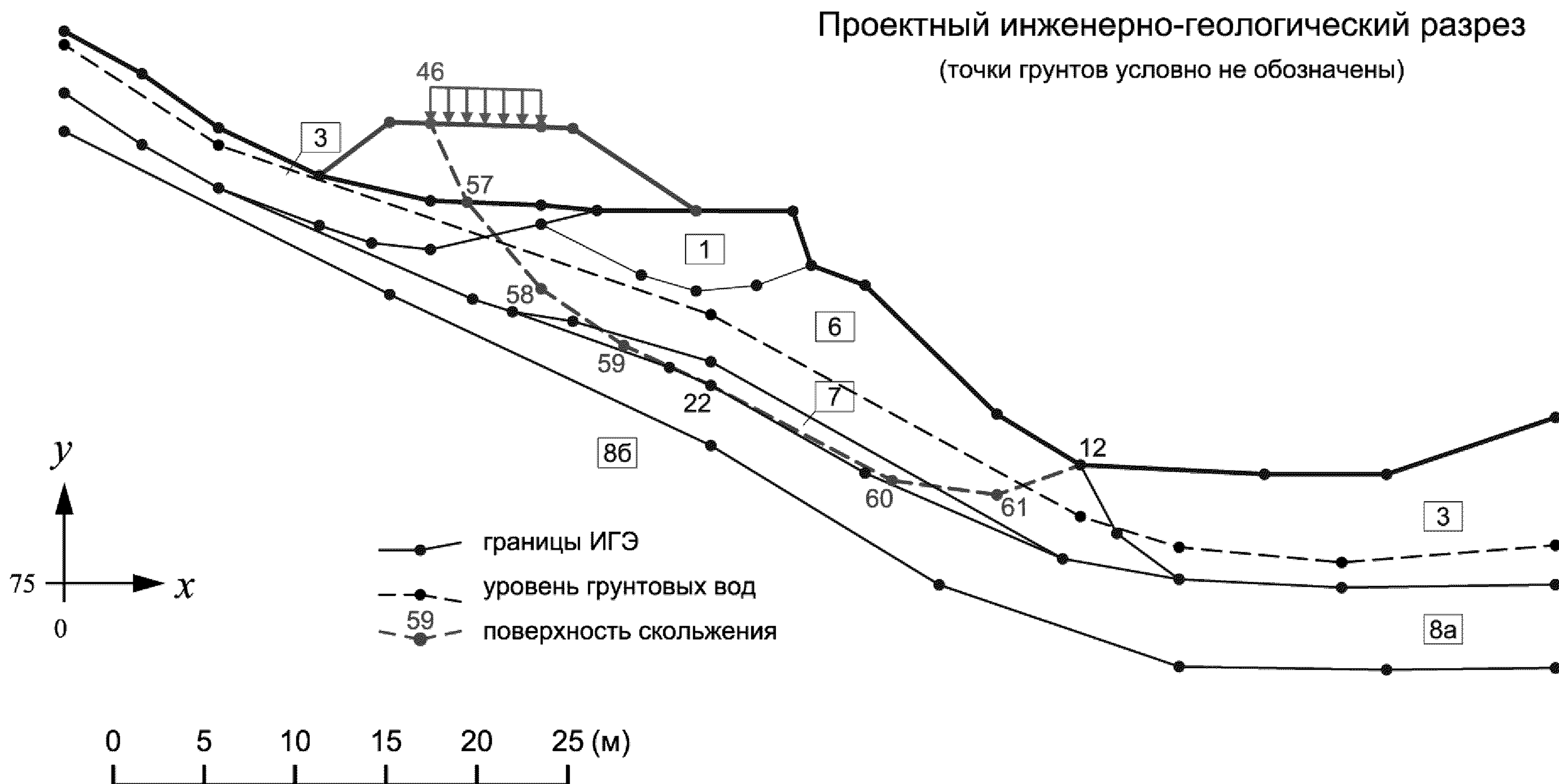
Рисунок Б.3 – Расчетная схема с поверхностью скольжения
