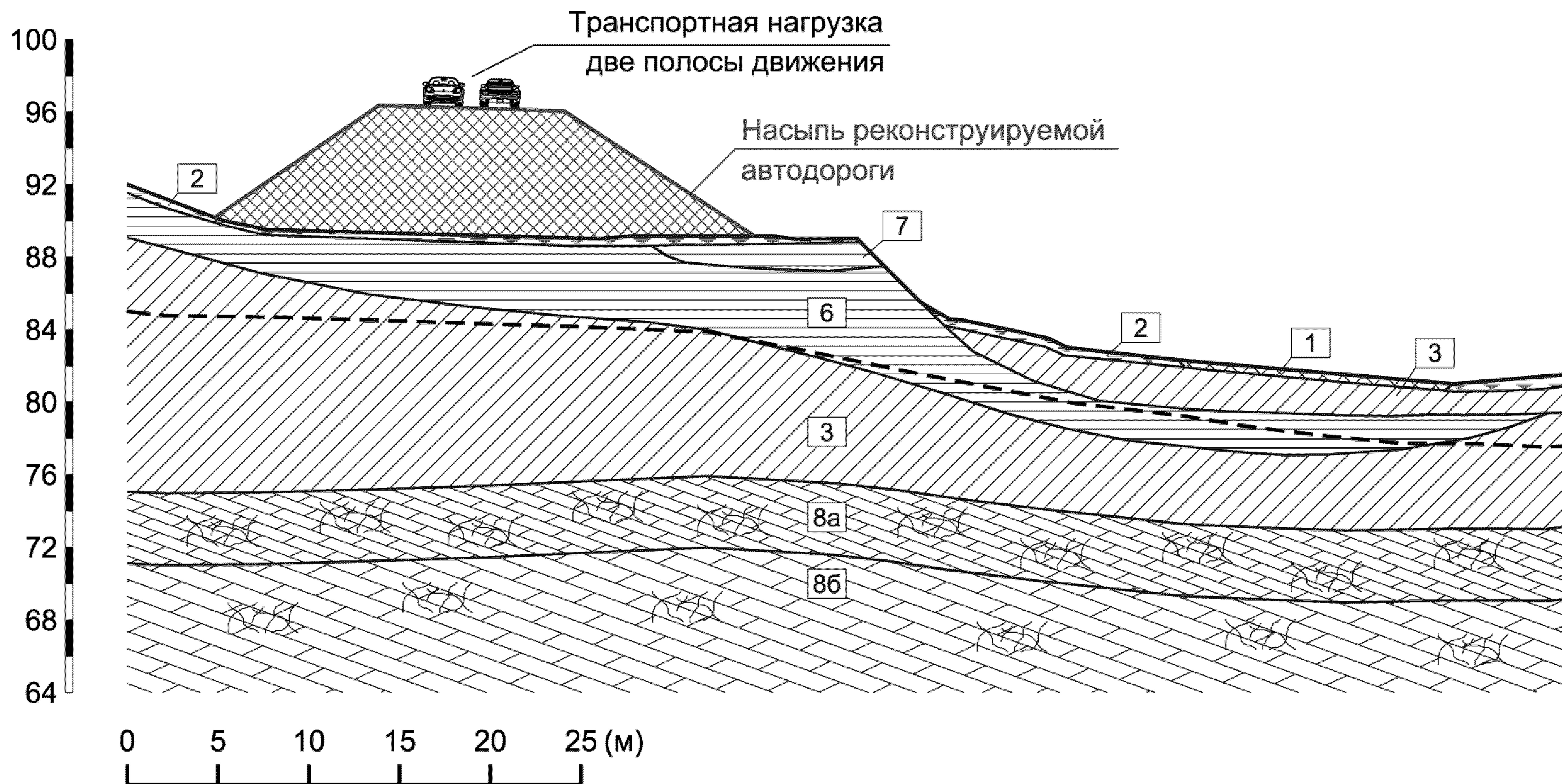
Рисунок А.4 – Инженерно-геологический разрез линии 1-1
