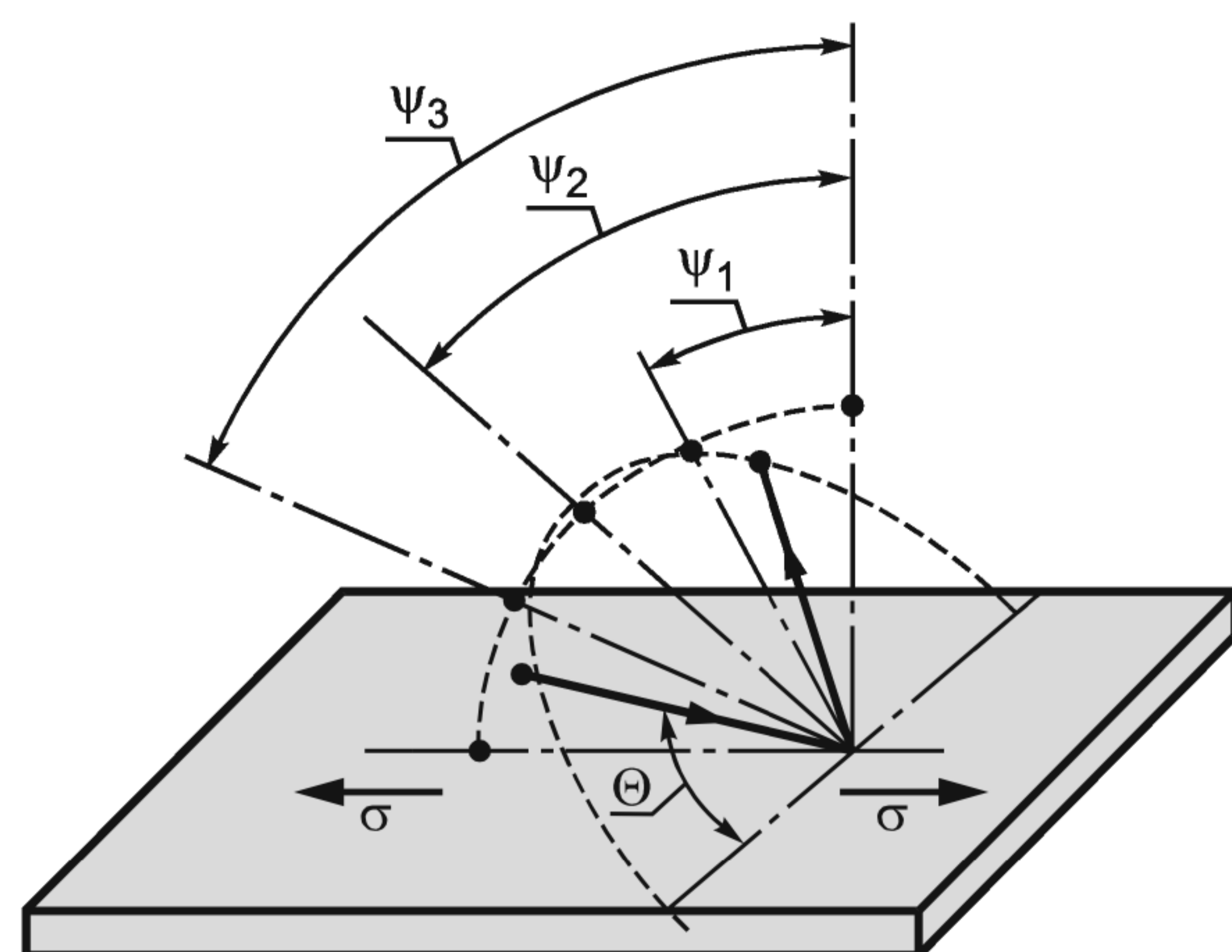
Рисунок 1 — Схема измерения для различных углов \psi
