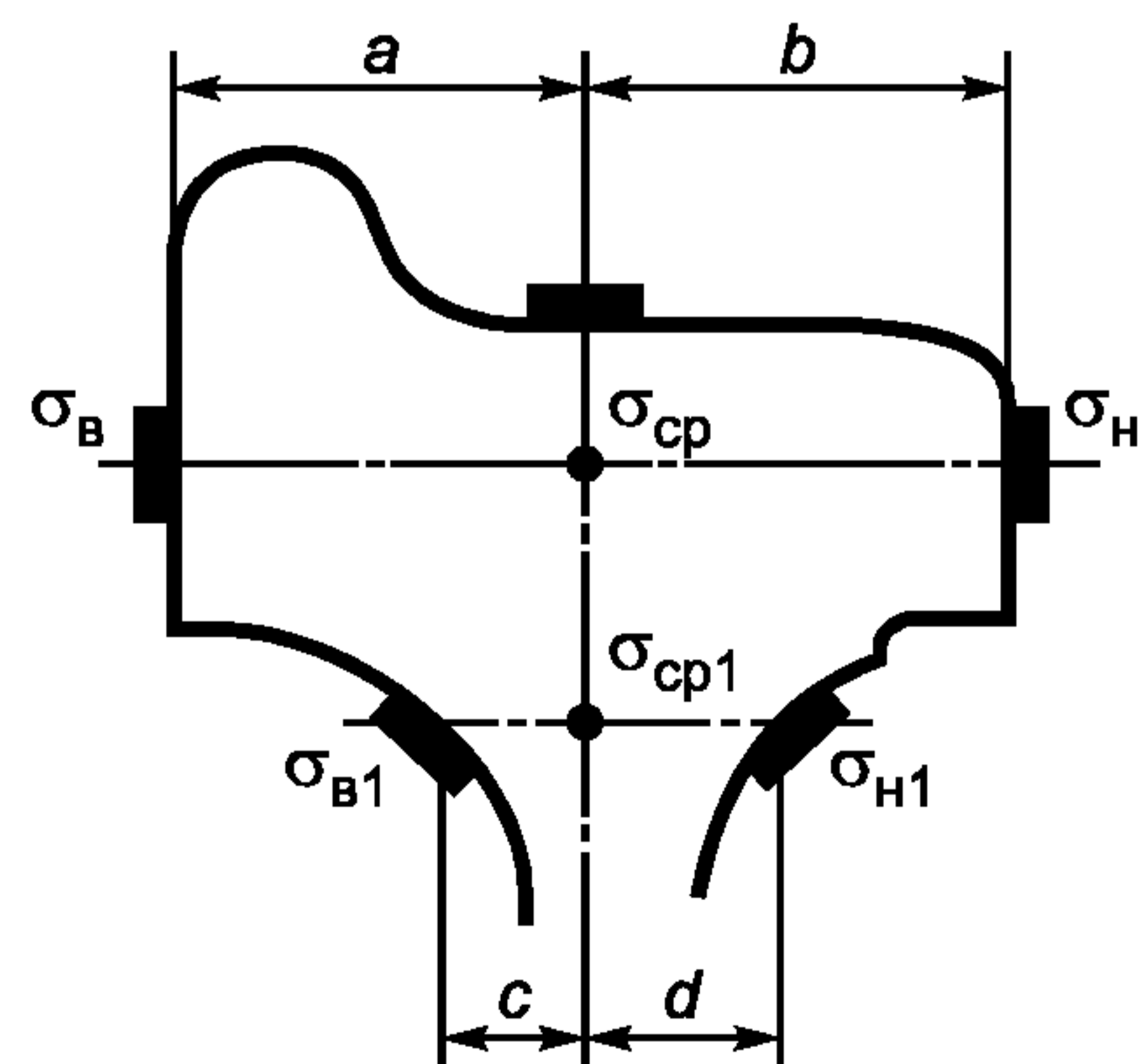
Рисунок А.6 — Схема приведения к плоскости круга катания ( \sigma_{ср} и \sigma_{ср1} ) напряжений замеренных ( \sigma_{в} , \sigma_{н} , \sigma_{в1} , \sigma_{н1} ) на боковых поверхностях обода (бандажа) и прибородной части диска
