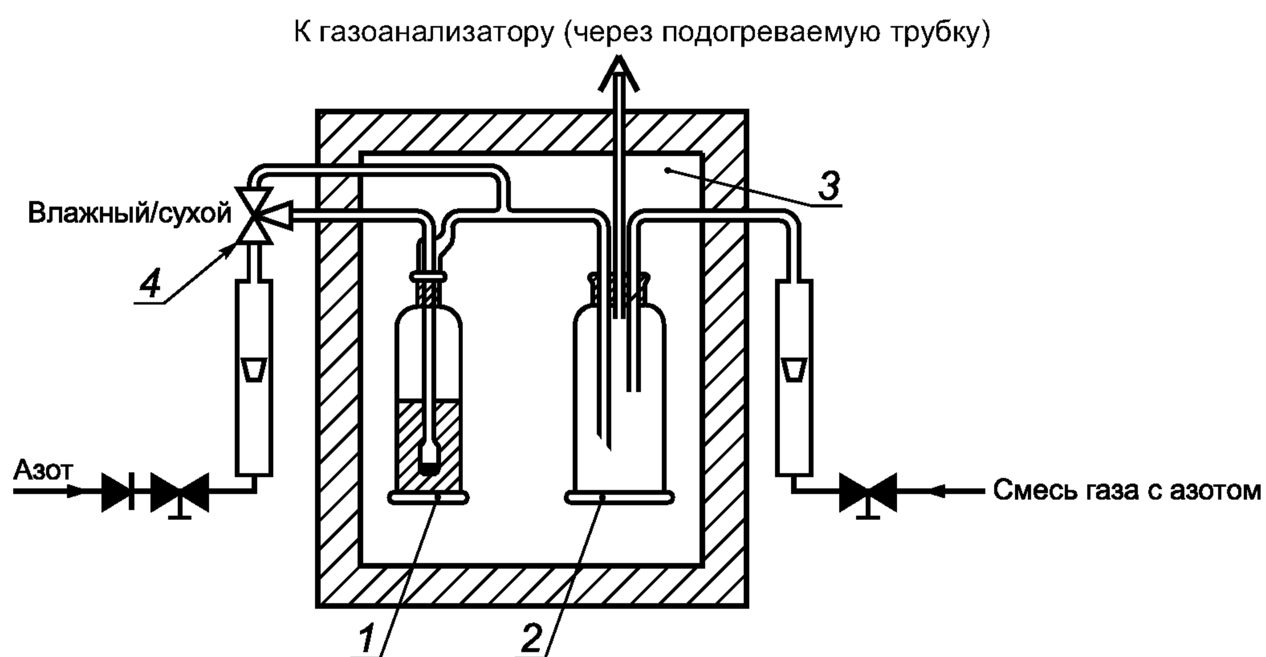
Рисунок А.3а — Простое устройство увлажнения газовой смеси для системы отбора пробы
