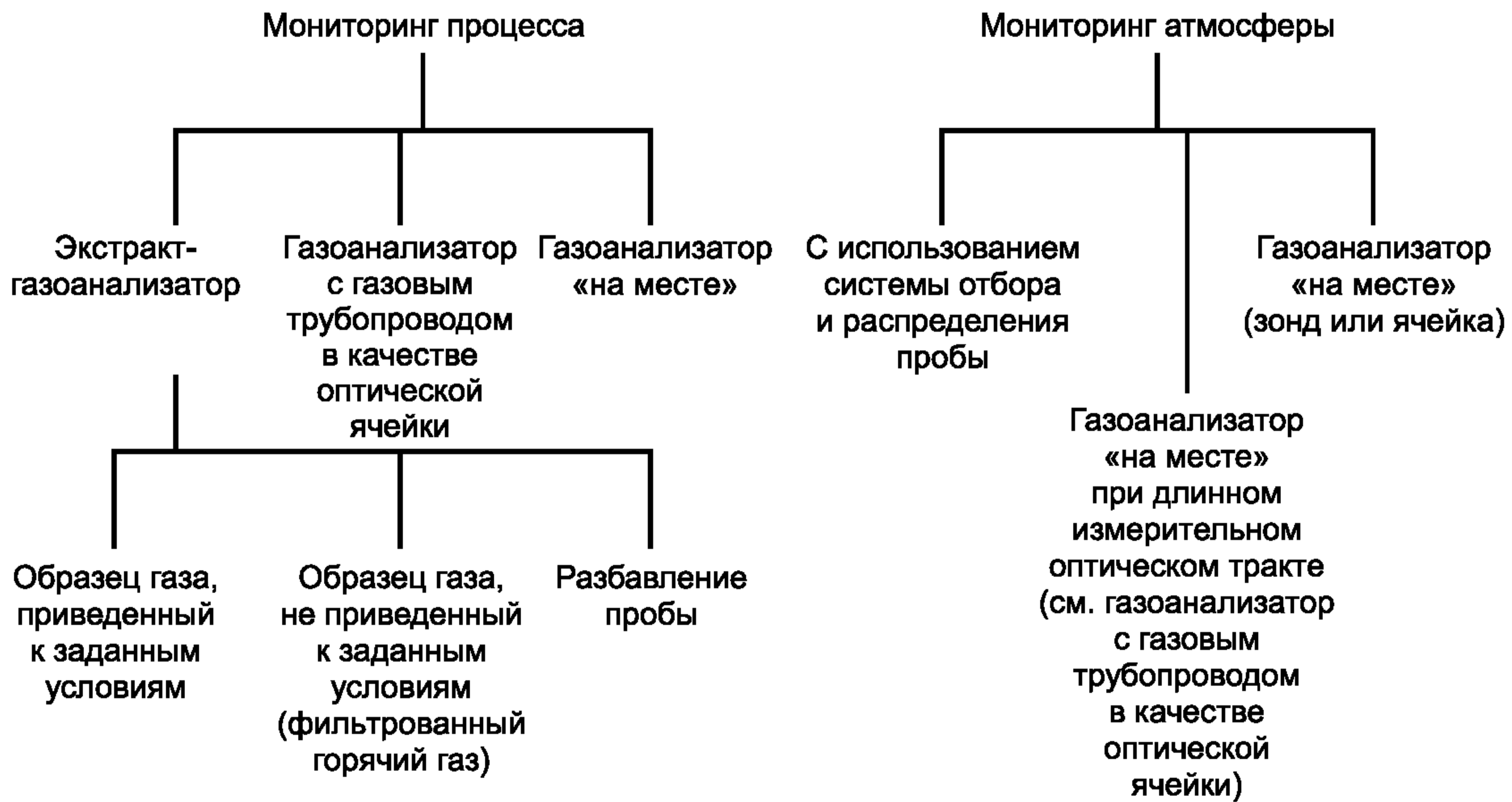
Рисунок А.2 — Системы анализа для газов
