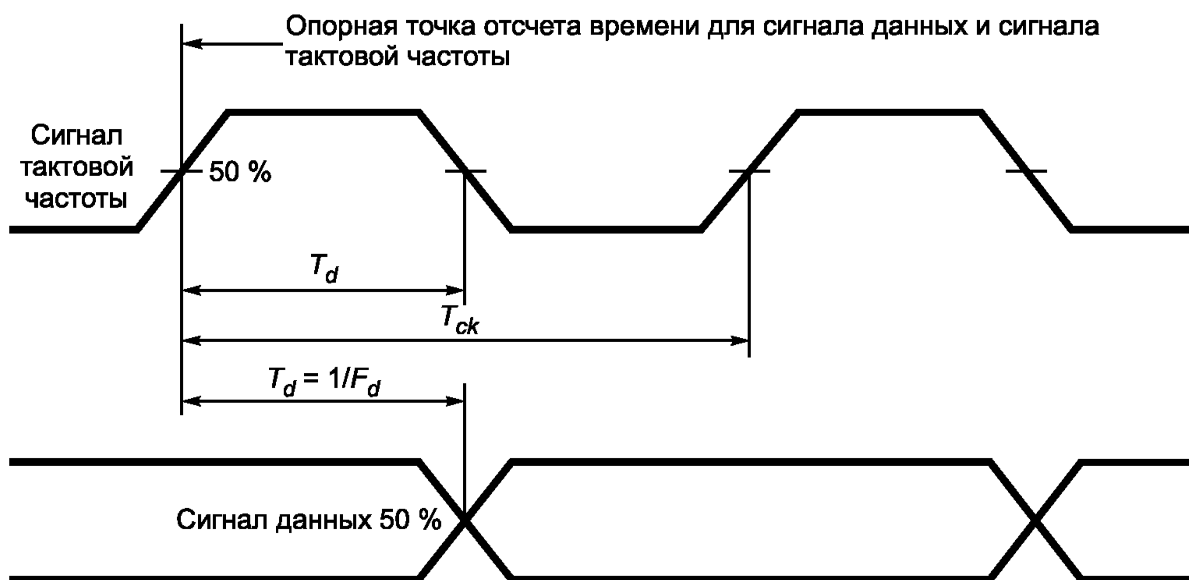
Рисунок 7 — Соотношения параметров синхронизации сигнала и данных
