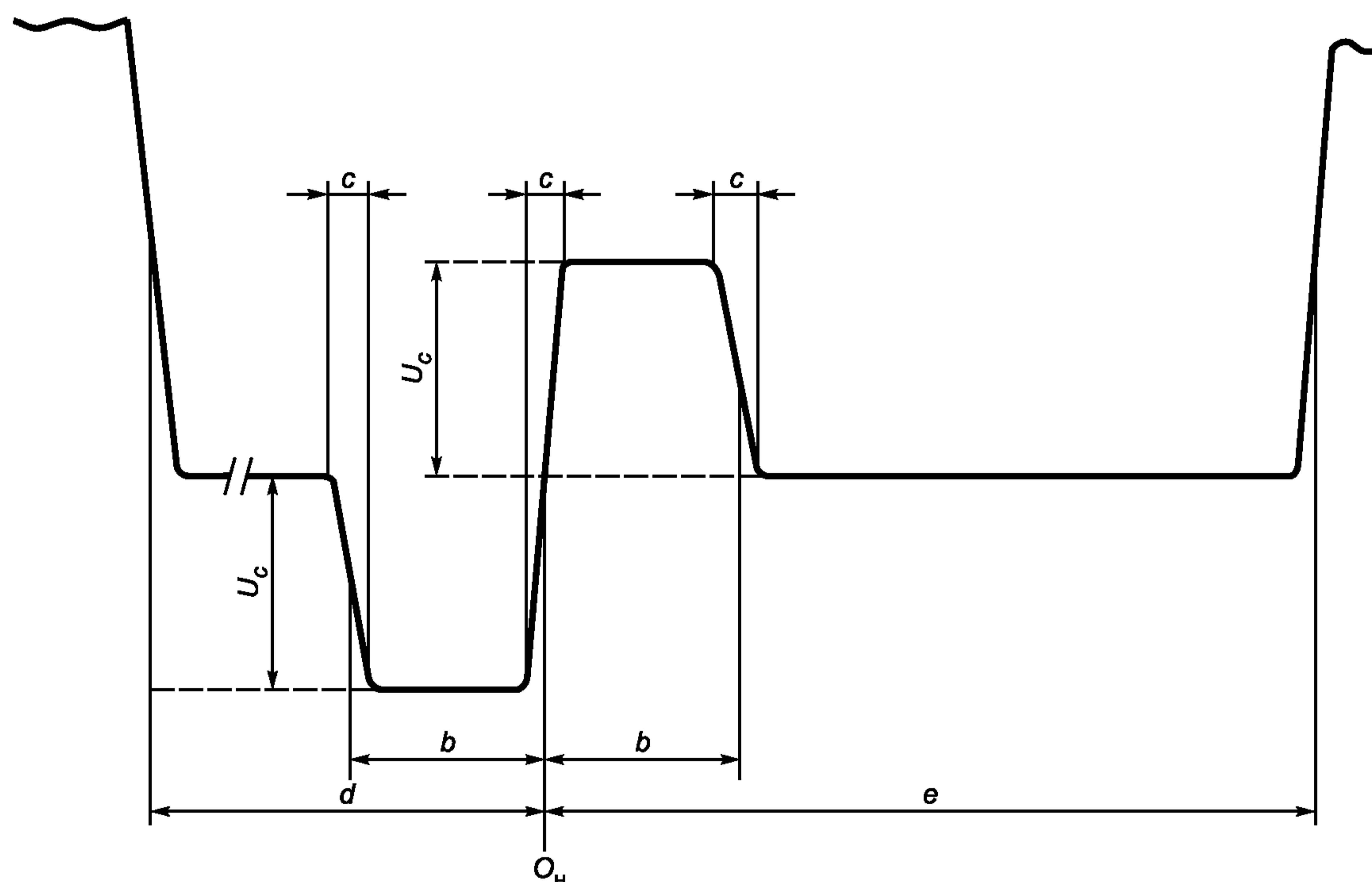
Рисунок 2 — Структура сигнала синхронизации на интервале гашения строки
