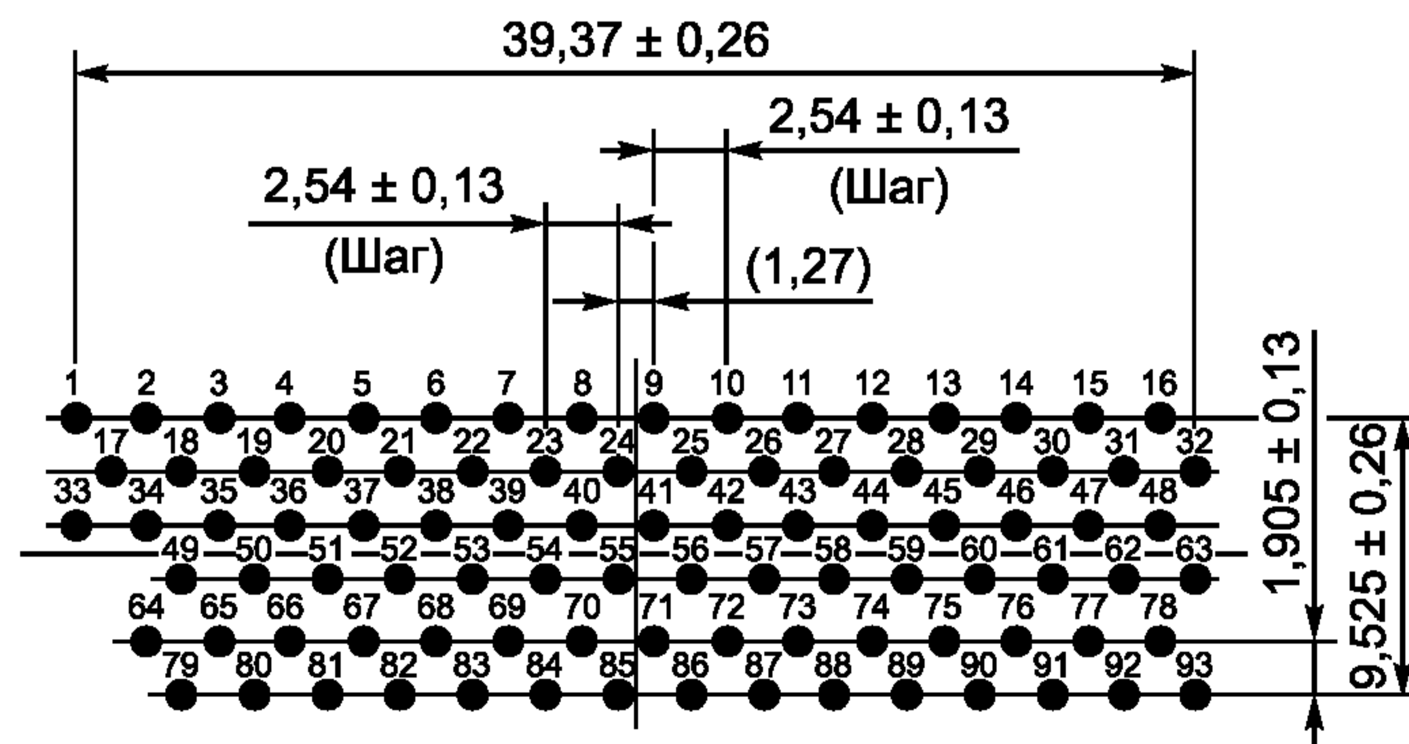
Расположение контактов
