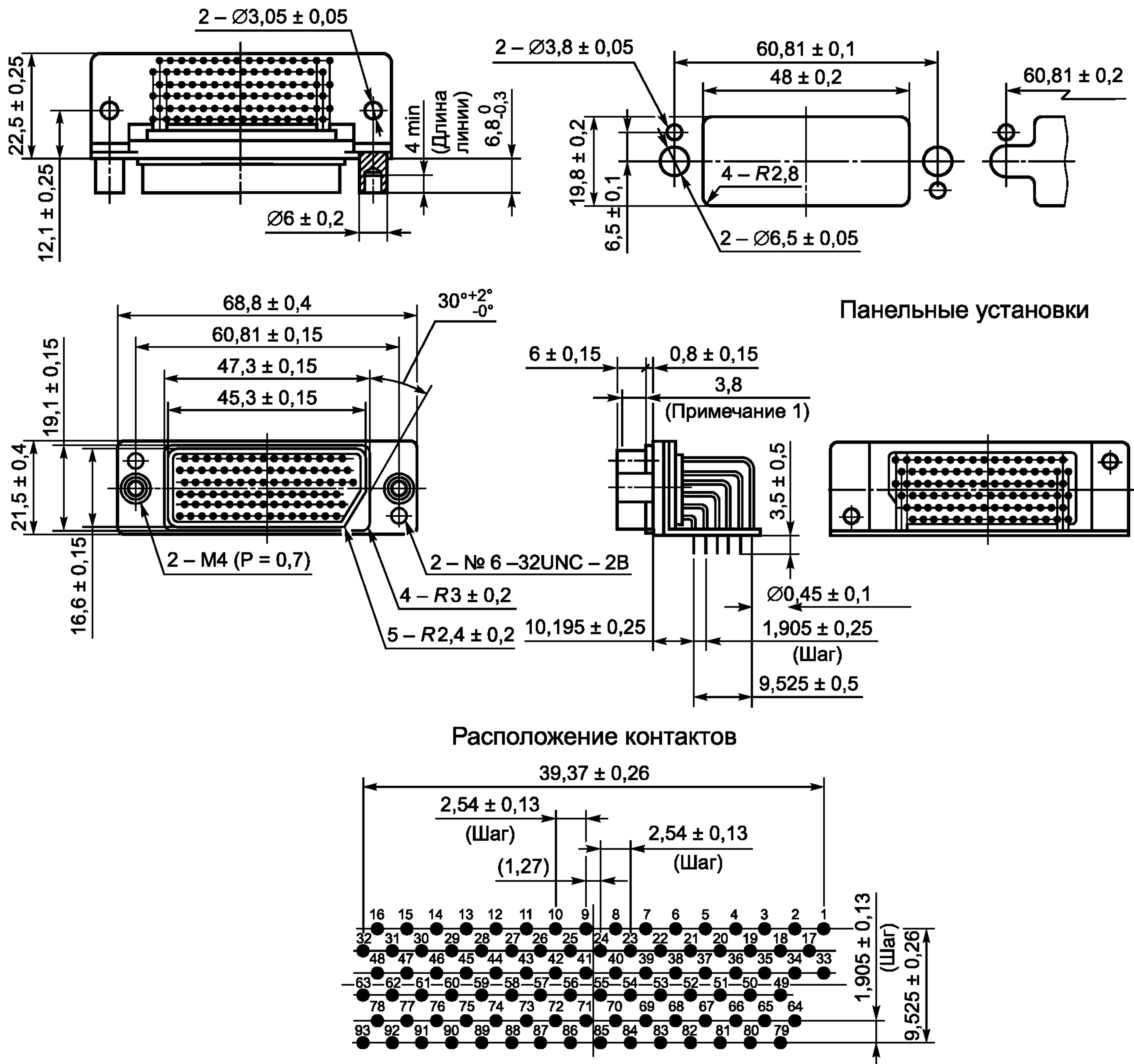
Рисунок 11 — 93-й контактный разъем (розетка)
