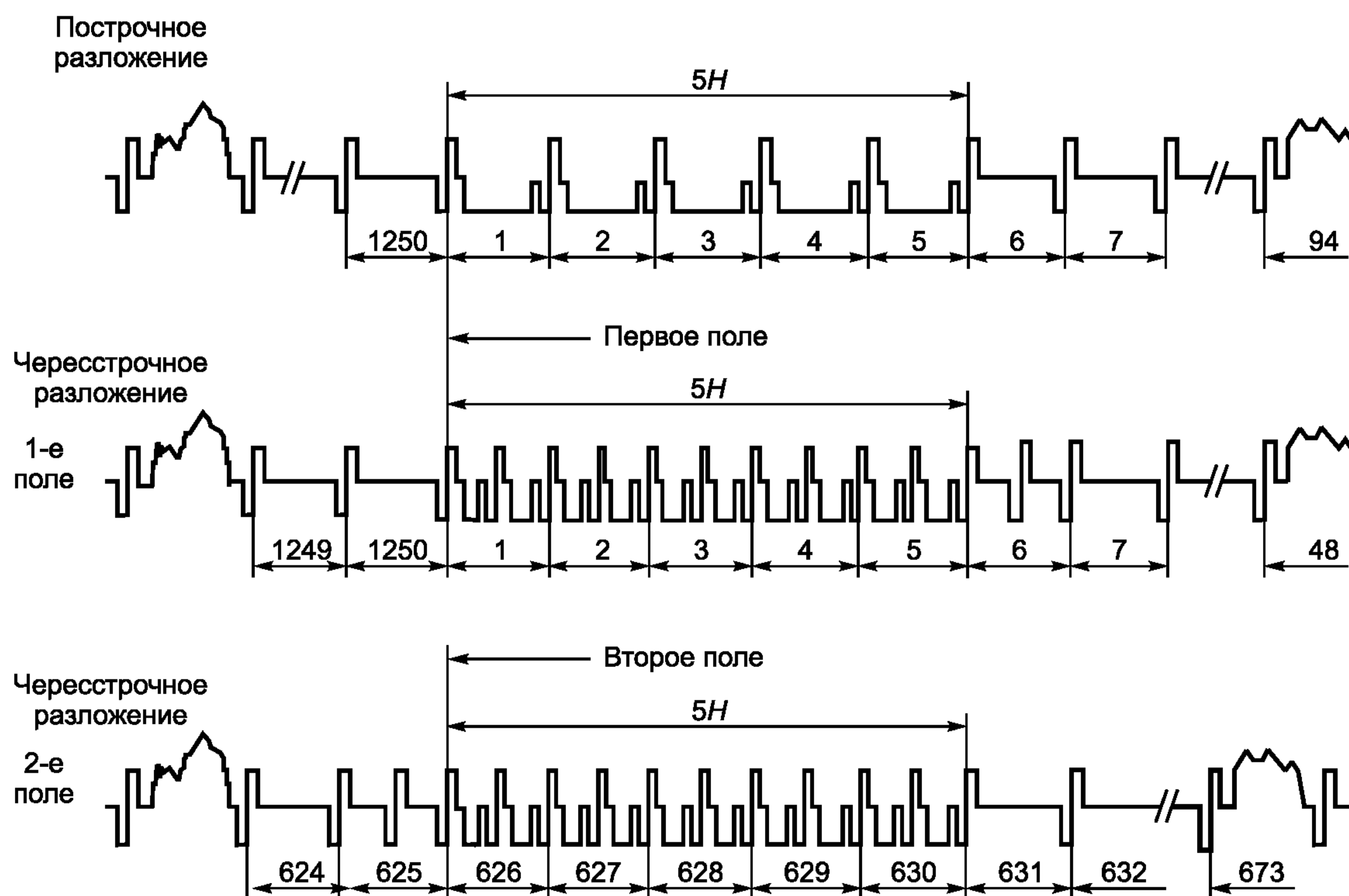
Рисунок 3 — Структура синхросигнала на интервале гашения поля
