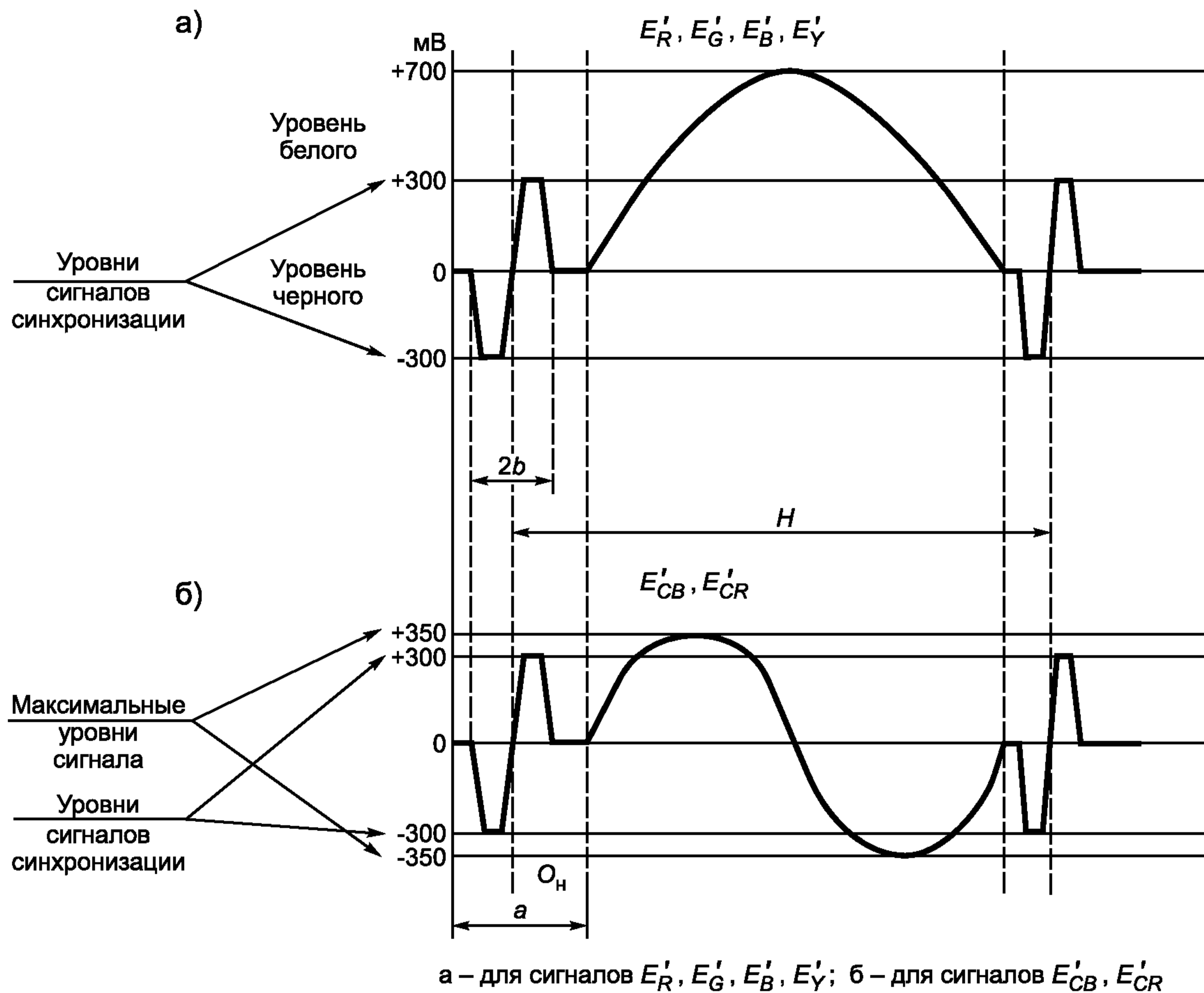
Рисунок 1 — Структура компонентных сигналов на интервале строки
