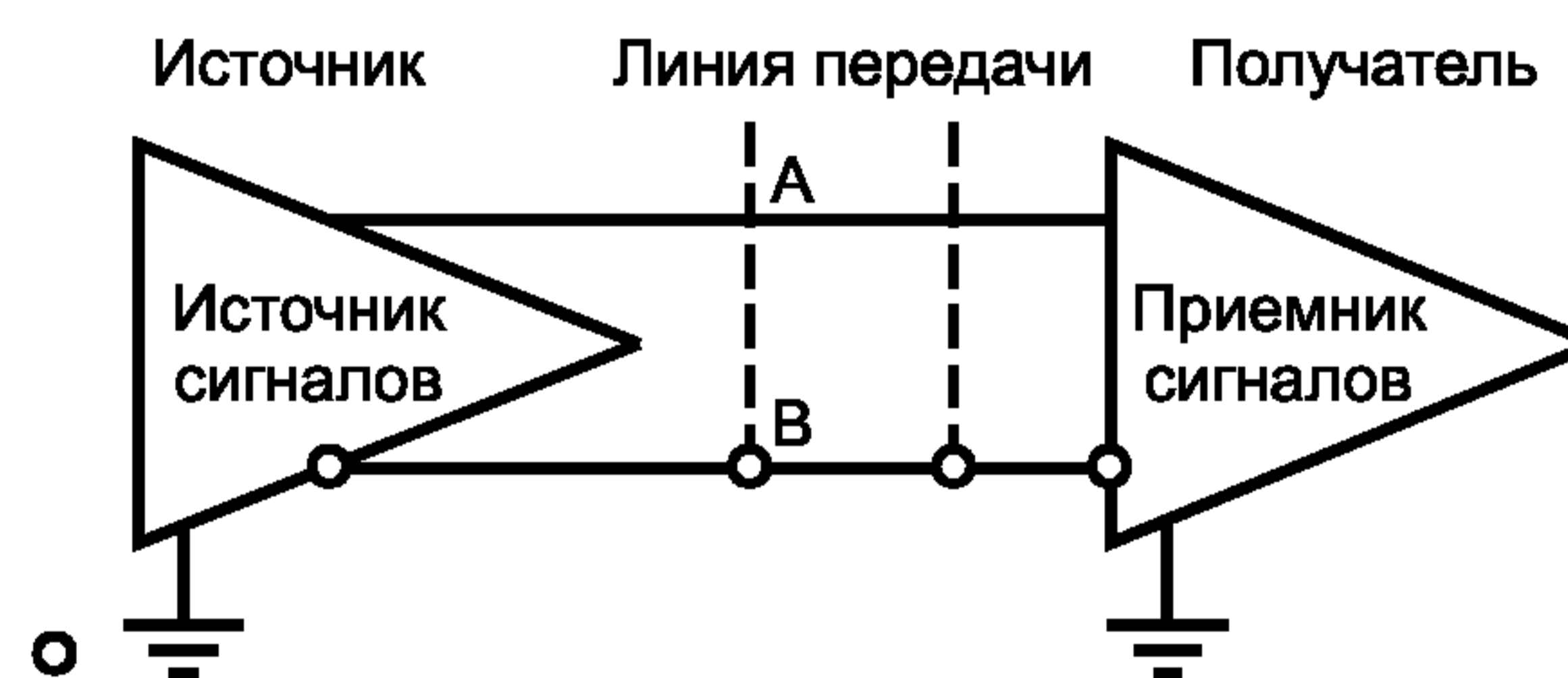
Рисунок 8 — Соединение источника сигналов и приемника сигналов
