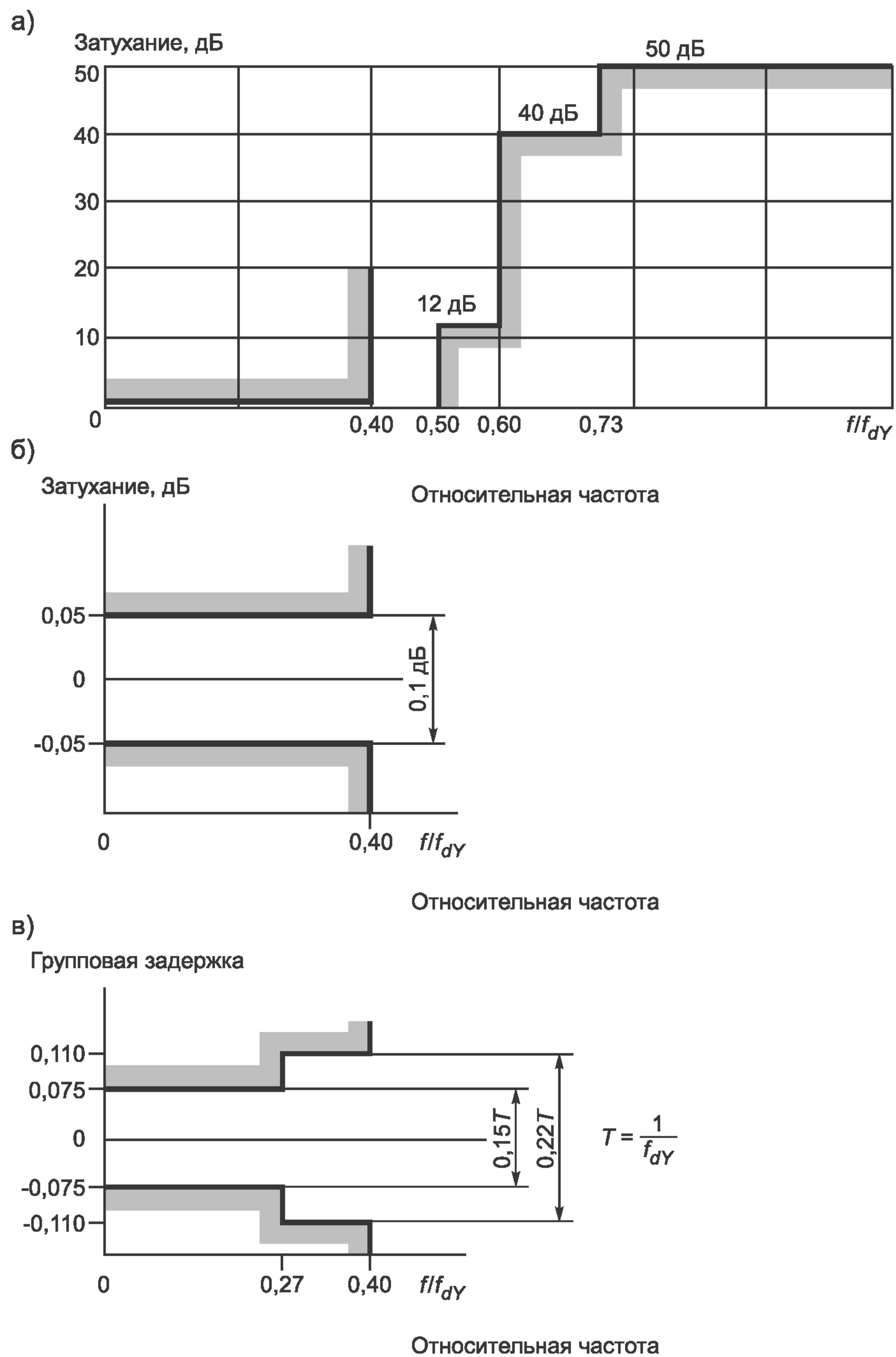
Рисунок А.1 — Характеристики фильтров низких частот для сигналов E_Y
