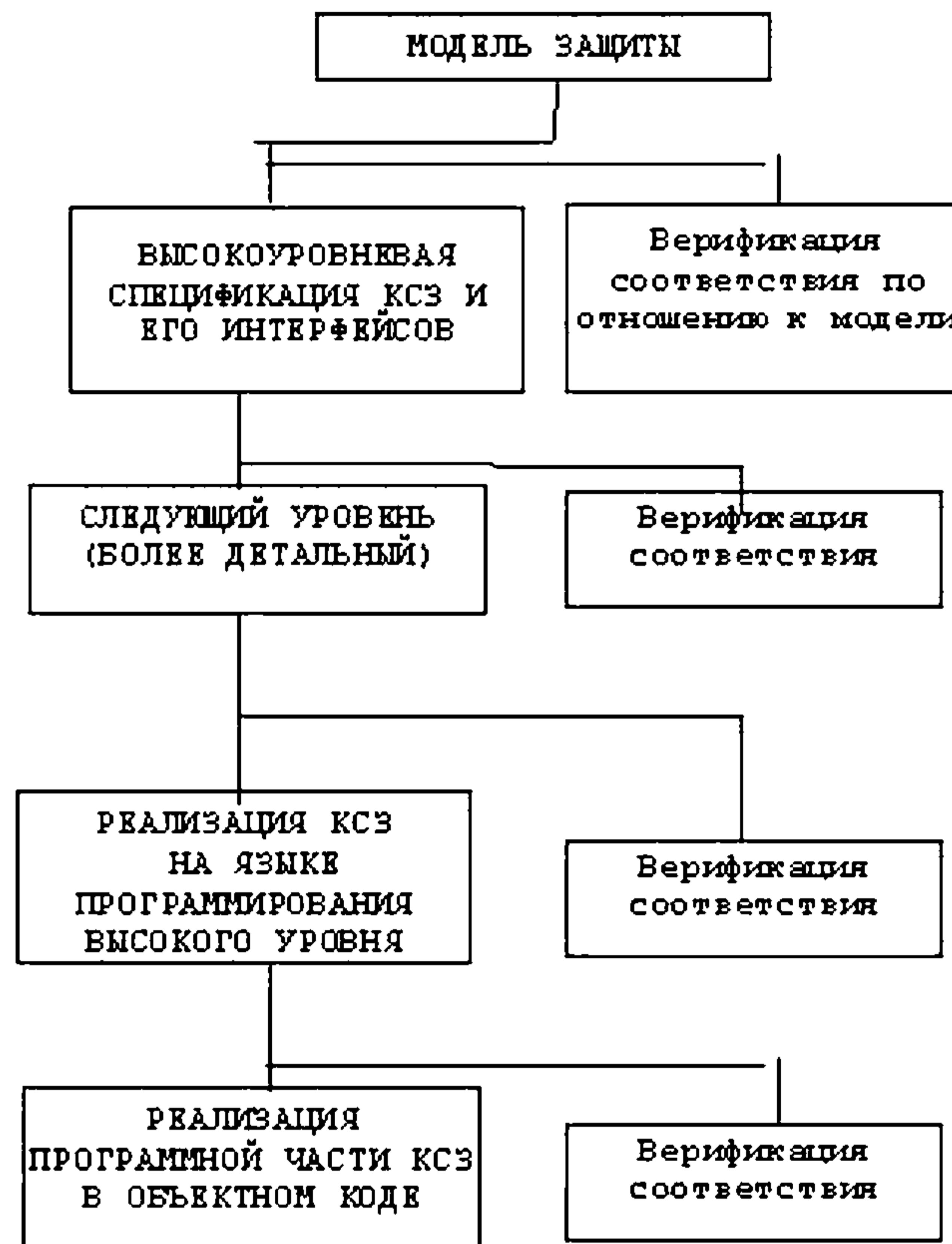
СХЕМА МОДЕЛИ ЗАЩИТЫ (к п. 2.6.9)
