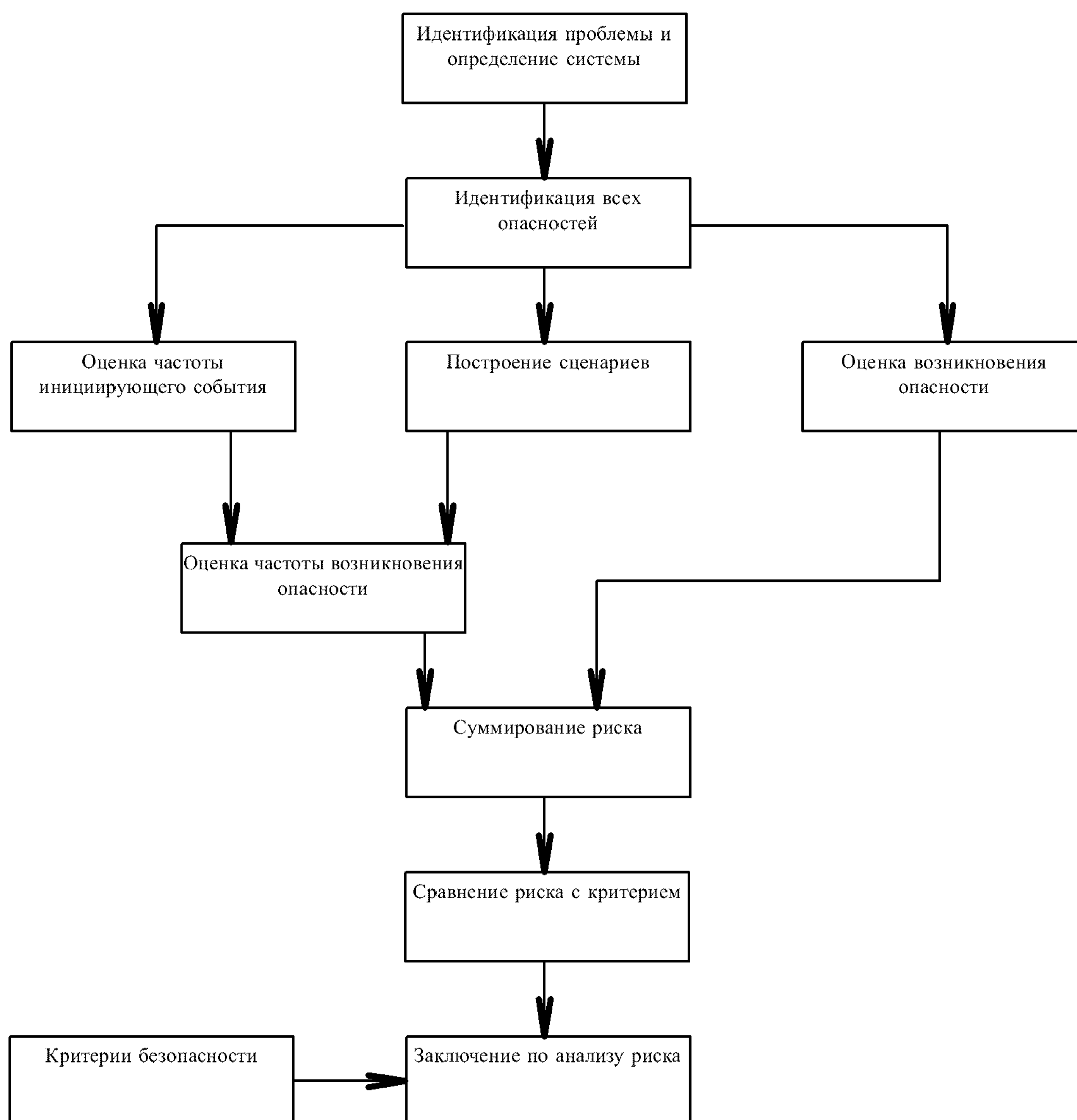
Рис. 2.6.2 Последовательность количественного анализа риска
