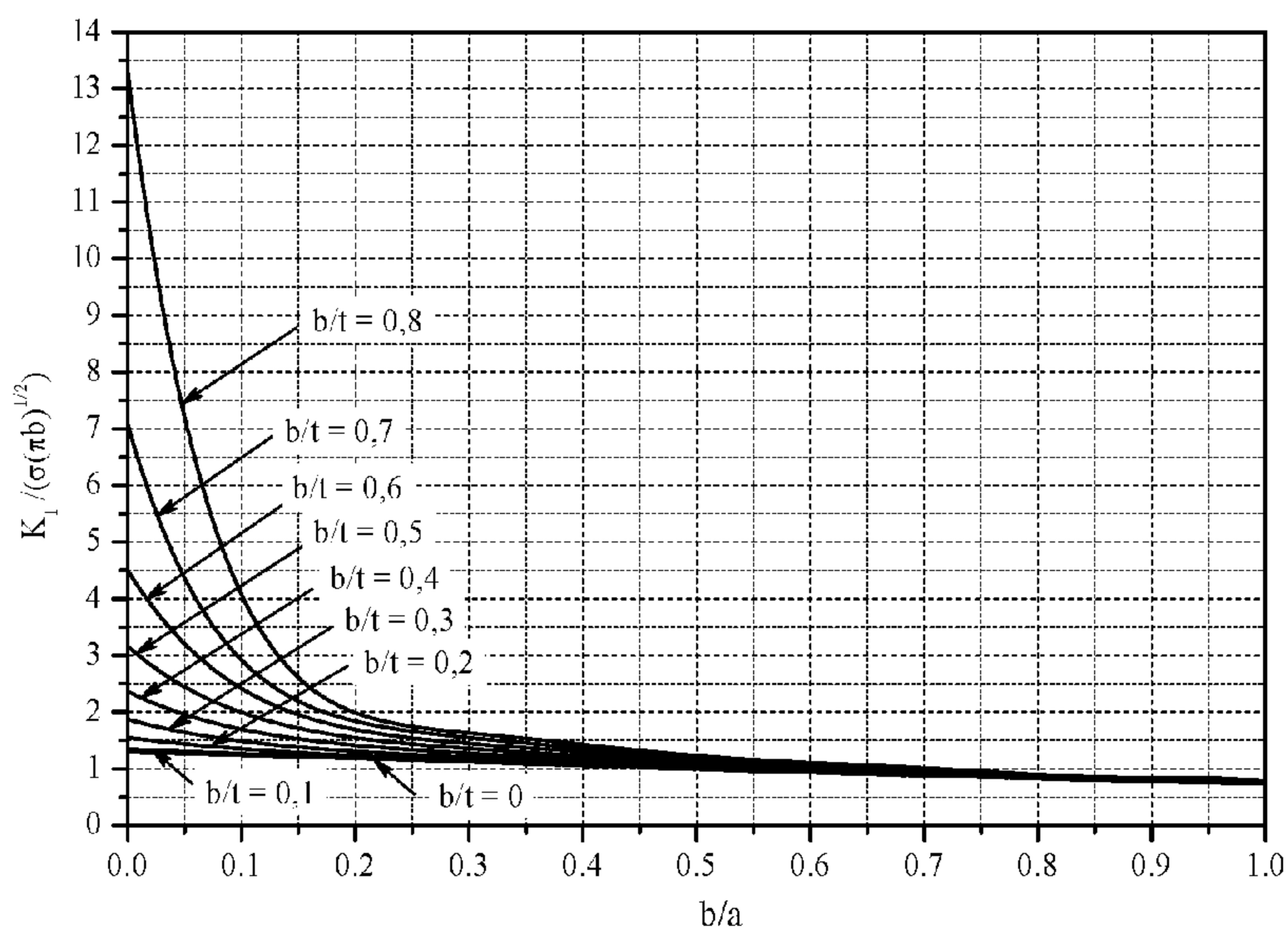
Рис. П.1.1 Значения A_T для продольной внутренней трещины, R/t = 10
