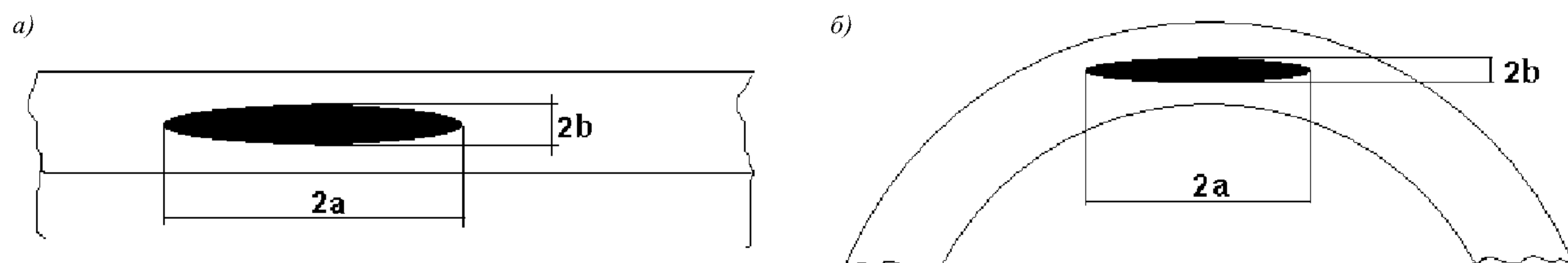
Рис. 8.2 Классификация подповерхностных трещин: а) продольная; б) поперечная
