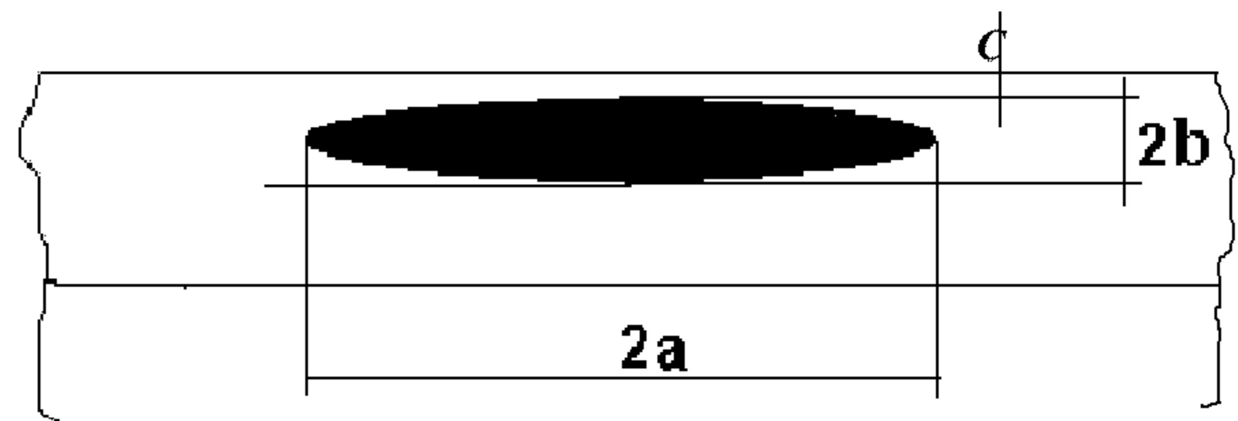
Рис. П.5.1 Геометрические параметры подповерхностной продольной трещины.
