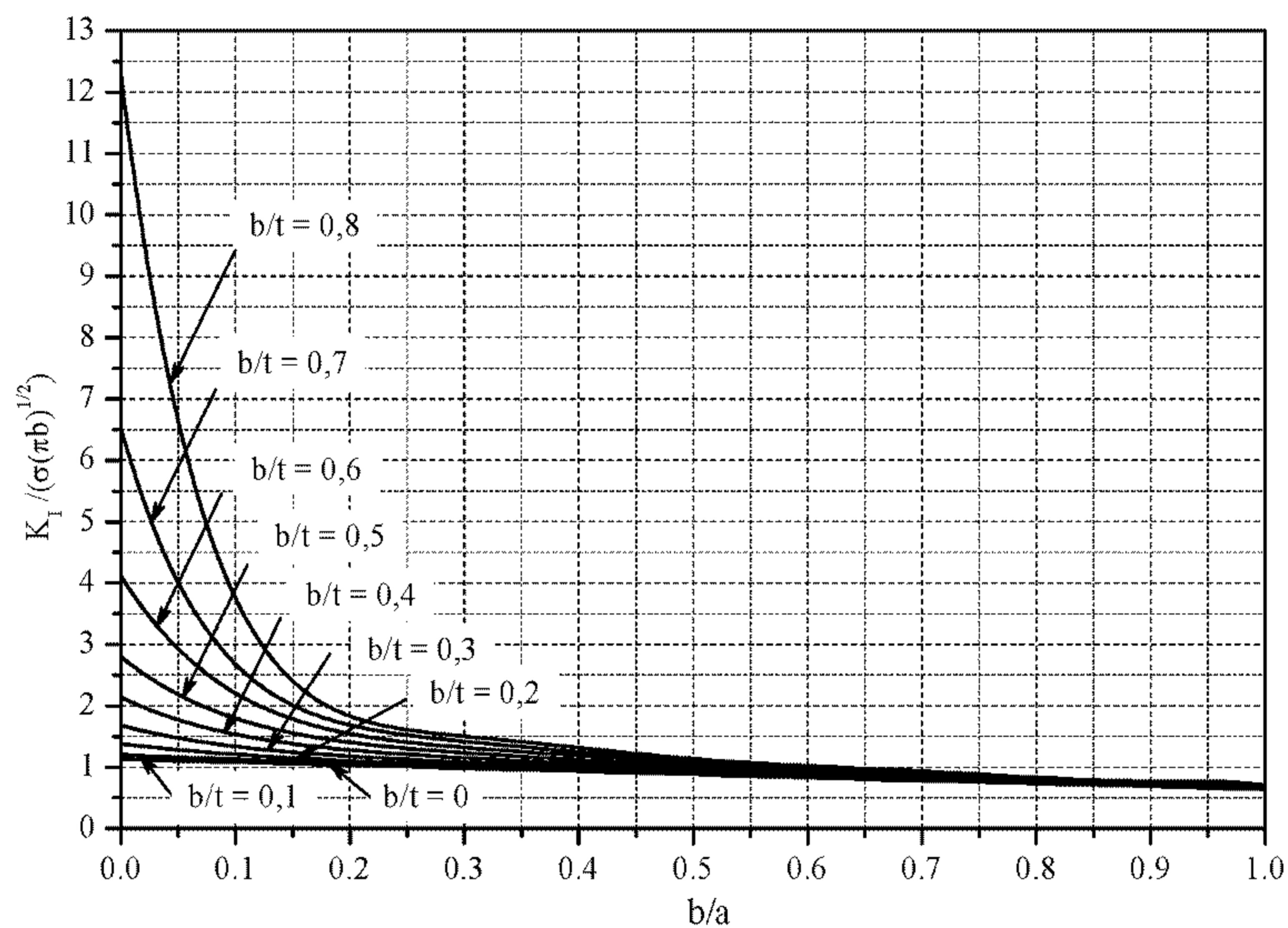
Рис. П.2.4 Значения A_T для продольной внешней трещины, R/t=40
