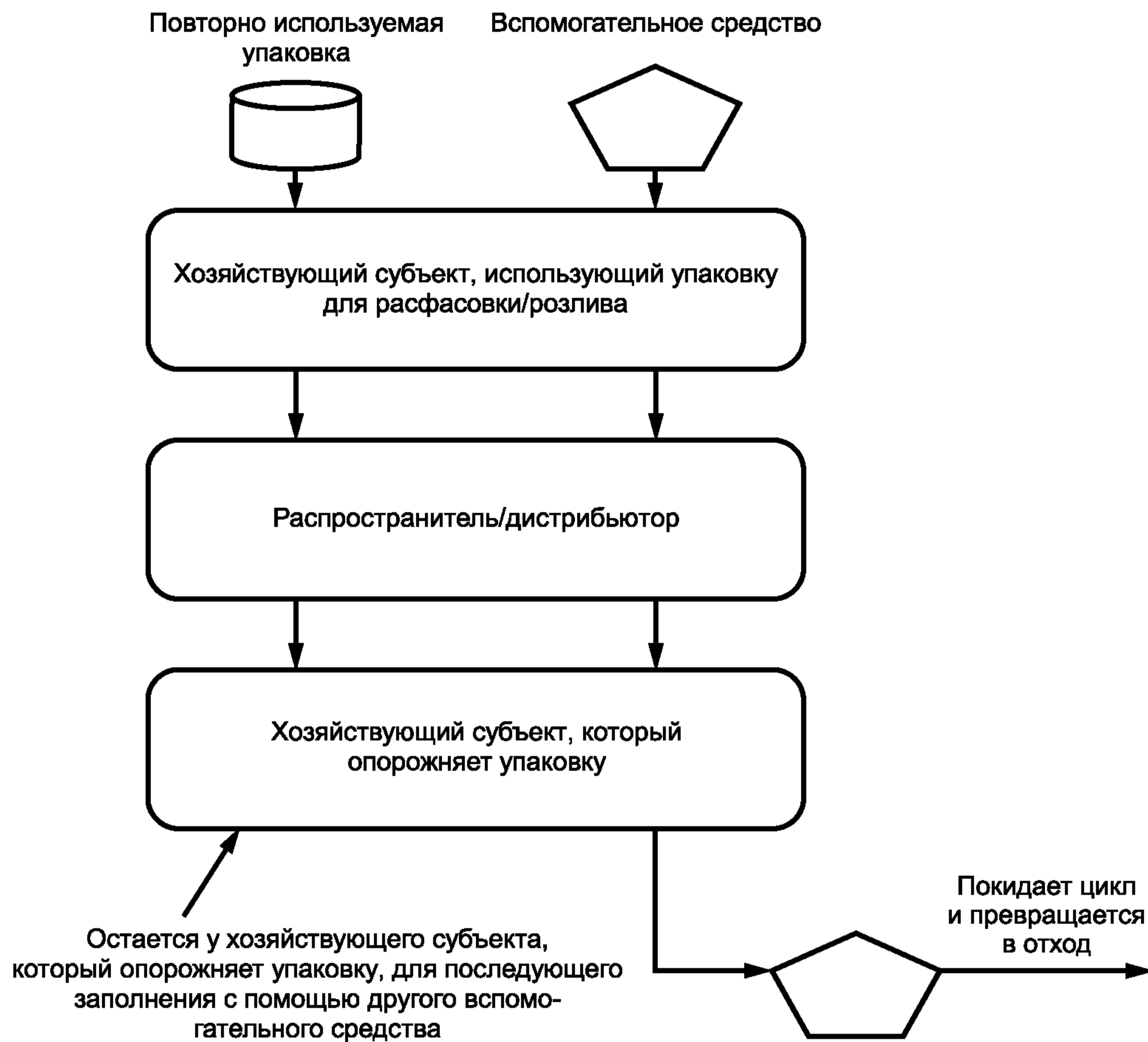
Рисунок 3 — Смешанная система
