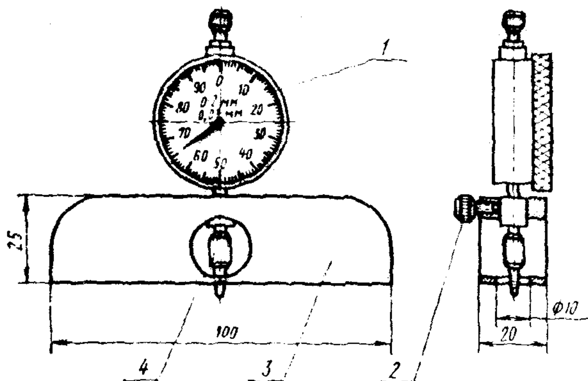
1—индикатор; 2—винт; 3—колотка; 4—наконечник индикатора.
