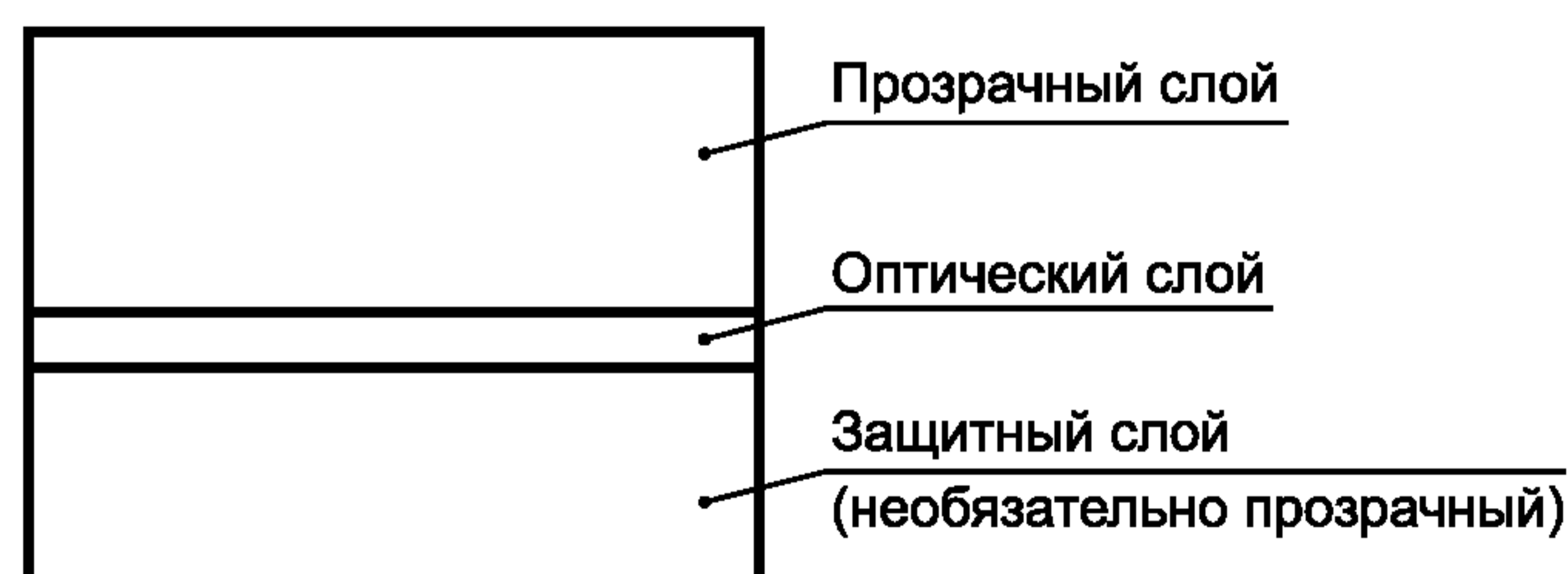
Рисунок 1 — Поперечное сечение карты в оптической зоне
