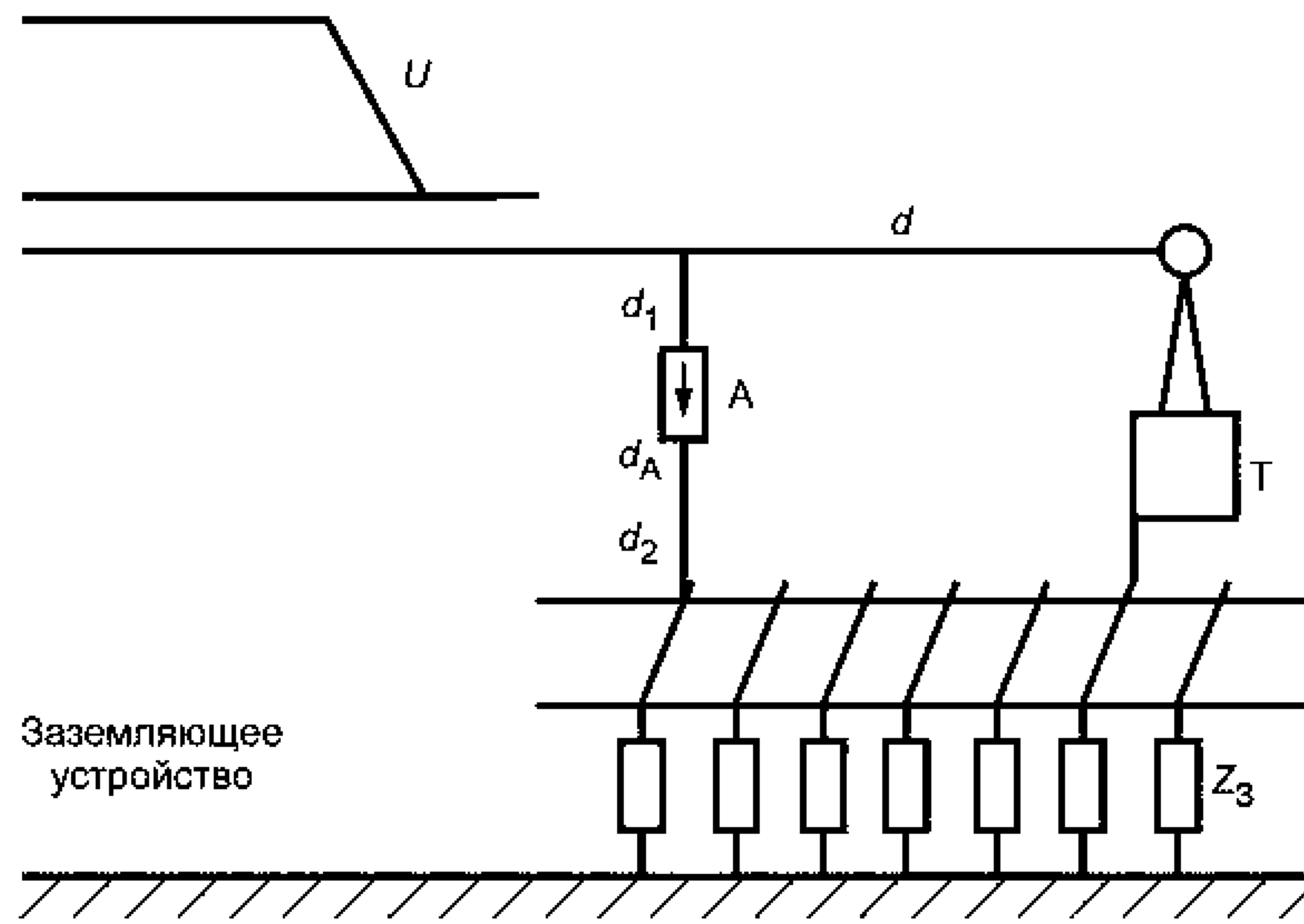
Рисунок 2б — Установки с контуром заземления (подстанции)
