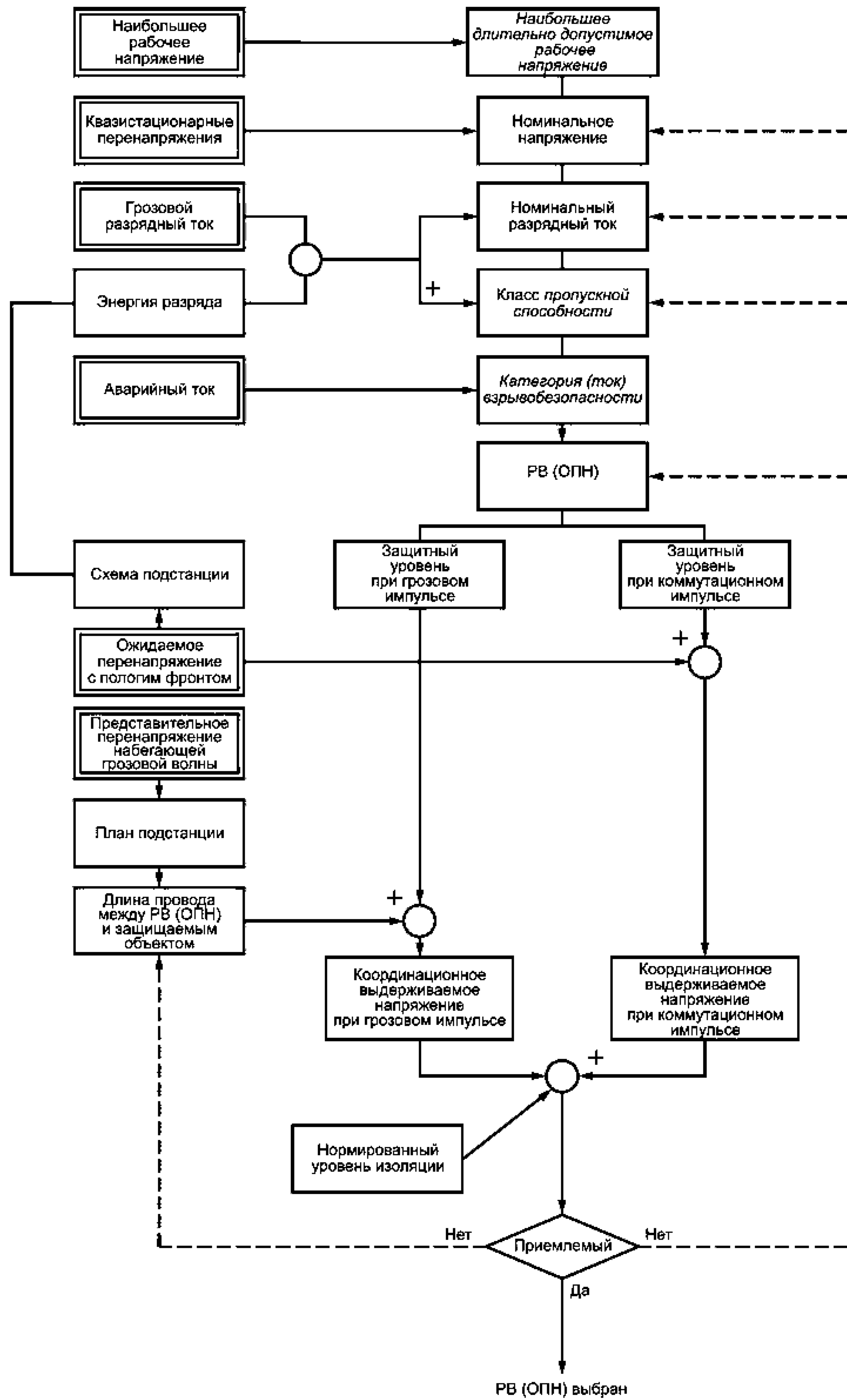
Рисунок 1 — Структурная схема выбора РВ (ОПН)
