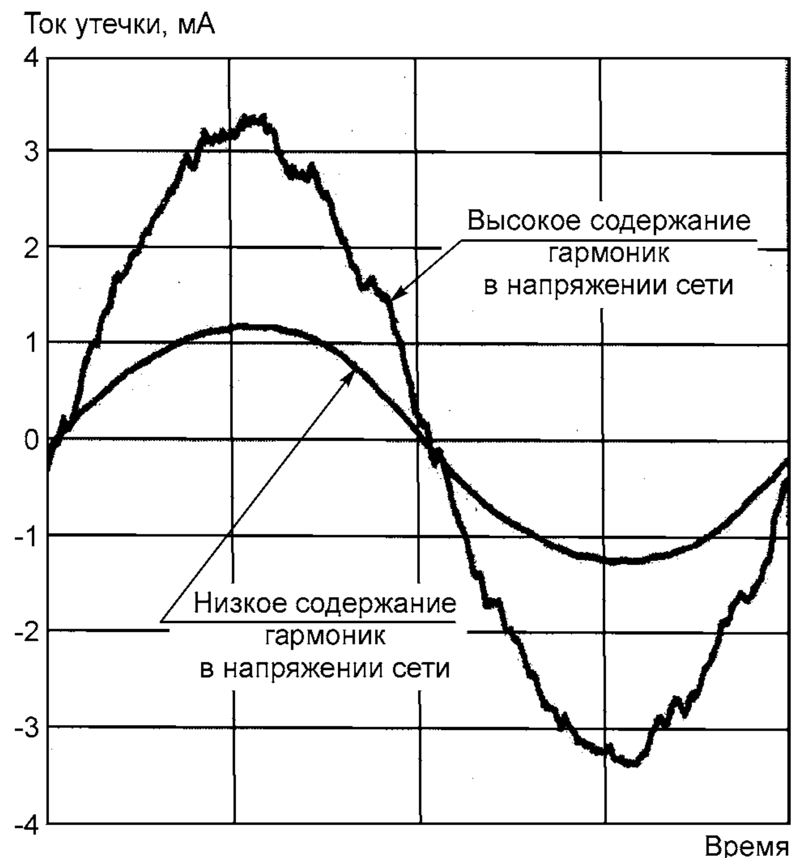
Рисунок 4 — Типичный ток утечки ОПН в условиях эксплуатации
