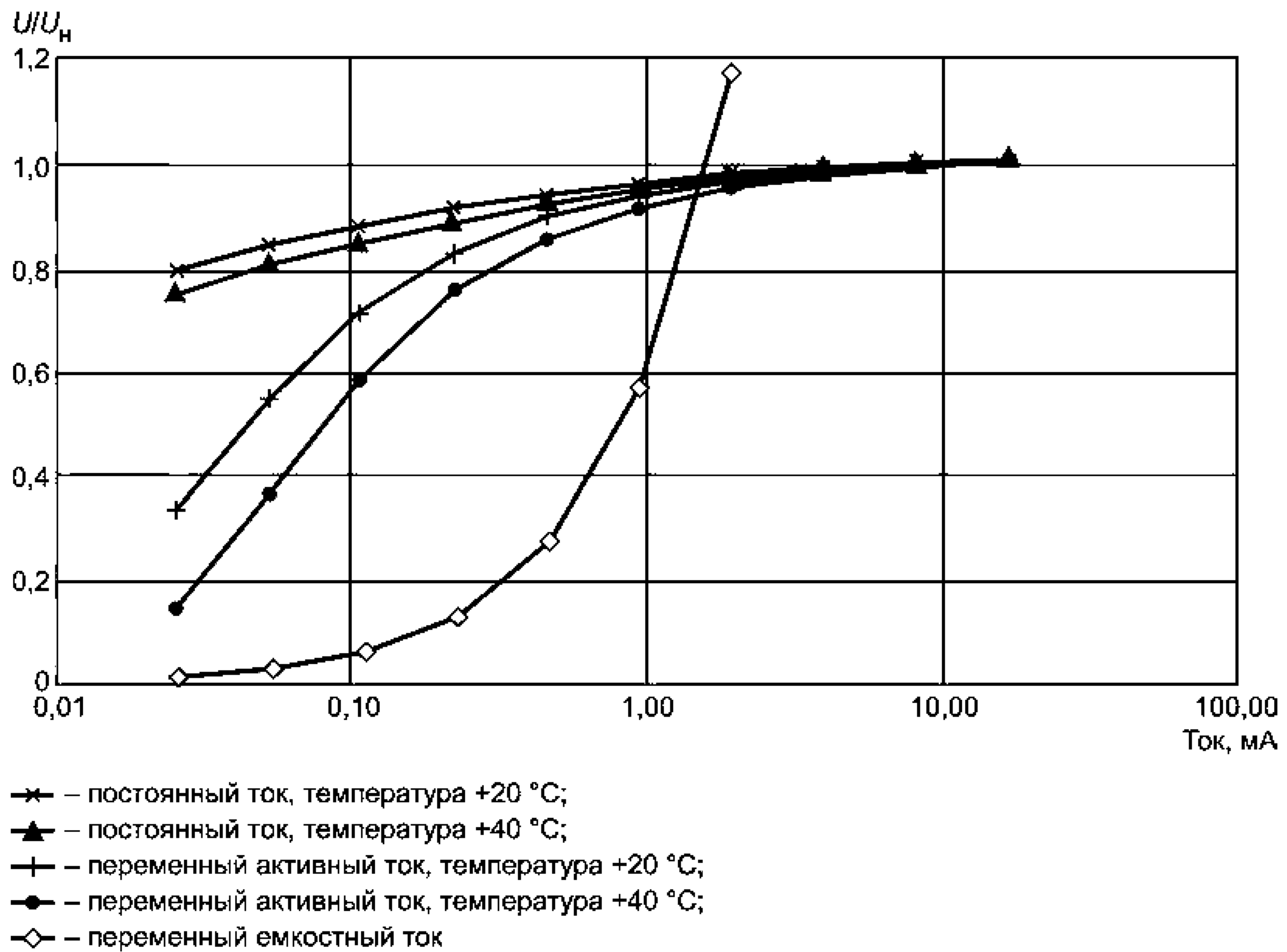
Рисунок 5 — Типичные вольтамперные характеристики нелинейных металлооксидных резисторов
