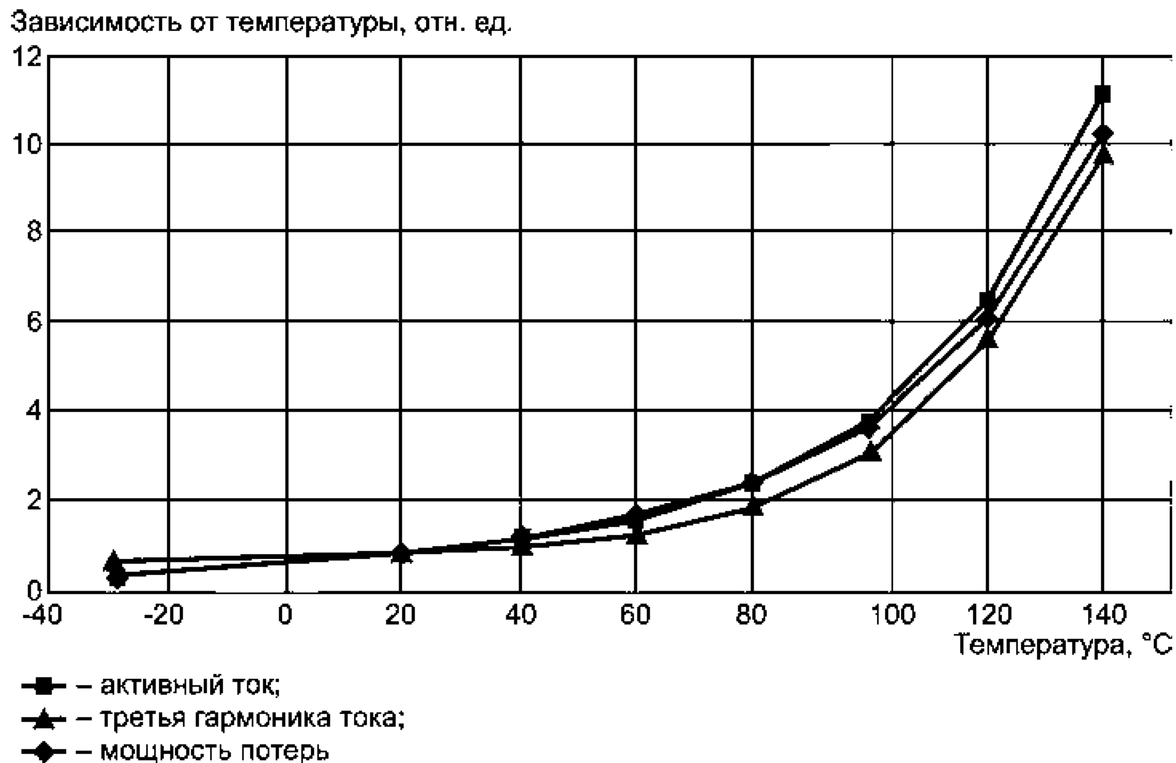
Рисунок 7 — Типичная нормализованная зависимость от температуры при наибольшем длительно допустимом рабочем напряжении U_{нр}
