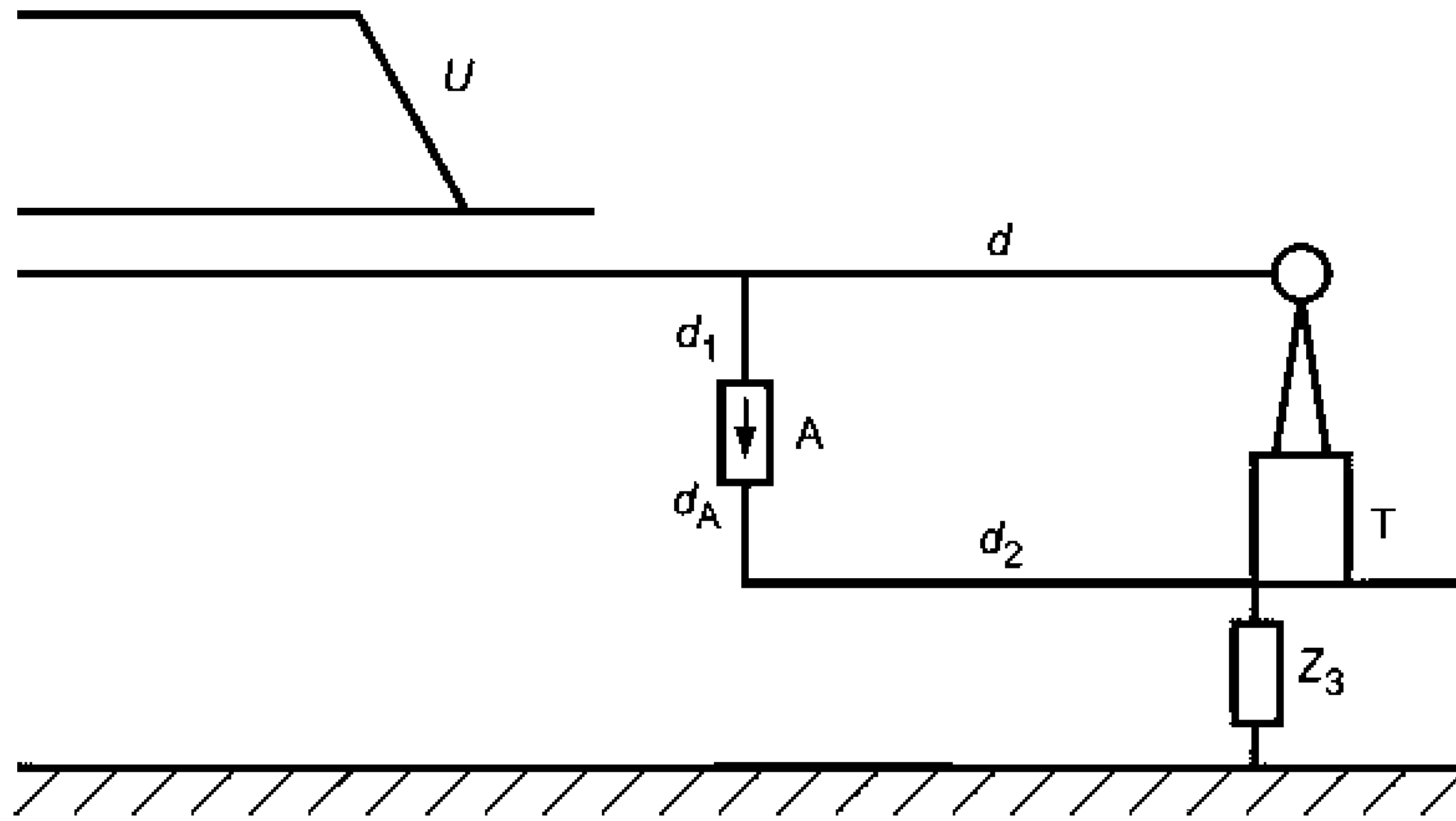
Рисунок 2а — Установки без контура заземления (распределительные сети)
