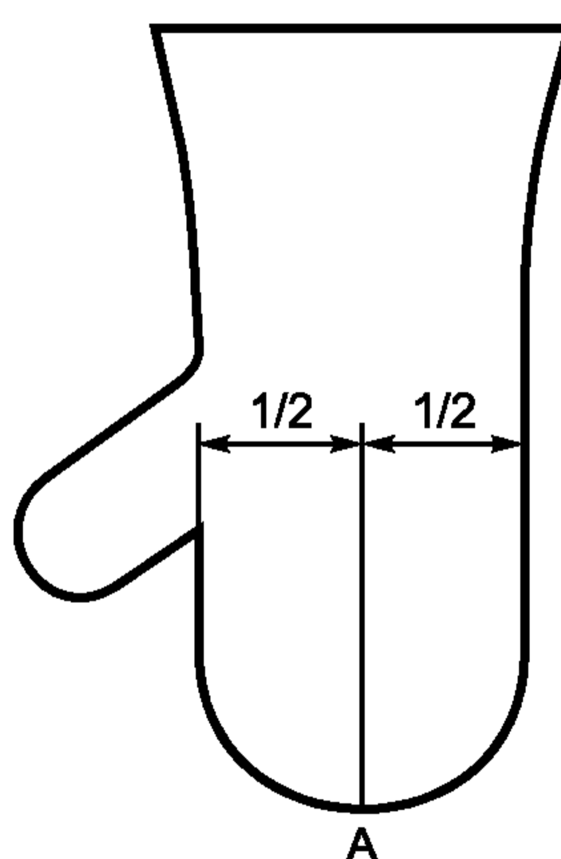
Рисунок 1 — Подвешивание перчатки для испытания
