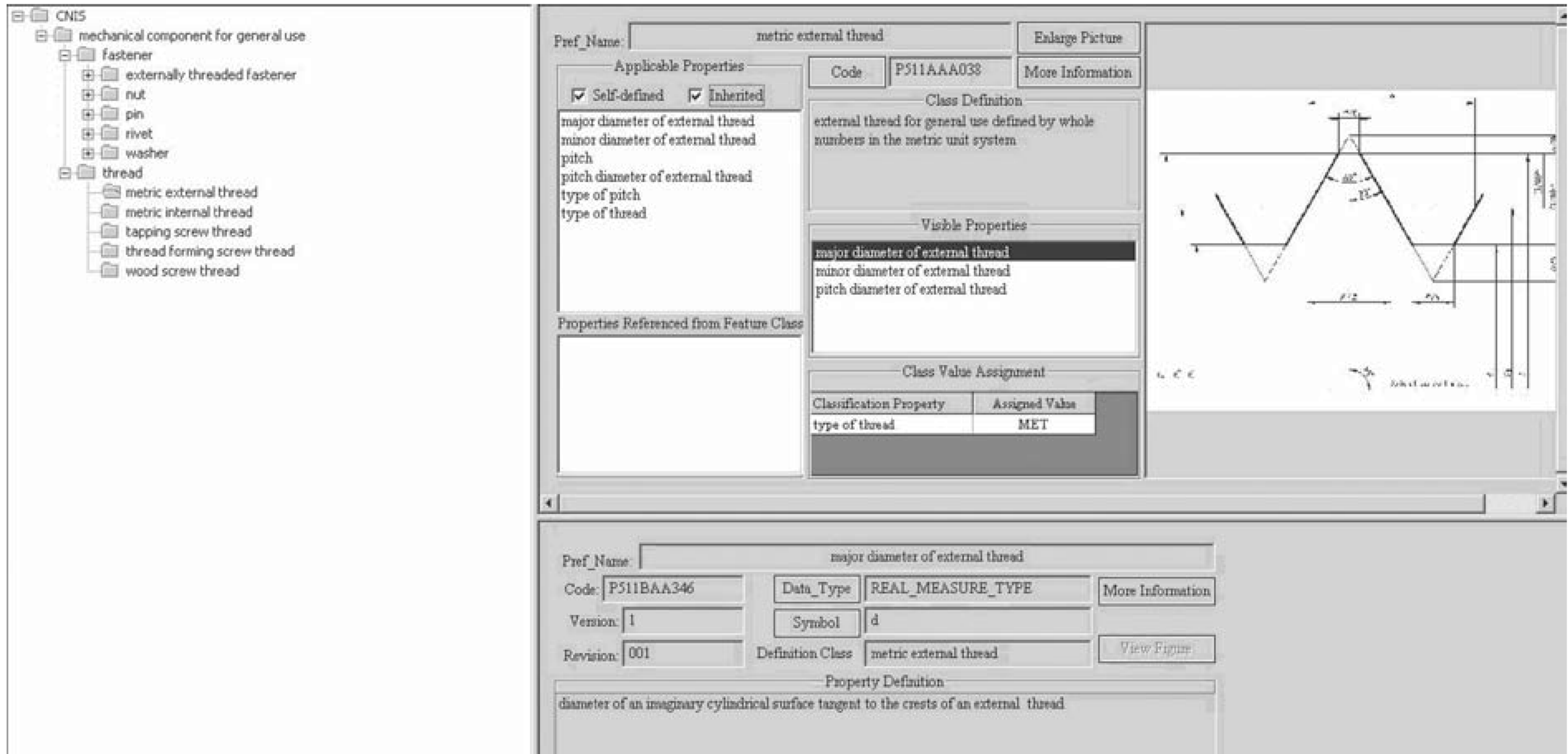
Рисунок 4 — Характеристический класс резьб по ИСО 13584-511
