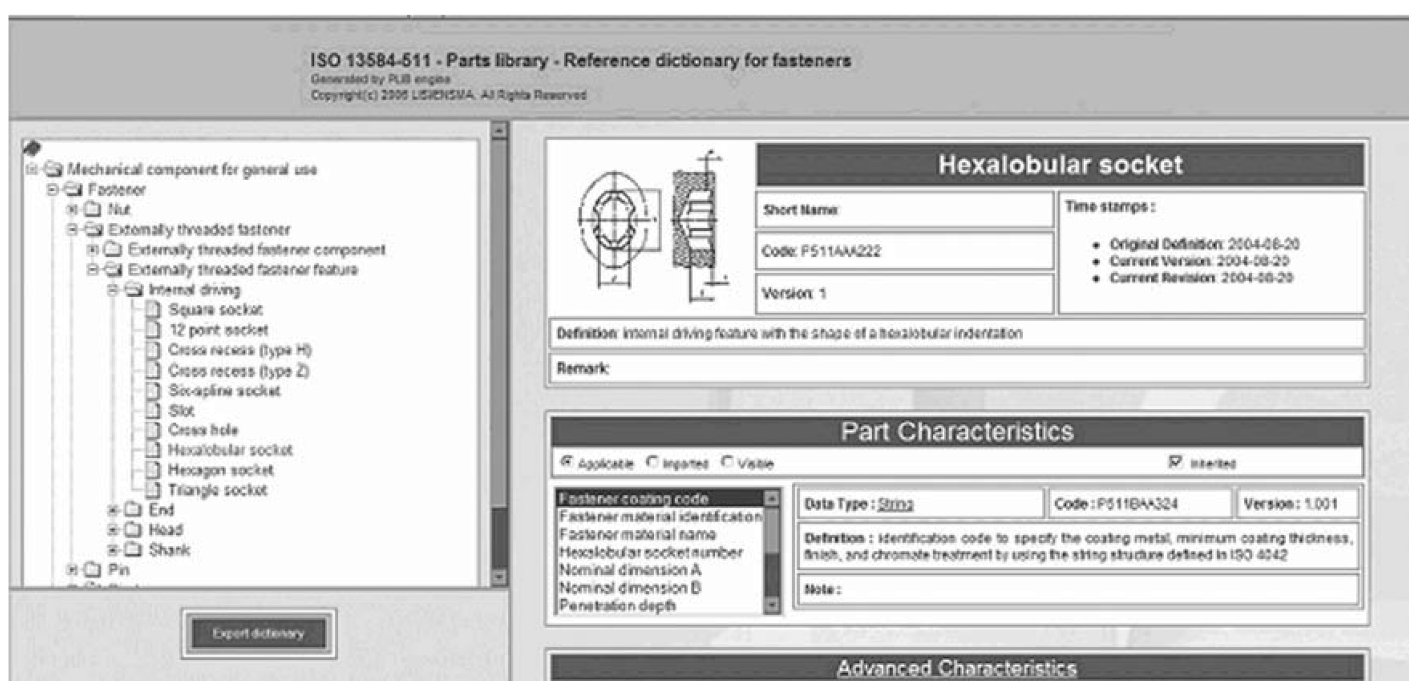
Рисунок 7 — Использование параметрического моделирования согласно ИСО 13584-511
