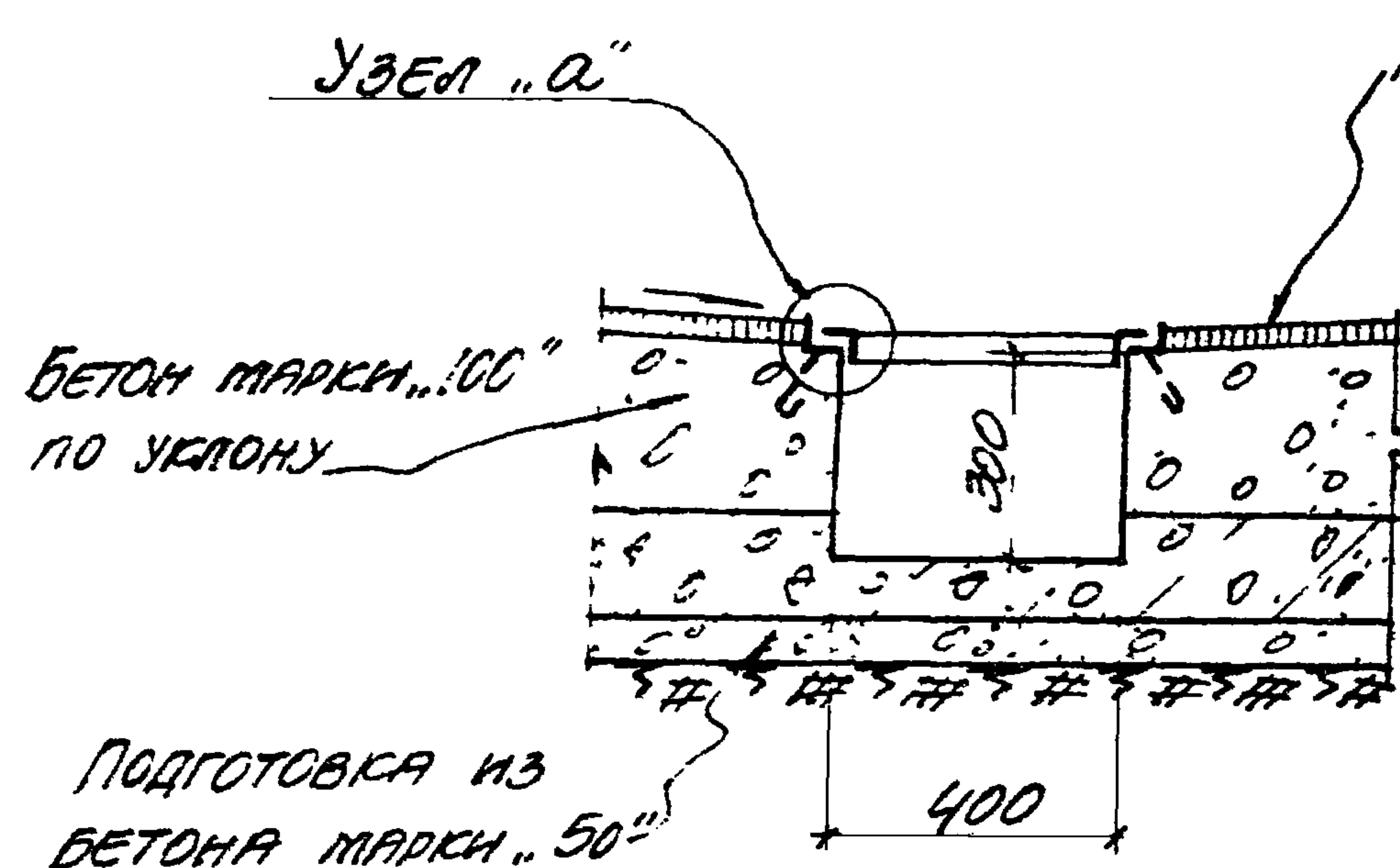
По А-А
