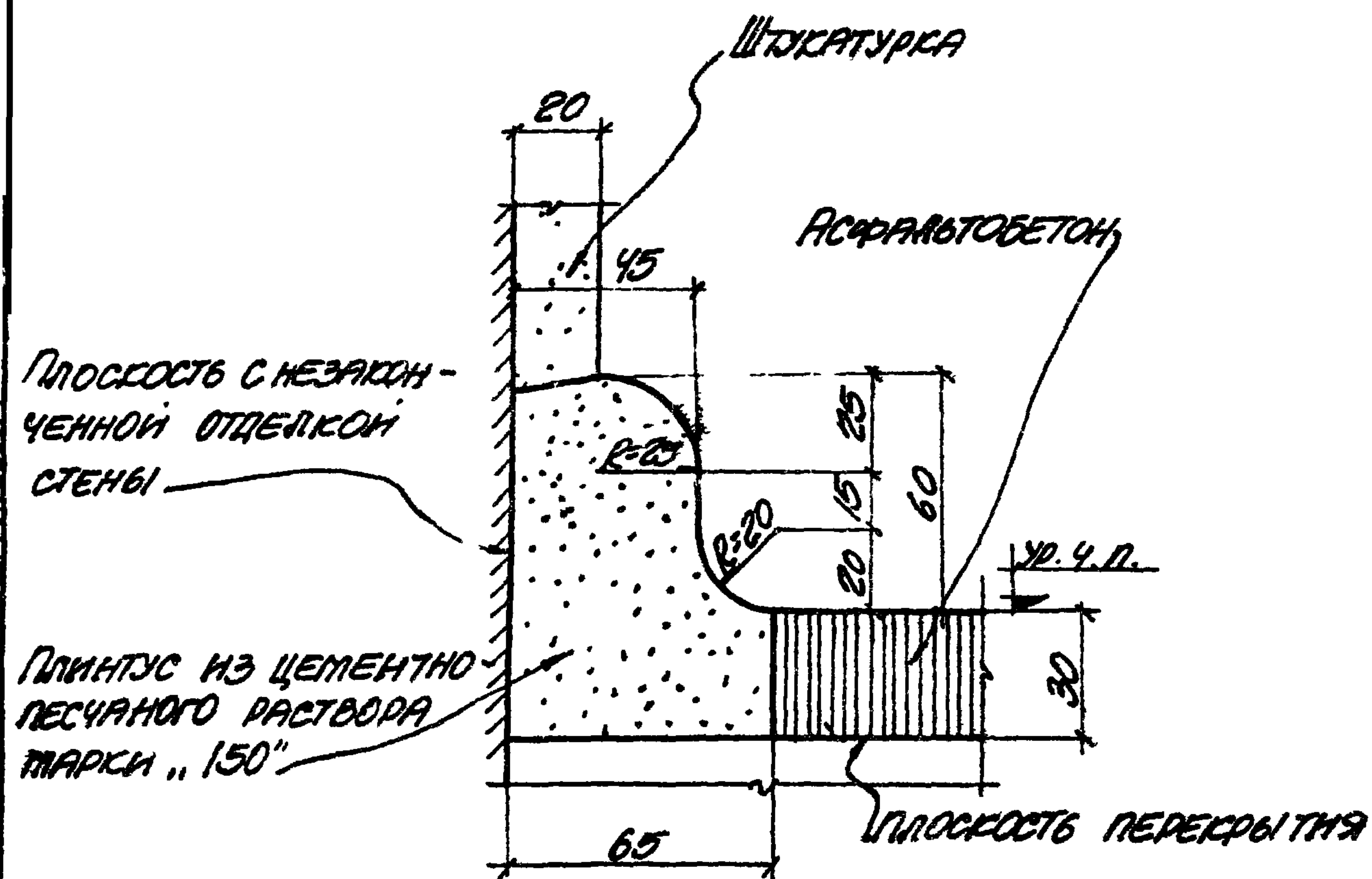
Деталь плинтуса
