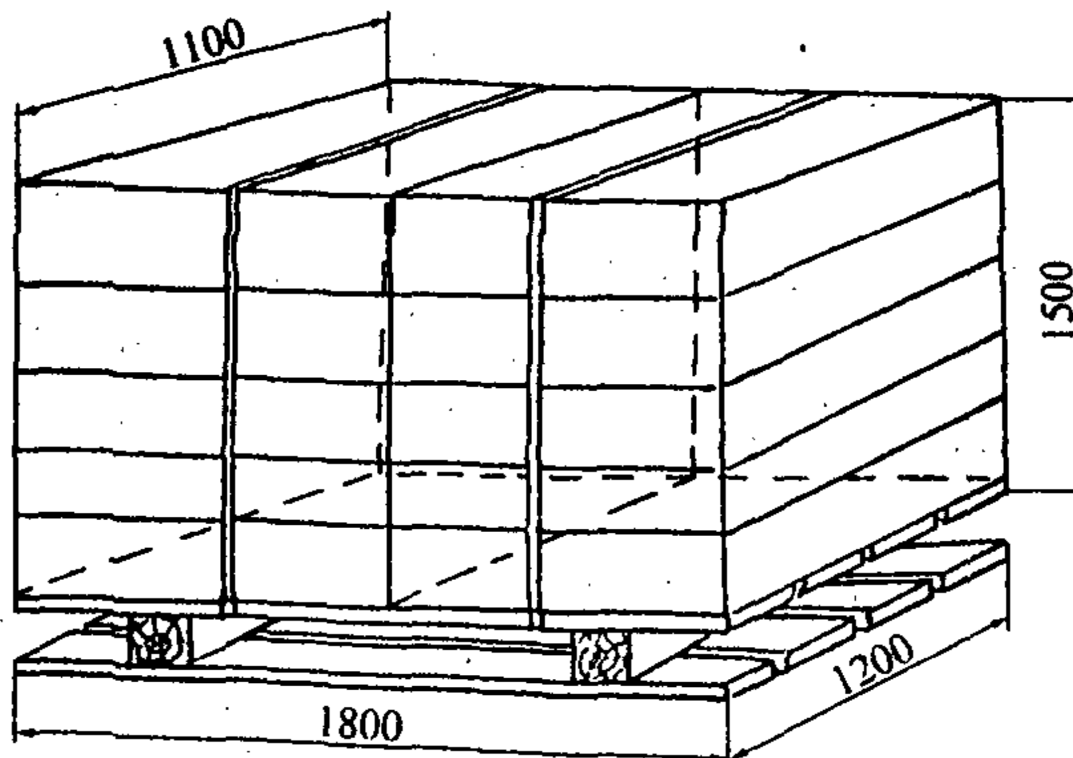
Рис. 7.3.4. Схема формирования пакета №4
