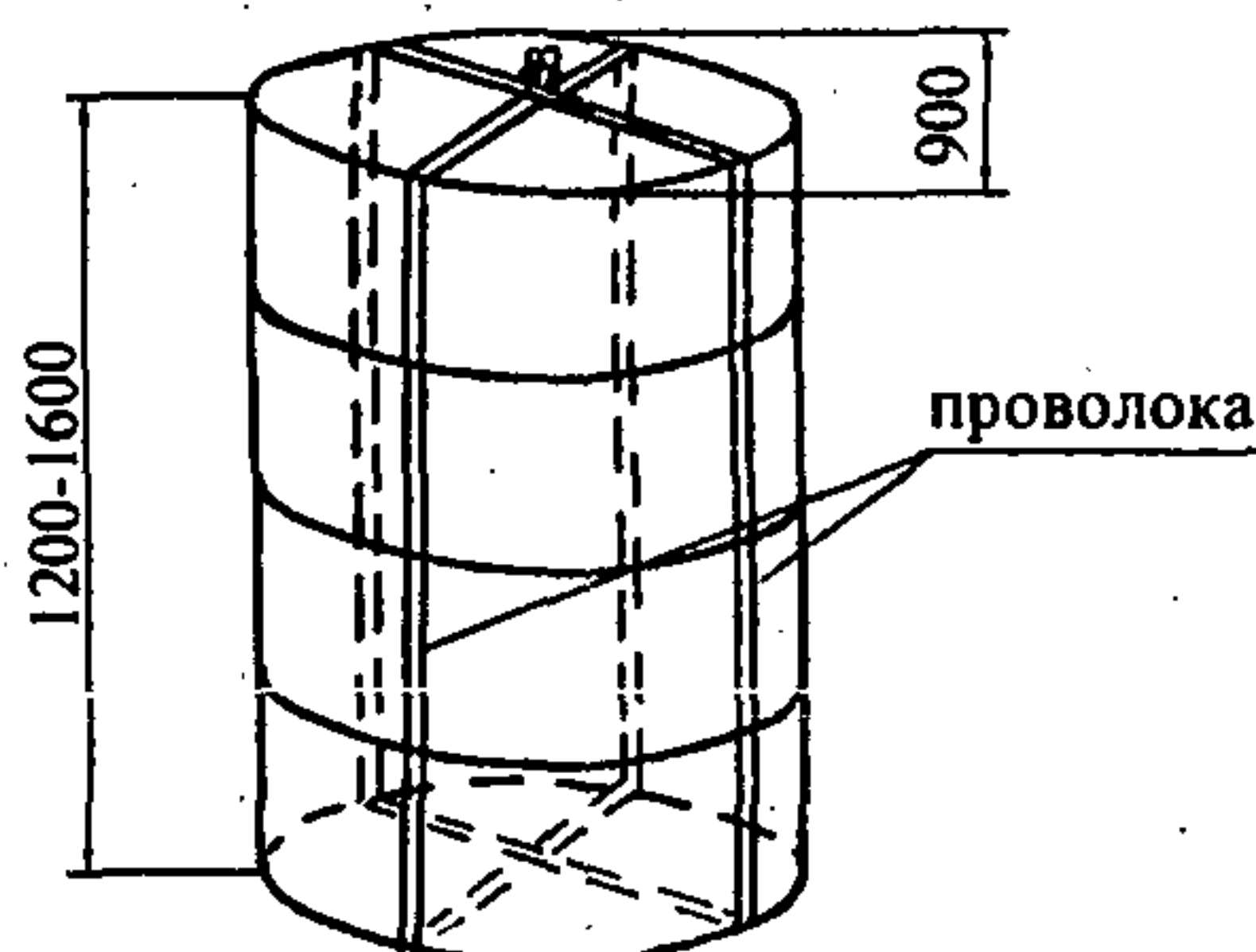
Рис. 7.3.1. Схема формирования пакета №1
