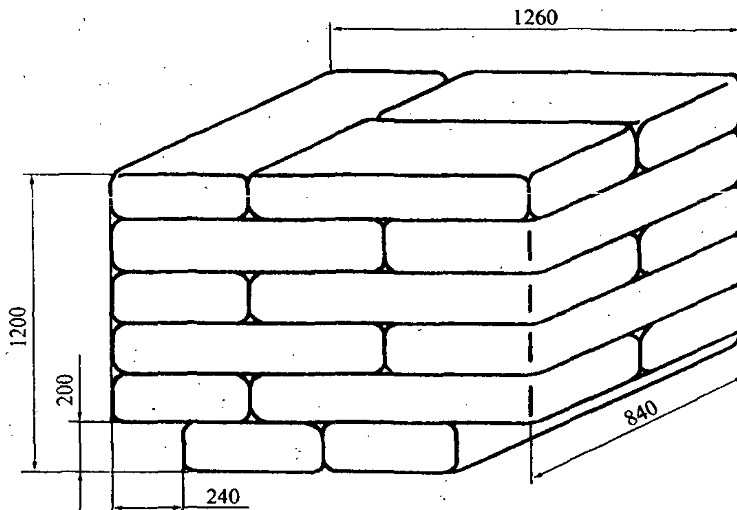
Рис. 7.2.1. Схема укладки мешков в пакете
