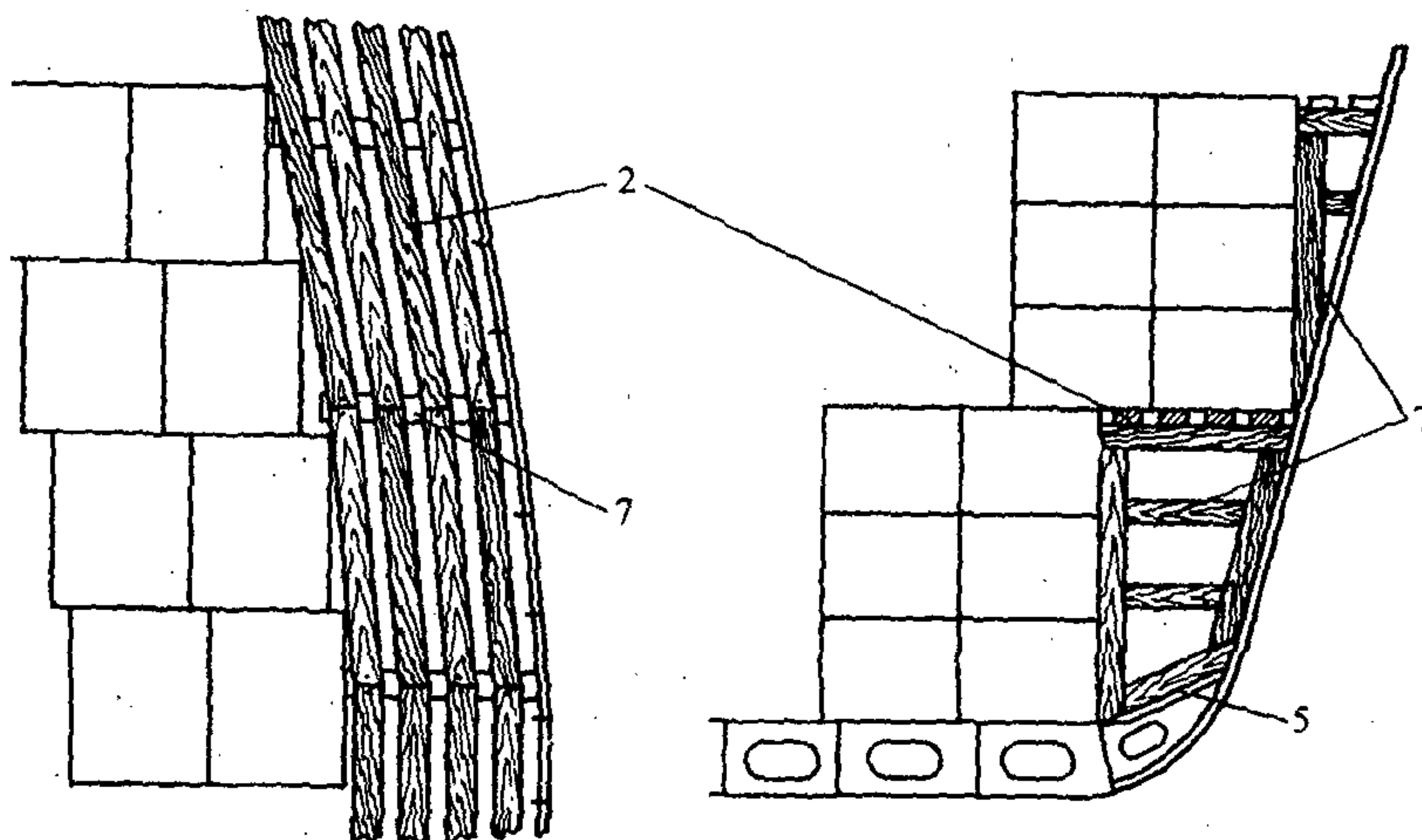
Рис. П.5.2. Конструкции бортовых выгородок:
