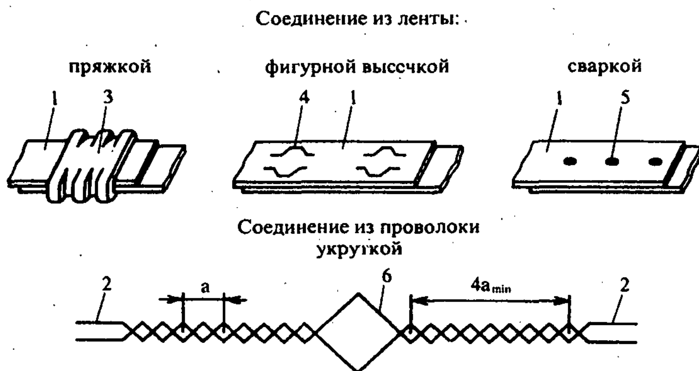
Рис. П.4.2. Соединение концов обвязок:
