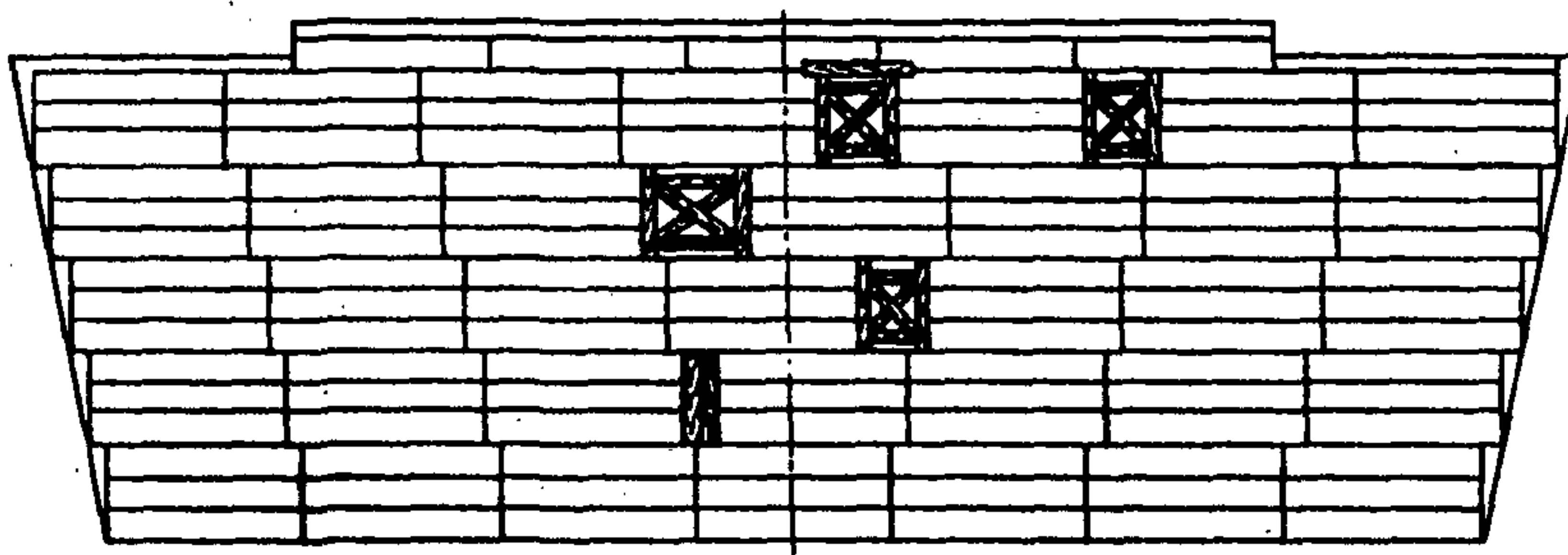
Рис. 7.5.1. Раскрепление пустот между пакетами клетками из брусьев
