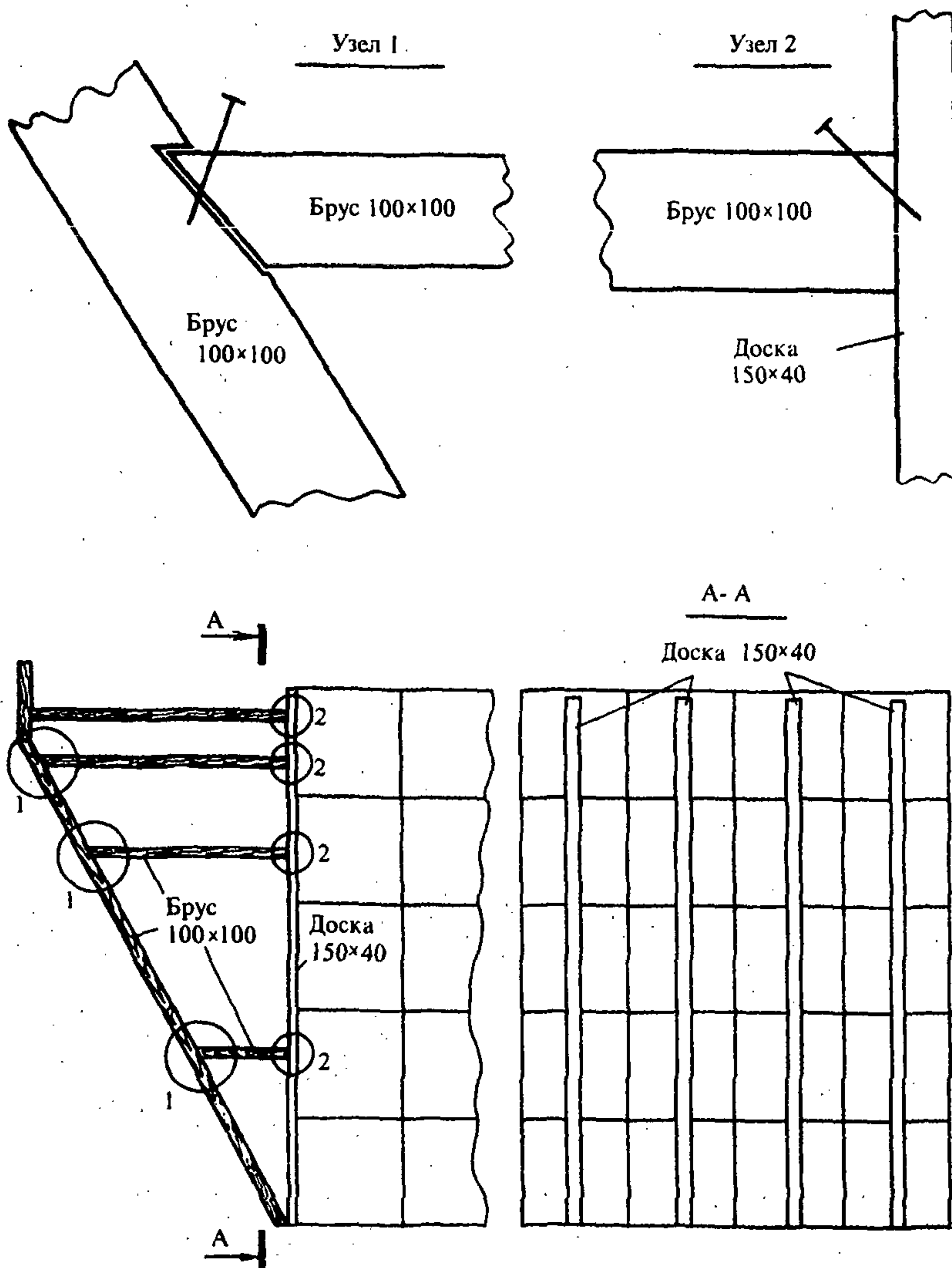
Рис. 7.1.3. Схема устройства опорных конструкций
