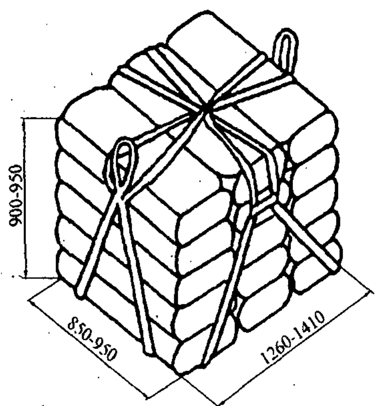
Рис. 7.4.2. Схема формирования строп-пакета типа СПК-1,05t-2,9
