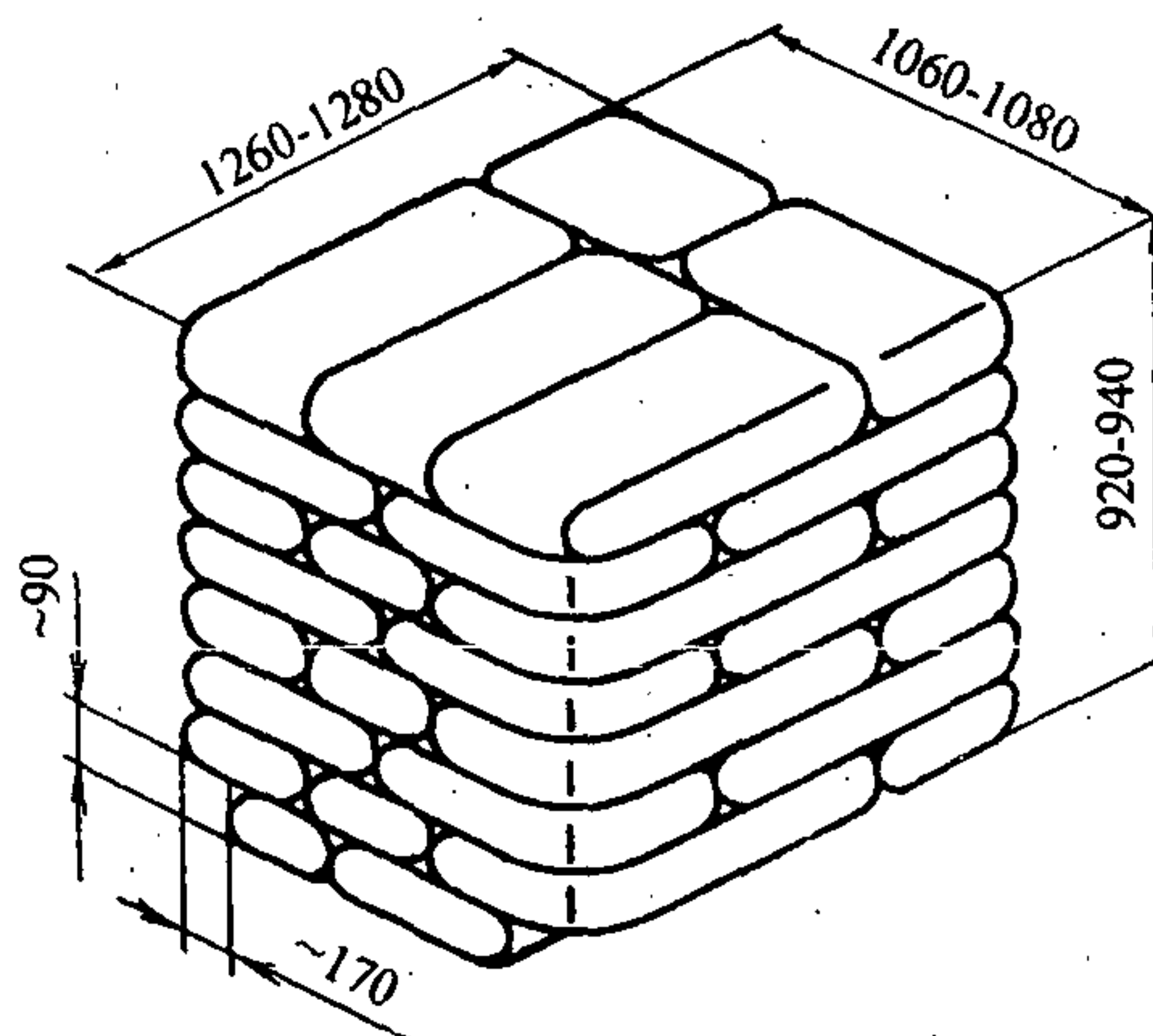
Рис. 7.1.1. Общий вид пакета цемента
