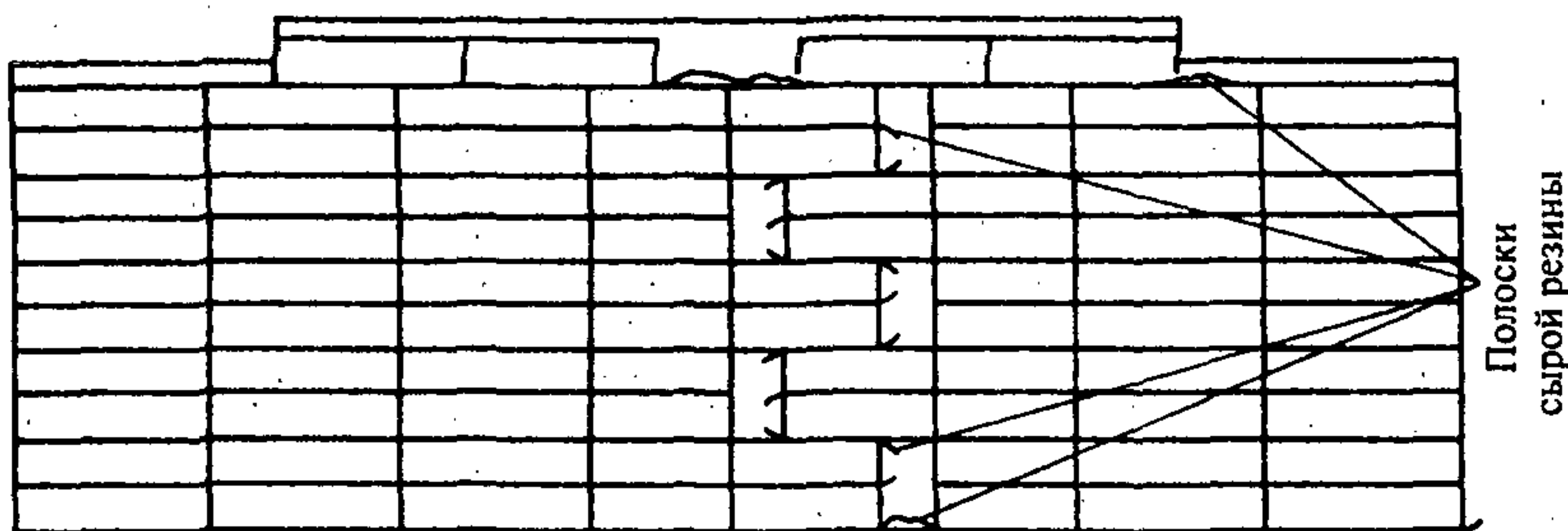
Рис. 7.5.2. Крепление полосками сырой резины
