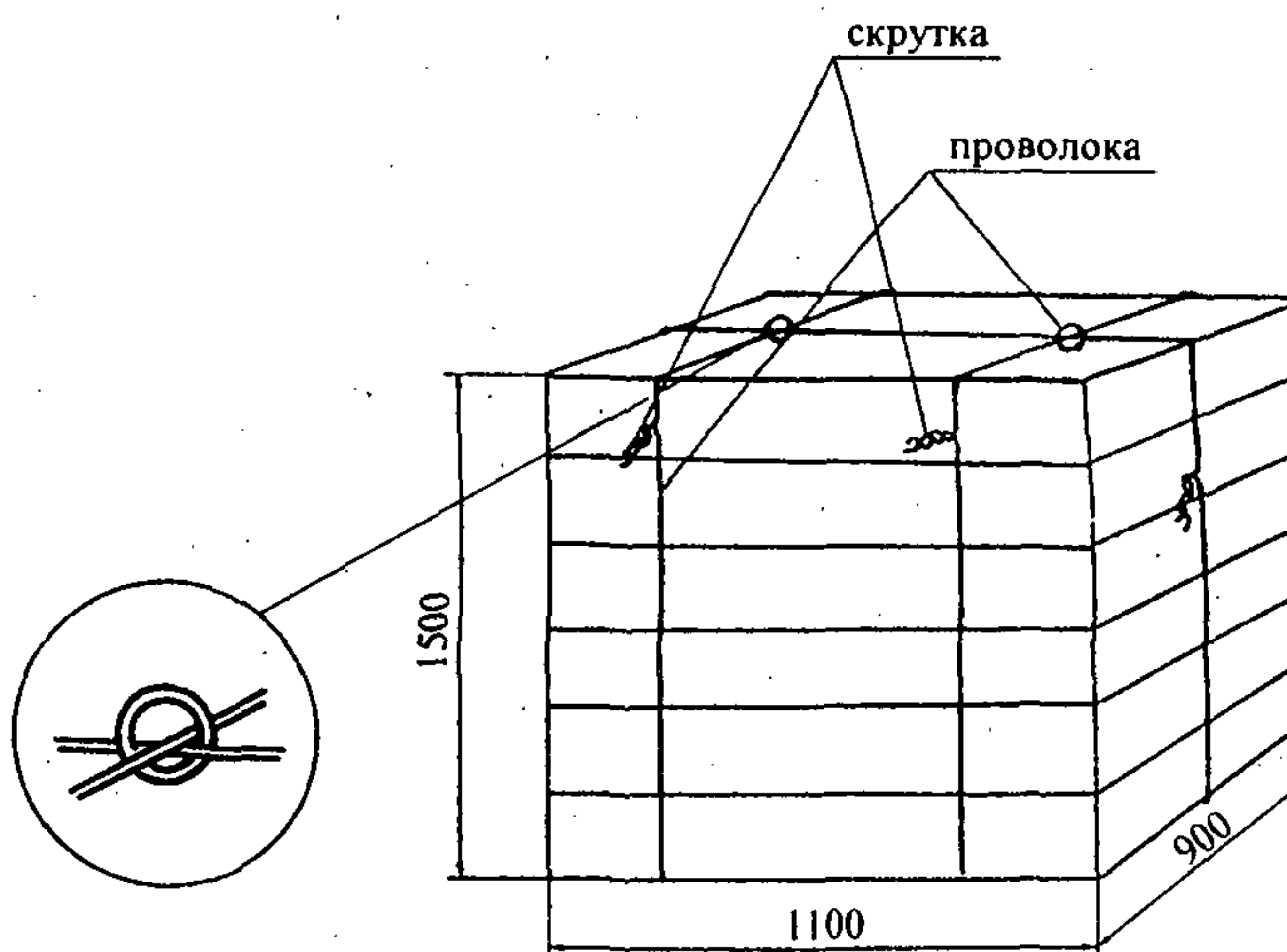
Рис. 7.3.2. Схема формирования пакета №2
