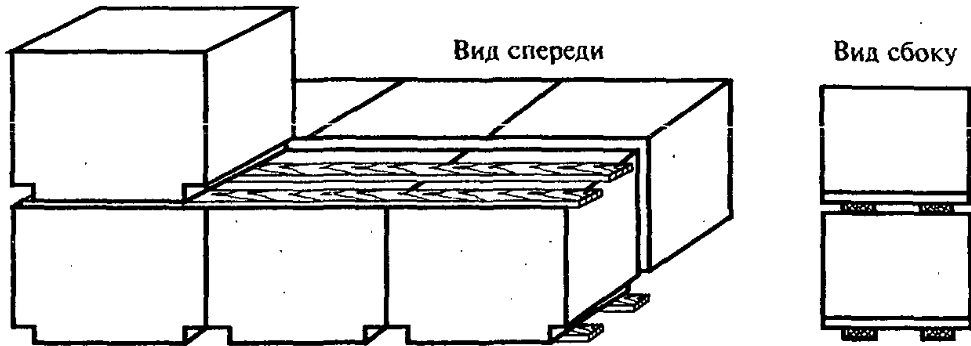
Рис. 7.1.4. Размещение прокладок вдоль длинной стороны пакетов
