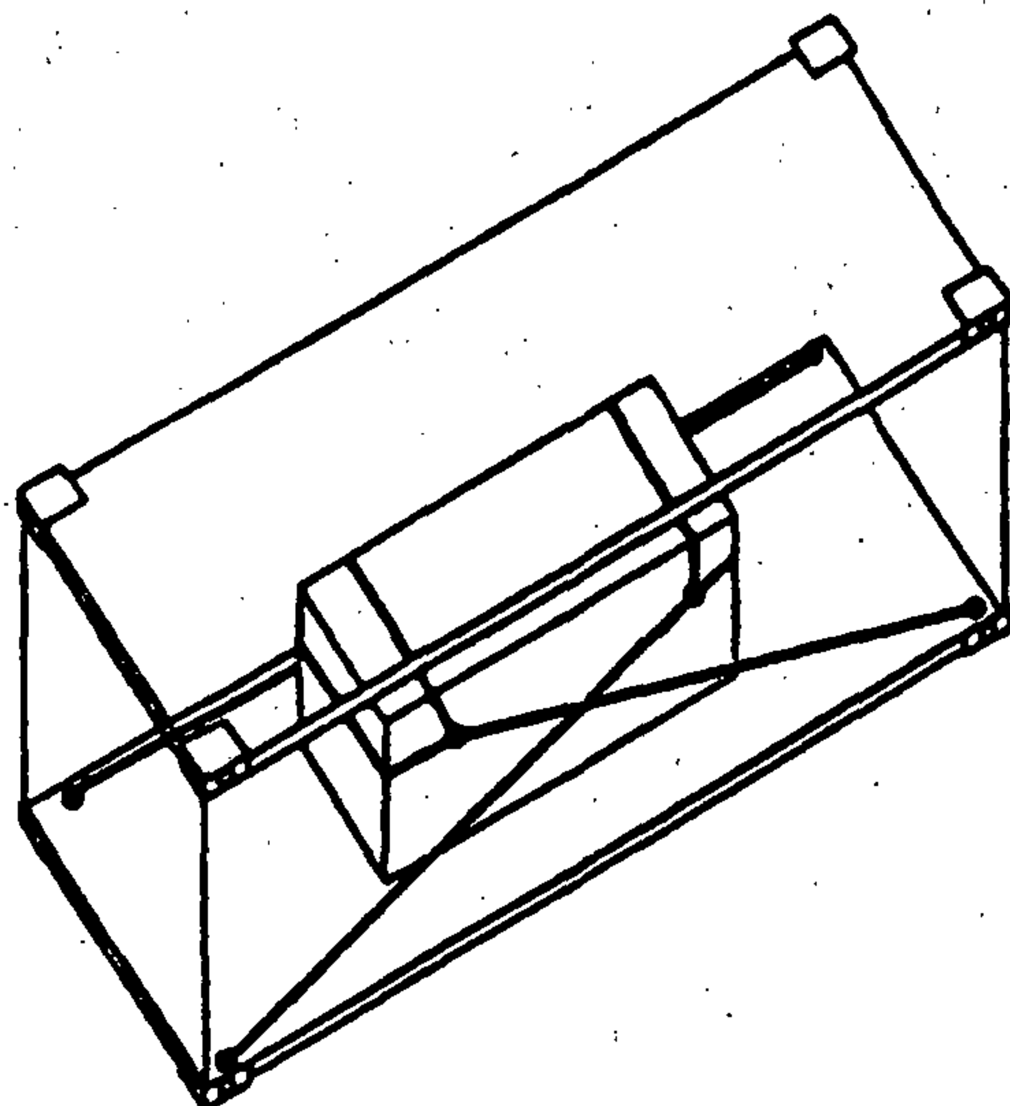
Правильное крепление тяжелых единичных грузовых мест
