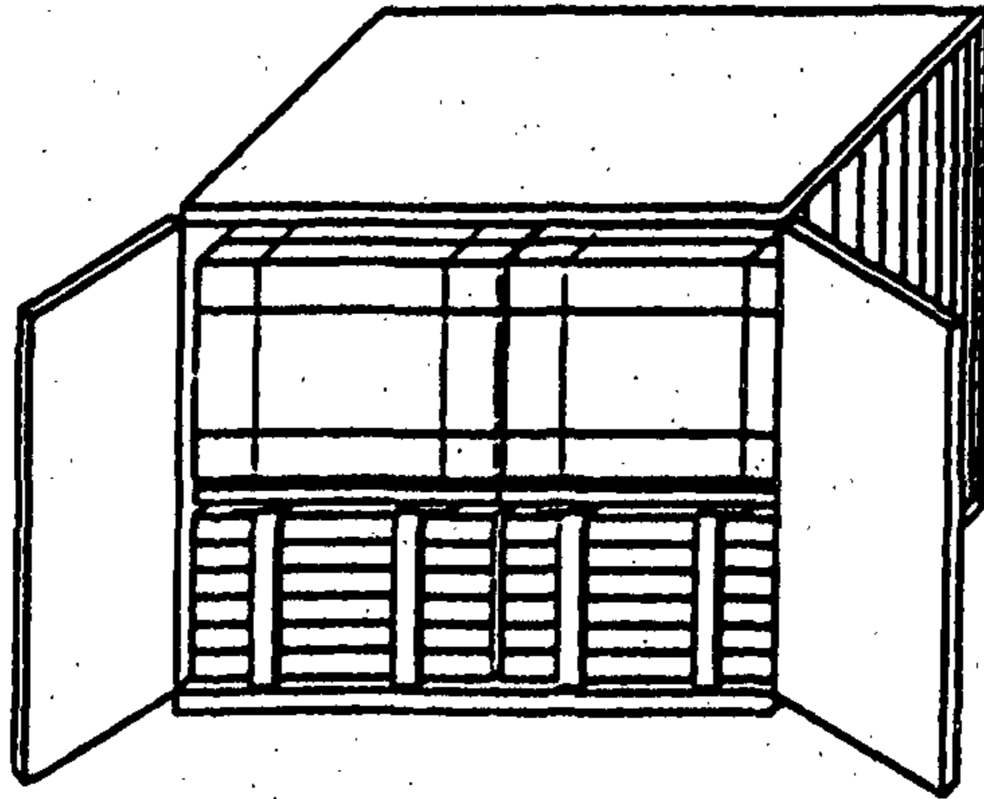
Крепление груза при помощи промежуточных настилов
