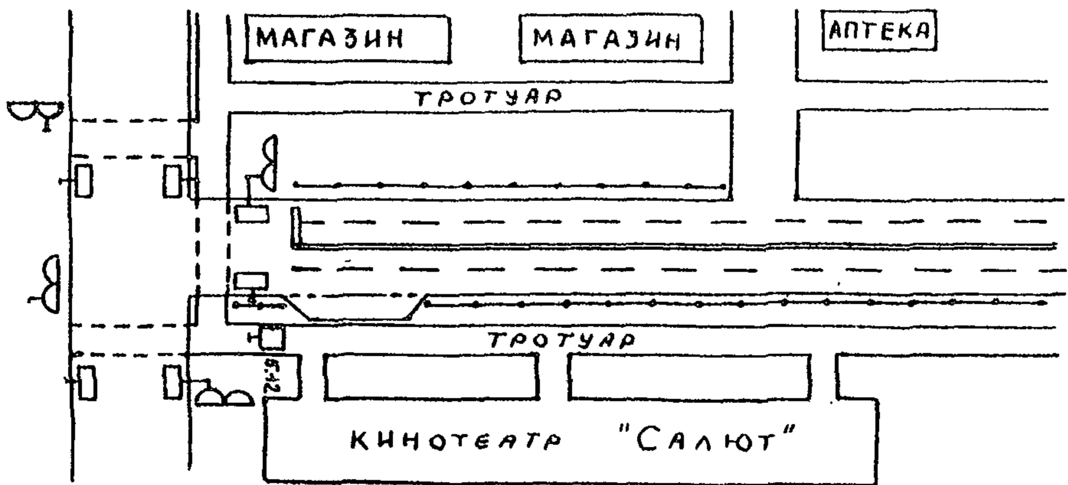
Рис. П5.4. Предлагаемая схема организации движения.
