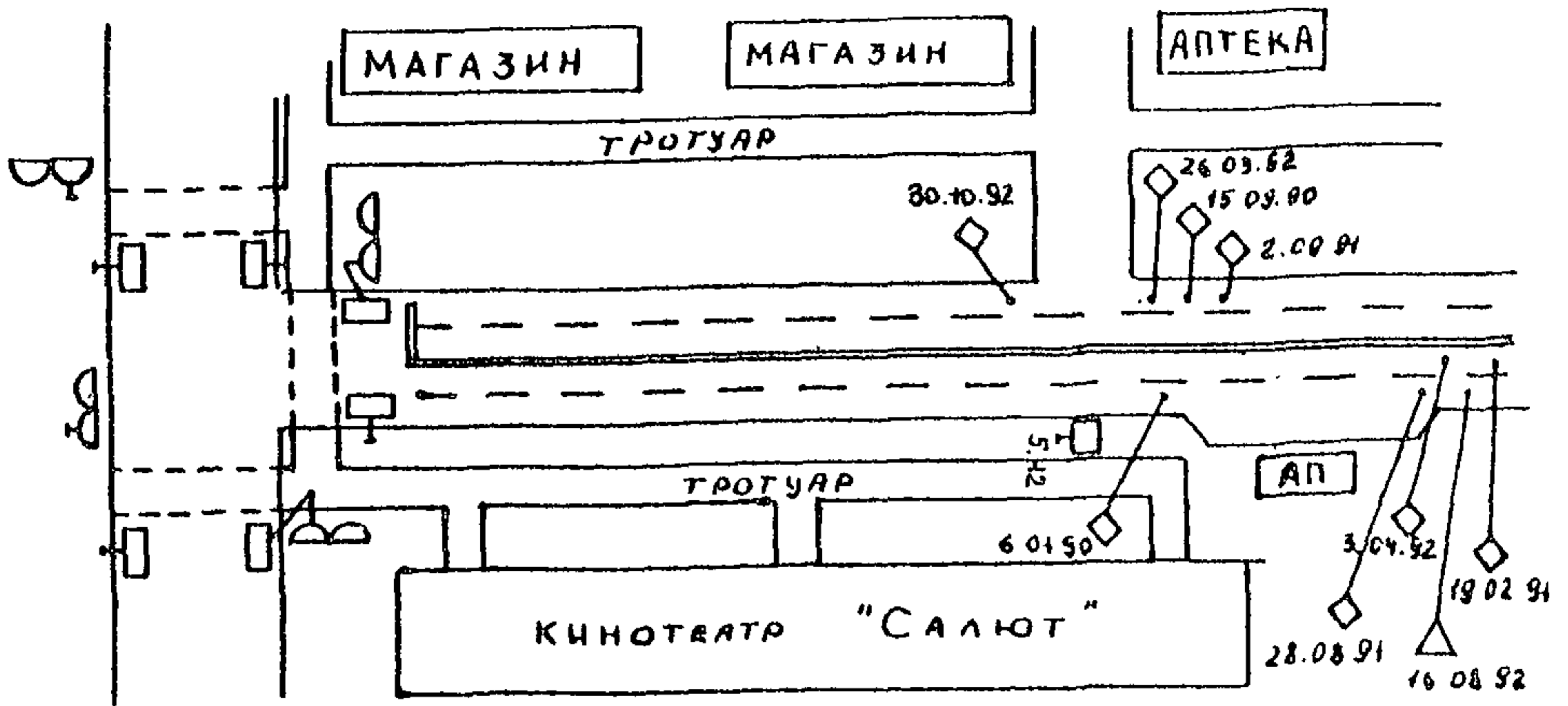
Рис. П5.3. Существующая схема организации движения.
