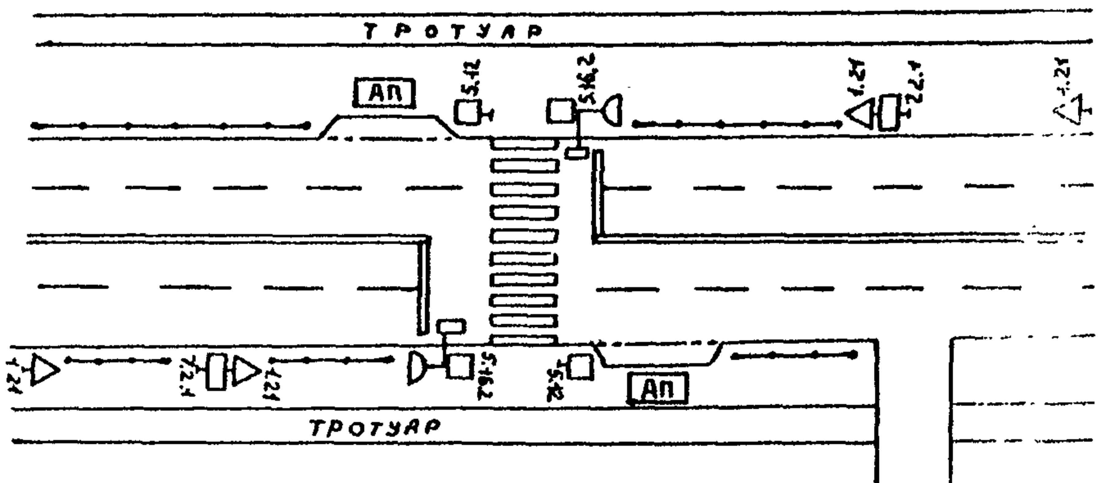
Рис. П5.6. Предлагаемая схема организации движения.
