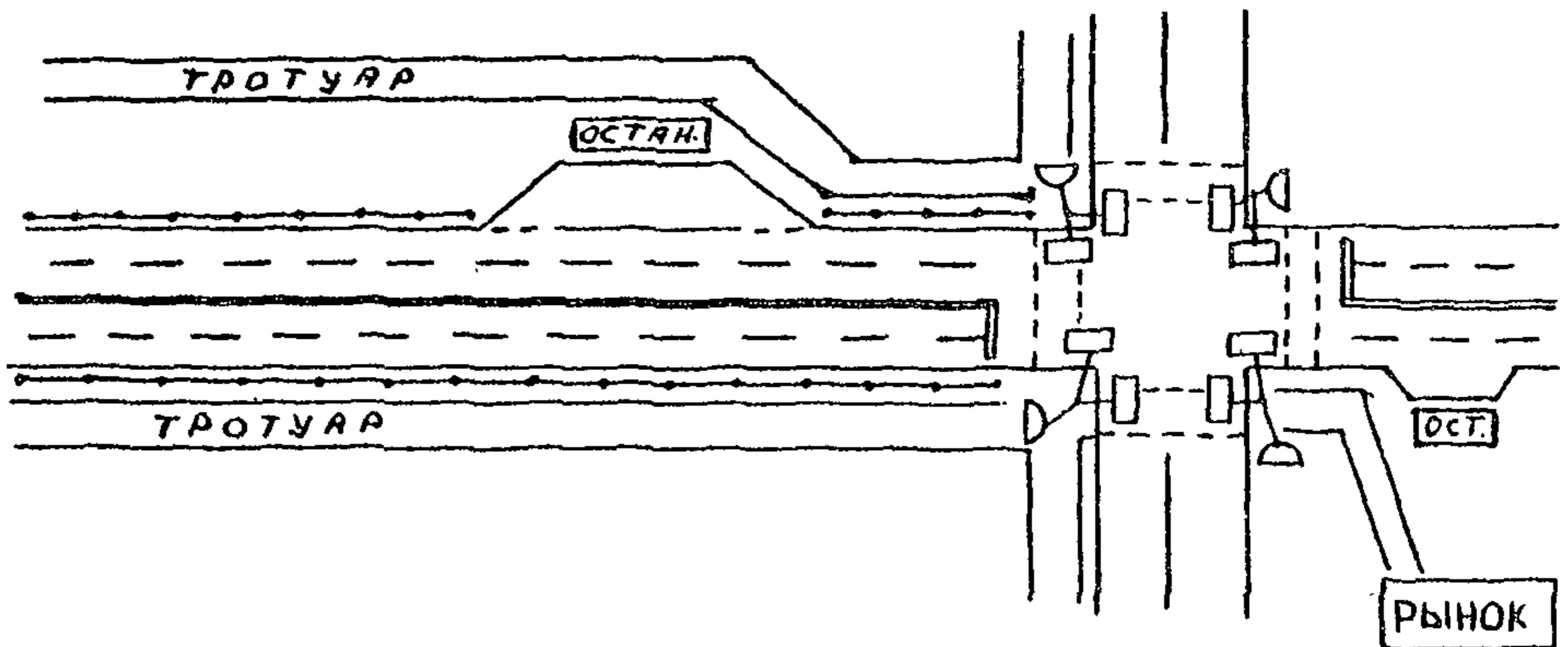
Рис. П5.8. Предлагаемая схема организации движения.
