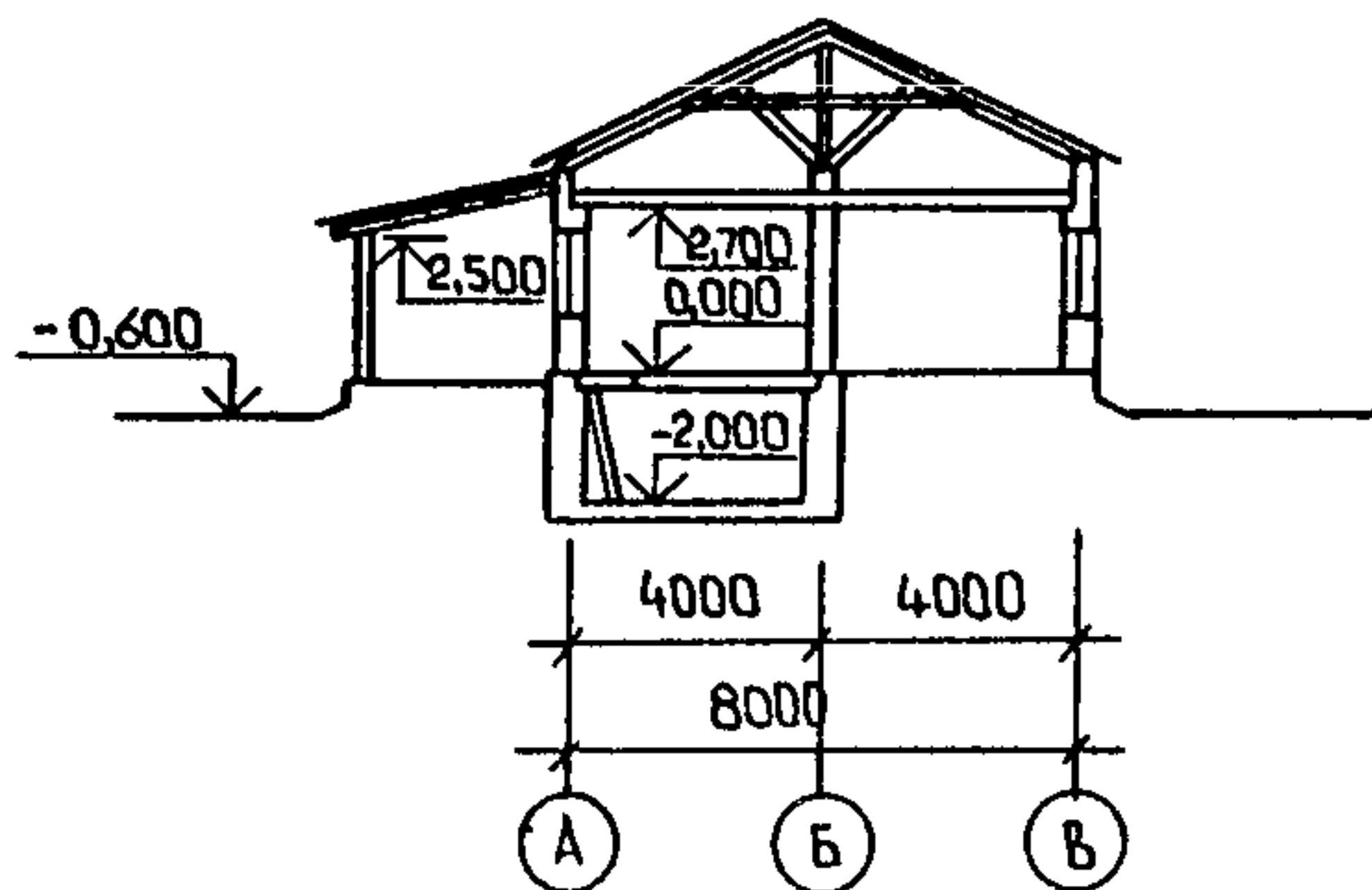
Рис. В.1. Пасечный дом с хозяйственным блоком на 100 пчелиных семей (ТП 808-5-48.92):
