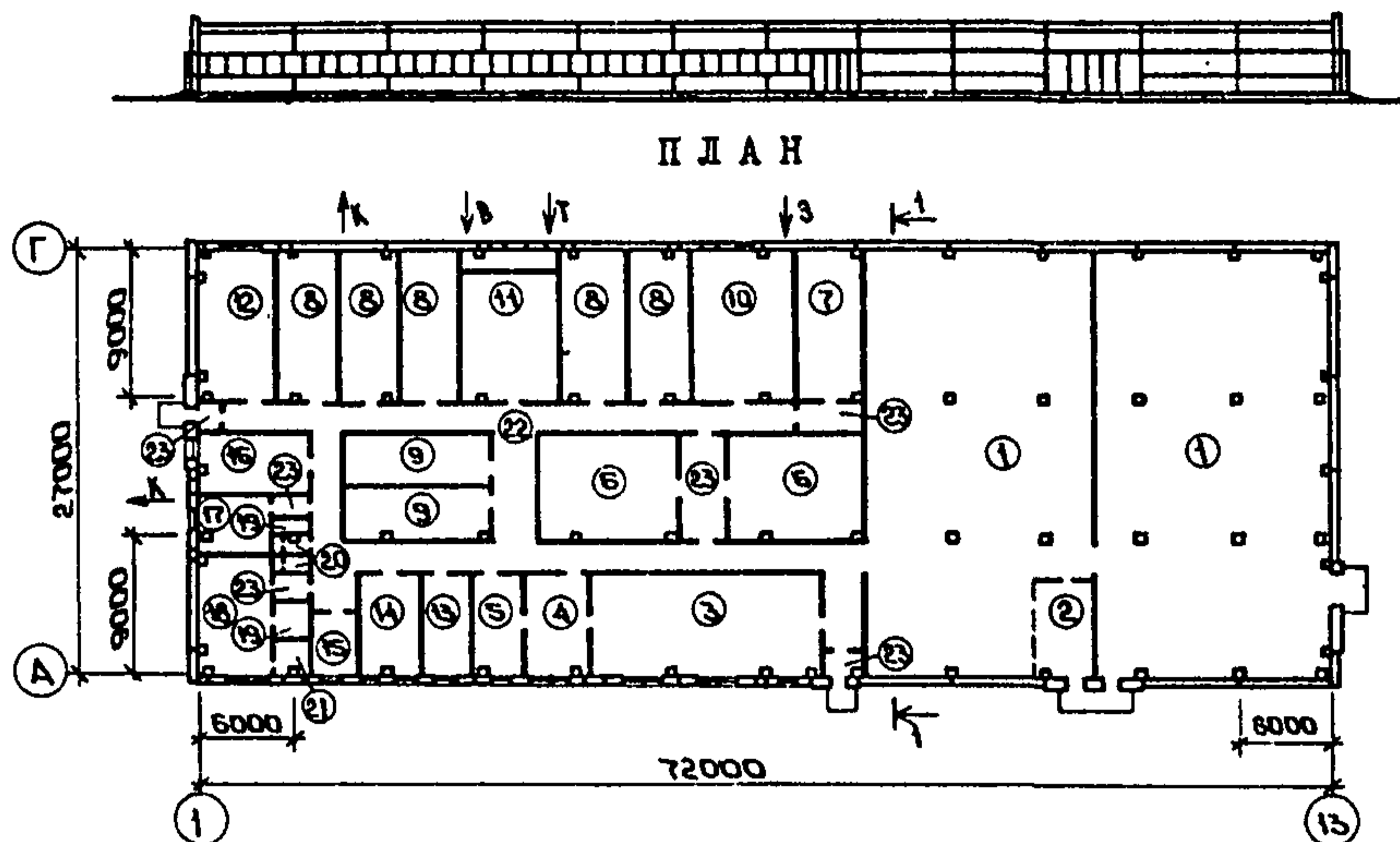
Рис. Г.5. Производственный корпус цеха по содержанию и разведению пчел-листорезов (ТП 808-5-17.86): 1-помещение для дозаривания коконов вместимостью на 12500 ульев; 2-участок разборки ульев; 3-помещение вычесывания коконов; 4-помещение сортировки коконов; 5-помещение взвешивания и затаривания коконов в коробки; 6-холодильная камера на 40 млн коконов; 7-холодильная камера на 20 млн коконов; 8-инкубатор на 10 млн коконов; 9-инкубатор на 5 млн коконов; 10- машинный зал с электрощитовой; 11- венткамера; 12-комната приема пищи; 13-лаборатория; 14-кабинет начальника цеха; 15- комната специалистов; 16-комната отдыха; 17-гардеробная женская; 18-гардеробная мужская; 19-душевая женская, мужская; 20-уборная женская и мужская; 21-помещение для хранения уборочного инвентаря; 22-коридор; 23-тамбур
