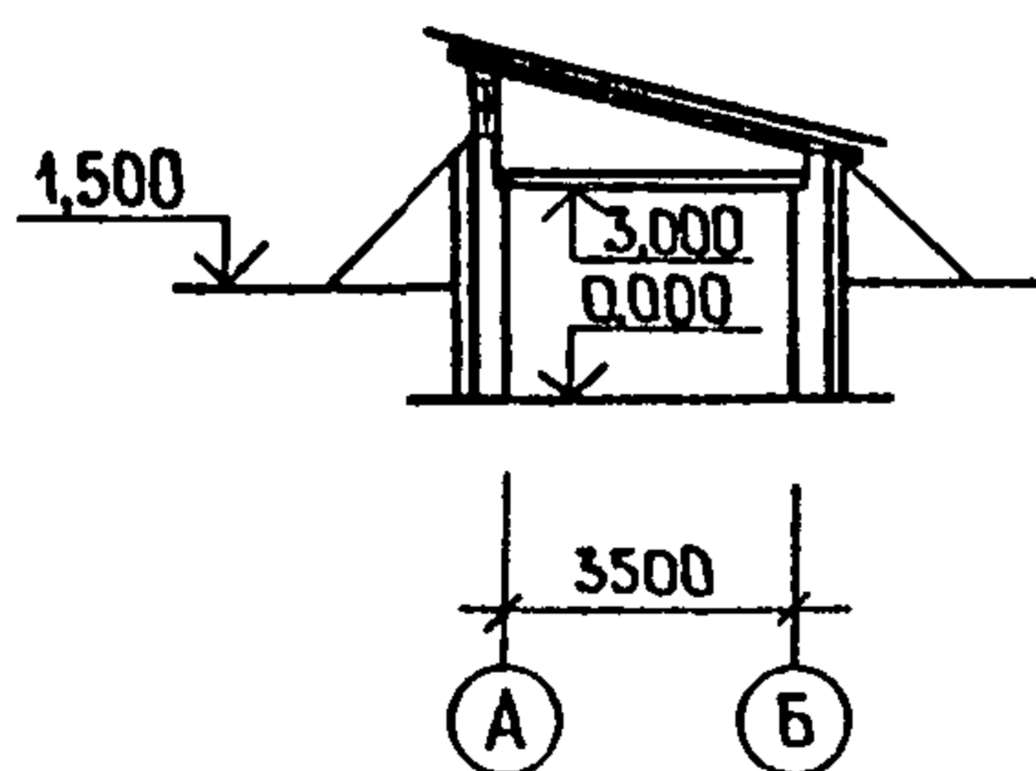
Рис. Д.1. Зимовник на 100 пчелиных семей (ТП 808-5-52.92) полузаглубленный: 1-помещение для ульев; 2-тамбур
