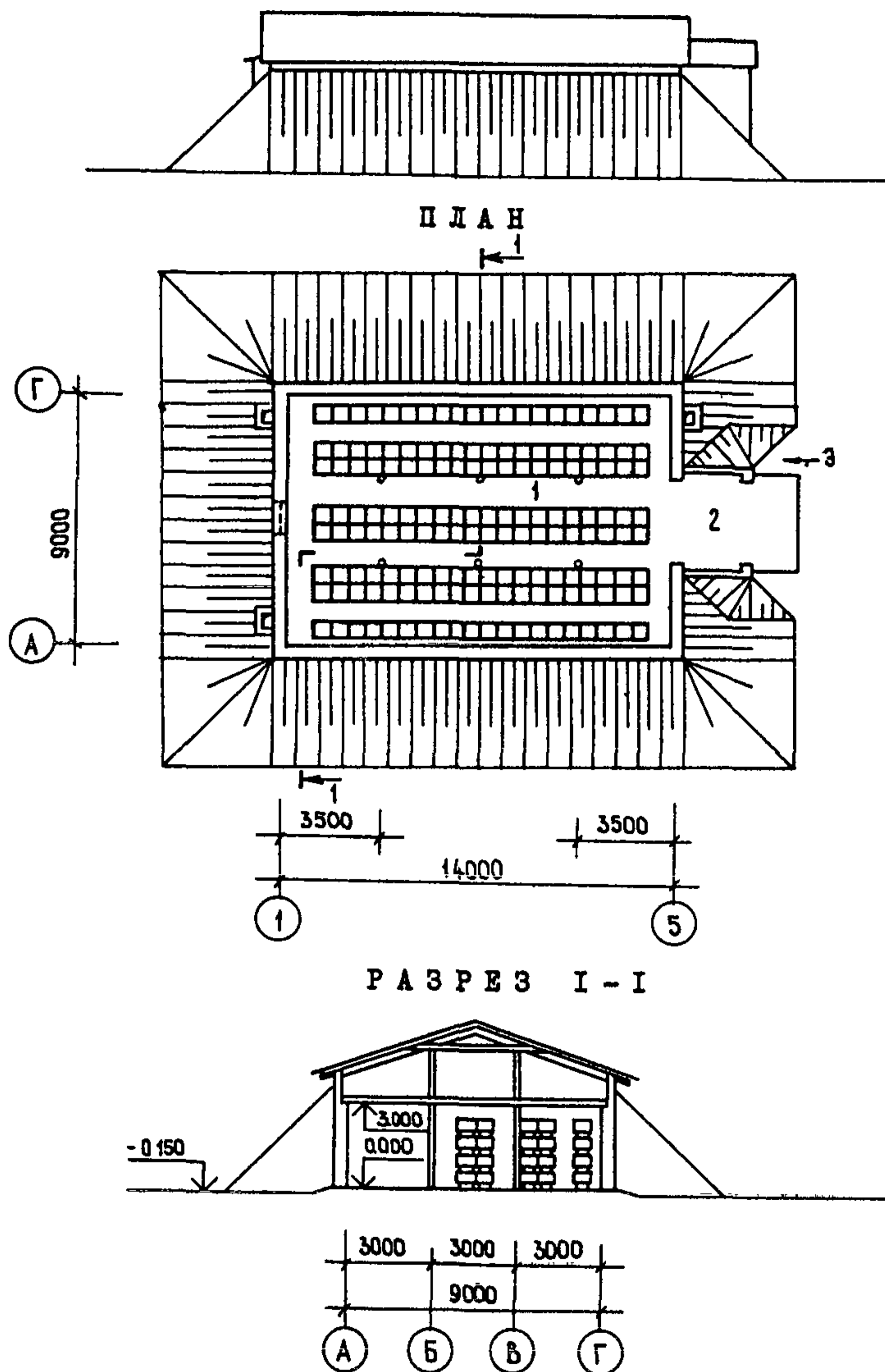
Рис. Д.8. Зимовник на 600 пчелиных семей (ТП 808-5-31.86) наземный: 1-помещение для ульев; 2-тамбур
