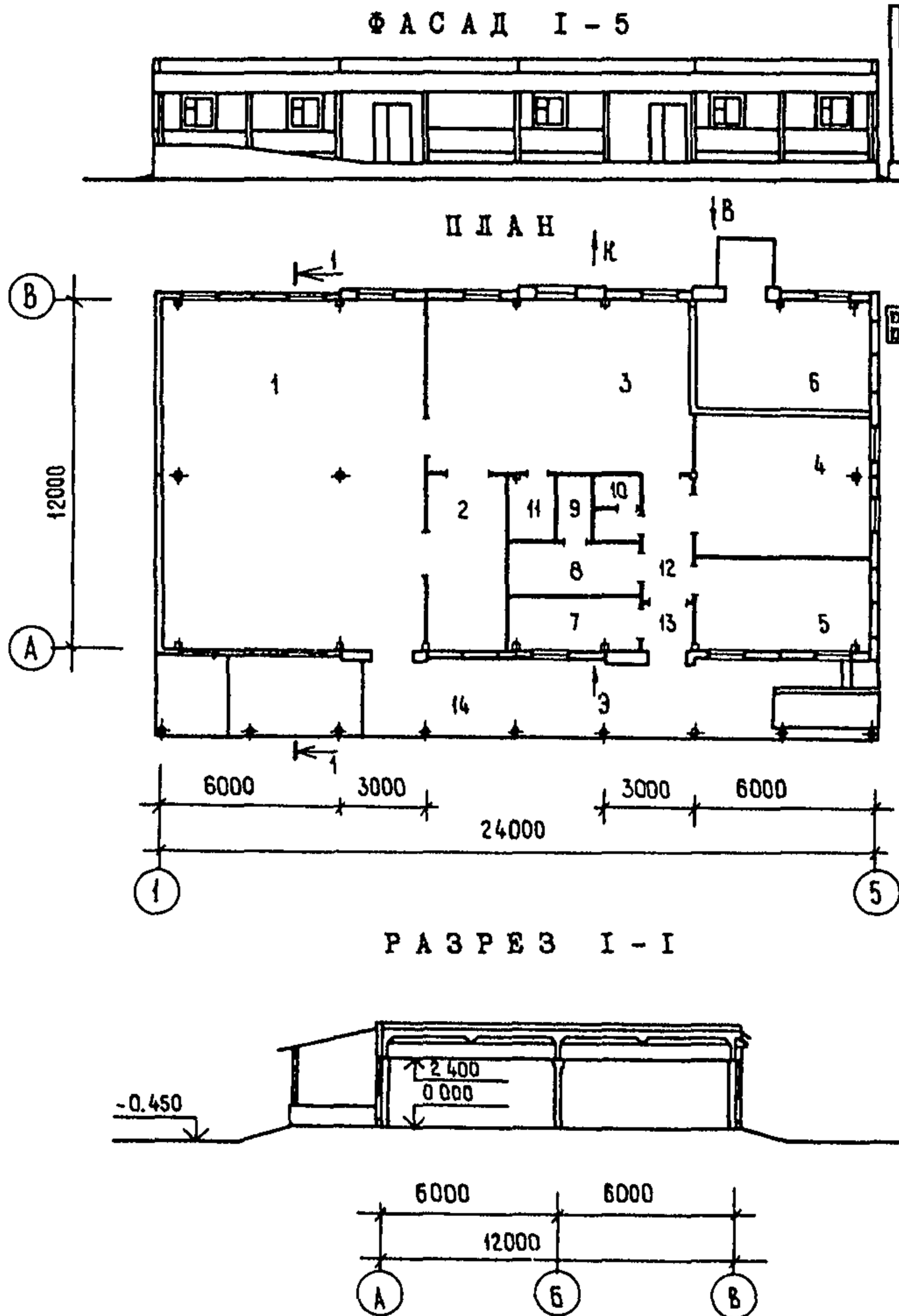
Рис. Г.1. Производственный корпус для пчеловодческой фермы на 600 пчелиных семей (ТП 808-5-40.86):
