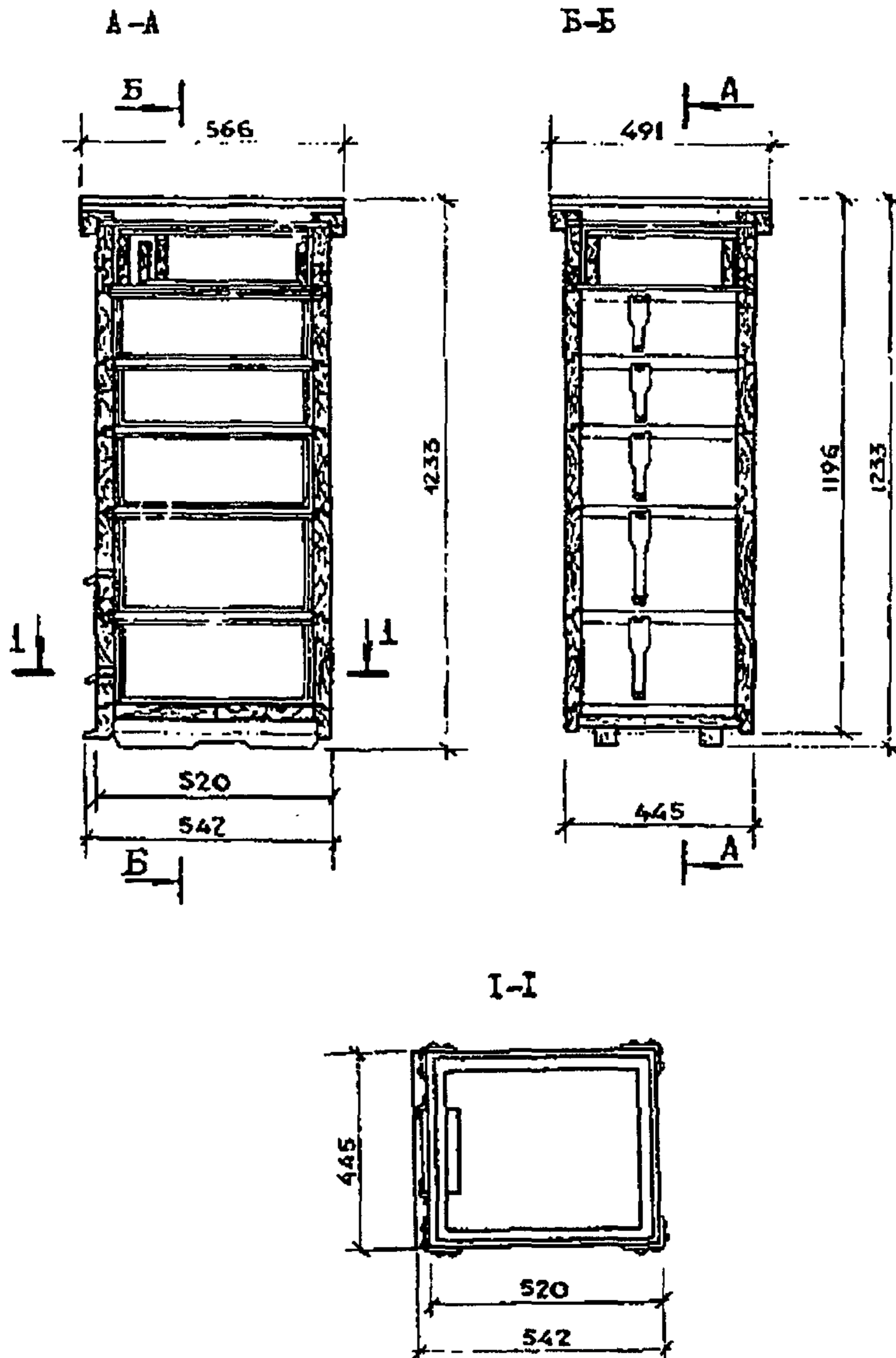
Рис. Е.6. Улей двухкорпусный с магазинами (серия 3.808-2)
