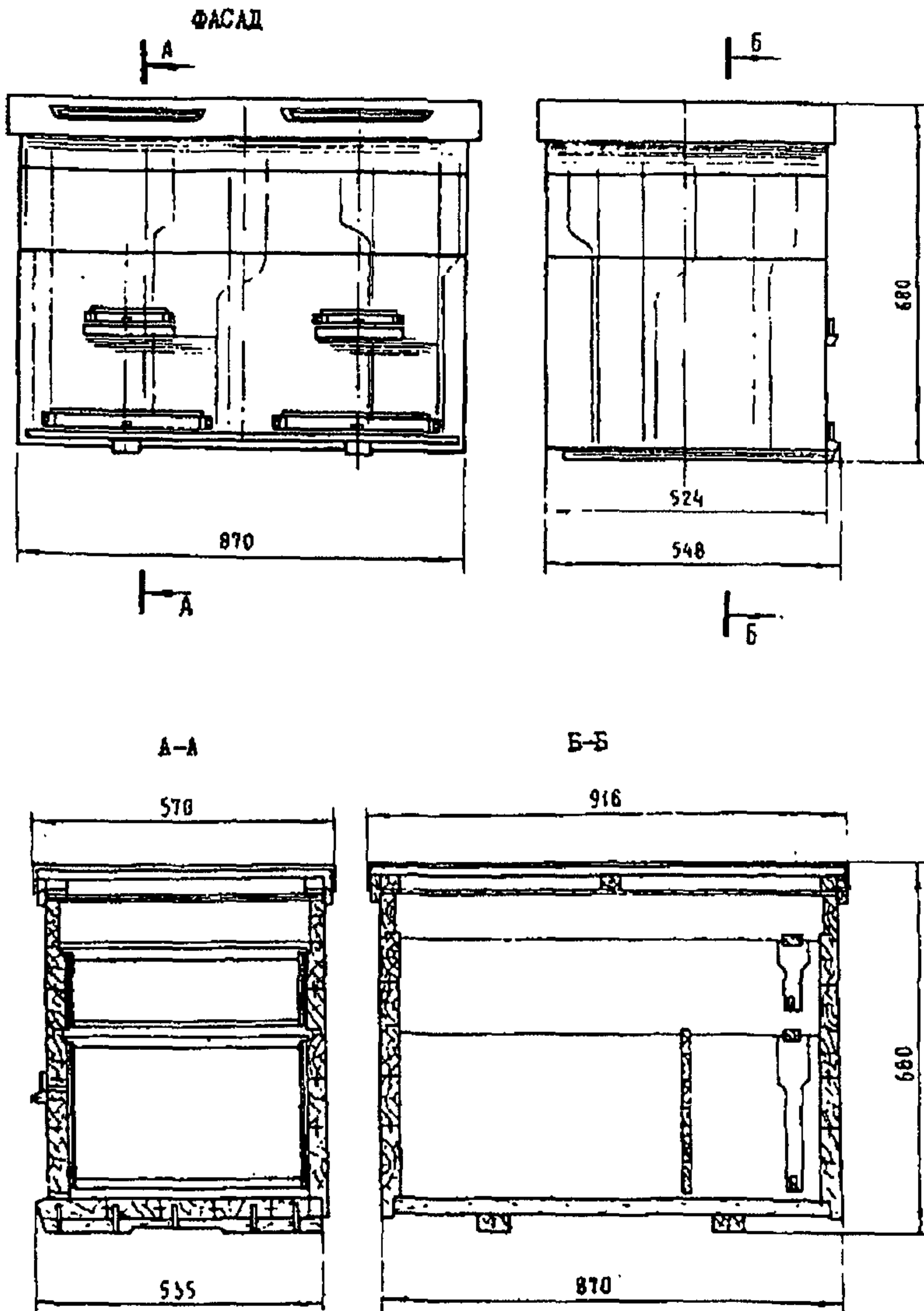
Рис. Е.4. Улей-лежака на 20 рамок с надставкой (серия 3.808-1)
