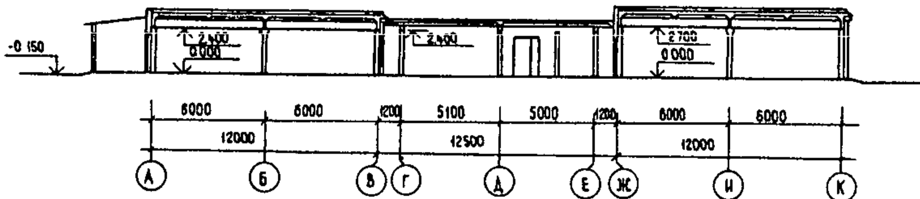
Рис. Г.4. Производственный корпус для пчеловодческой фермы на 4800 пчелиных семей (ТП 808-5-46.86):
