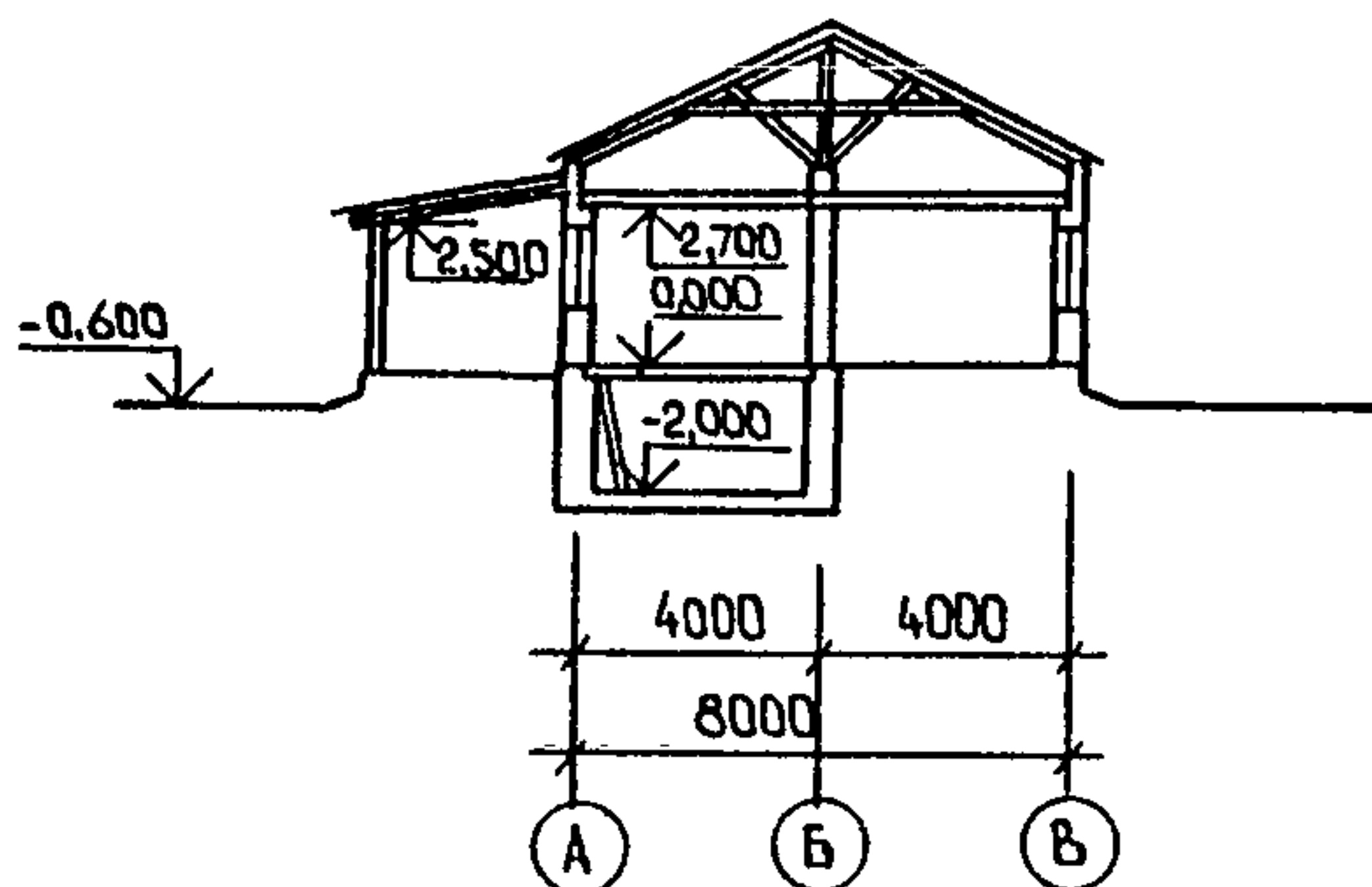
Рис. В.3. Пасечный дом с хозяйственным блоком на 200 пчелиных семей (ТП 808-5-50.92):
