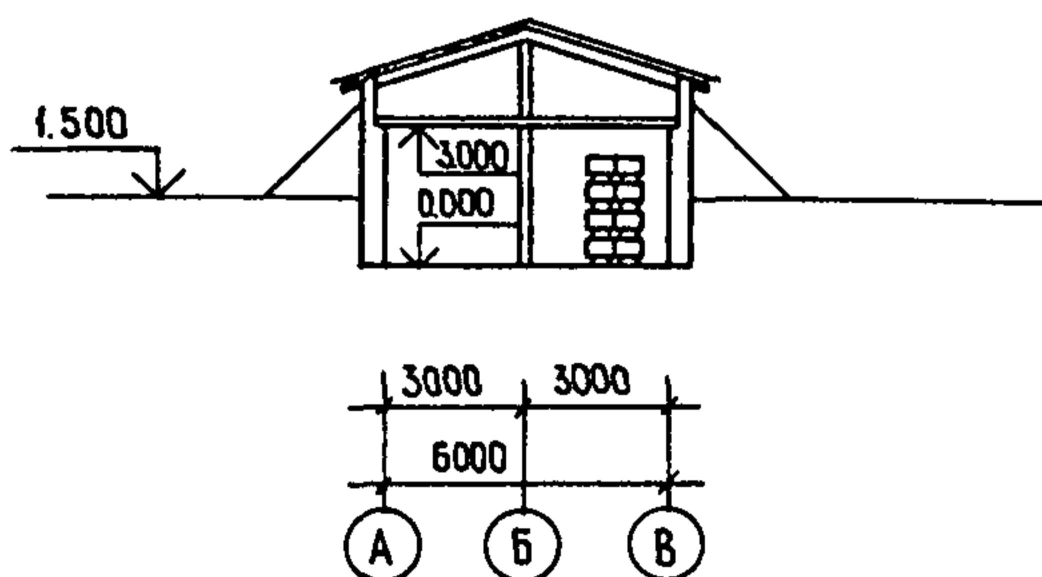
Рис. Д.7. Зимовник на 300 пчелиных семей (ТП 808-5-28.86) – полузаглубленный: 1-помещение для ульев; 2-тамбур
