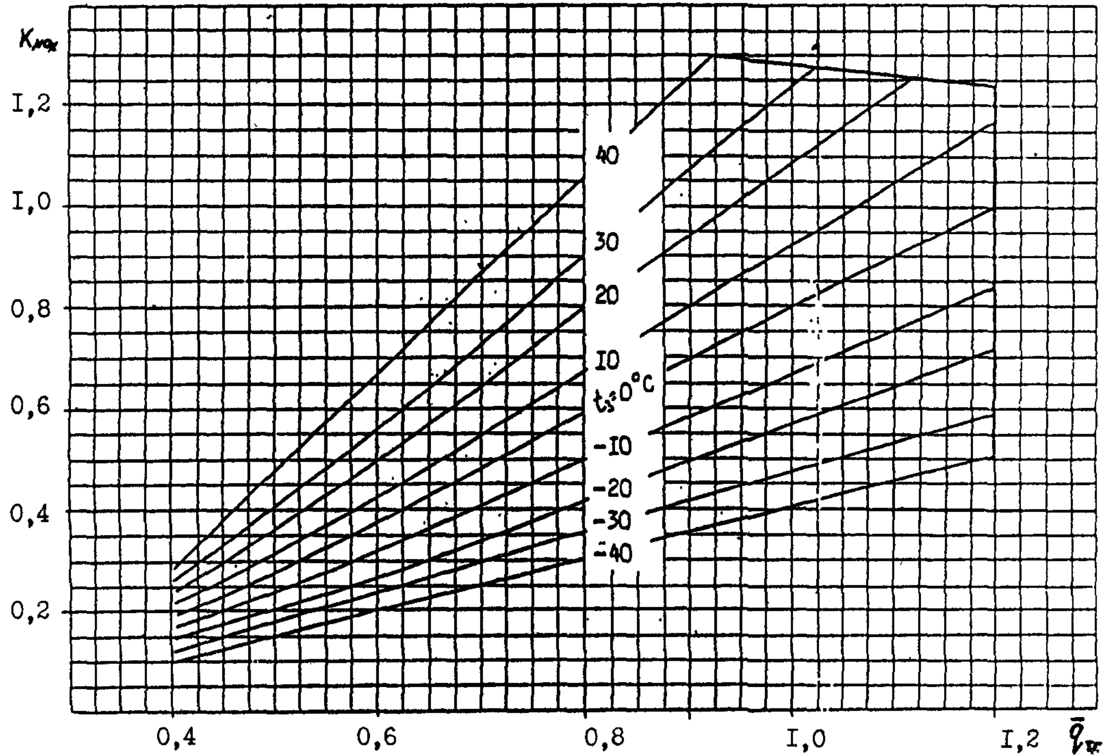
Рис.2. Зависимость коэффициента K_{NOx} от температуры воздуха на входе в компрессор и относительного расхода топливного газа \bar{q}_{TG} .
