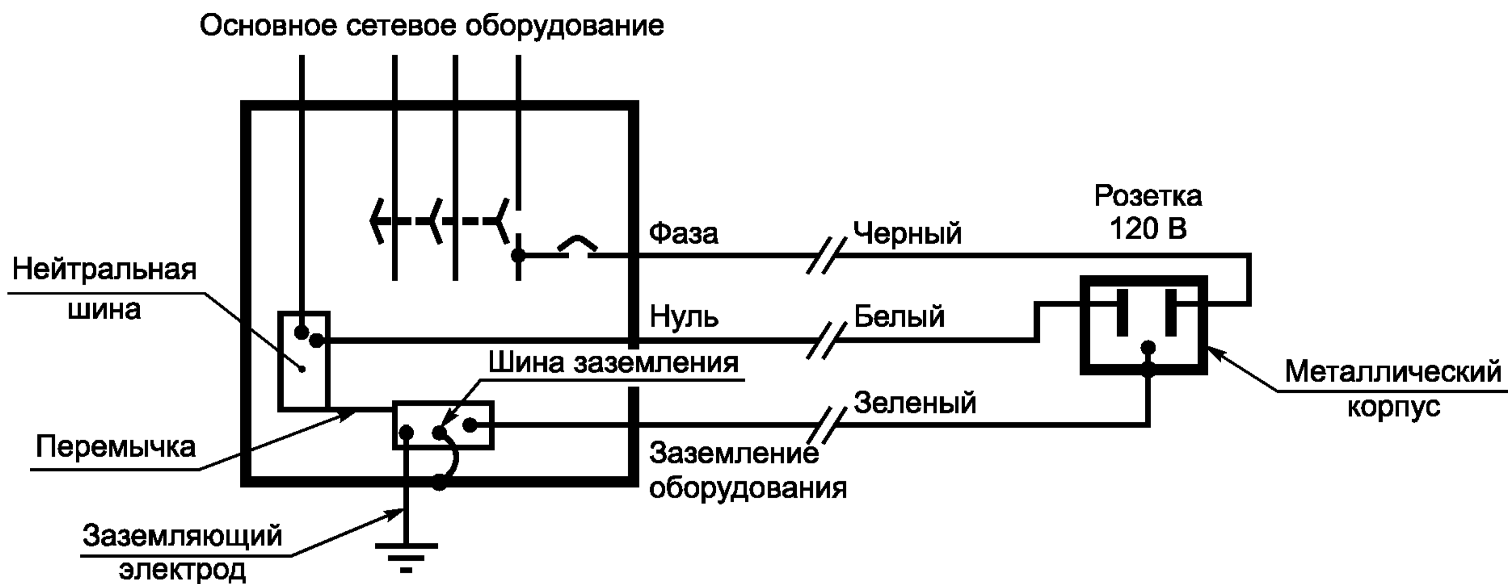
Рисунок 4а — Пример Североамериканской энергосистемы
