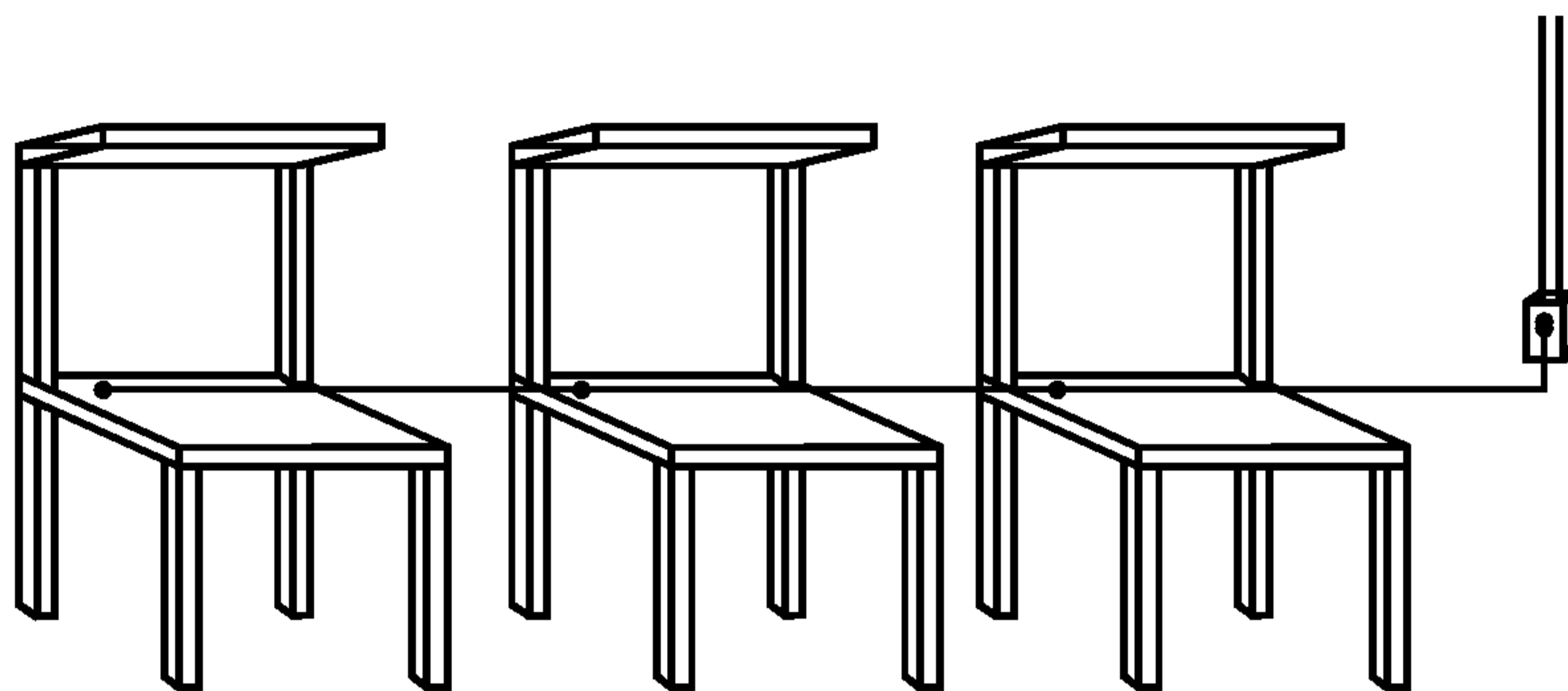
Рисунок 6 — Пример нерекондуемого заземления последовательно соединенных столов
