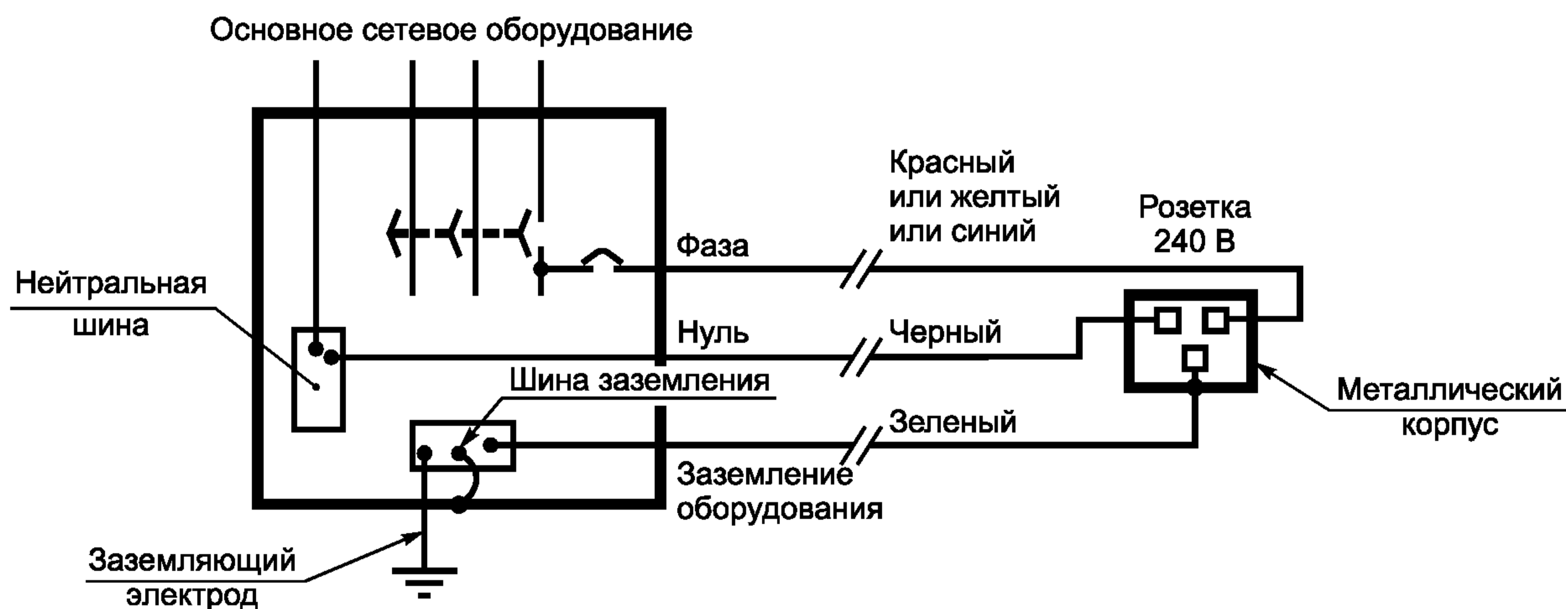
Рисунок 4б — Пример Малазийской энергосистемы
