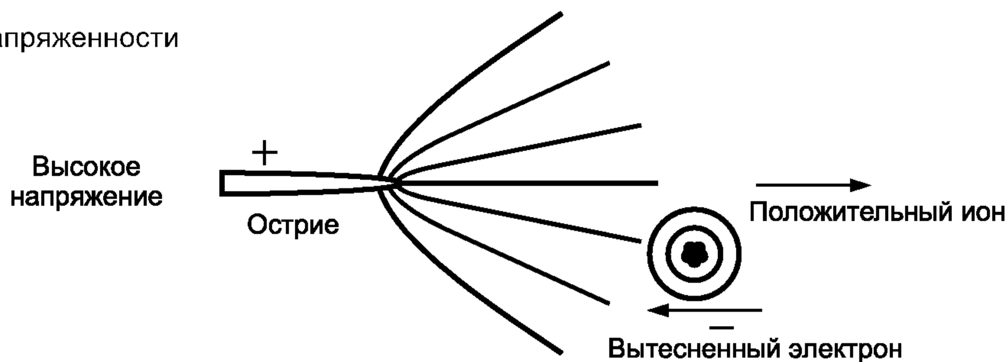
Рисунок 10 — Коронная ионизация — положительная
