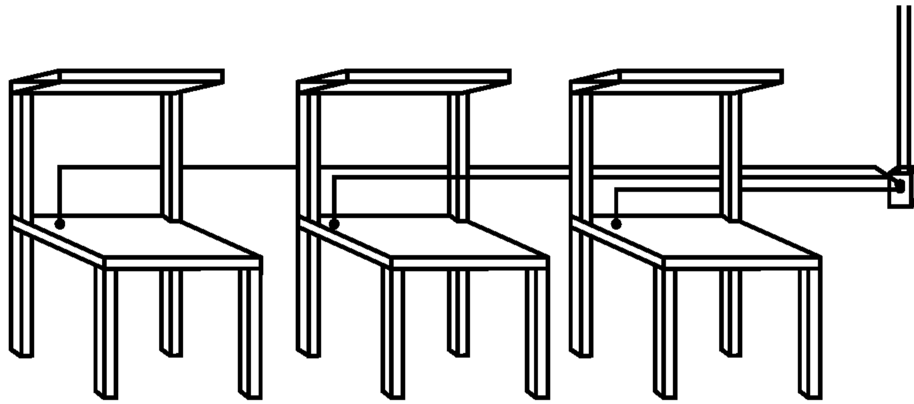
Рисунок 5 — Пример рекомендуемого индивидуального заземления столов
