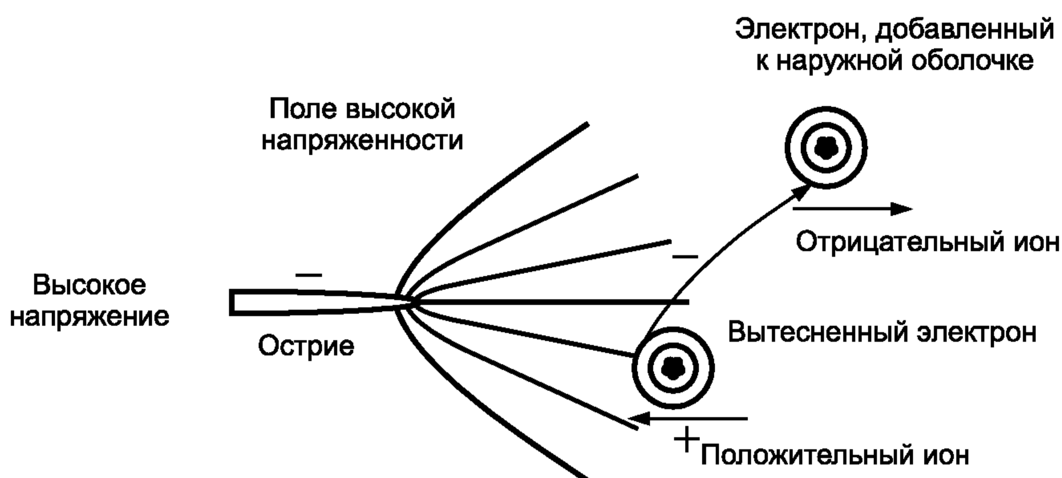
Рисунок 11 — Коронная ионизация — отрицательная
