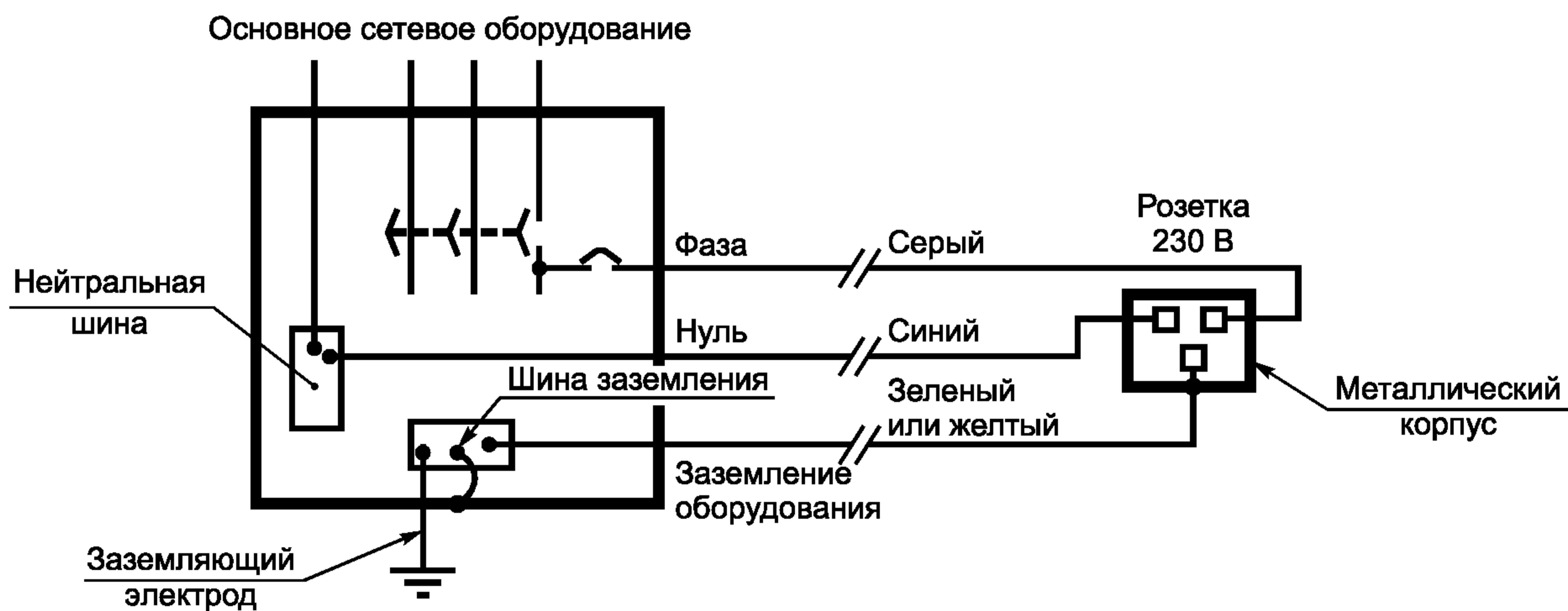
Рисунок 4в — Пример энергосистемы Великобритании — Однофазная система
