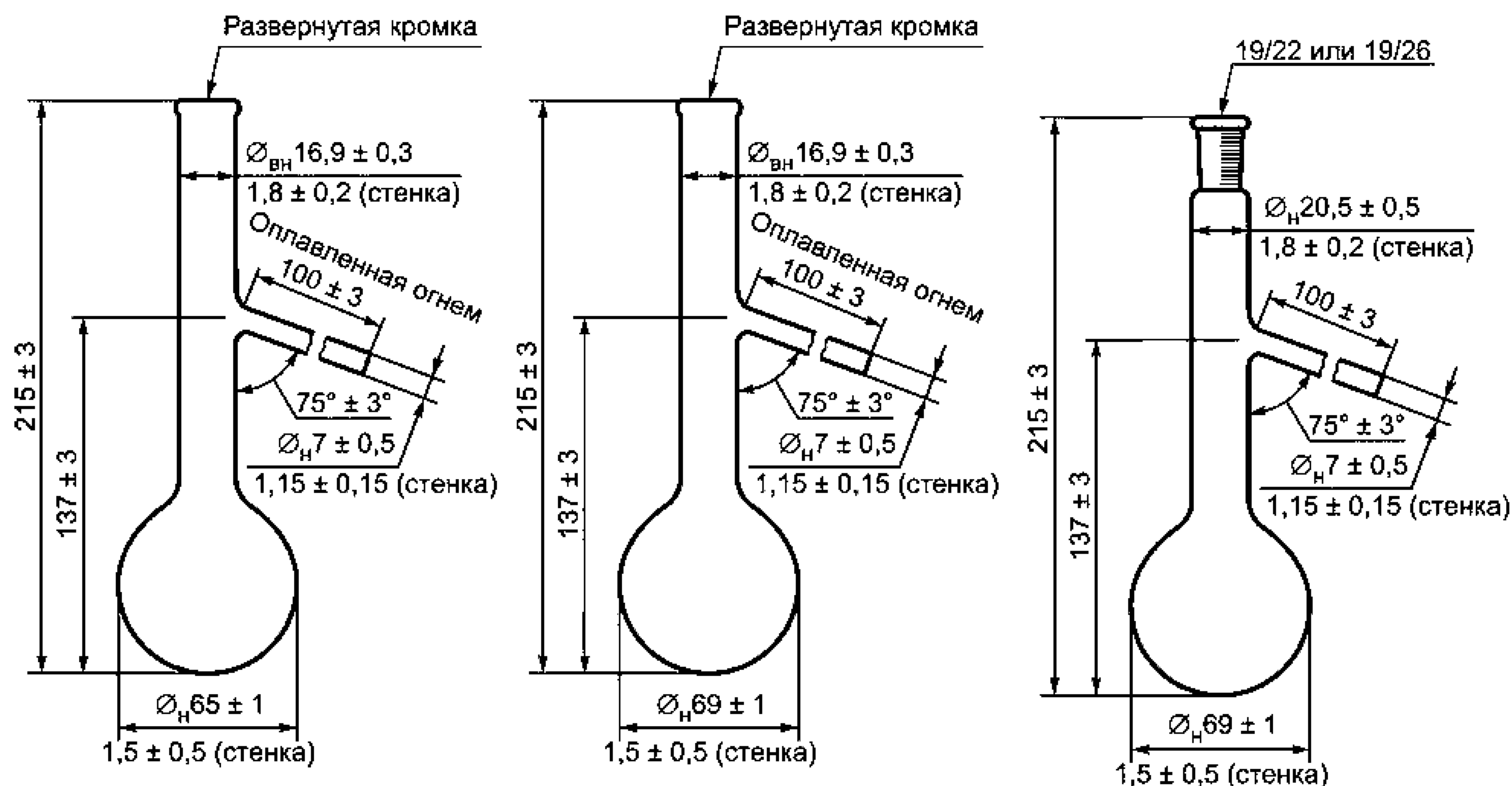
a — Колба А вместимостью 100 см 3
