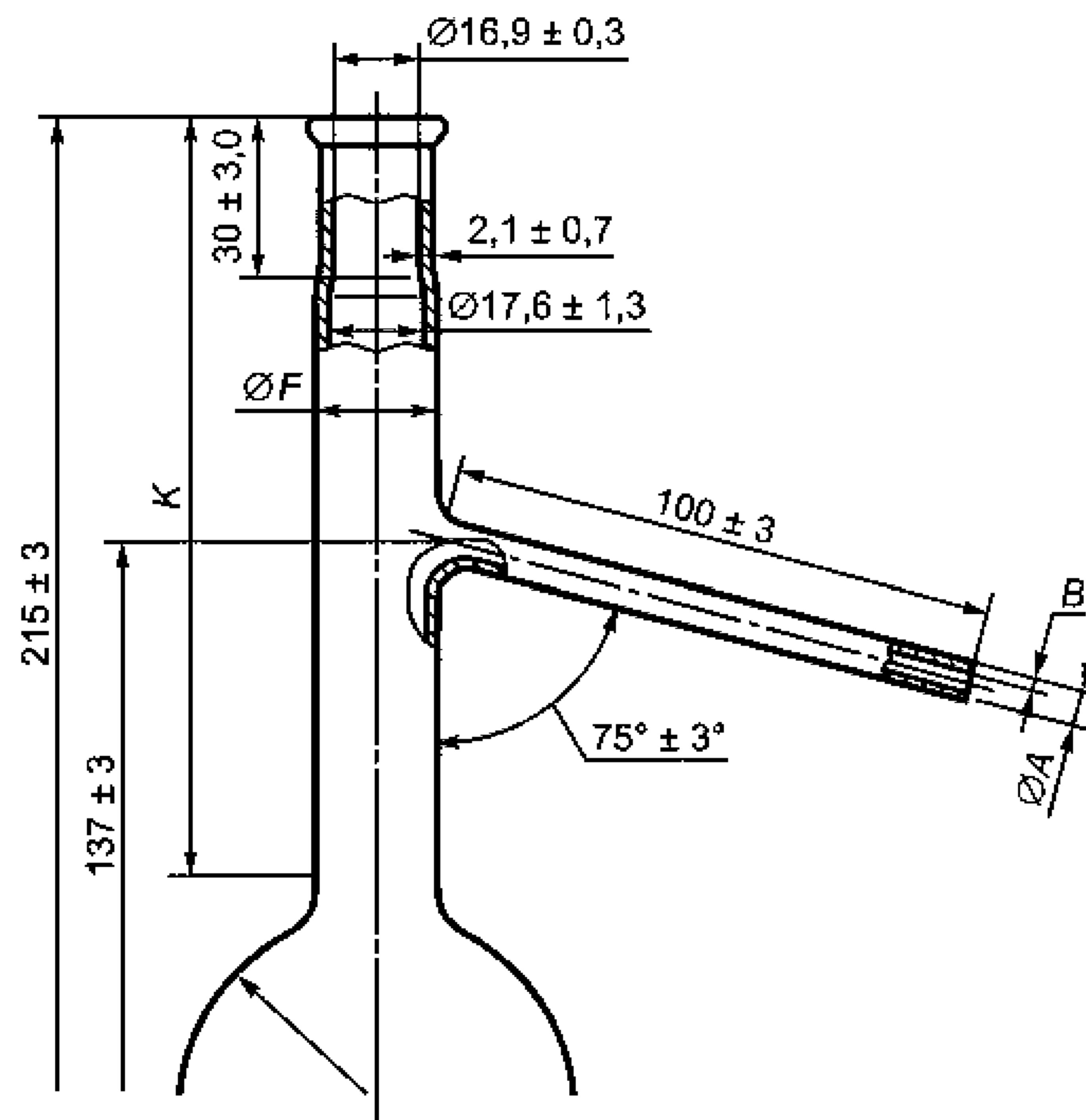
Рисунок А2.2 — Верхняя часть колбы
