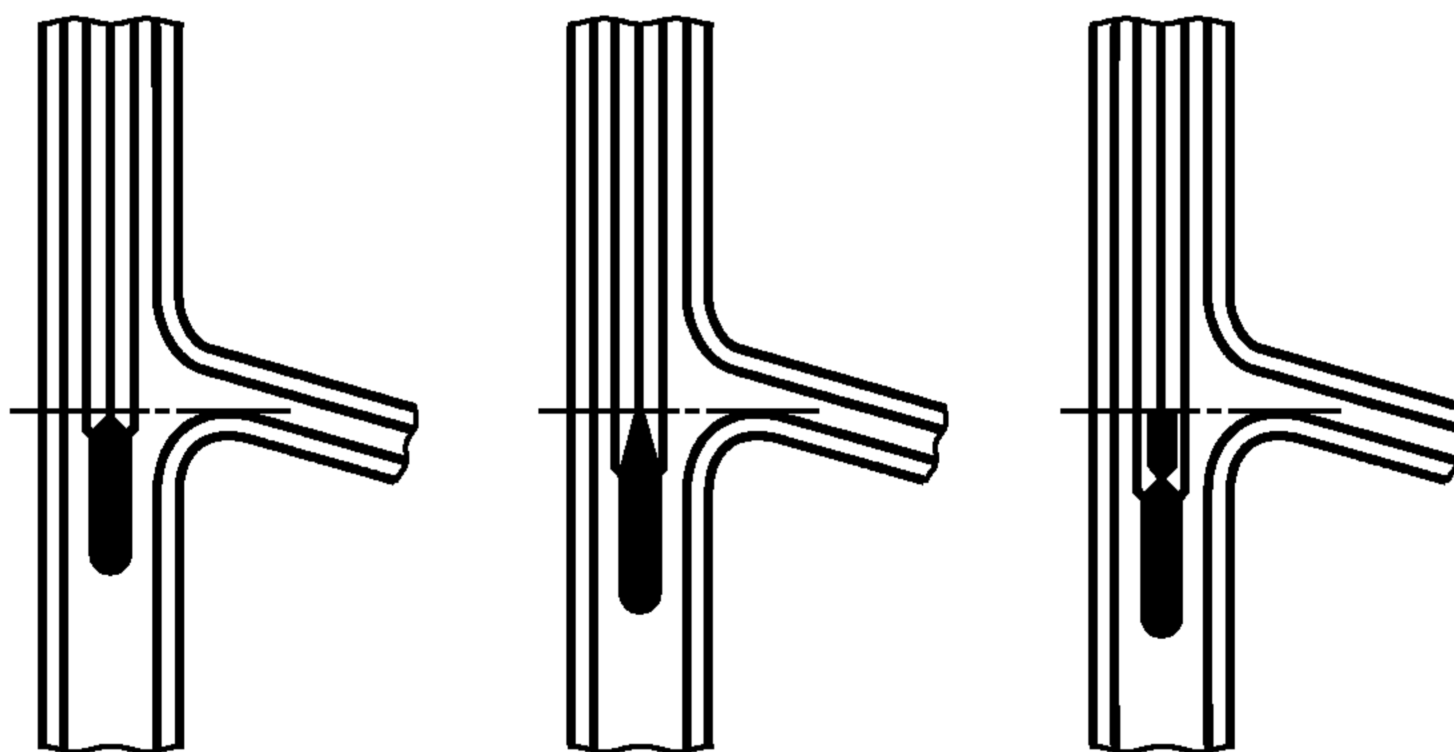
Рисунок 5 — Положение термометра в колбе для разгонки
