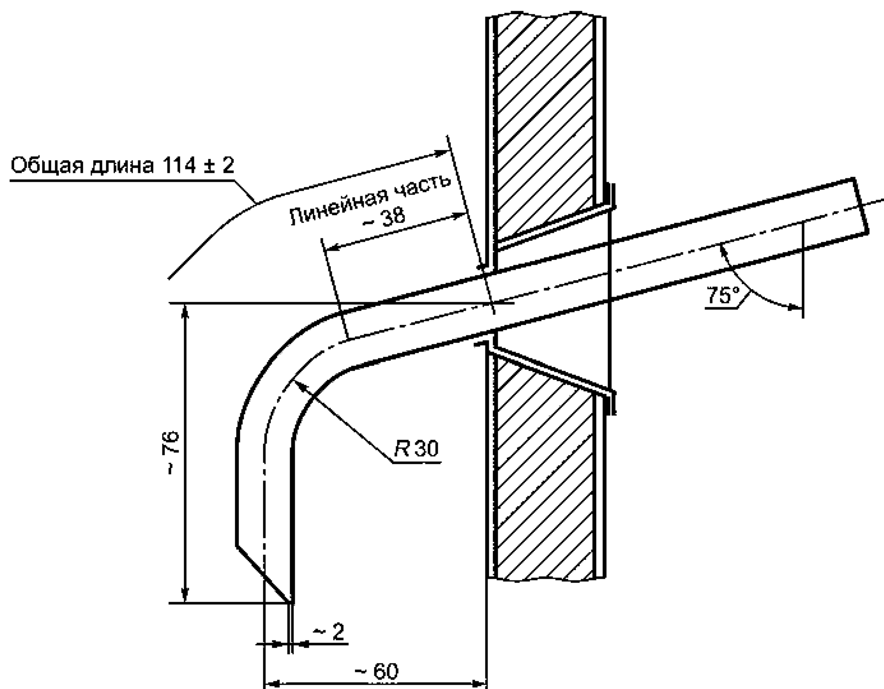
Рисунок А2.3 — Нижний конец трубки конденсатора
