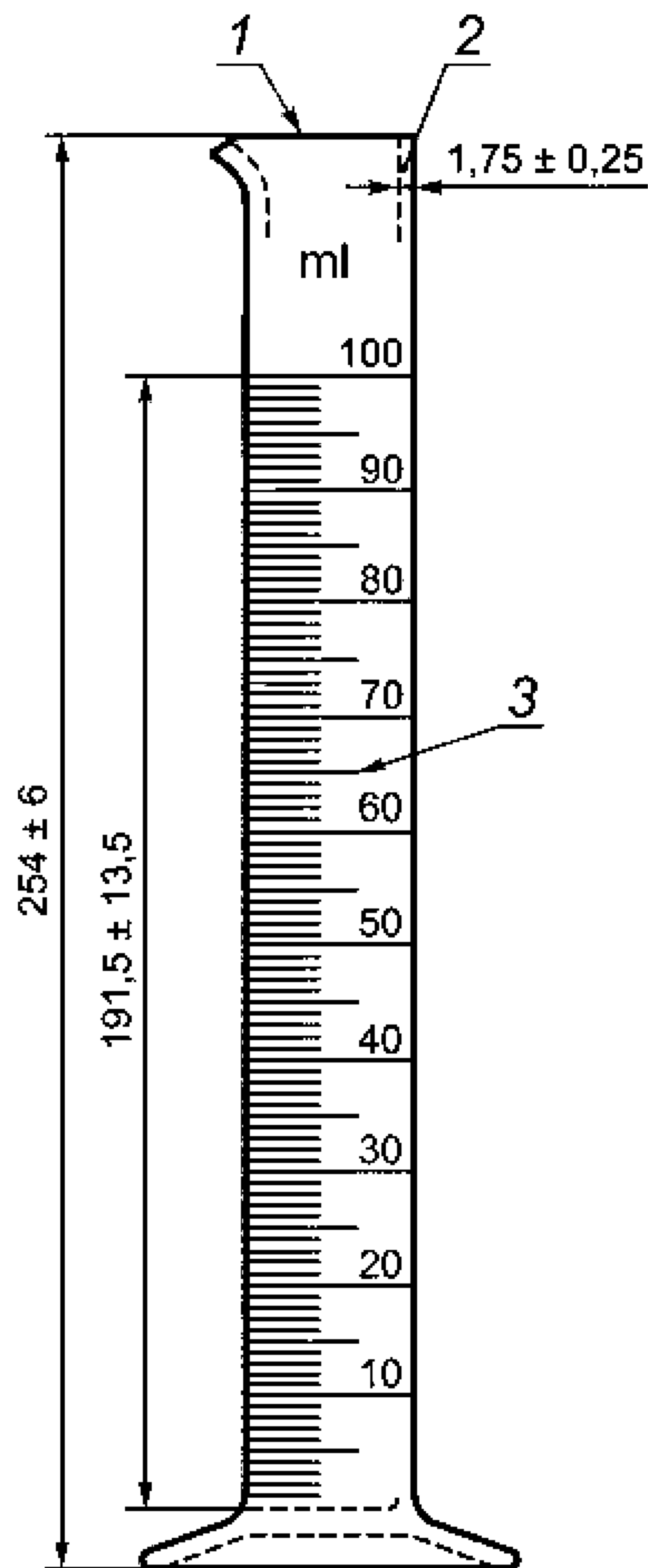
1 — оплавленный край; 2 — стенка; 3 — шкала
