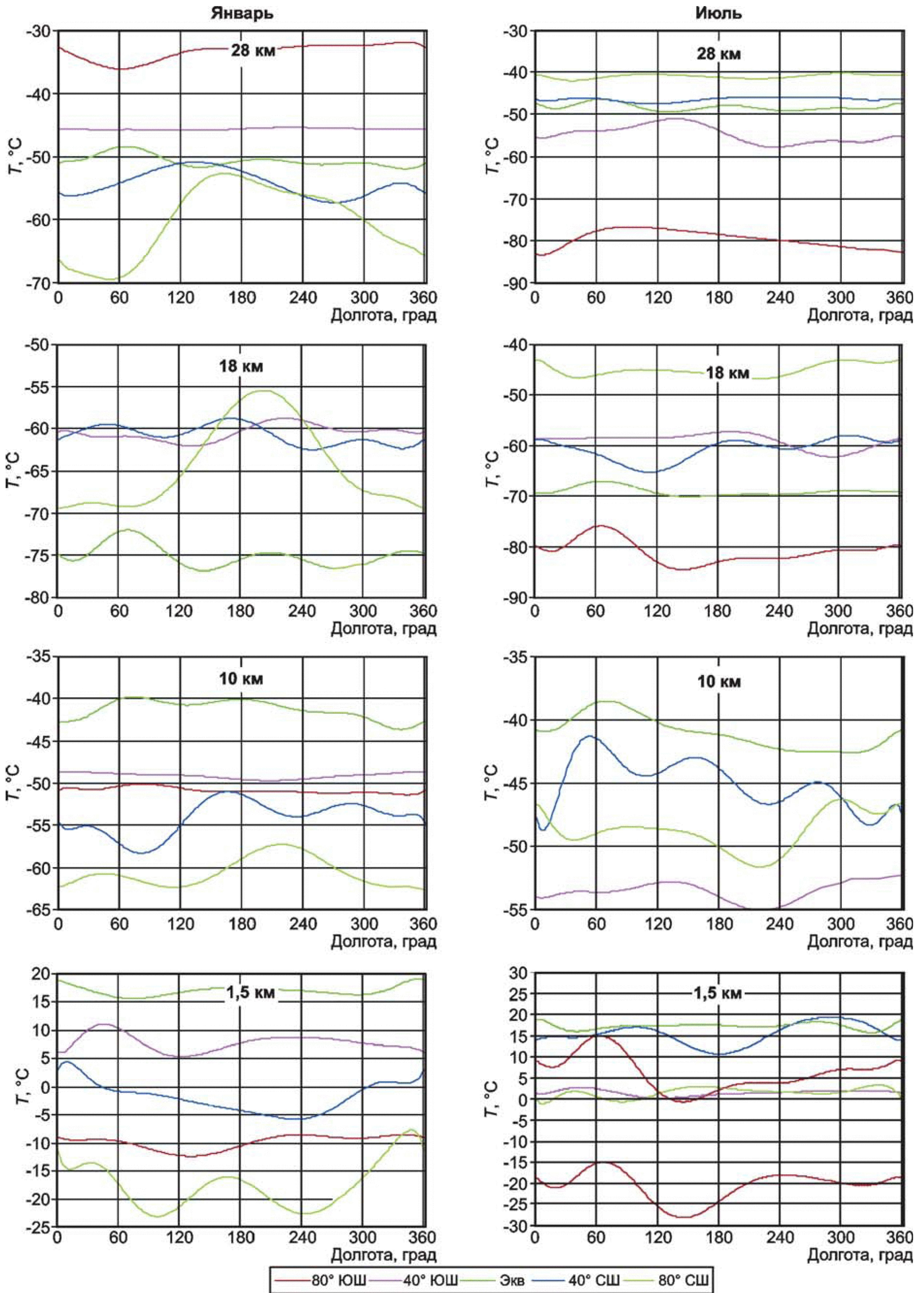
Рисунок Б.9 — Долготная изменчивость температуры T при ее аппроксимации полиномом 10-й степени вдоль долготы на различных высотах атмосферы и в различных широтных поясах для января и июля
