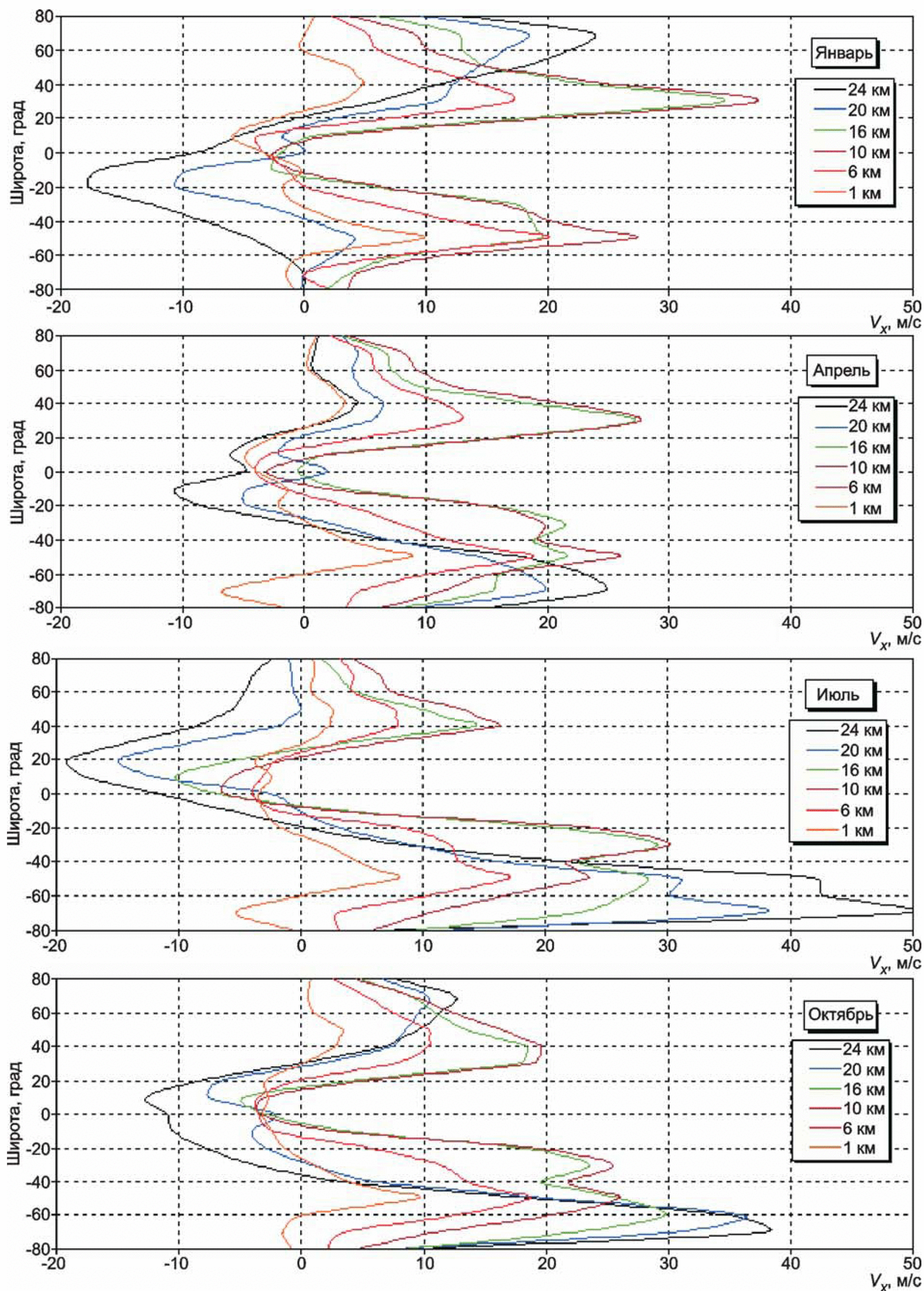
Рисунок А.17 — Широтная зависимость средних широтных значений зональной скорости ветра на высотах атмосферы до 30 км
