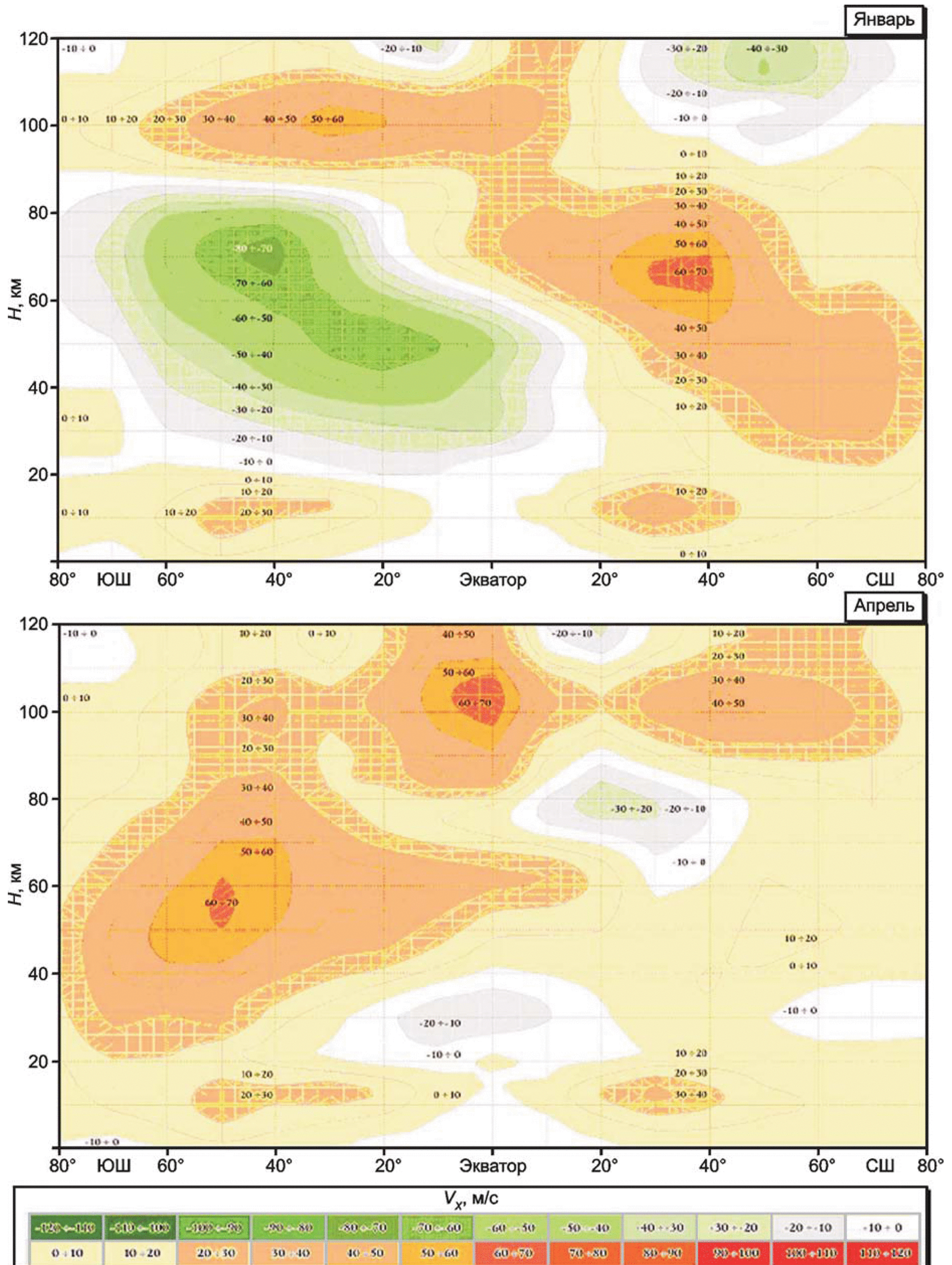
Рисунок А.13 — Изолинии средних широтных значений зональной скорости ветра в атмосфере на широтно-высотной сетке для центральных месяцев сезонов
