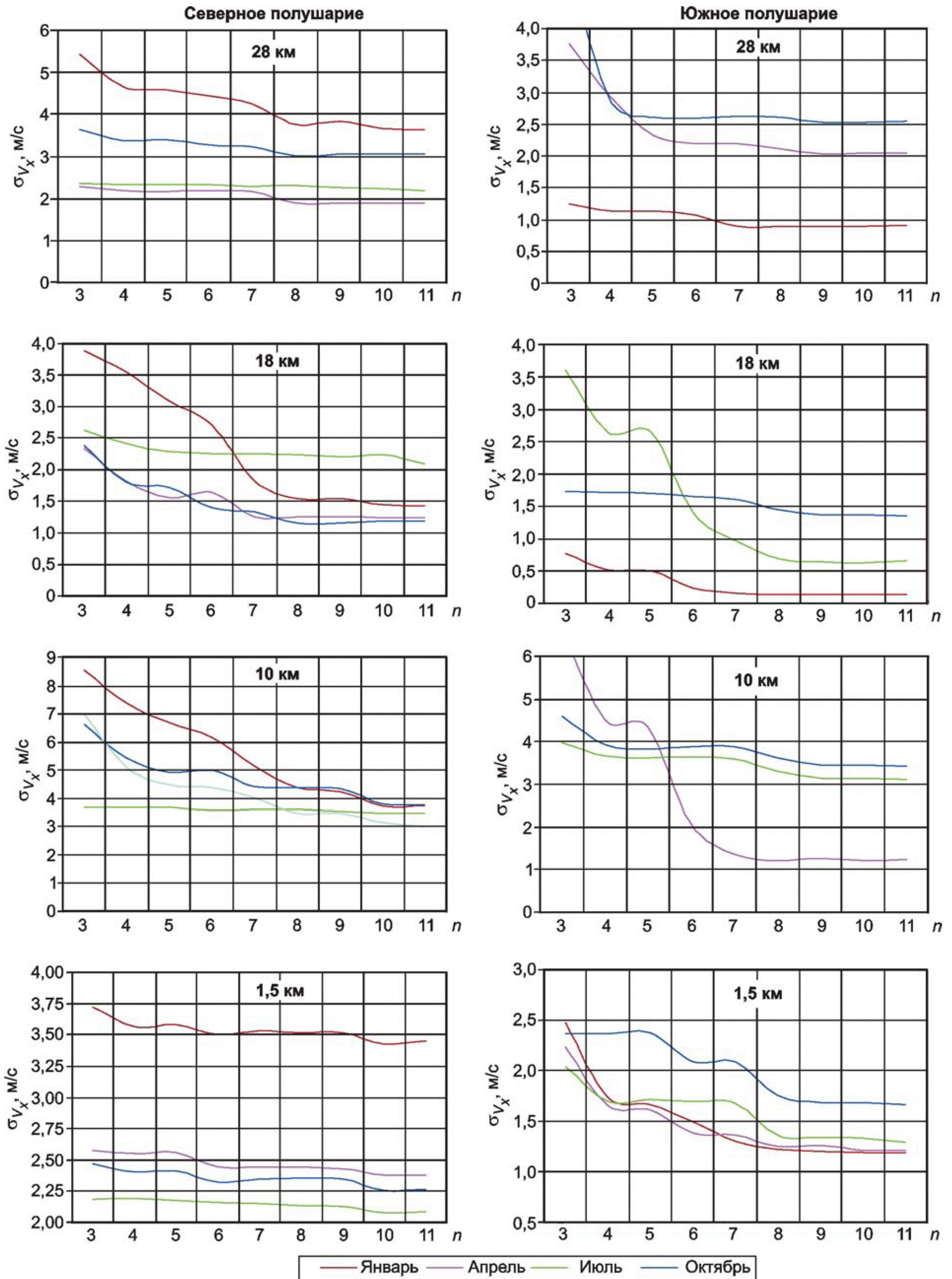
Рисунок Б.5 — Зависимость точности моделирования долготных вариаций зональной скорости ветра \sigma_{V_x} от степени аппроксимирующего полинома n на различных высотах нижней атмосферы в широтных поясах 35^\circ - 45^\circ в северном и южном полушариях
