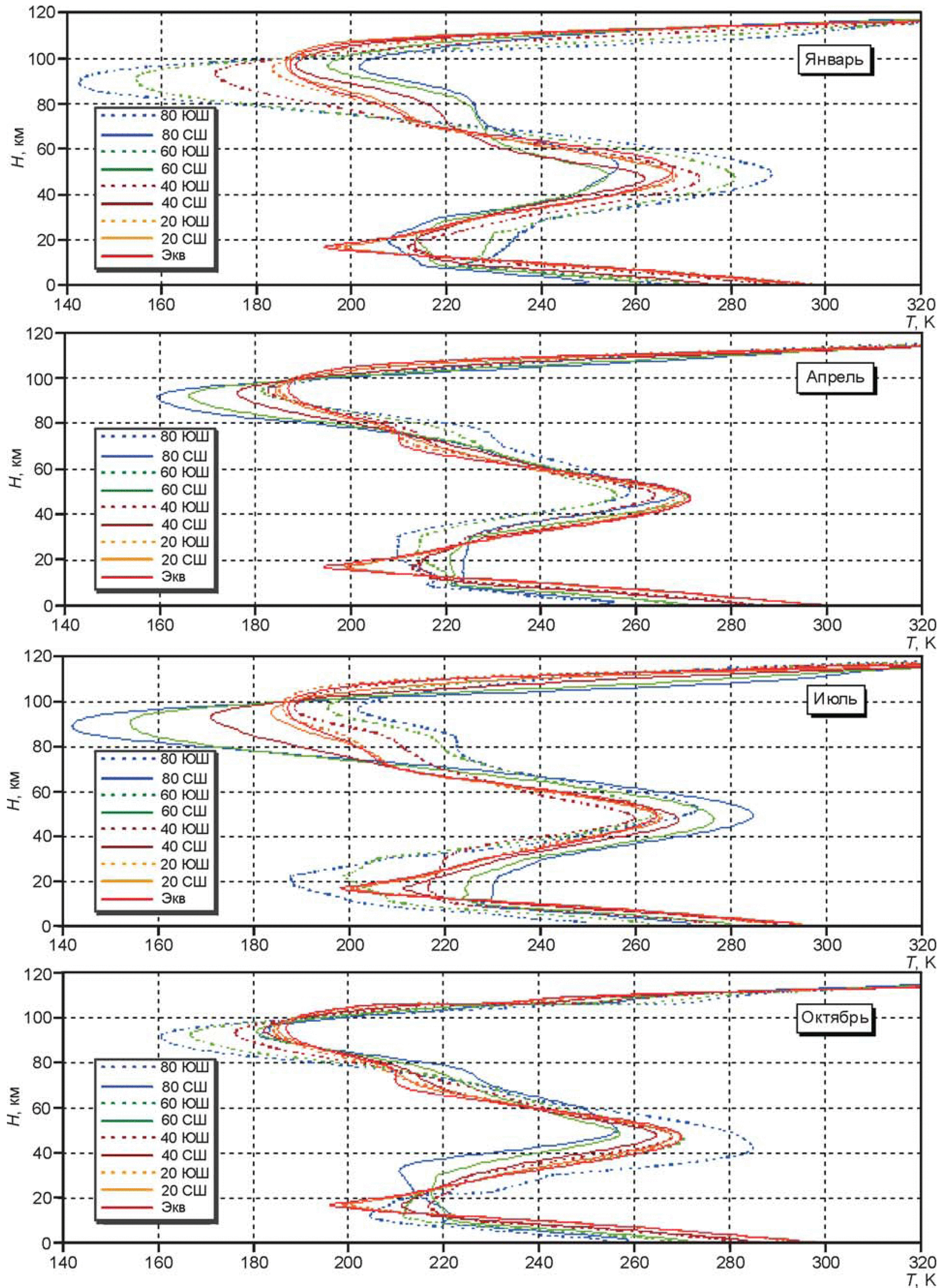
Рисунок А.1 — Вертикальные профили средних широтных значений температуры в атмосфере для центральных месяцев сезонов
