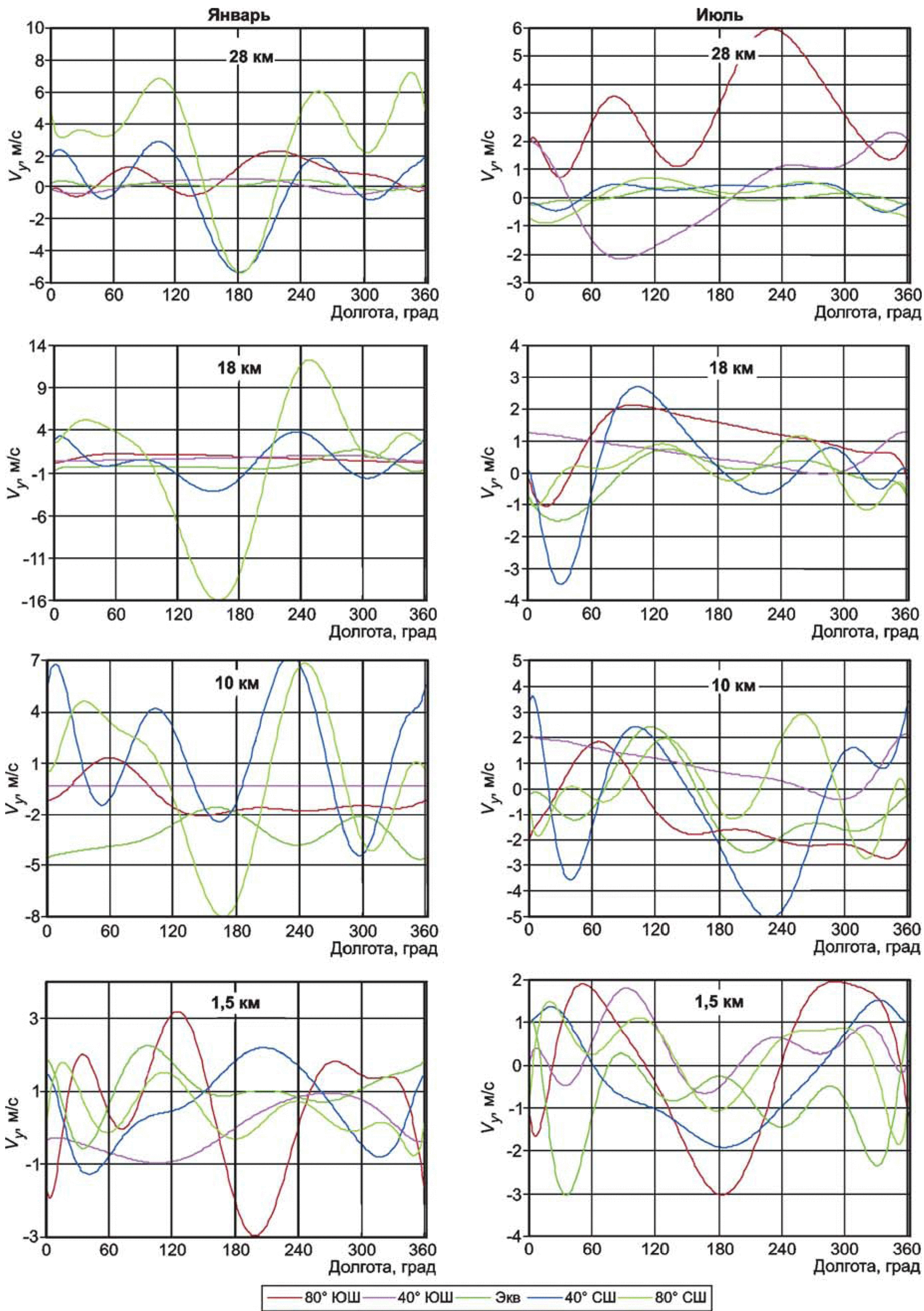
Рисунок Б.11 — Долготная изменчивость меридиональной скорости ветра при ее аппроксимации полиномом 10-й степени вдоль долготы на различных высотах атмосферы и в различных широтных поясах для января и июля
