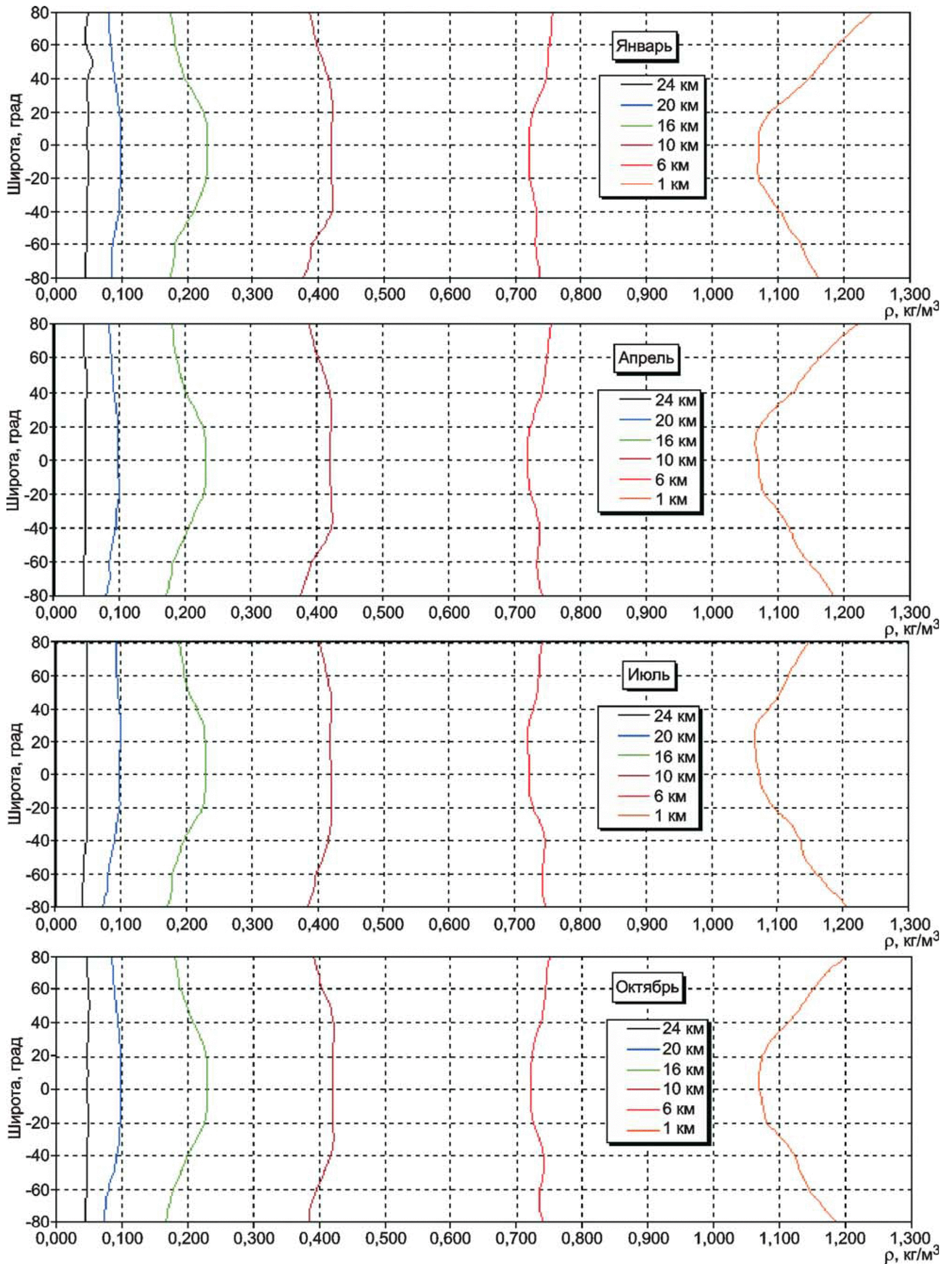
Рисунок А.11 — Средняя многолетняя широтная изменчивость средних широтных значений плотности на различных высотах атмосферы до 30 км для центральных месяцев сезонов
