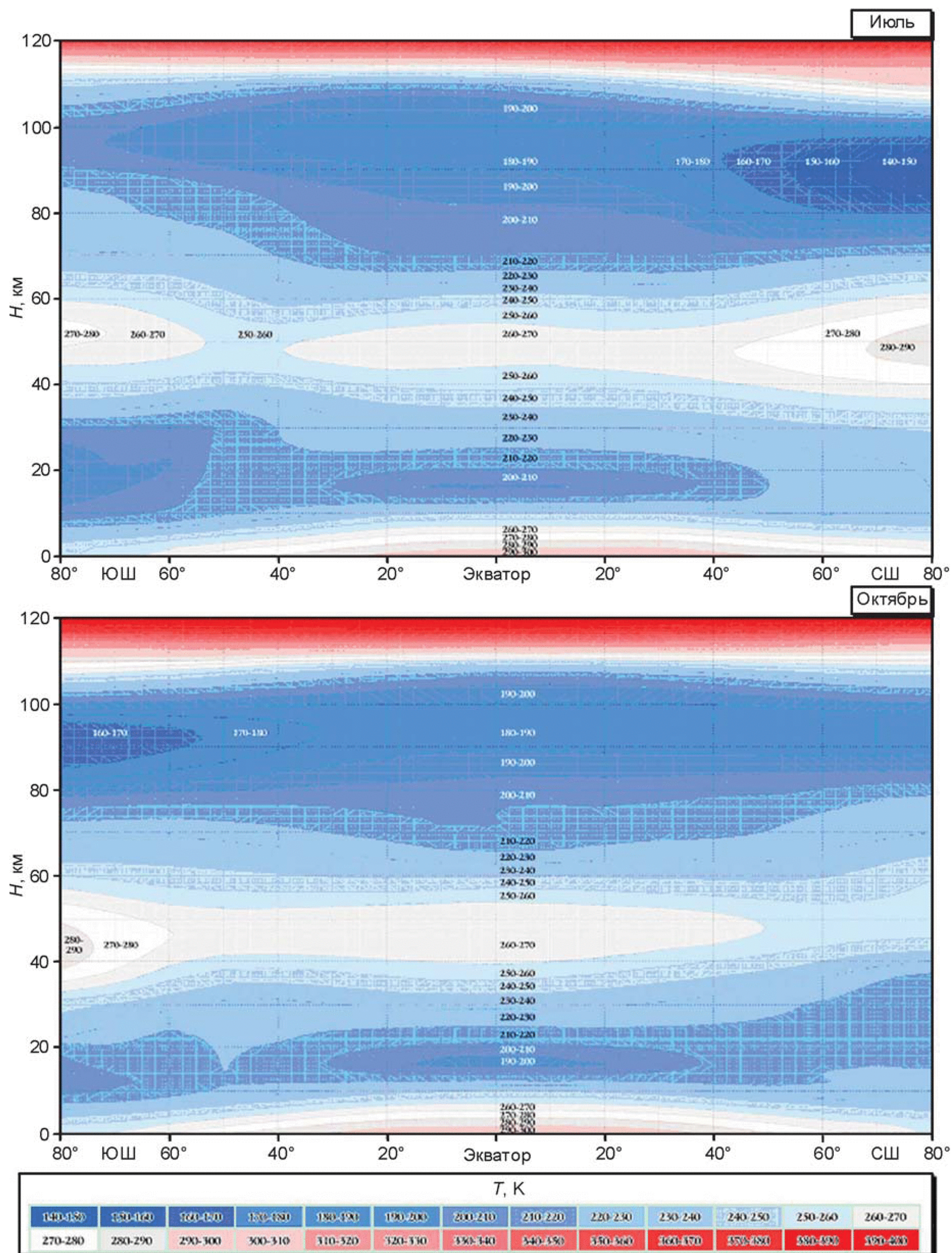
Рисунок А.3 — Изотермы средних широтных значений температуры в атмосфере на высотно-широтной сетке для центральных месяцев сезонов
