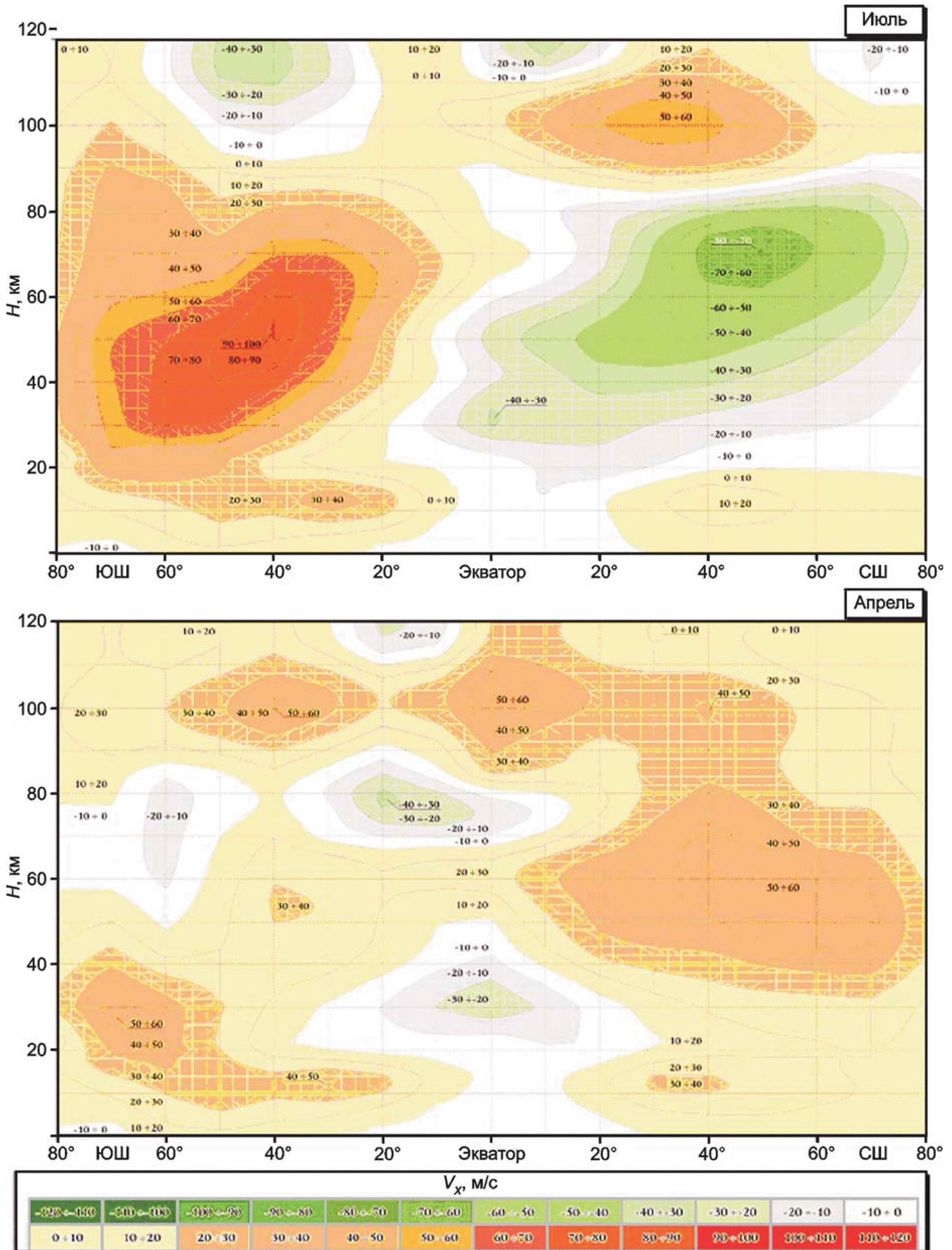
Рисунок А.14 — Изолинии средних широтных значений зональной скорости ветра в атмосфере на широтно-высотной сетке для центральных месяцев сезонов
