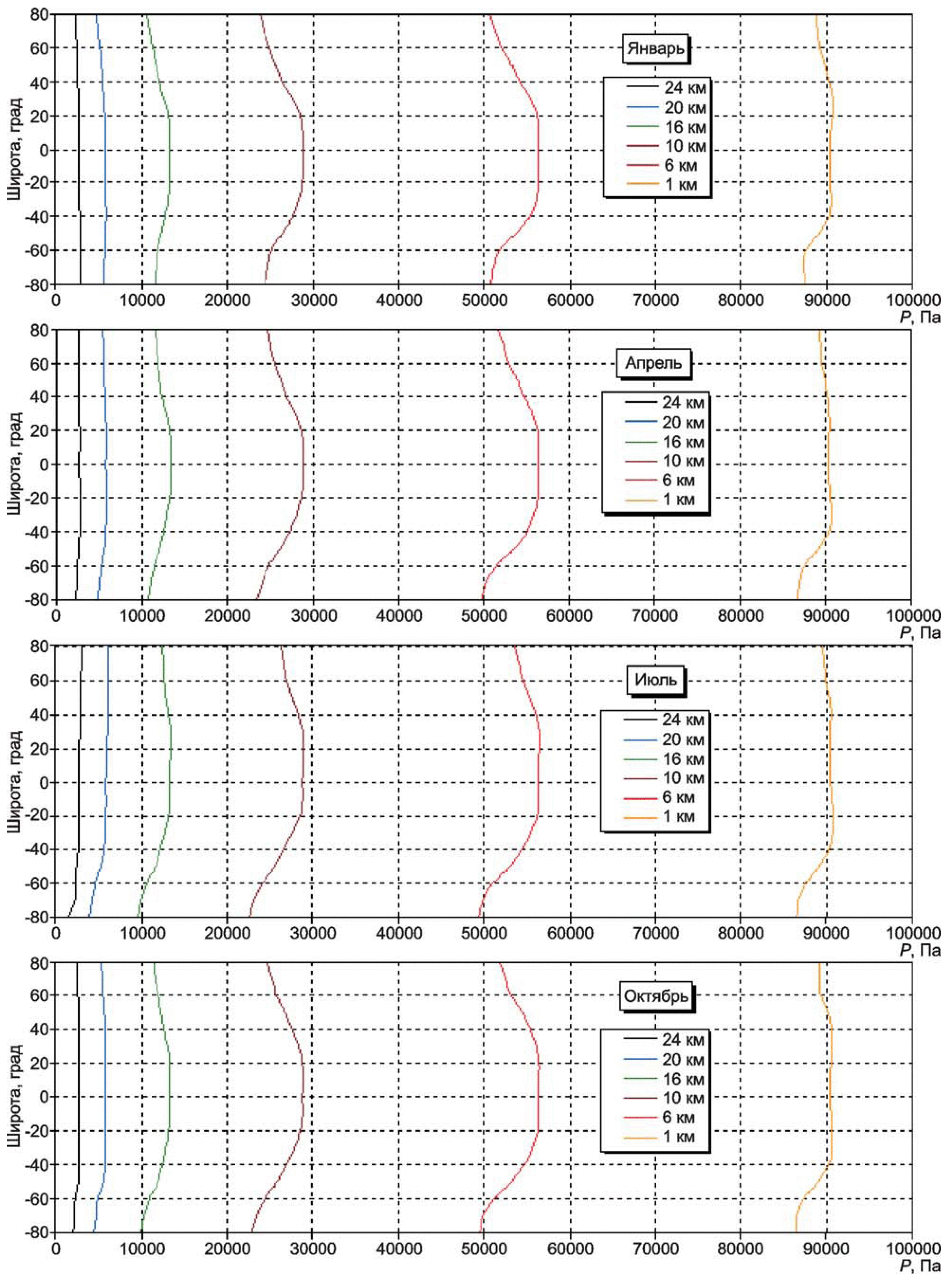
Рисунок А.8 — Зависимость от широты средних широтных значений давления в атмосфере на высотах до 30 км для центральных месяцев сезона
