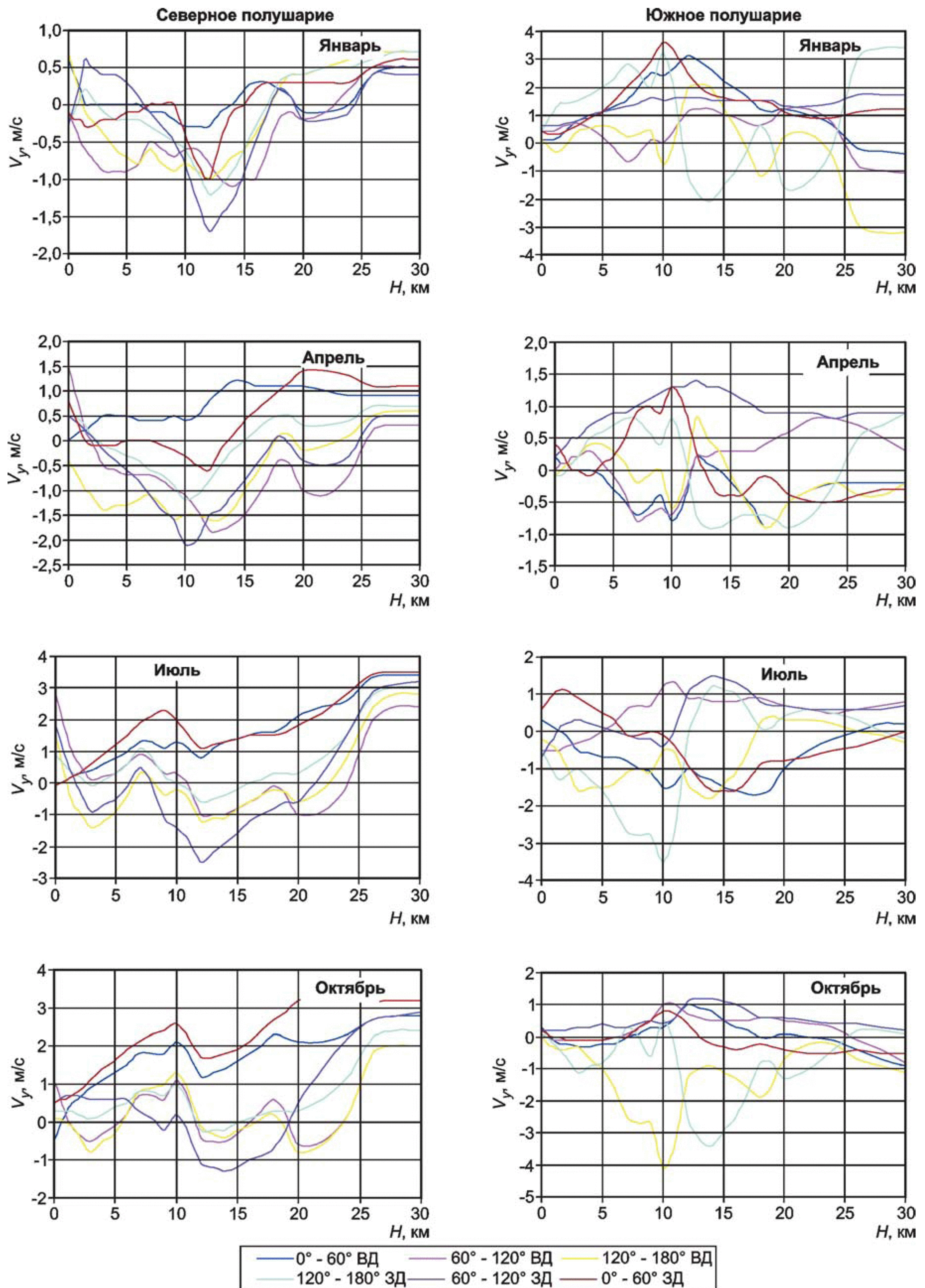
Рисунок Б.14 — Высотные профили меридиональной скорости ветра V_y при их аппроксимации полиномом 10-й степени на высотах от 0 до 30 км на разной долготе в широтных поясах 35^\circ — 45^\circ в северном и южном полушариях
