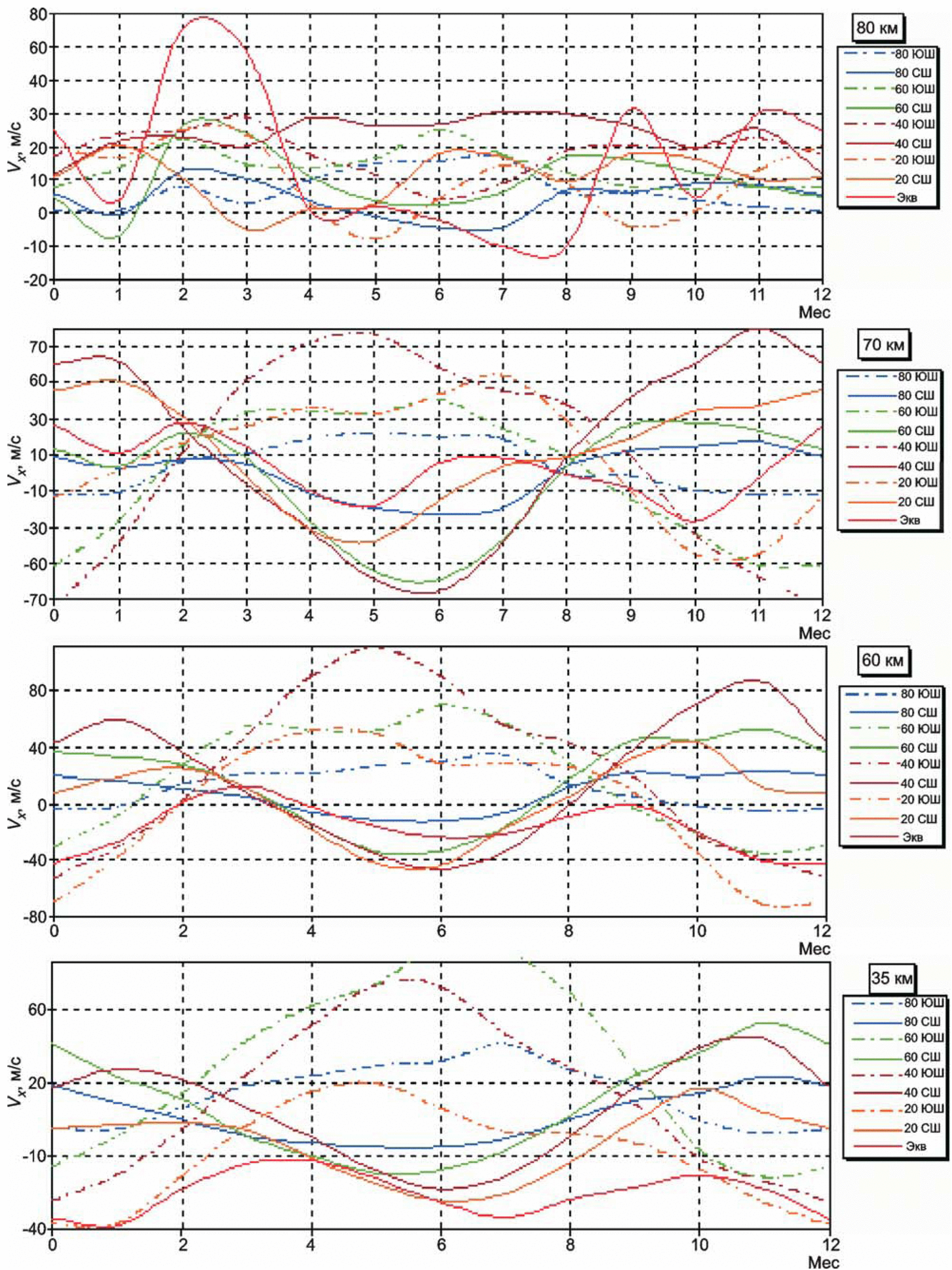
Рисунок А.16 — Средняя многолетняя внутригодовая изменчивость средних широтных значений зональной скорости ветра на разных широтах и высотах от 30 до 120 км
