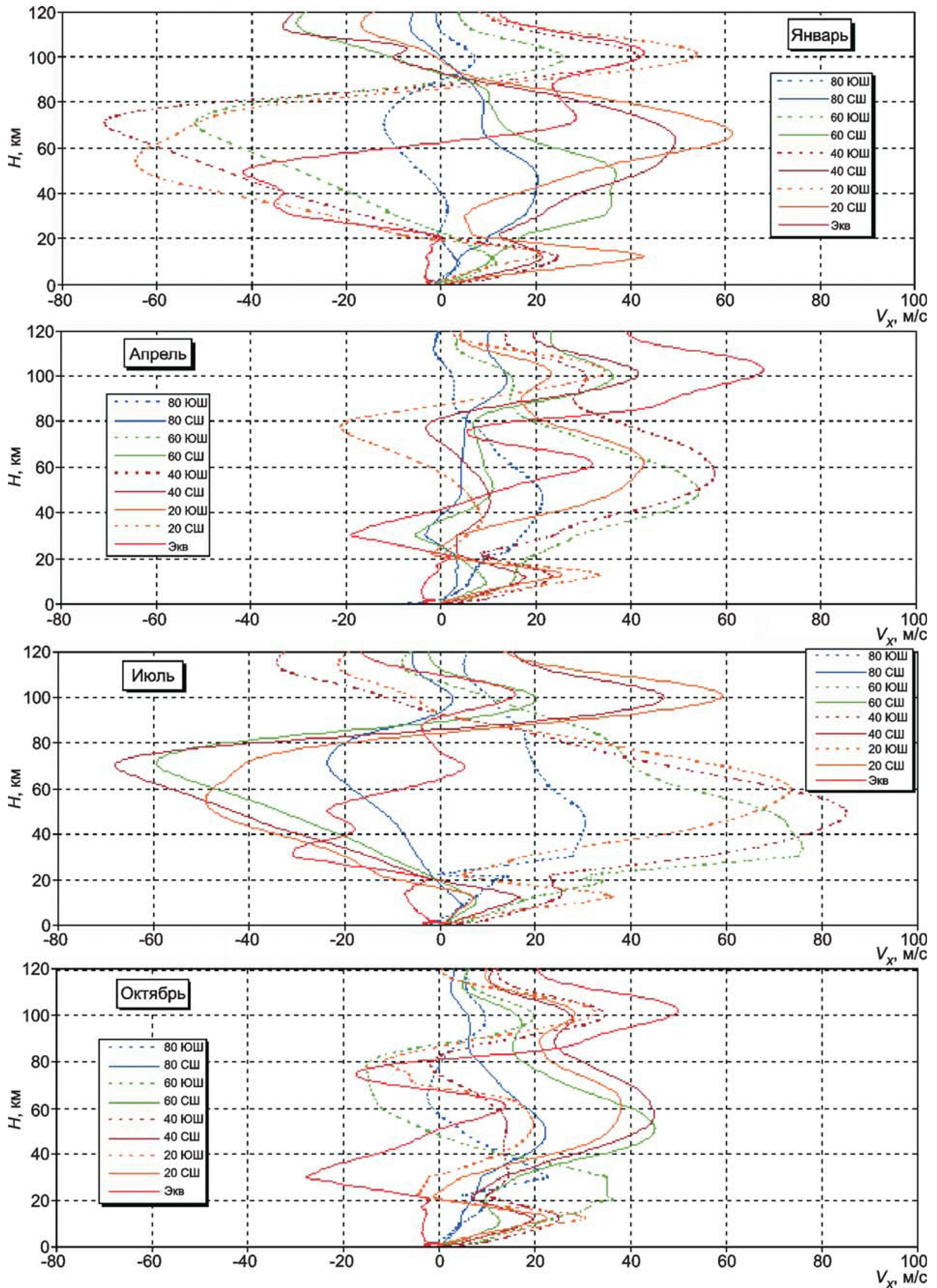
Рисунок А.19 — Вертикальные профили средних широтных значений зональной скорости ветра в атмосфере на разных широтах для центральных месяцев сезонов
