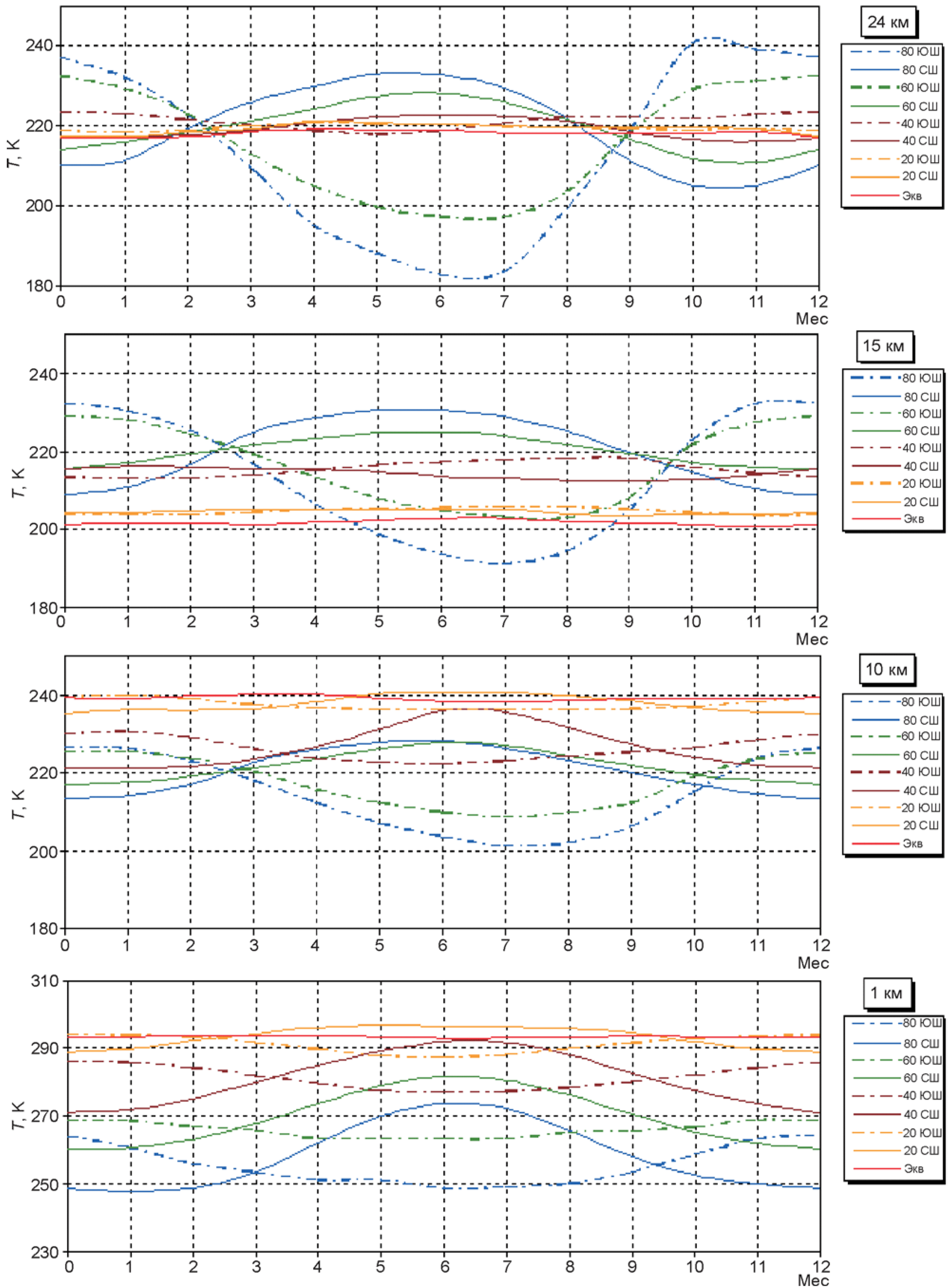
Рисунок А.6 — Внутригодовая изменчивость средних широтных значений температуры в атмосфере для различных широт и высот до 30 км
