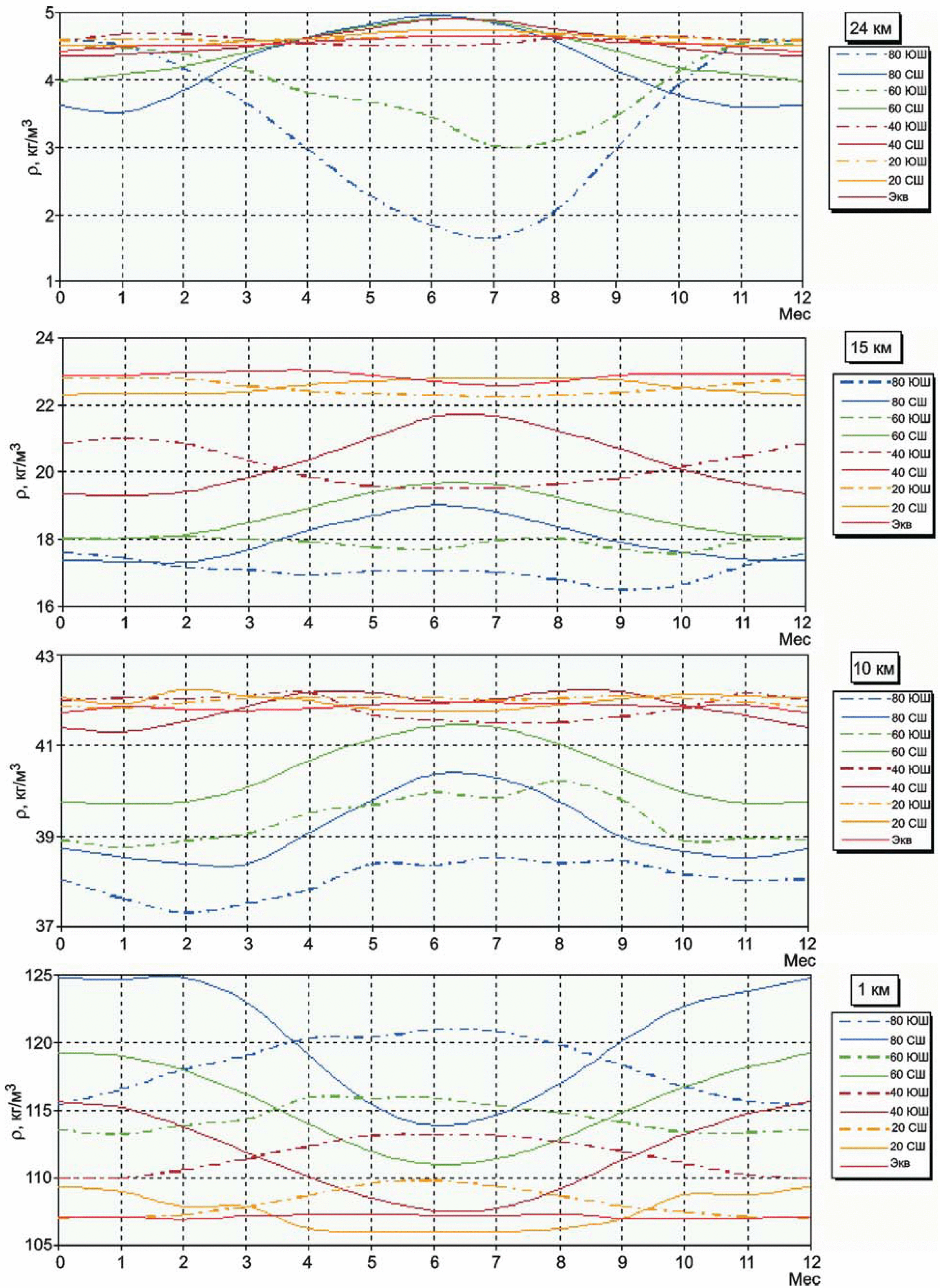
Рисунок А.12 — Средняя многолетняя внутригодовая изменчивость средних широтных значений плотности на разных широтах и высотах атмосферы до 30 км
