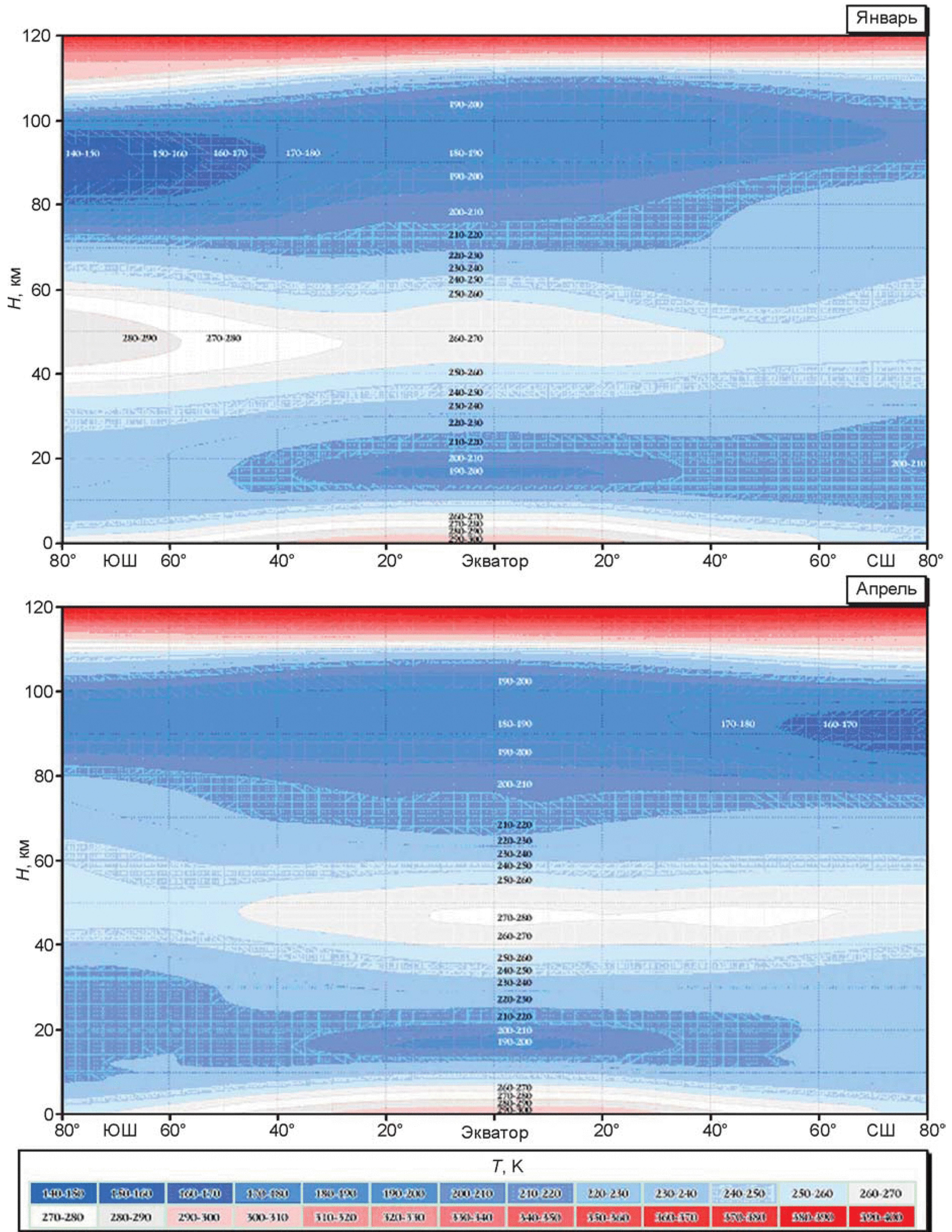
Рисунок А.2 — Изотермы средних широтных значений температуры в атмосфере на высотно-широтной сетке для центральных месяцев сезонов
