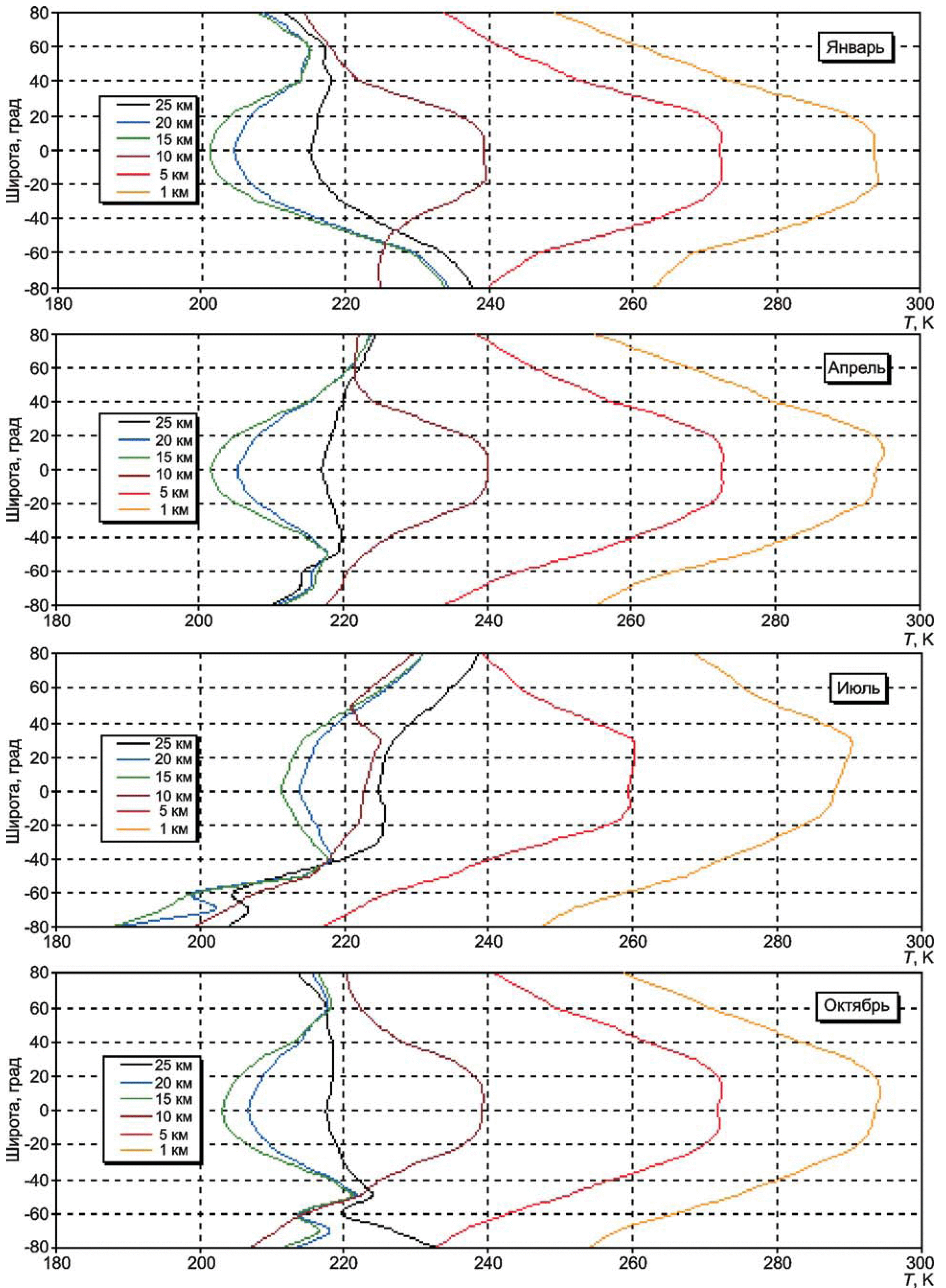
Рисунок А.4 — Вертикальные профили средних широтных значений температуры в атмосфере для различных широт и высот до 30 км для центральных месяцев сезонов
