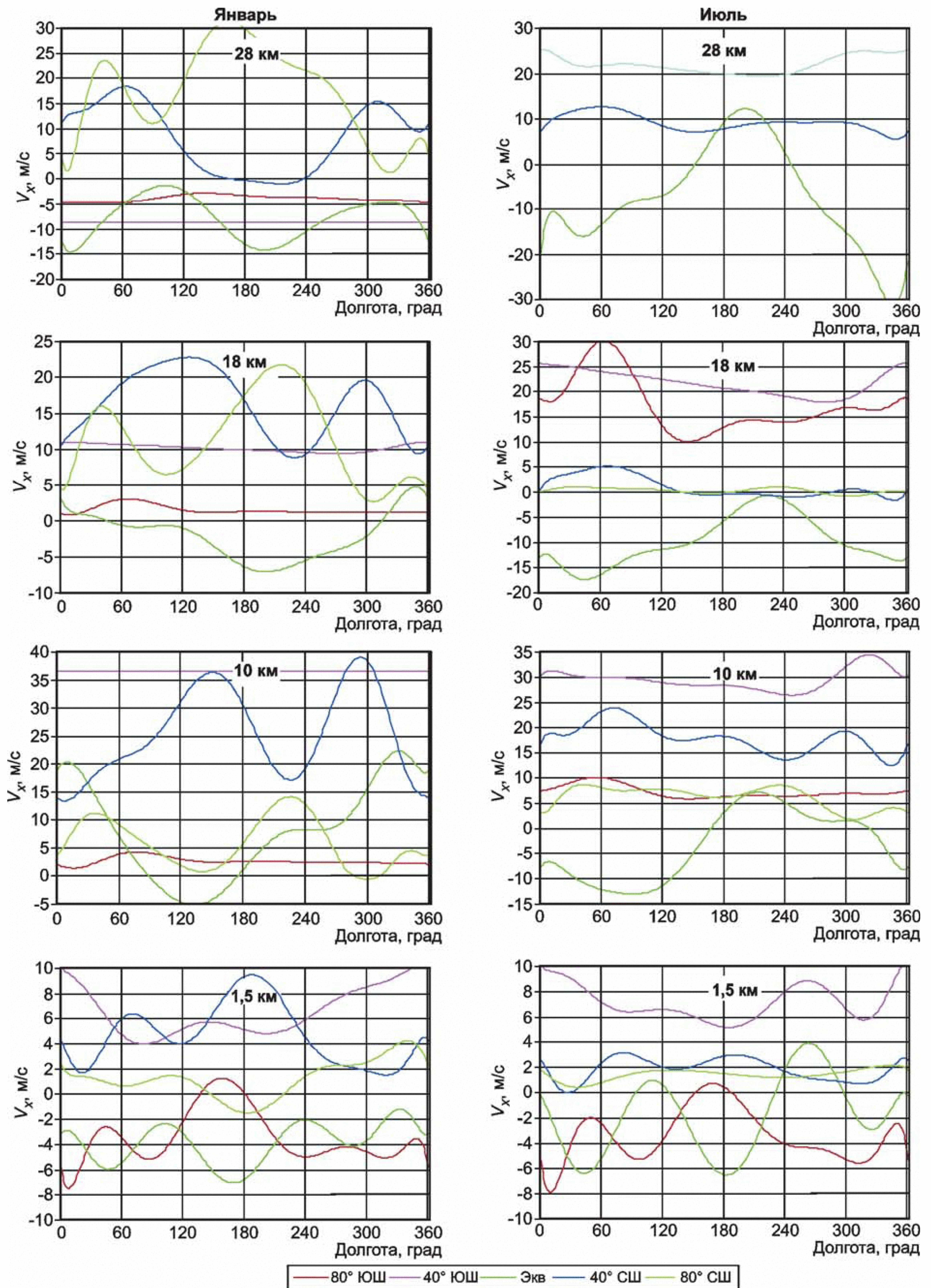
Рисунок Б.10 — Долготная изменчивость зональной скорости ветра при ее аппроксимации полиномом 10-й степени вдоль долготы на различных высотах атмосферы и в различных широтных поясах для января и июля
