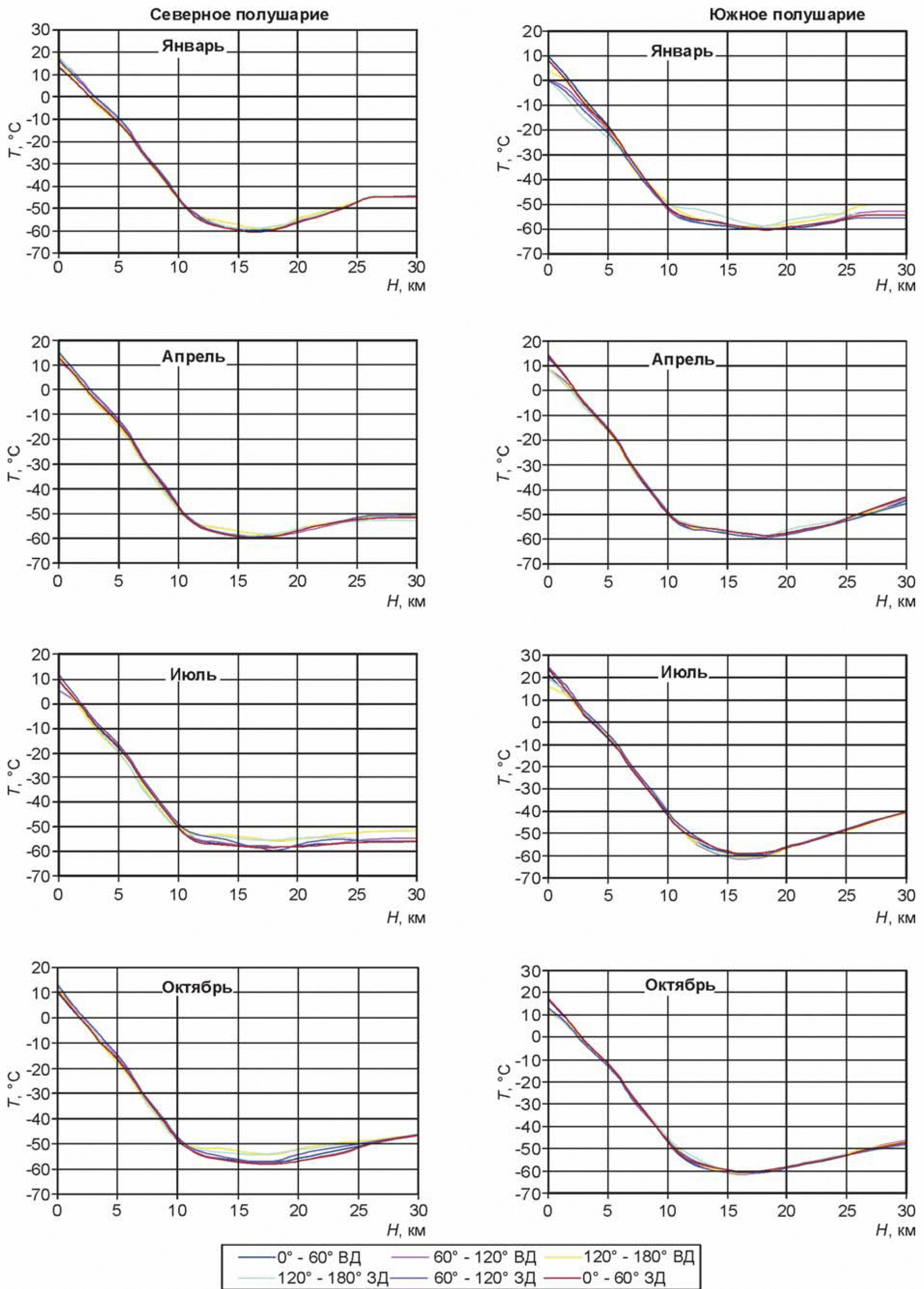
Рисунок Б.12 — Высотные профили температуры T при ее аппроксимации полиномом 10-й степени на высотах от 0 до 30 км на разной долготе в широтных поясах 35^\circ — 45^\circ в северном и южном полушариях
