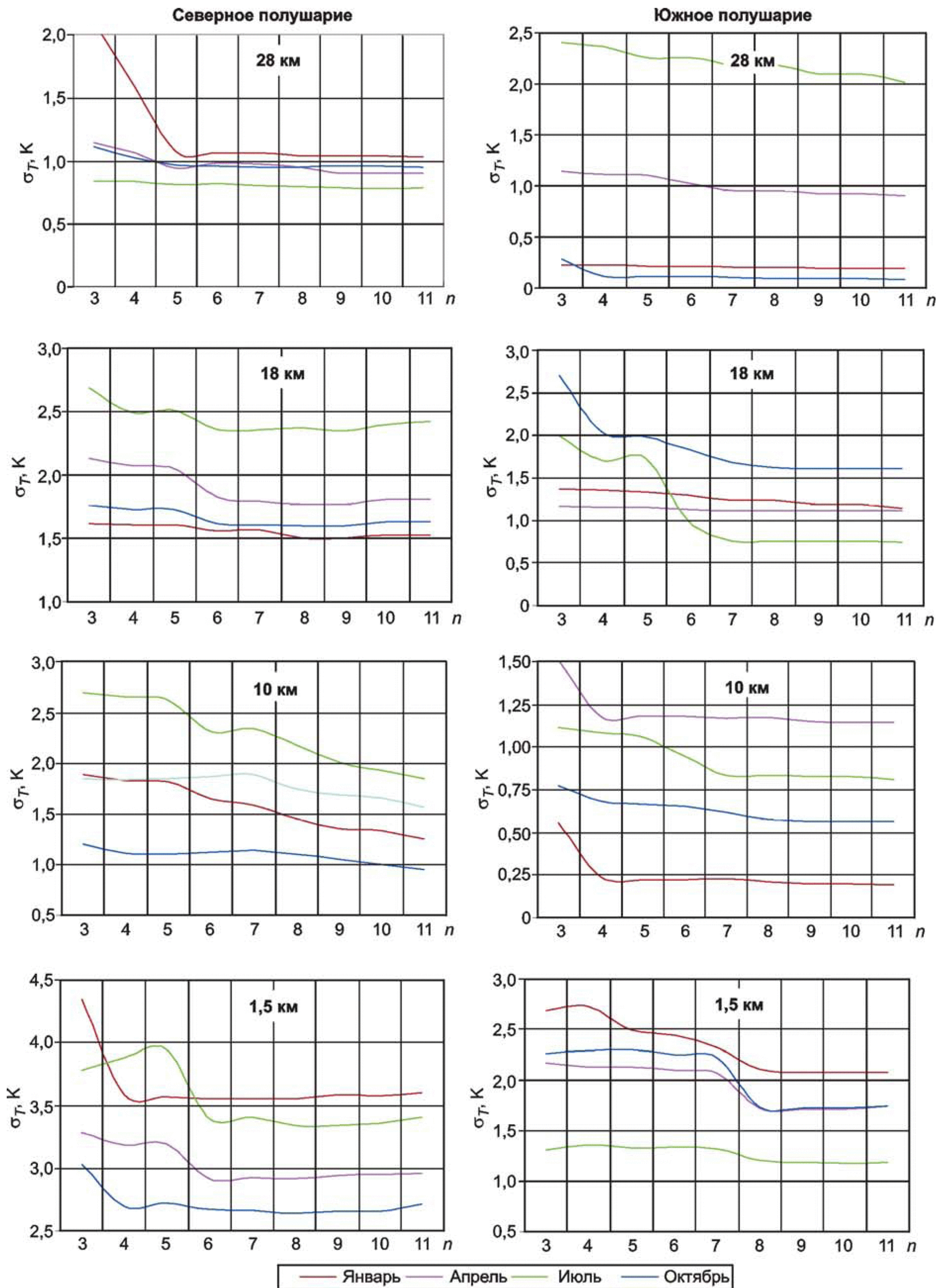
Рисунок Б.4 — Зависимость точности моделирования долготных вариаций температуры \sigma_T от степени аппроксимирующего полинома n на различных высотах нижней атмосферы в широтных поясах 35^\circ — 45^\circ в северном и южном полушариях
