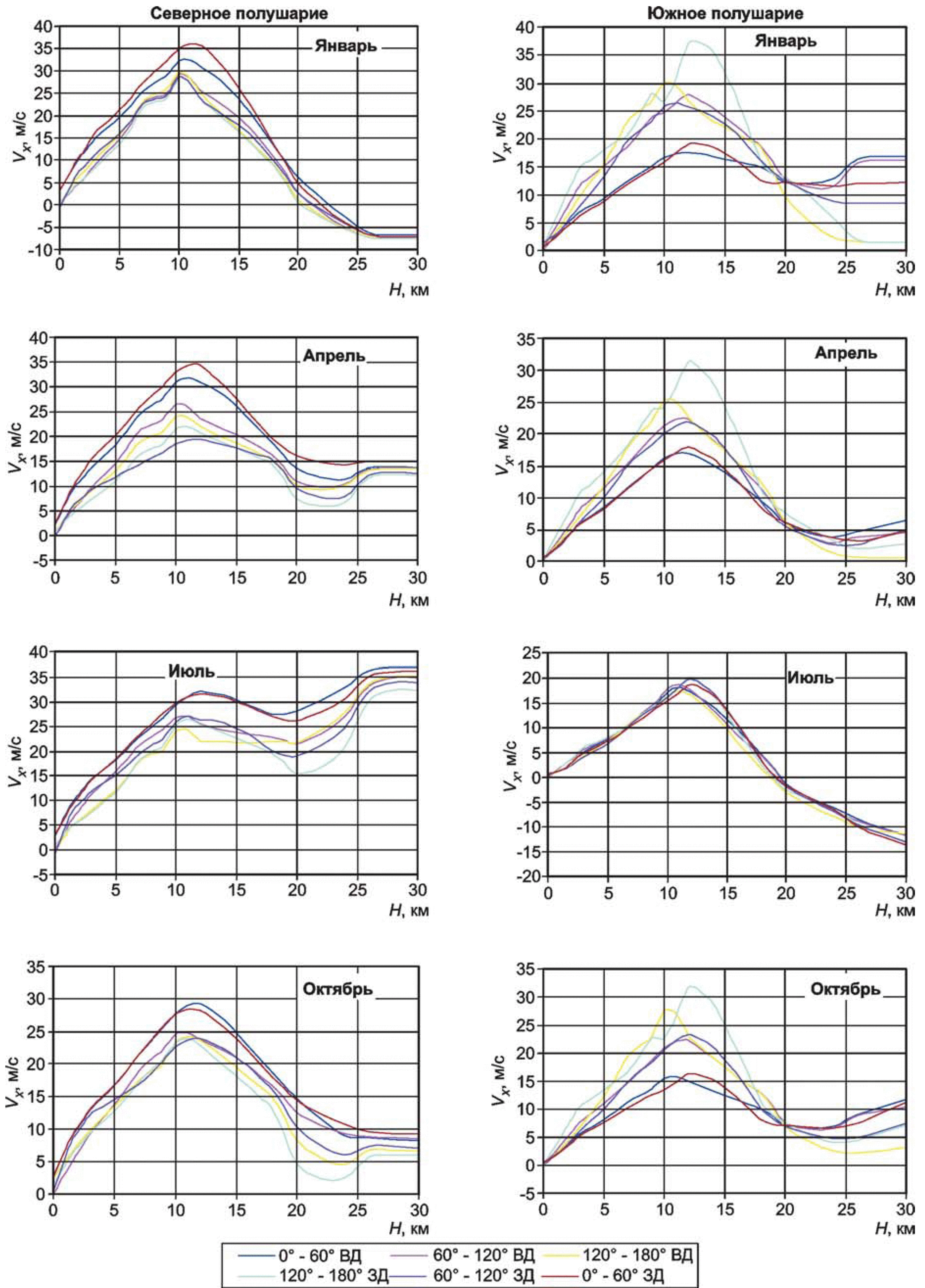
Рисунок Б.13 — Высотные профили зональной скорости ветра V_x при их аппроксимации полиномом 10-й степени на высотах от 0 до 30 км на разной долготе в широтных поясах 35^\circ - 45^\circ в северном и южном полушариях
