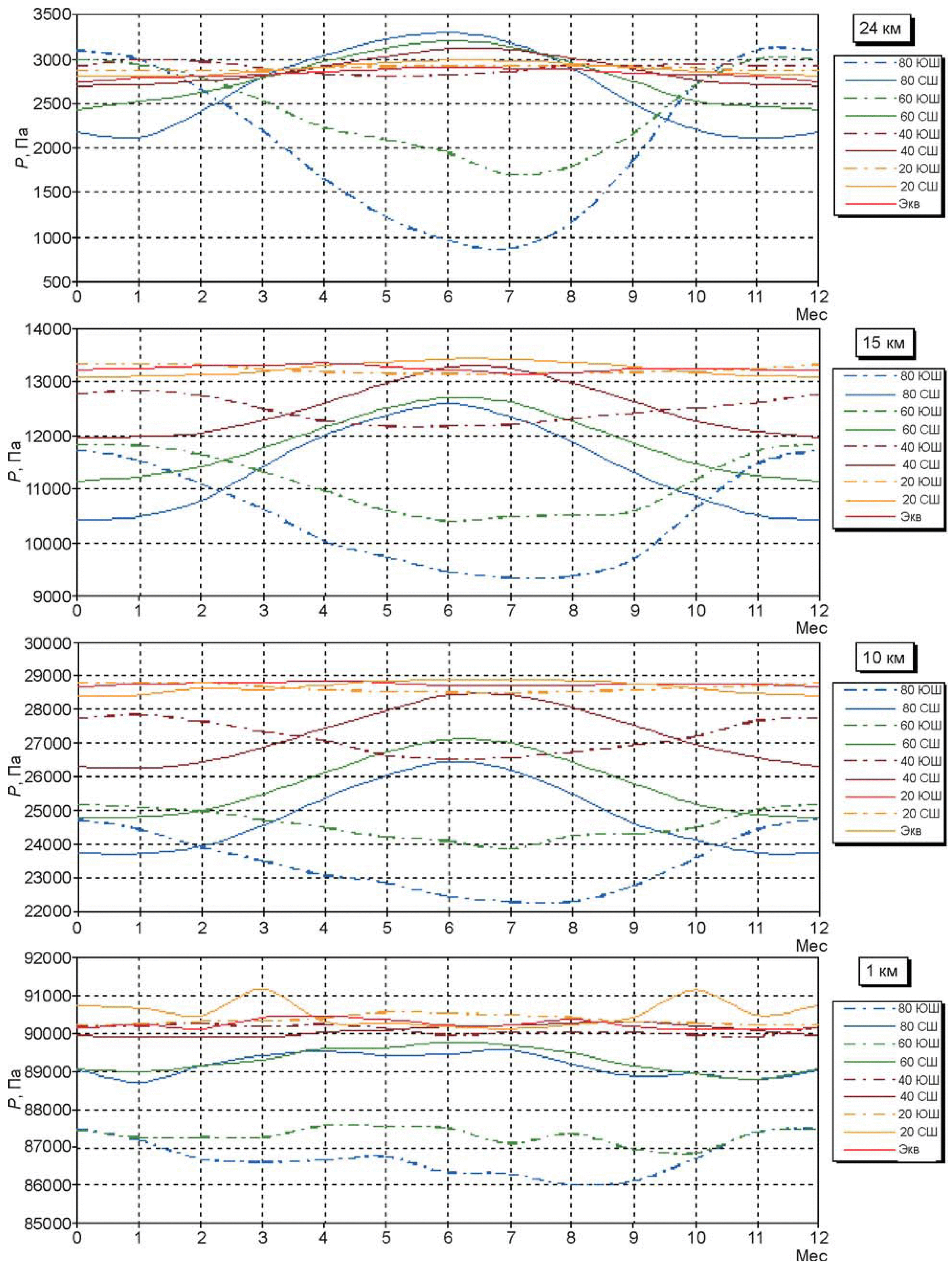
Рисунок А.9 — Средняя многолетняя внутригодовая изменчивость средних широтных значений давления на различных широтах и высотах атмосферы до 30 км
