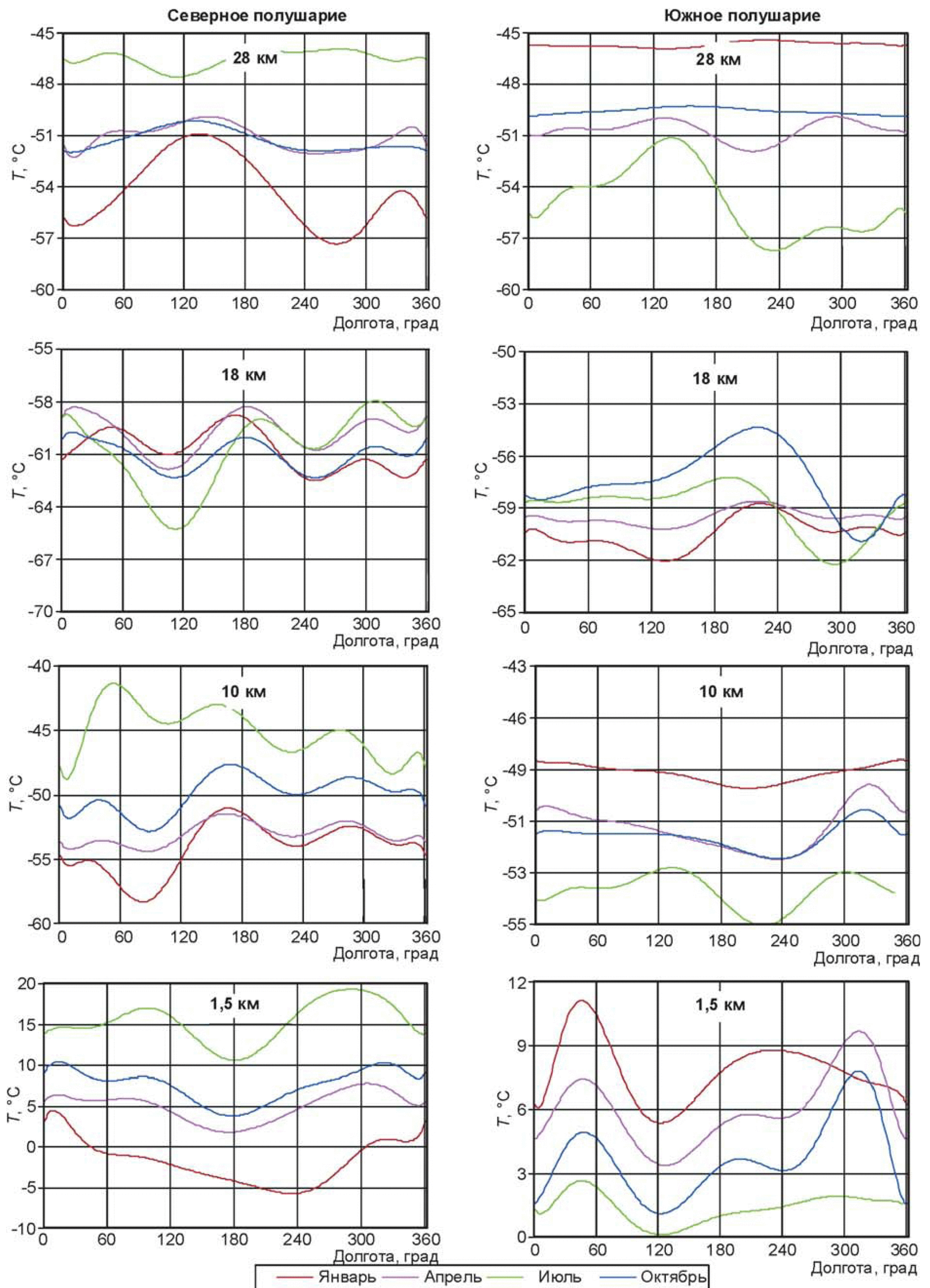
Рисунок Б.6 — Долготная изменчивость температуры T при ее аппроксимации полиномом 10-й степени вдоль долготы на различных высотах атмосферы в широтных поясах 35^\circ — 45^\circ в северном и южном полушариях
