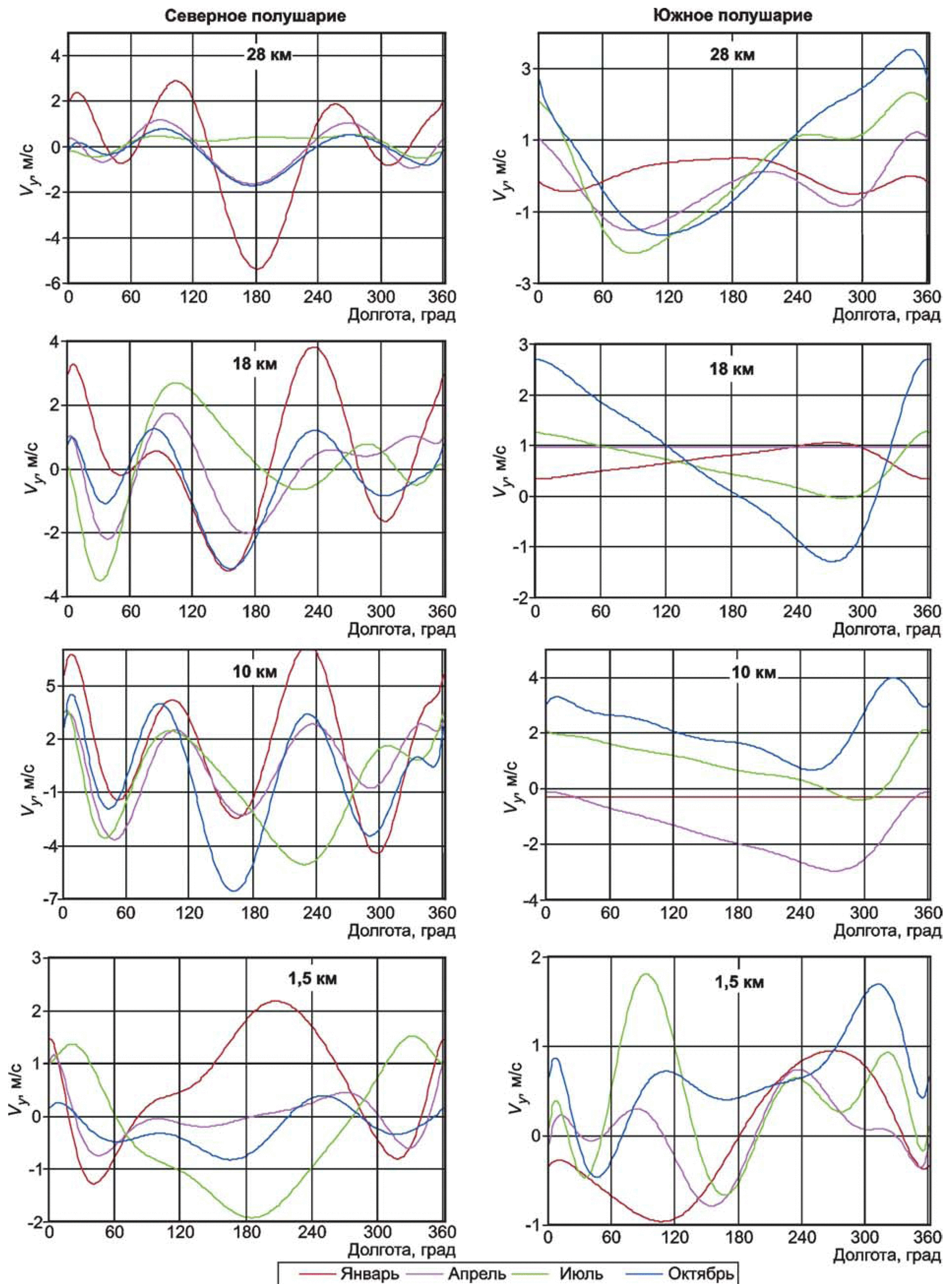
Рисунок Б.8 — Долготная изменчивость меридиональной скорости ветра при ее аппроксимации полиномом 10-й степени вдоль долготы на различных высотах в широтных поясах 35^\circ — 45^\circ в северном и южном полушариях
