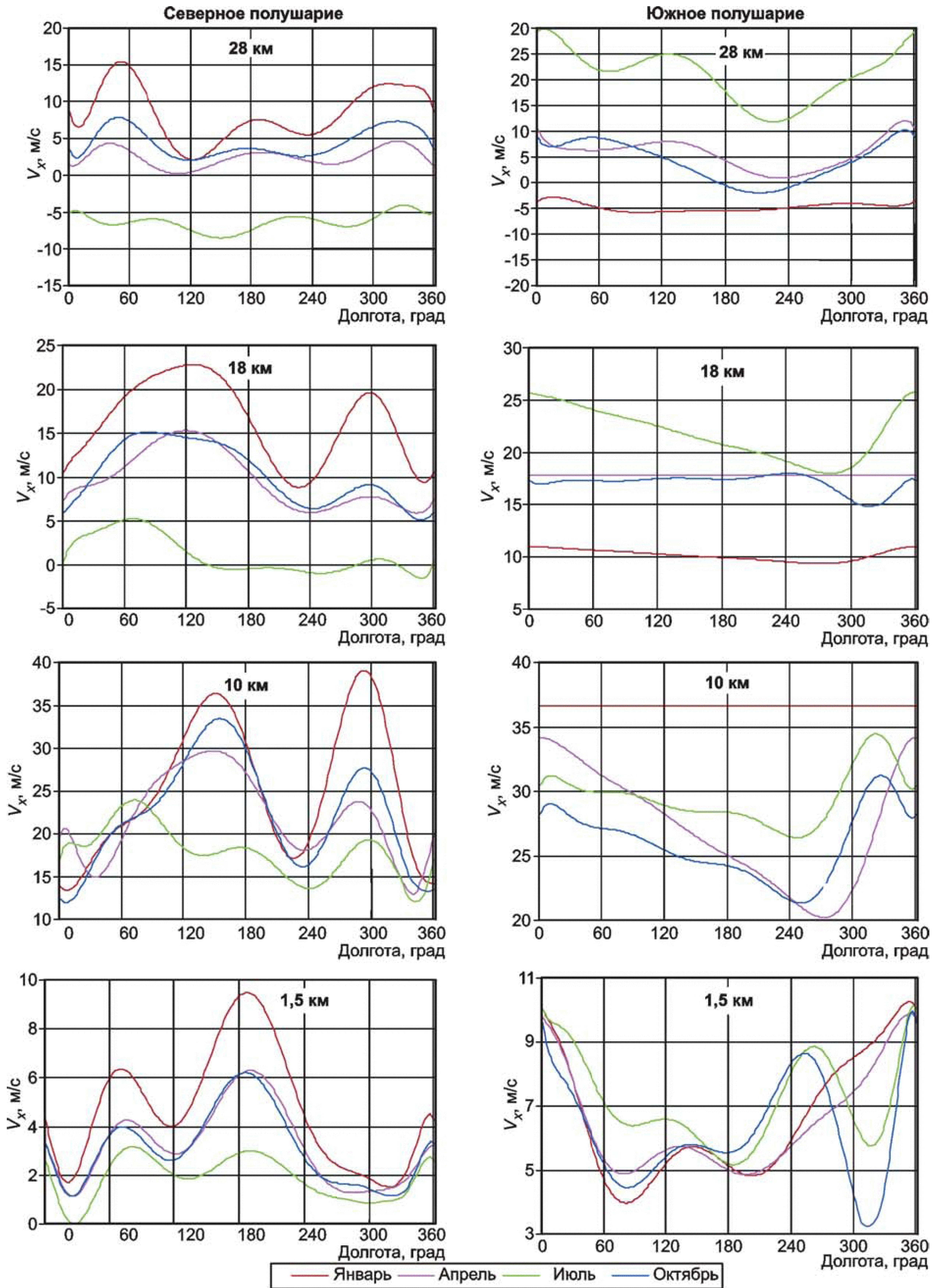
Рисунок Б.7 — Долготная изменчивость зональной скорости ветра при ее аппроксимации полиномом 10-й степени вдоль долготы на различных высотах в широтных поясах 35^\circ — 45^\circ в северном и южном полушариях
