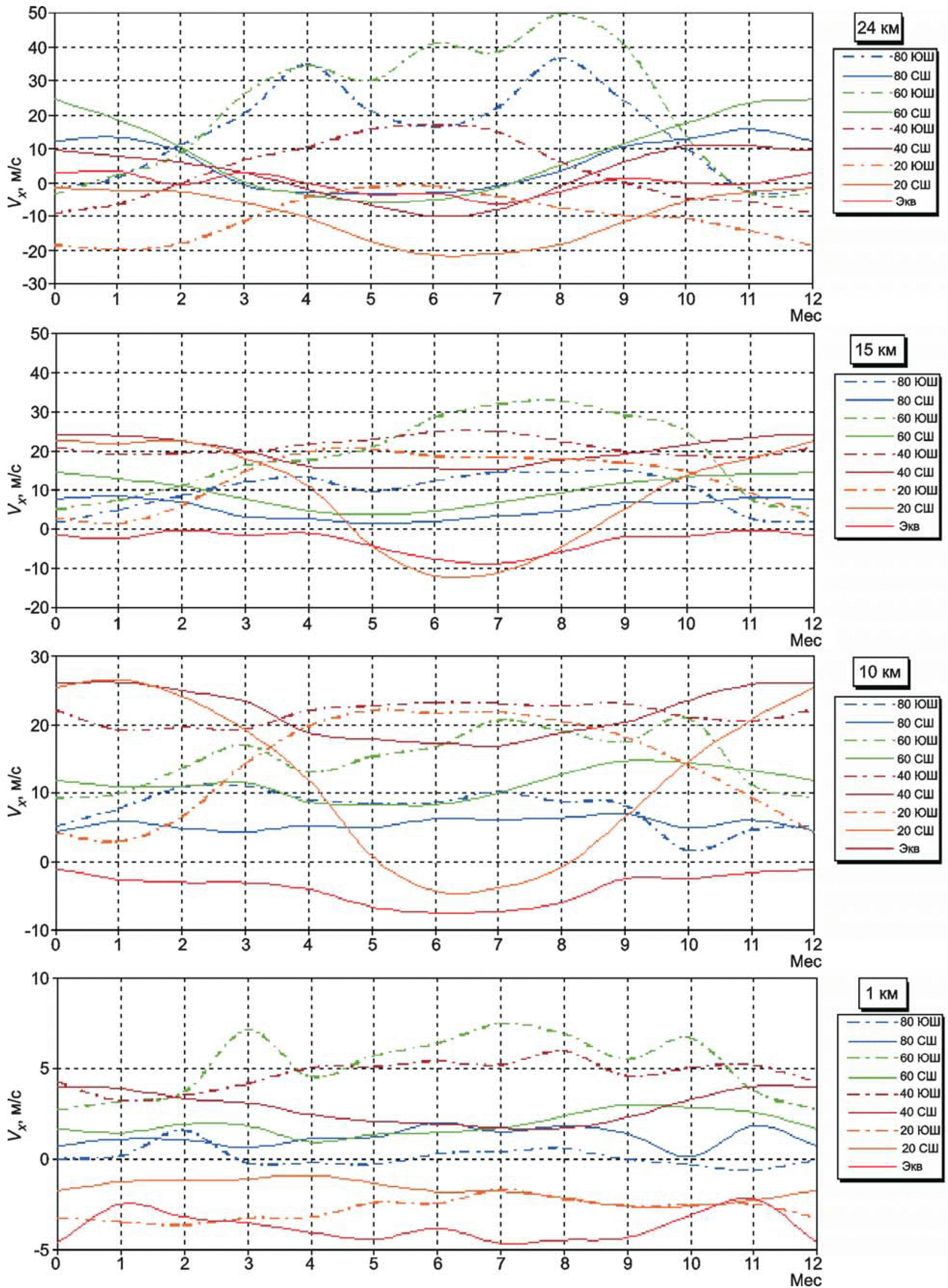
Рисунок А.15 — Средняя многолетняя внутригодовая изменчивость средних широтных значений зональной скорости ветра на различных широтах и высотах до 30 км
