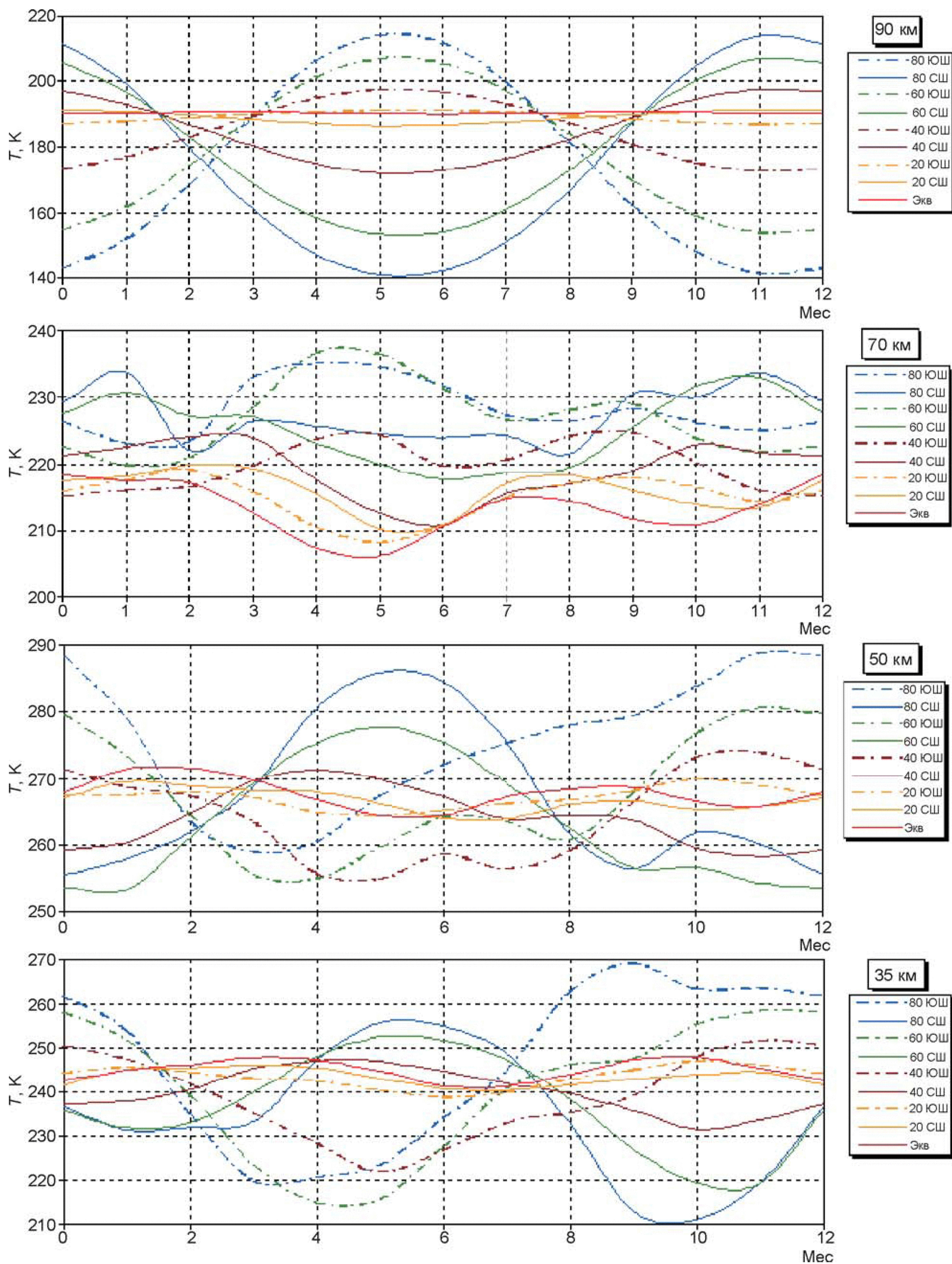
Рисунок А.7 — Внутригодовая изменчивость средних широтных значений температуры в атмосфере для различных широт и высот от 30 до 120 км
