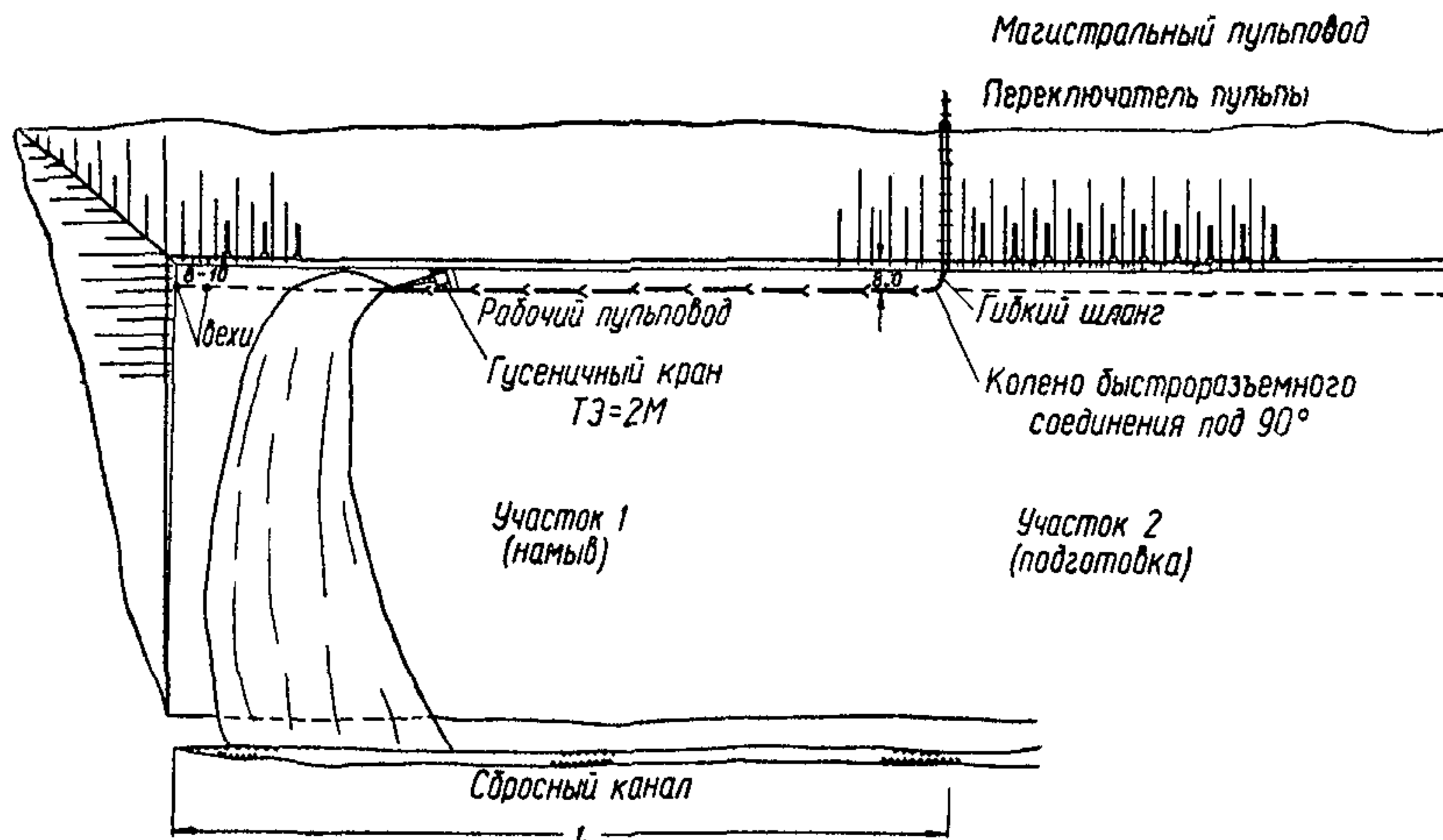
Рис. 4 Схема организации намыва
