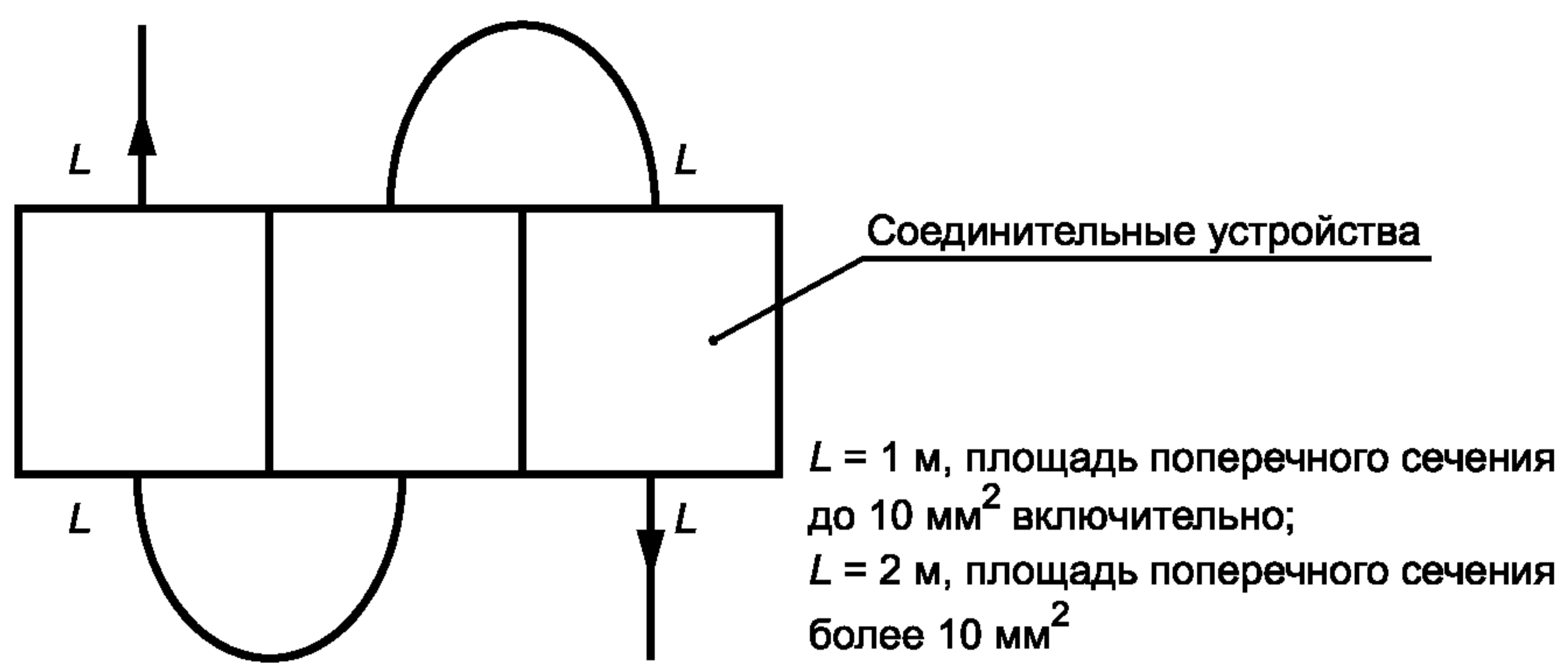
Рисунок 102 — Зажим на несколько направлений
