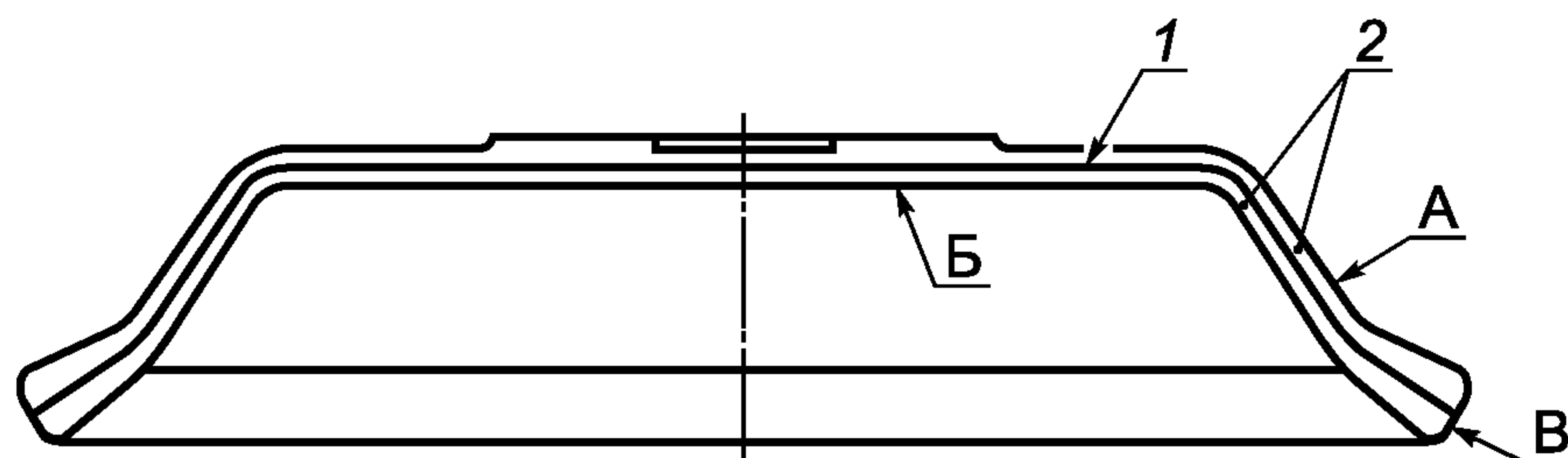
А, Б — поверхности тела мембраны, В — поверхность торца бурта мембраны, 1 — ткань, 2 — резина
