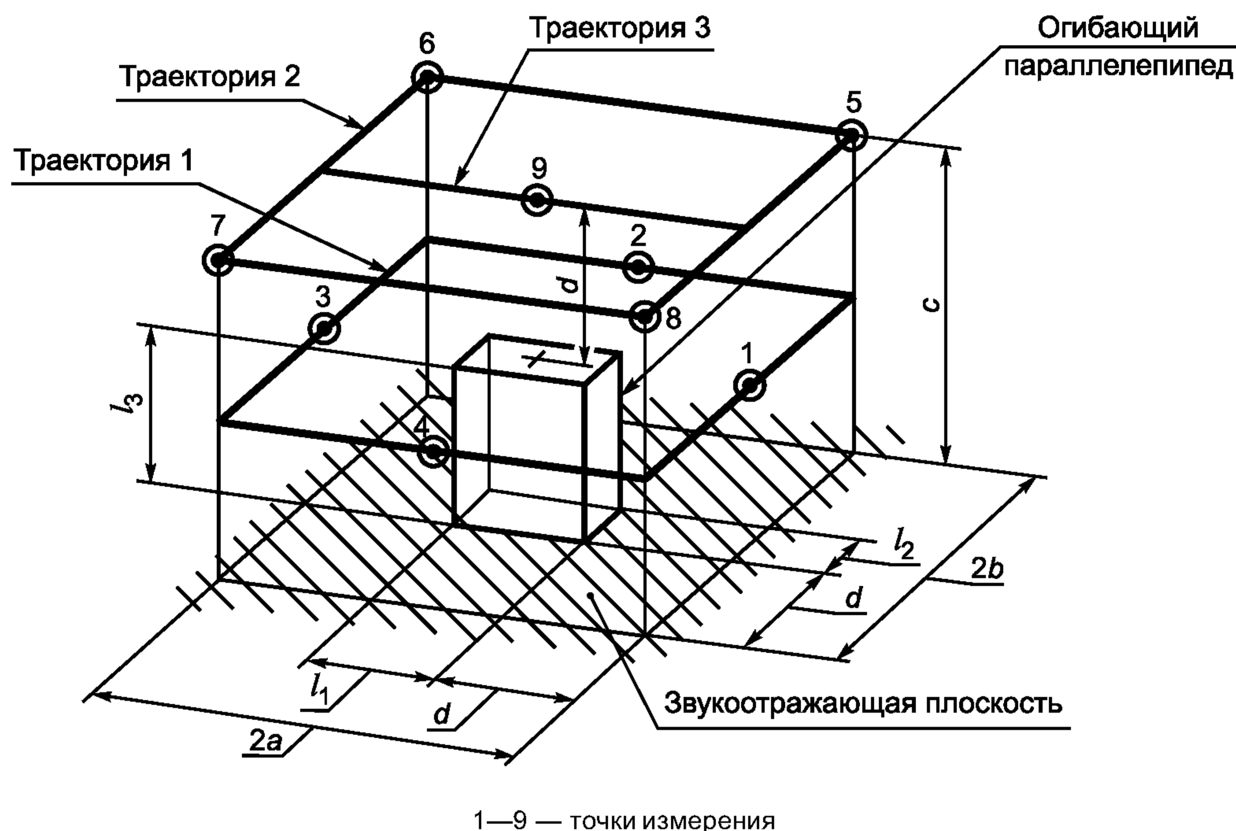
Рисунок 1 — Пример измерительной поверхности и положений (траекторий) микрофонов
