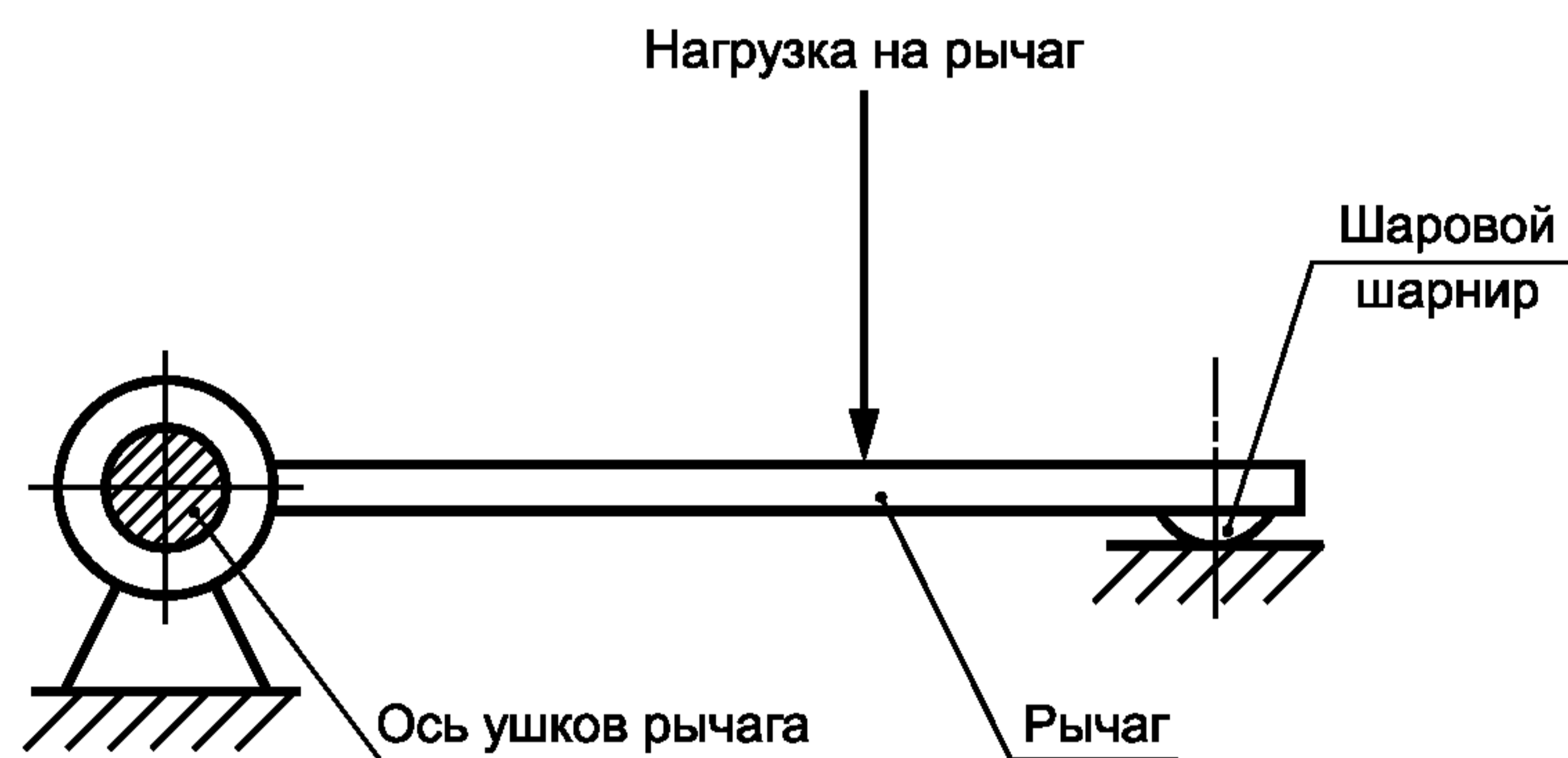
Рисунок 2 — Схема испытаний рычагов на прочность
