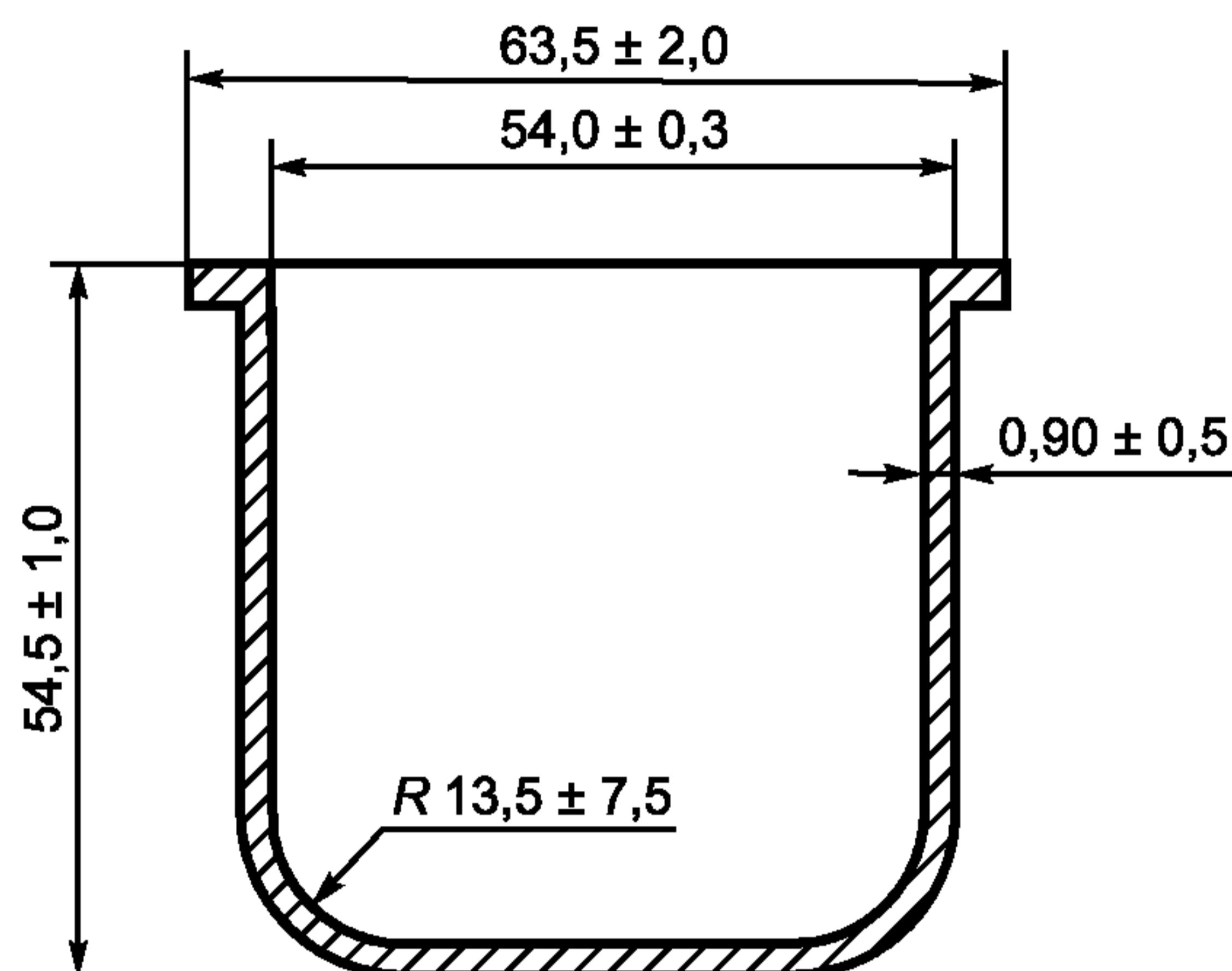
Рисунок А1.1 — Испытательный тигель
