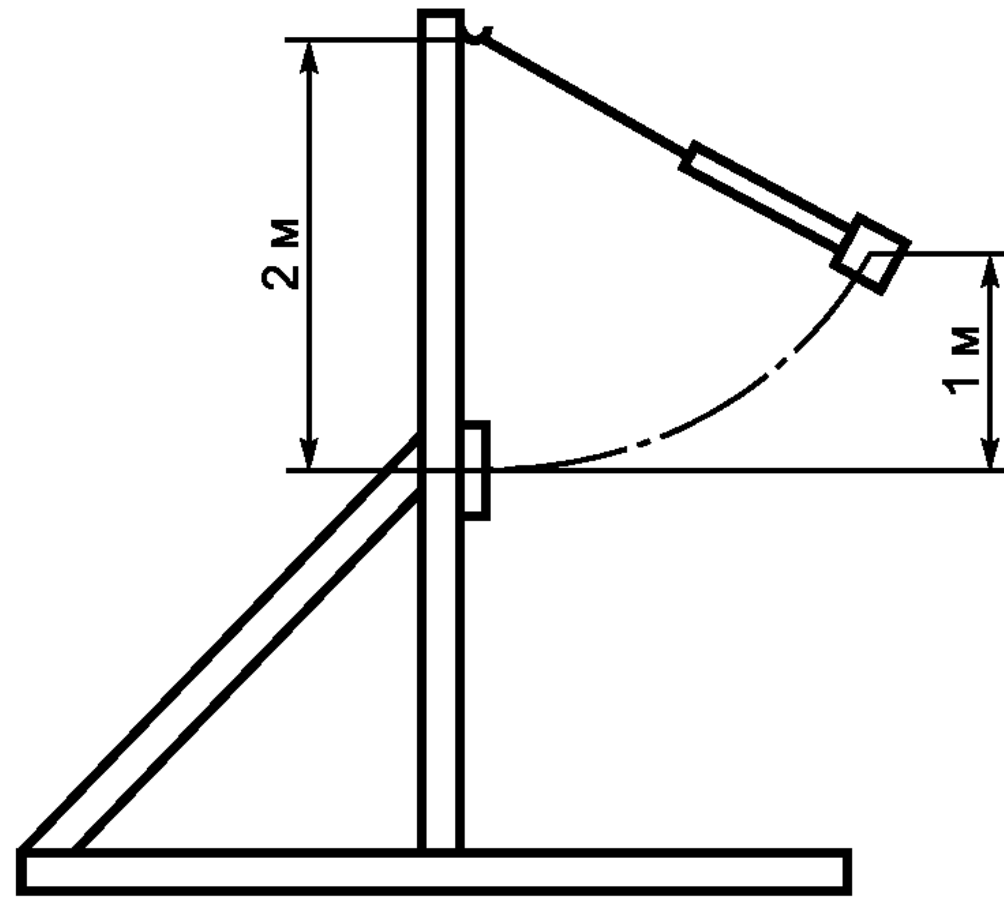
Рисунок А.1 — Испытание на механический удар
