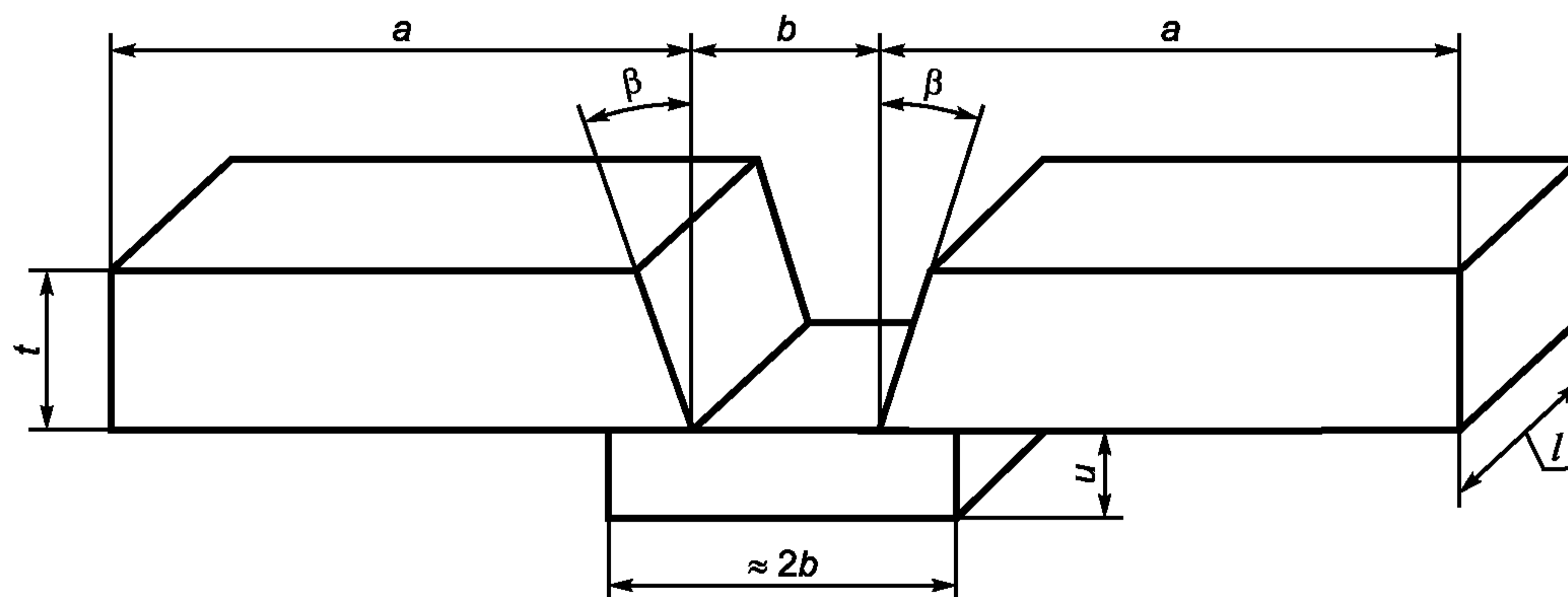
Рисунок 1 — Размеры контрольного соединения
