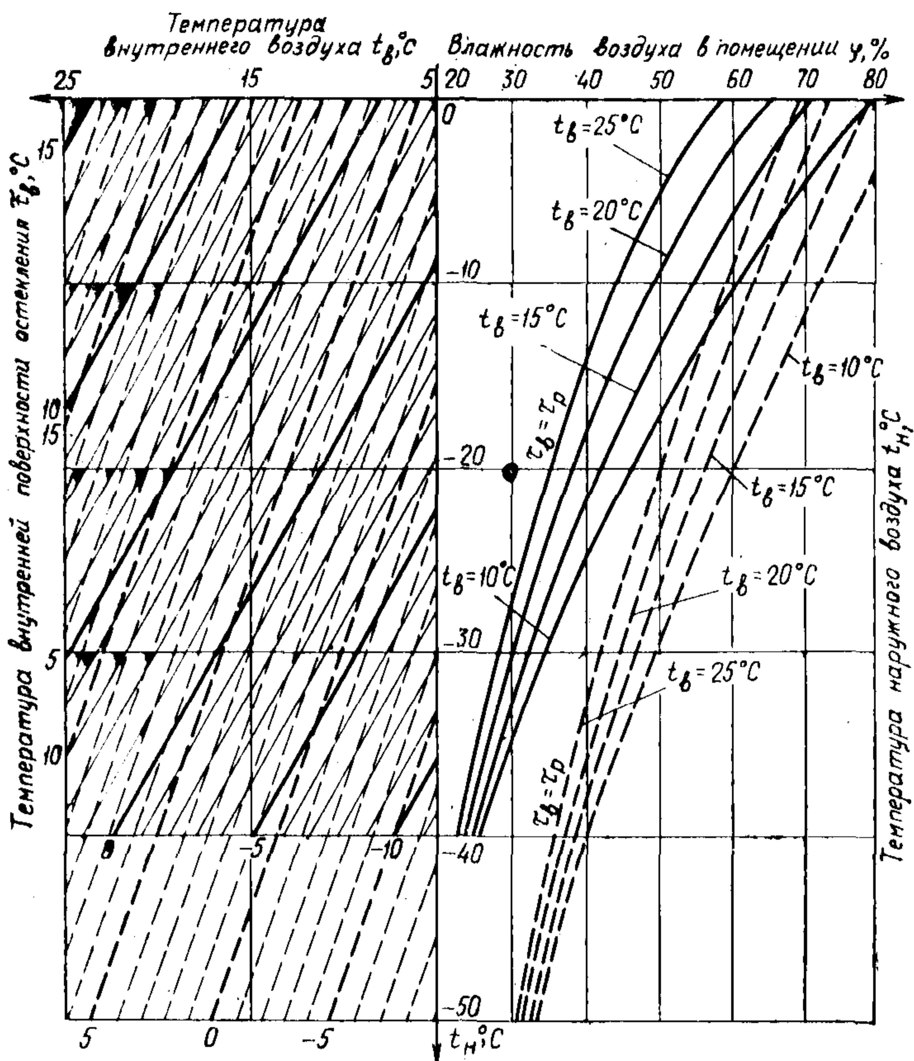
Рис 2. Номограмма для определения температур \tau_b , \tau_p и допустимых значений t_n , \varphi при теплотехнических расчетах окон с применением стеклопакетов
