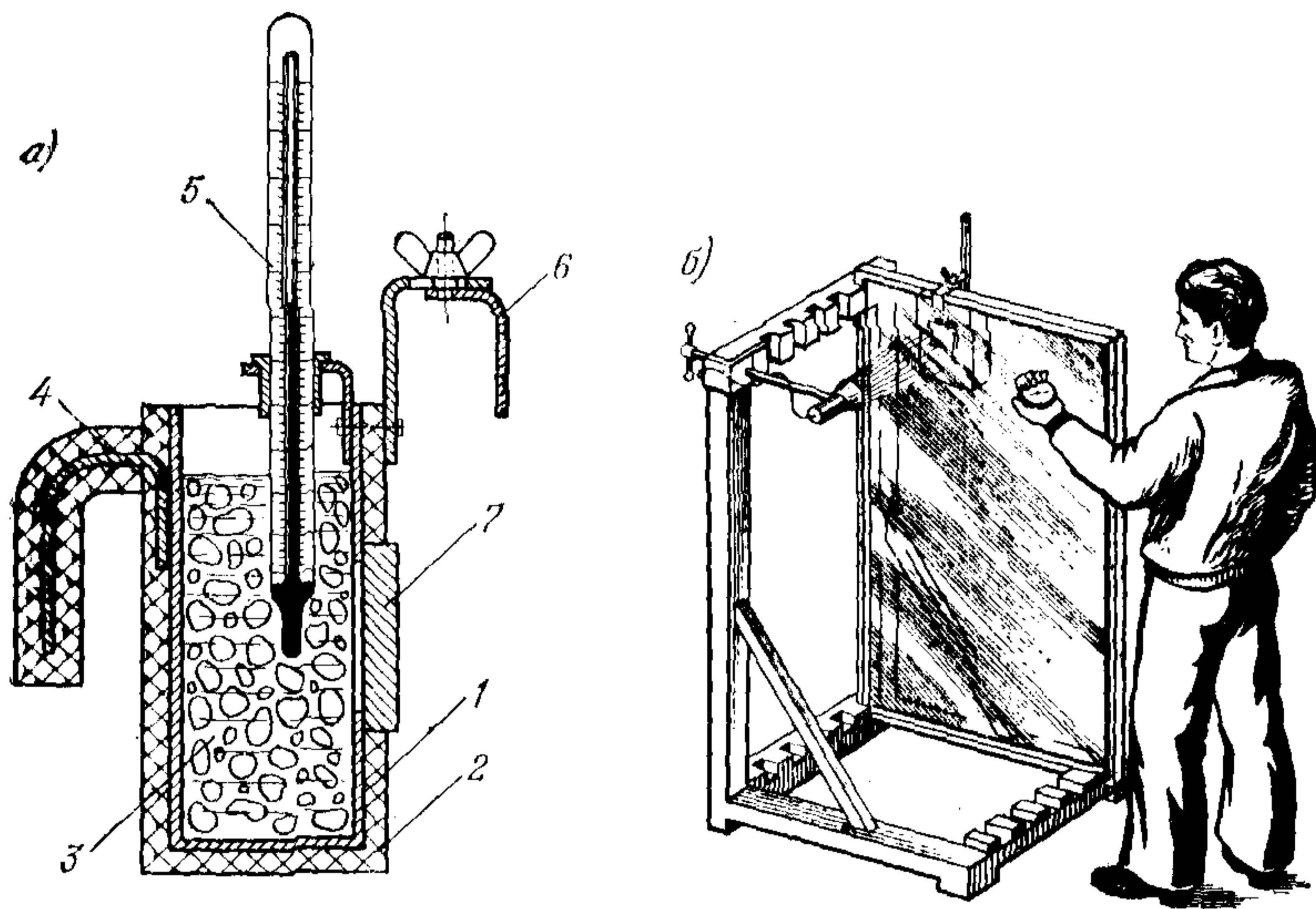
Рис. 14. Контроль точки росы в воздушной прослойке стеклопакета
