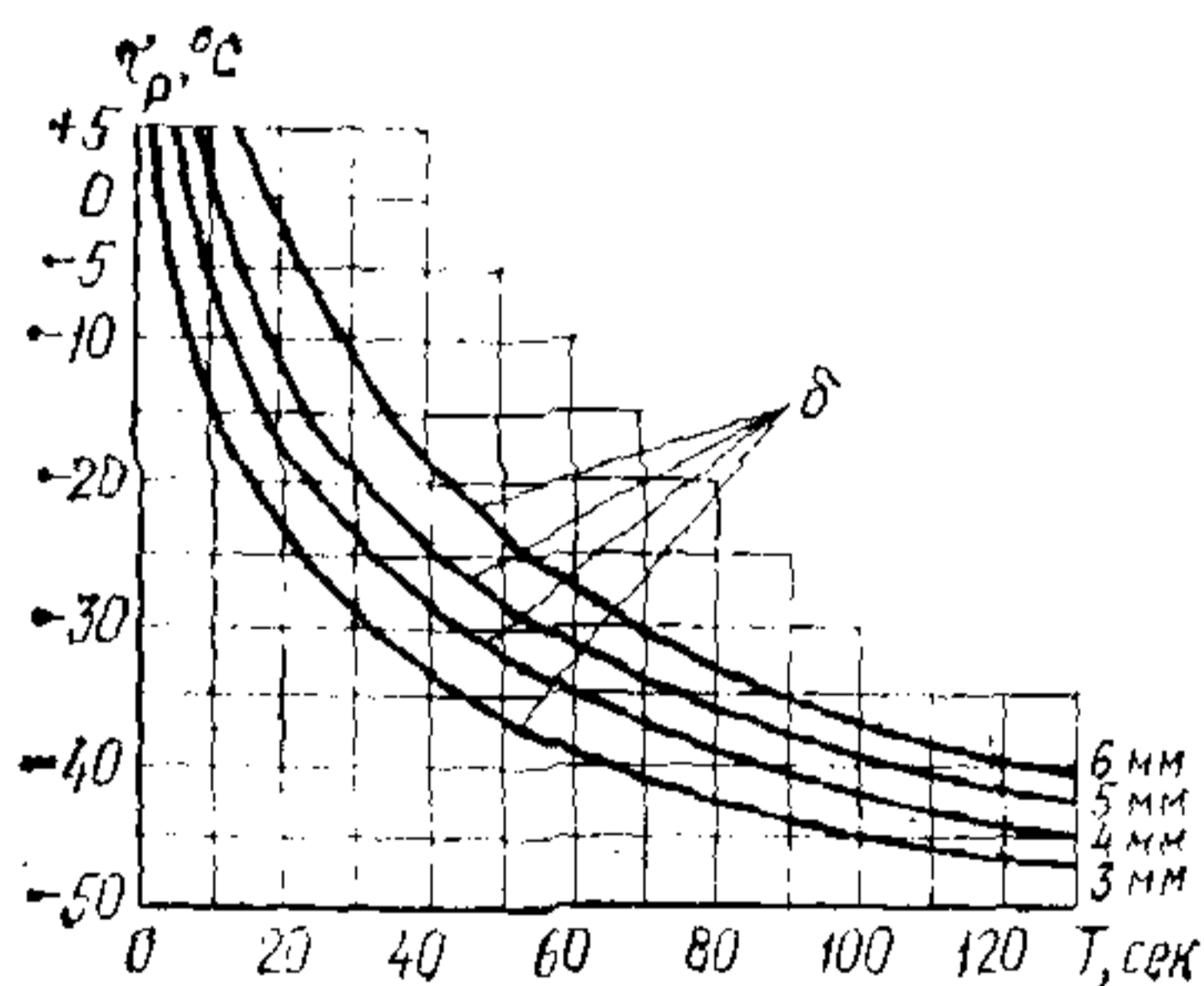
Рис. 15. График для определения точки росы \tau_p в зависимости от времени обнаружения инея T и толщины стекла \delta в стеклопакете
