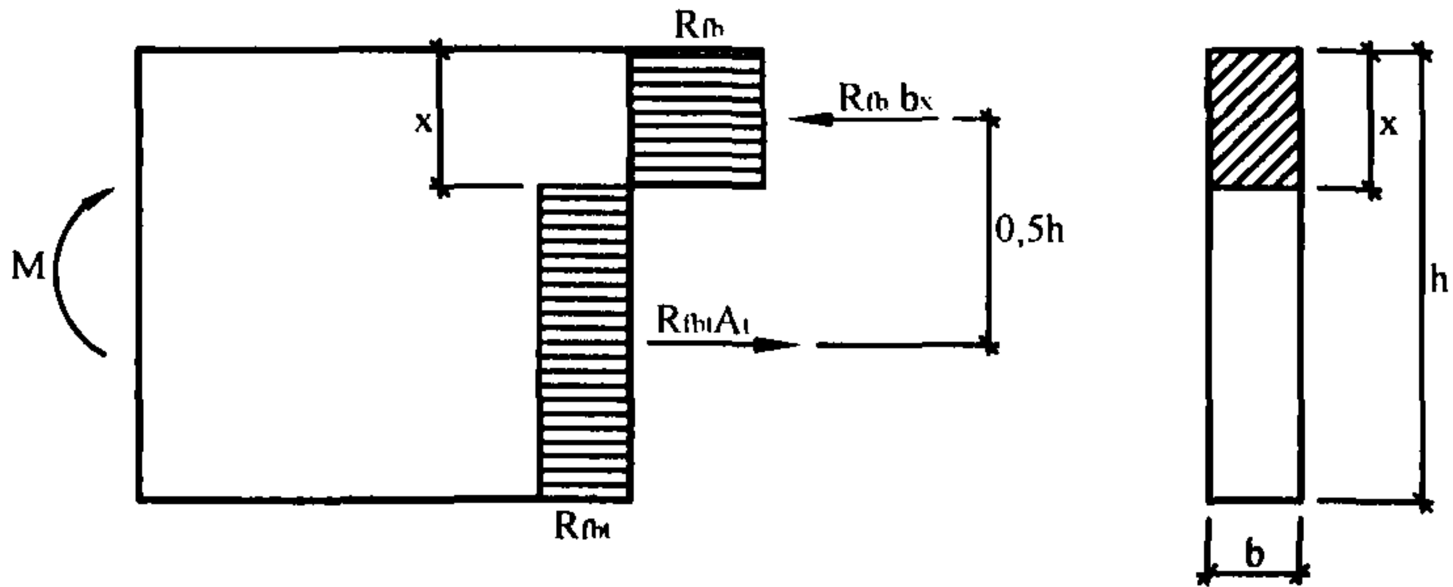
Рис.1. Схема внутренних усилий и эпюры напряжений в сечении, нормальном к продольной оси элемента (общий случай) l - сосредоточенная стержневая или проволочная арматура
