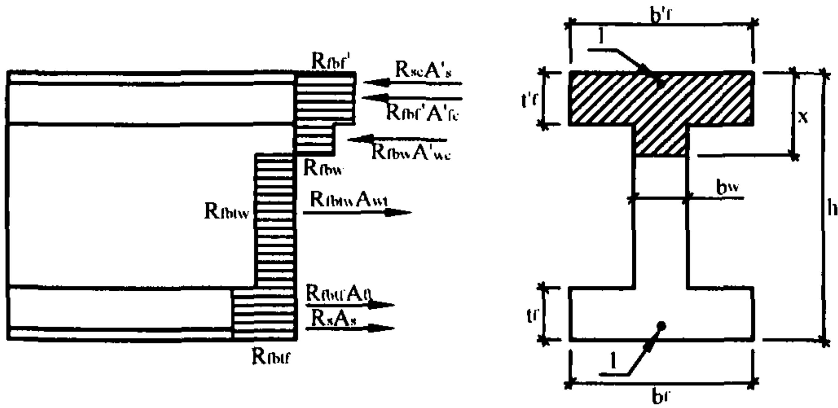
Рис.1. Схема внутренних усилий и эпюры напряжений в сечении, нормальном к продольной оси элемента (общий случай) l - сосредоточенная стержневая или проволочная арматура
