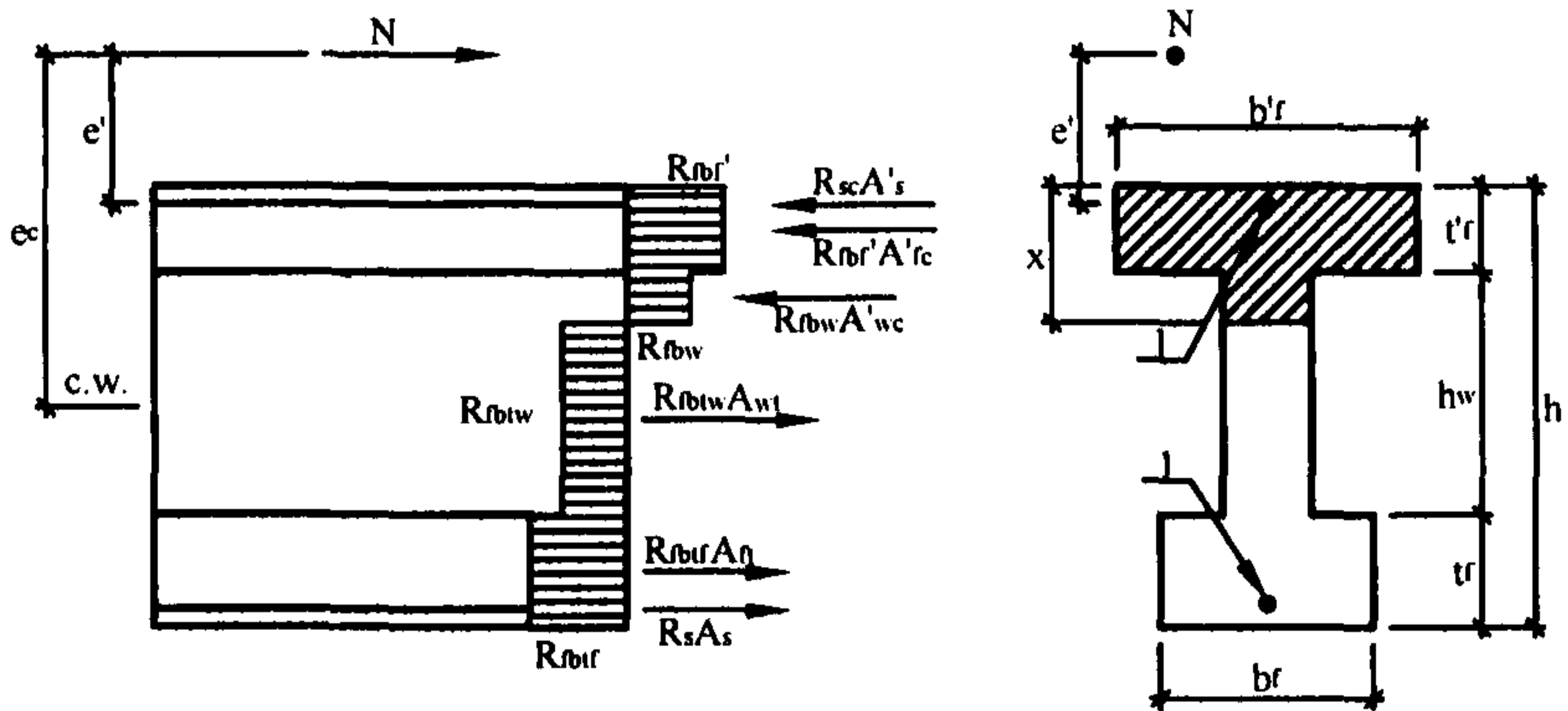
Рис.6. Схема усилий и эпюра напряжений во внецентренно сжатых элементах двутаврового сечения при комбинированном армировании при x > t'_f
