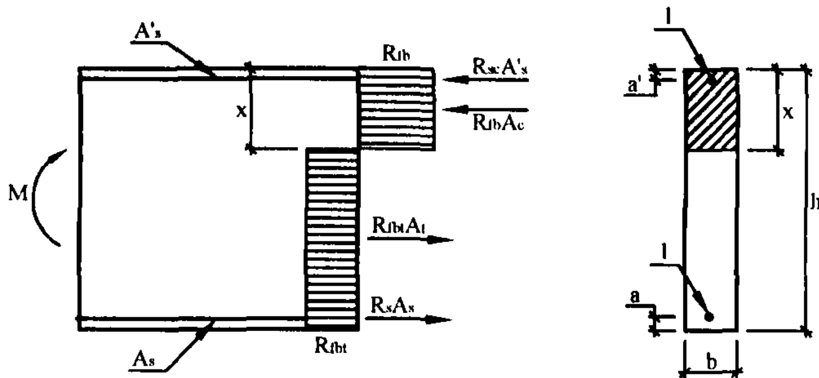
Рис.3. Схема усилий и эпюра напряжений в сечениях, нормальных к продольной оси изгибаемого железобетонного элемента прямоугольного сечения при комбинированном армировании l - стержневая или проволочная арматура
