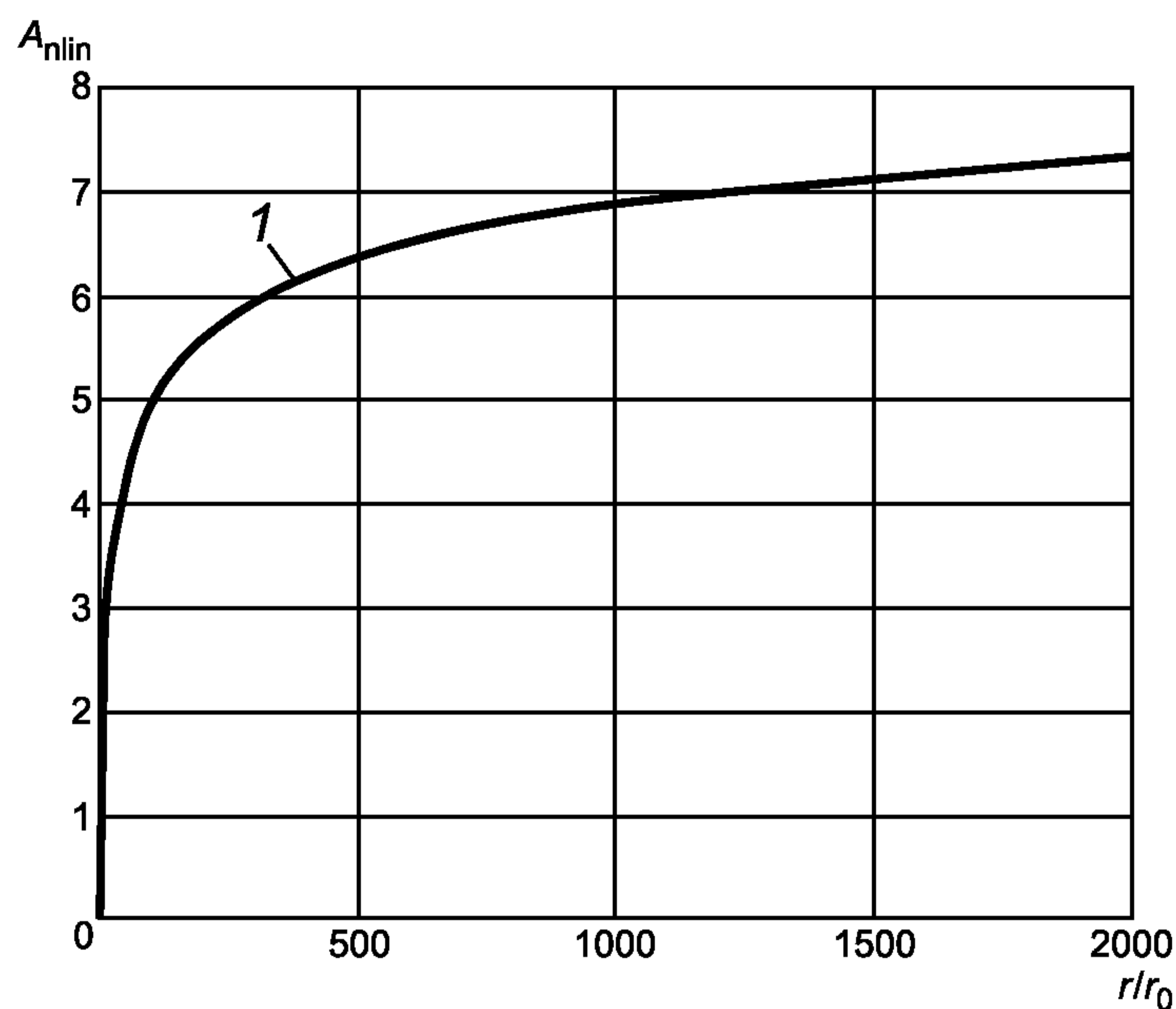
1 — M = 1,3 ; r_0 = 1 м; k = 0,8/340 м -1 ; A_{\text{нlin}} — нелинейное затухание, дБА; r — расстояние от точки источника до точки наблюдения, м
