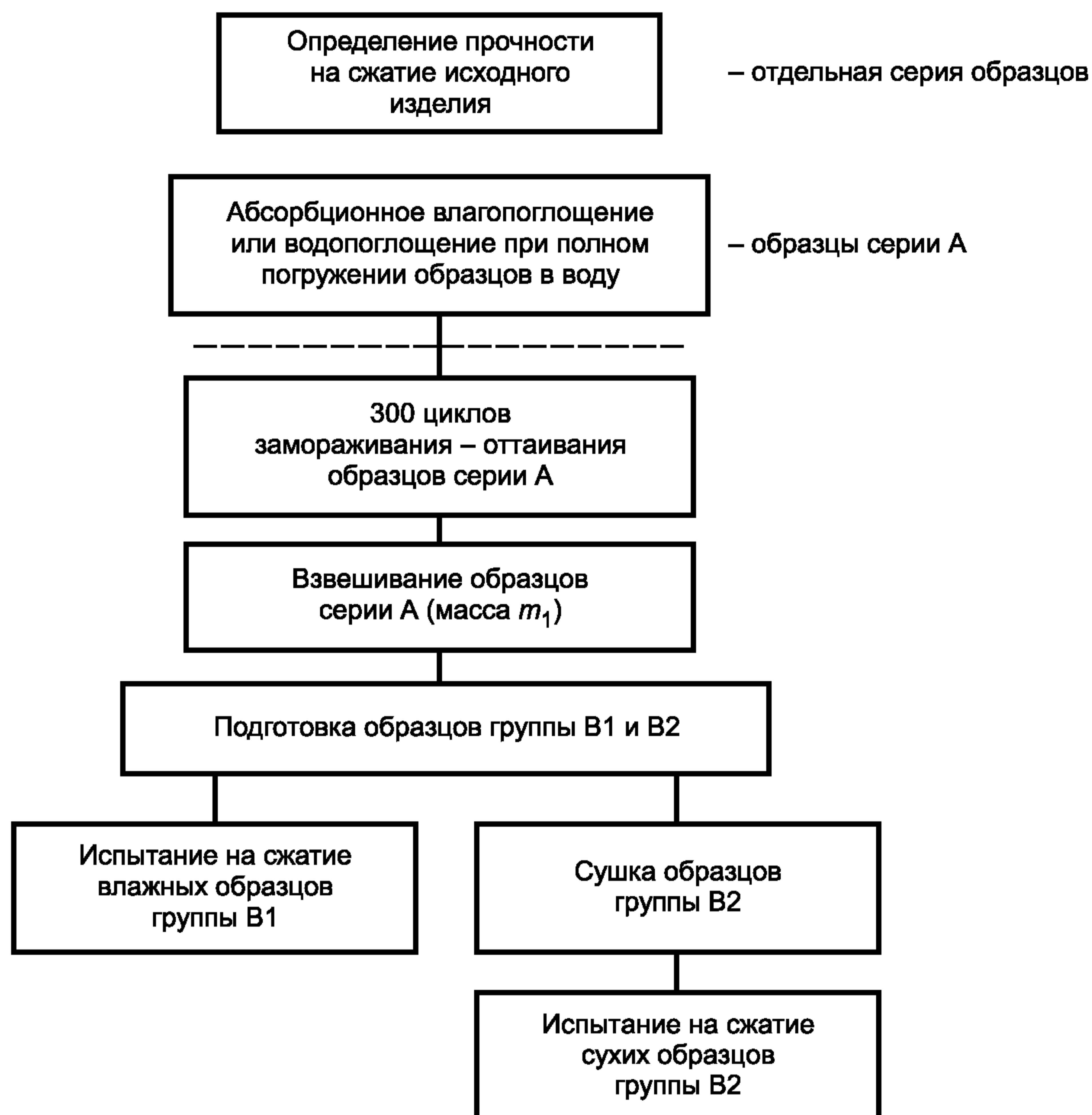
Рисунок 1 — Схема проведения испытания
