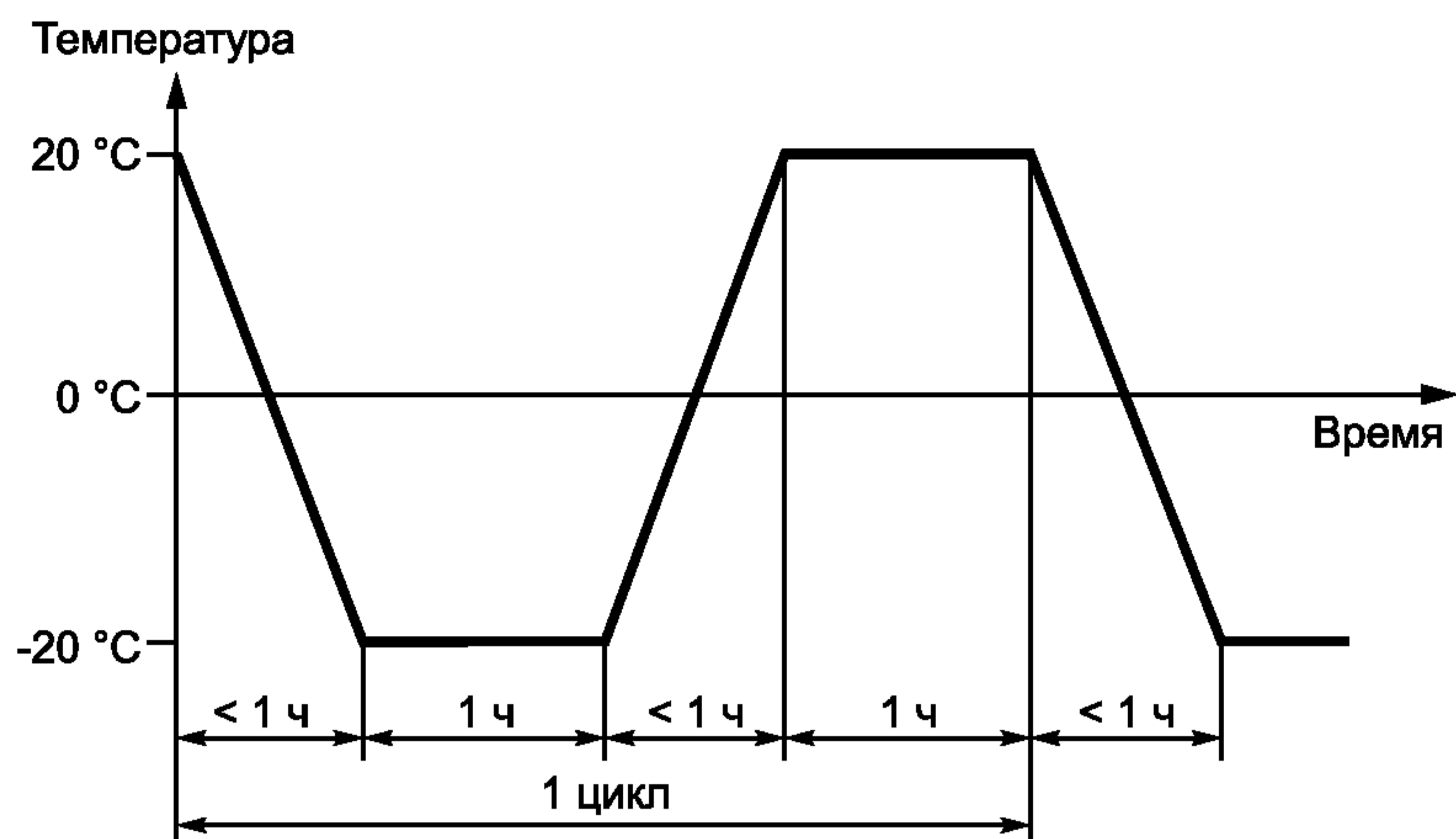
Рисунок 2 — Продолжительность одного цикла испытания
