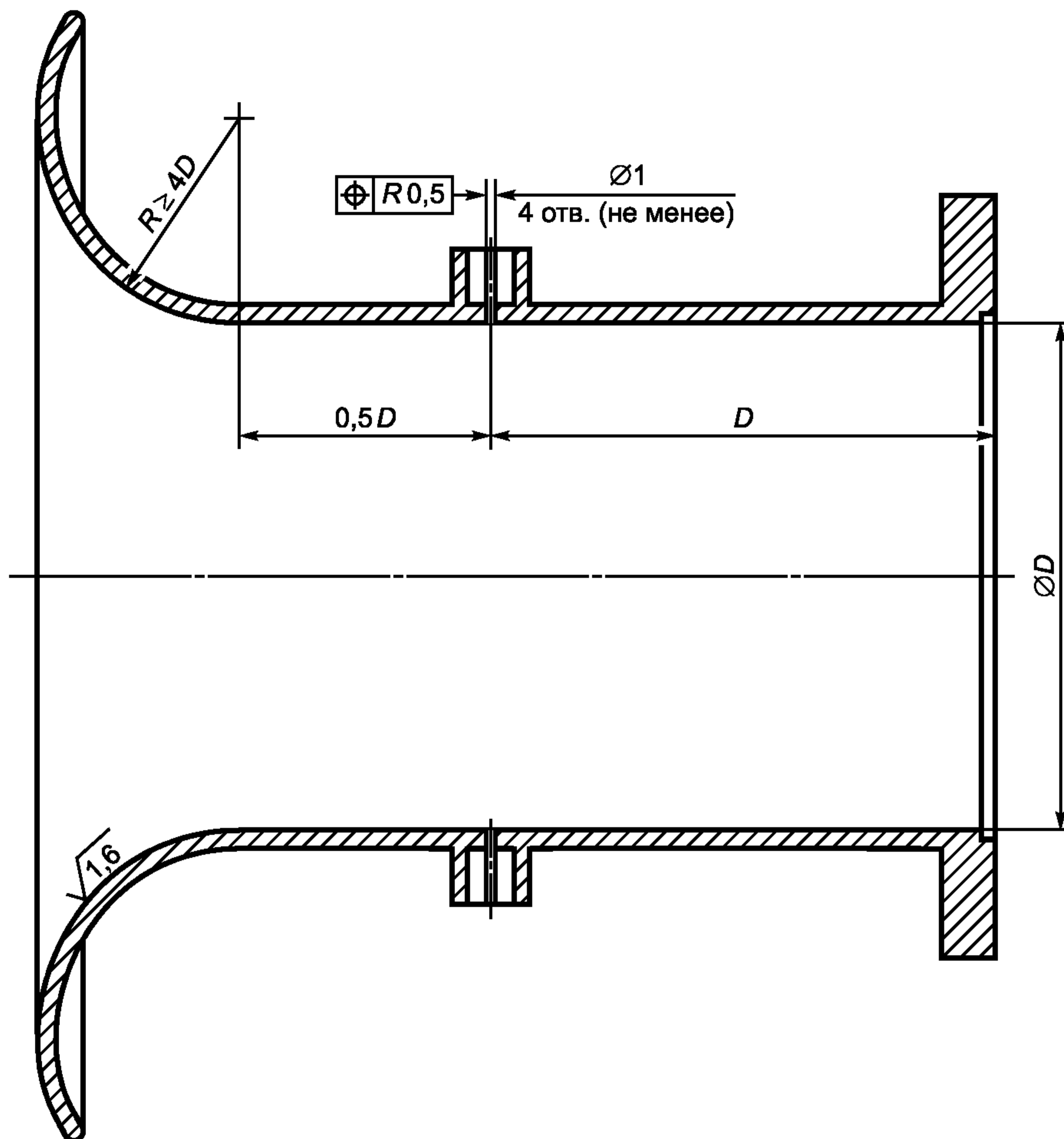
Рисунок 1 — Коллектор для измерения расхода воздуха
