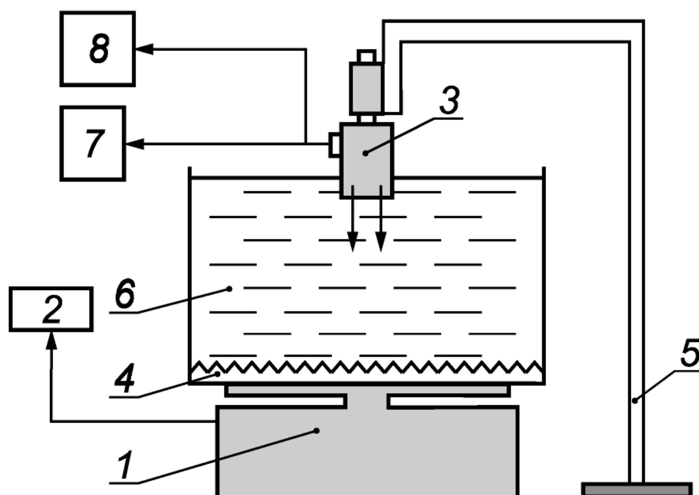
Рисунок F.4 — Компонетка С с поглощающей мишенью:
