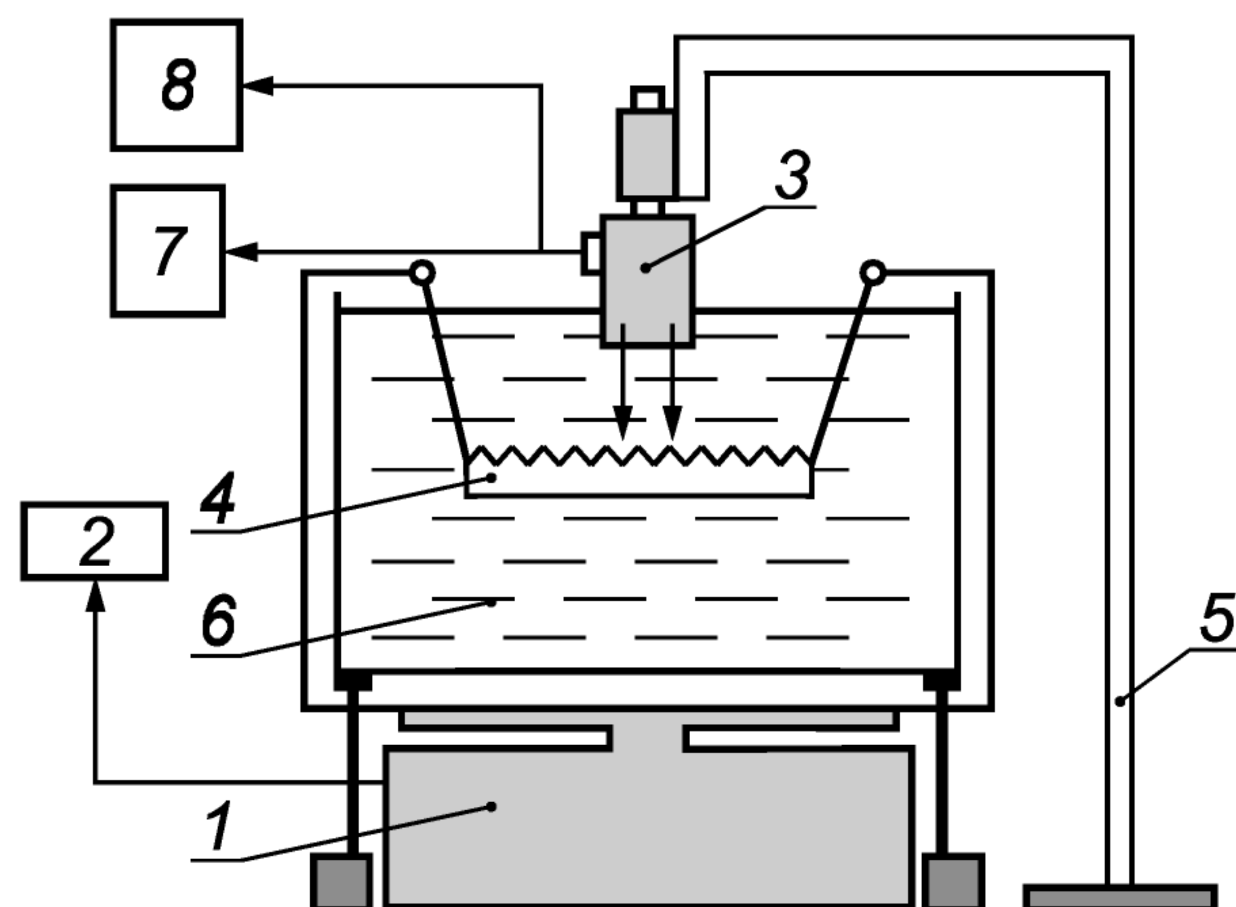
Рисунок F.3 — Компонетка В с поглощающей мишенью:
