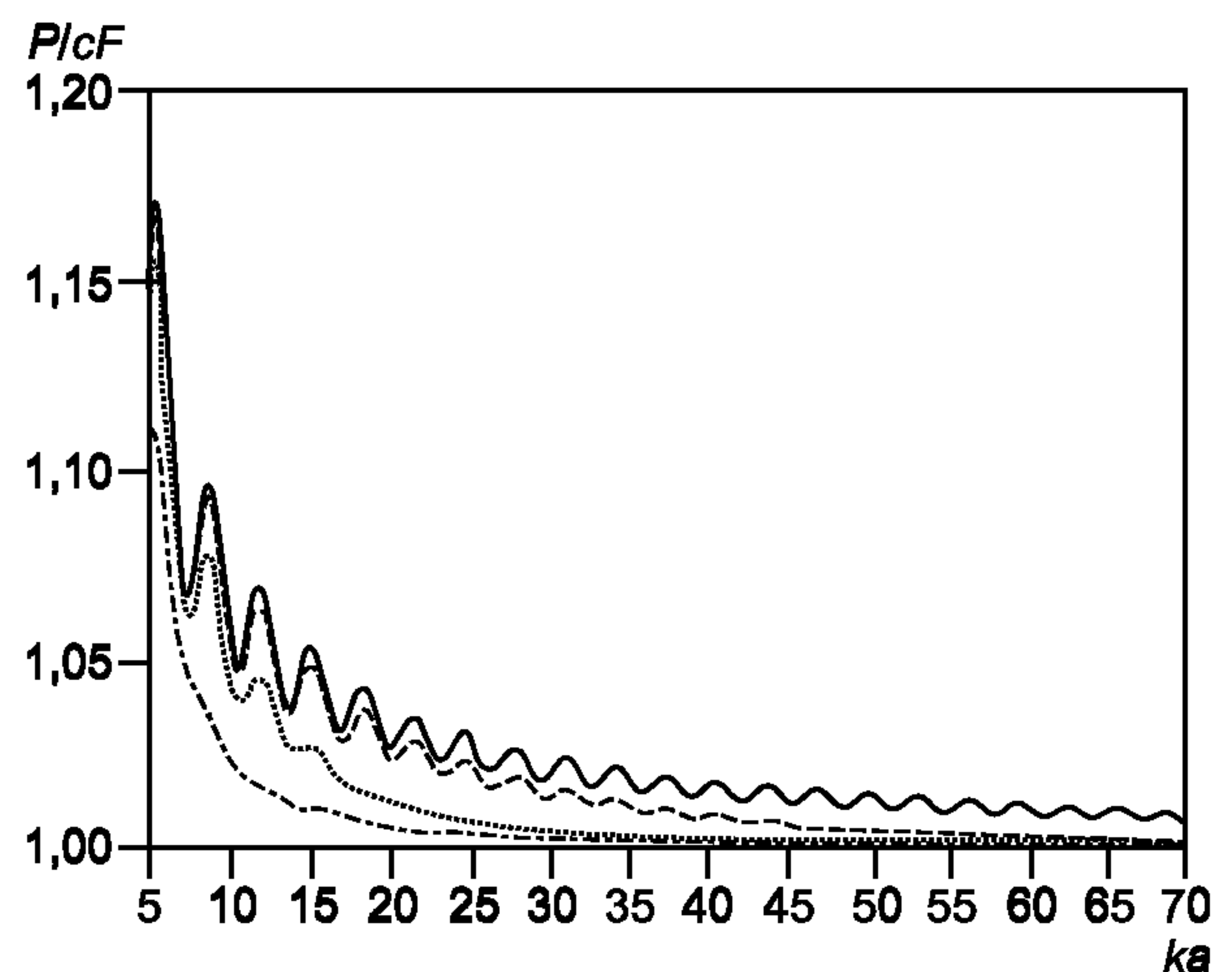
Рисунок Е.2 — Зависимость P/cF от ka для четырех различных псевдотрапециевидных амплитудных распределений: для \varepsilon = 0 (поршень) (сплошная кривая), \varepsilon = 0,1 (штриховая), \varepsilon = 0,25 (точечная), \varepsilon = 0,6 (штрихпунктирная)
