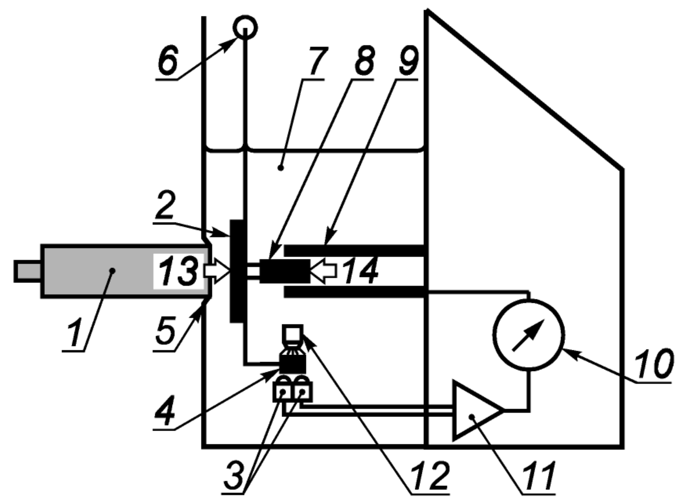
Рисунок F.7 — Компоновка F с поглощающей мишенью:
