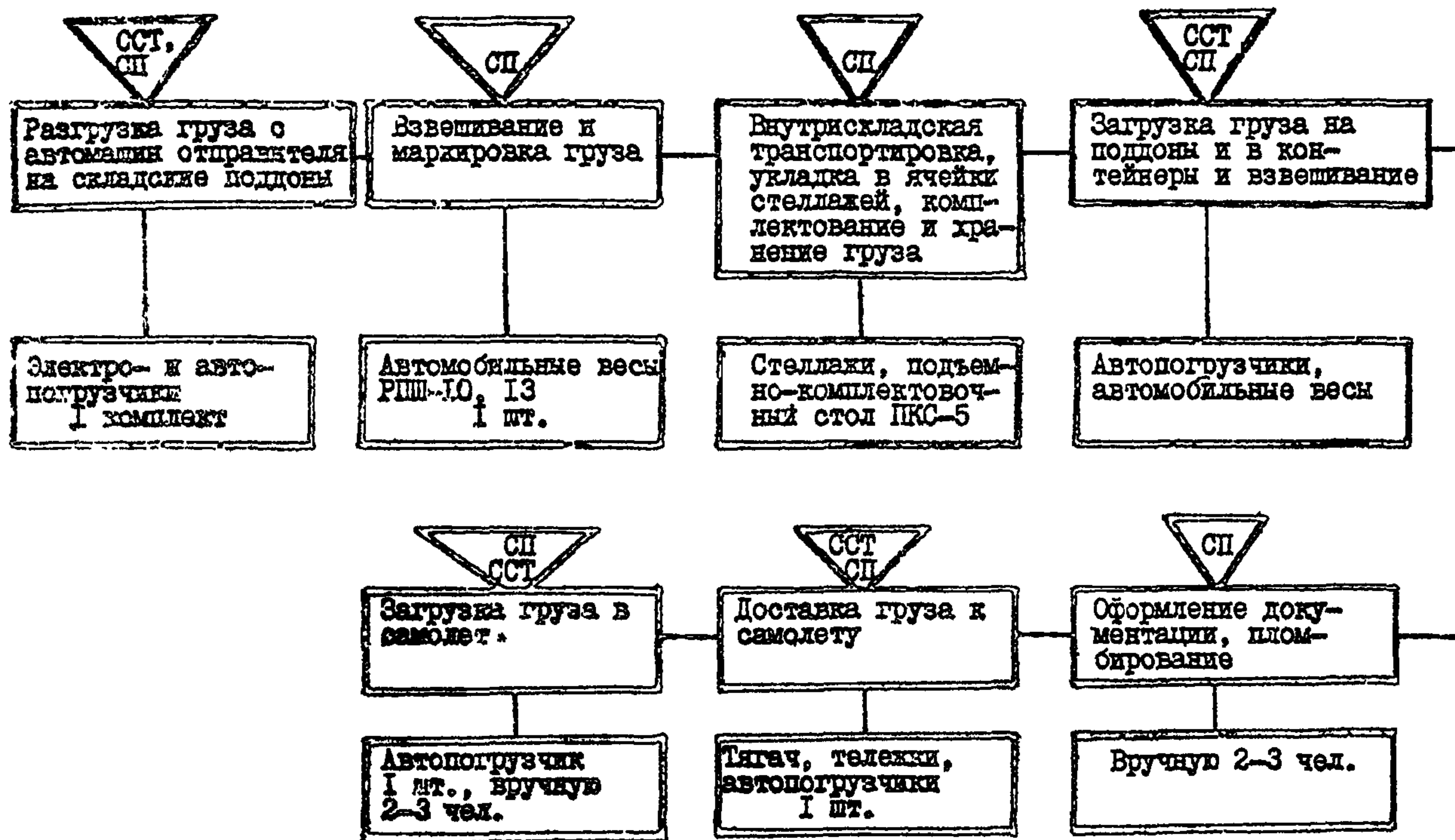
Рис. 6. Принципиальная технология обработки грузов, прибывших из города
