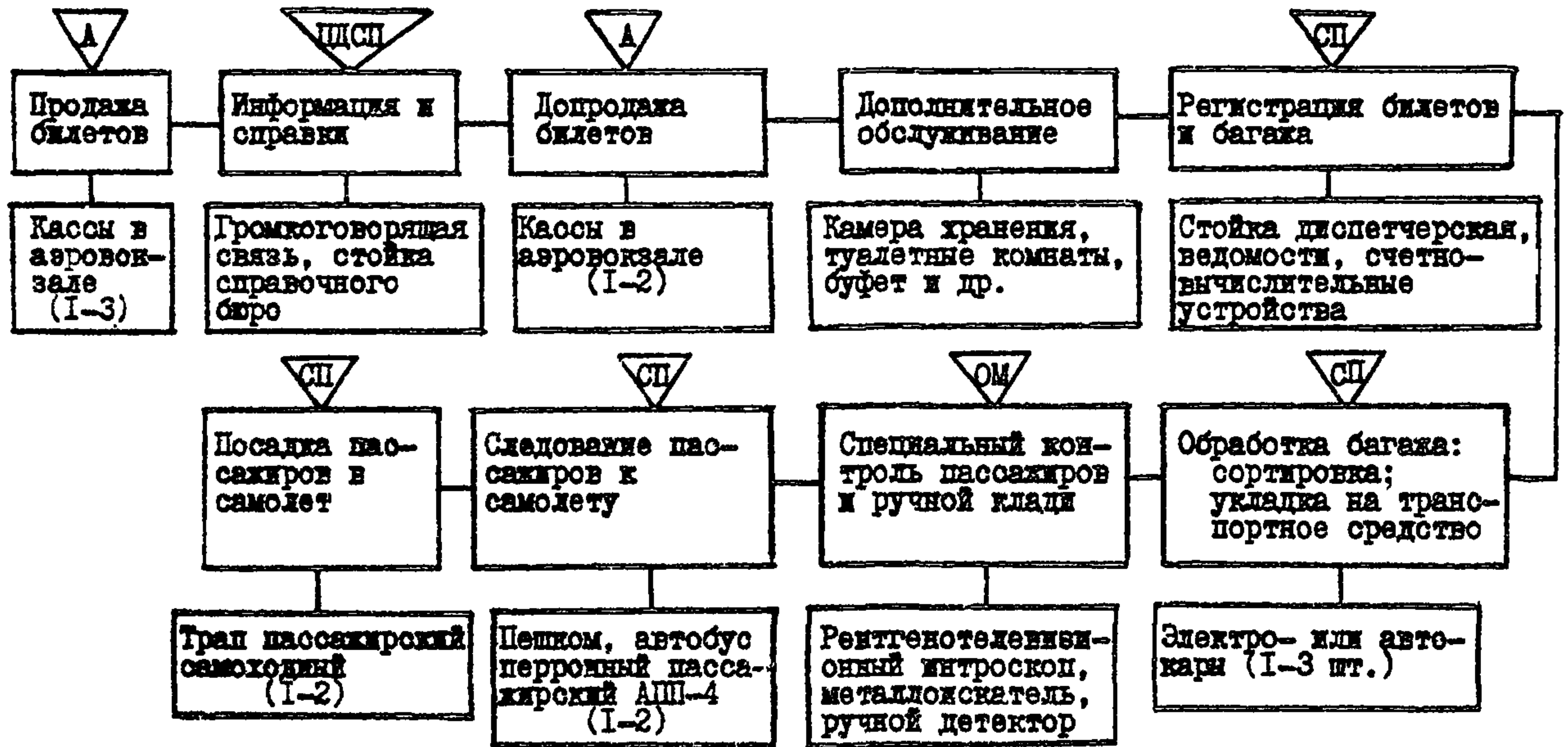
Рис. 3. Принципиальная схема обслуживания вылетающих пассажиров в аэропортах местных воздушных линий. Основной метод
