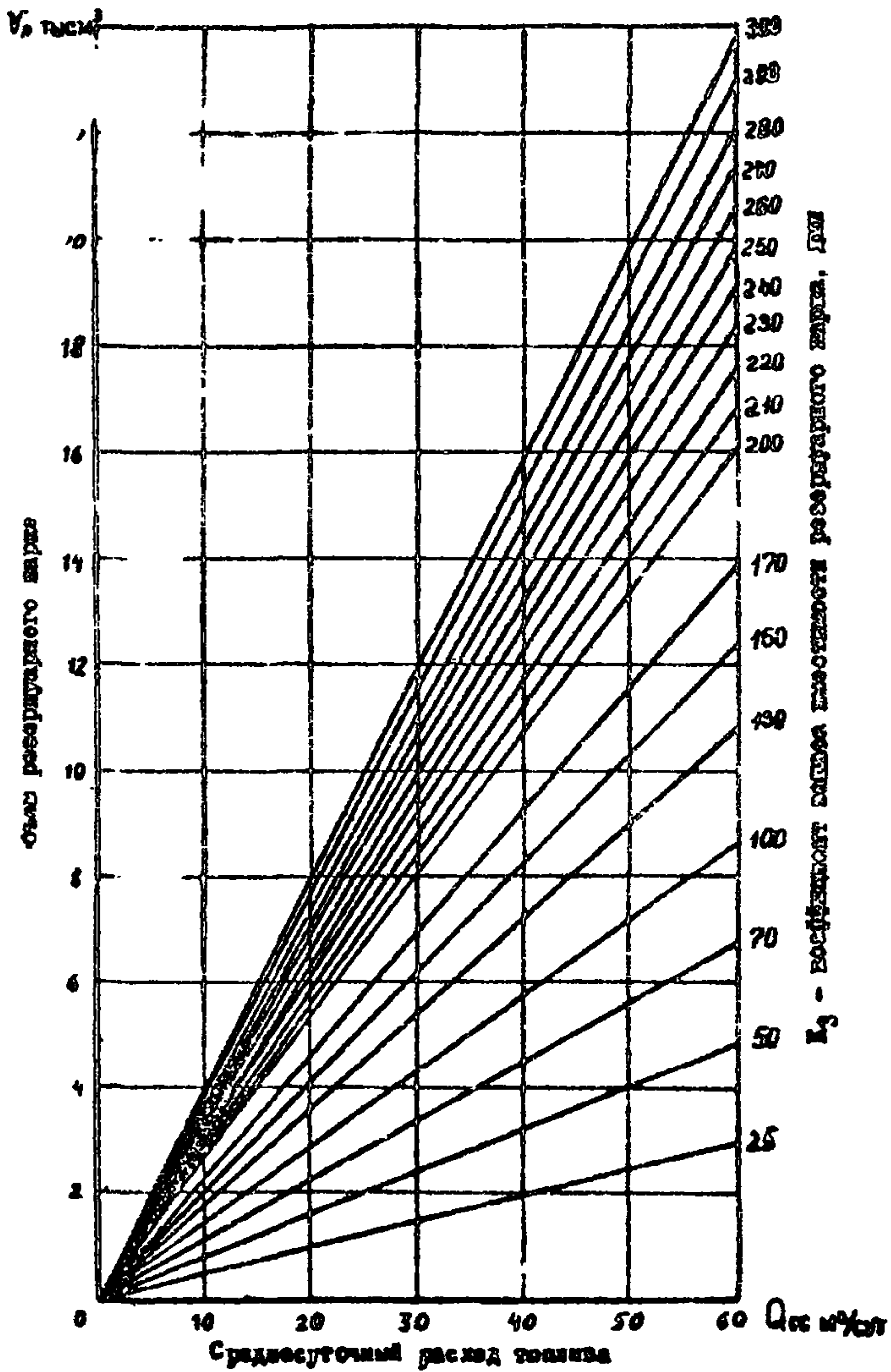
Рис. 12. График определения объема резервуарного парка при доставке топлива в аэропорт водным транспортом
