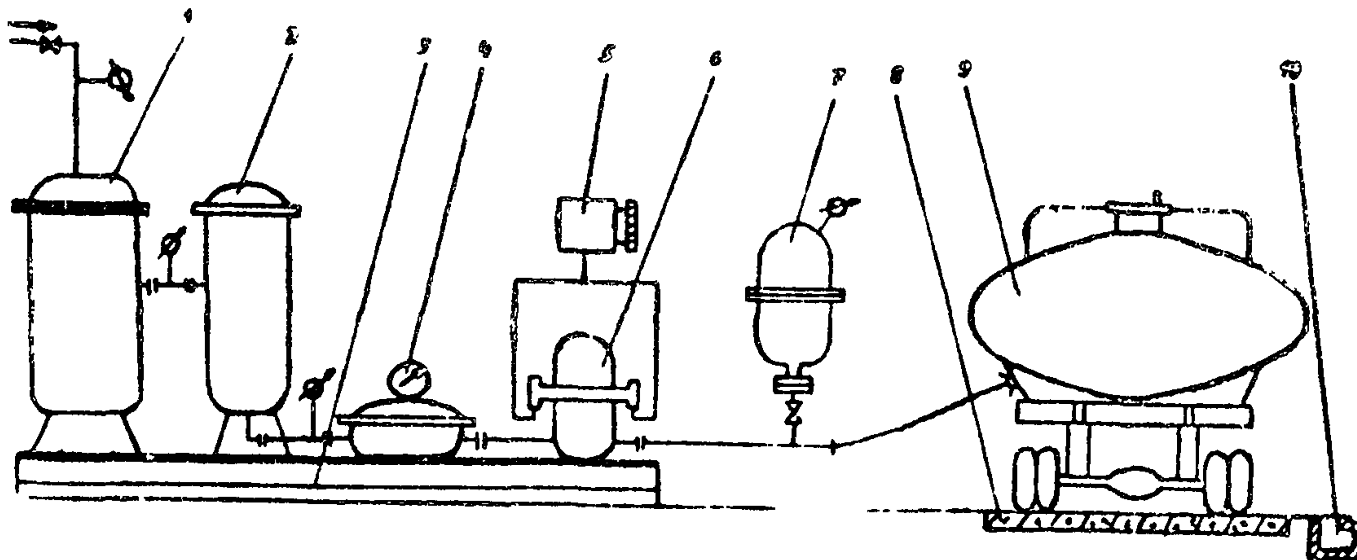
Принципиальная схема пункта налива: 1-фильтр-сепаратор; 2-фильтр с ТФБ; 3-рама; 4-счетчик топлива; 5-бак с ЦВК жидкостью; 6-дозатор; 7-гидроамортизатор; 8-площадка для ТЗ; 9-ТЗ; 10-сборник пролитого топлива
