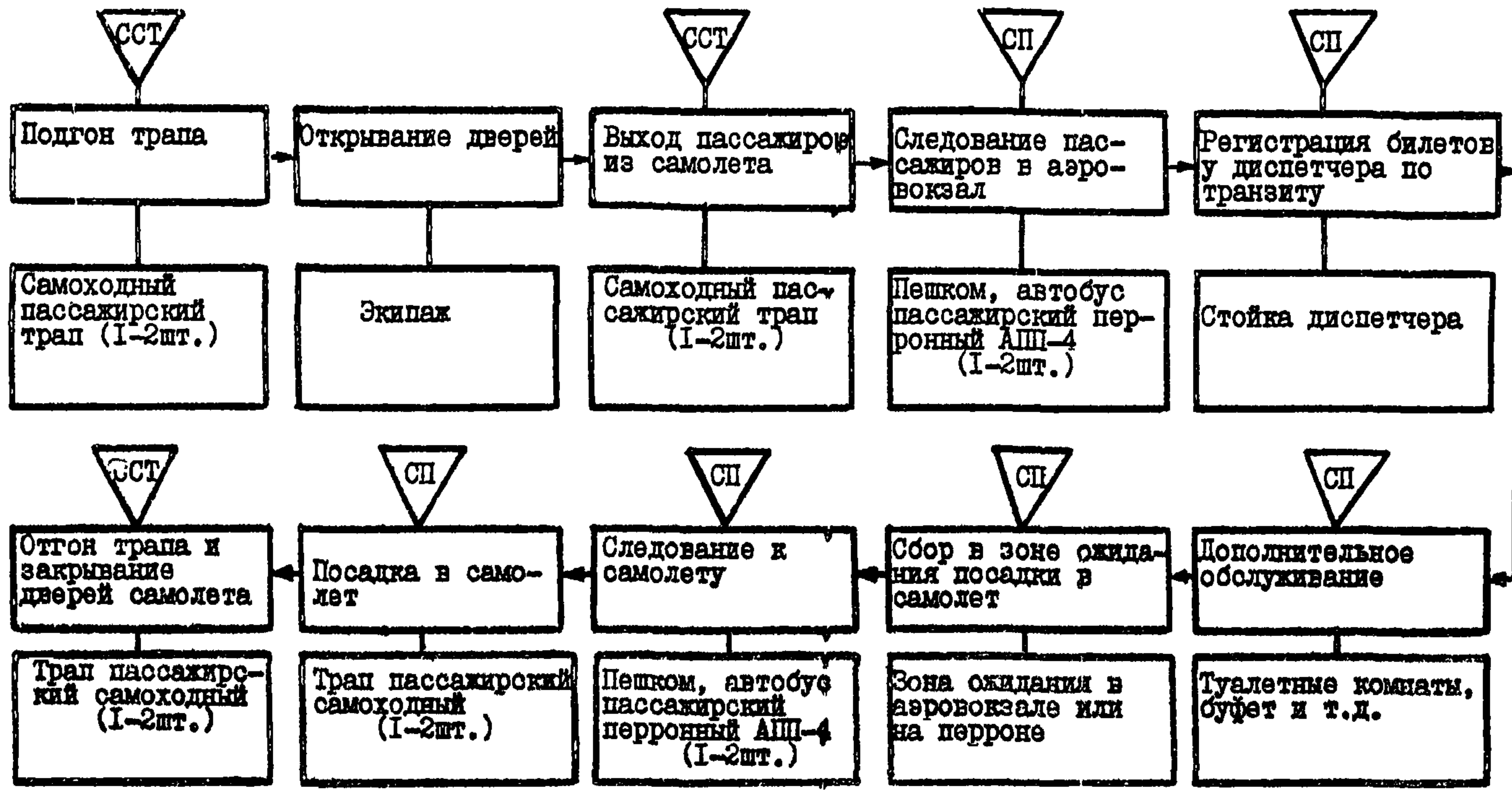
Рис. 2. Принципиальная схема обслуживания транзитных (трансферных) пассажиров
